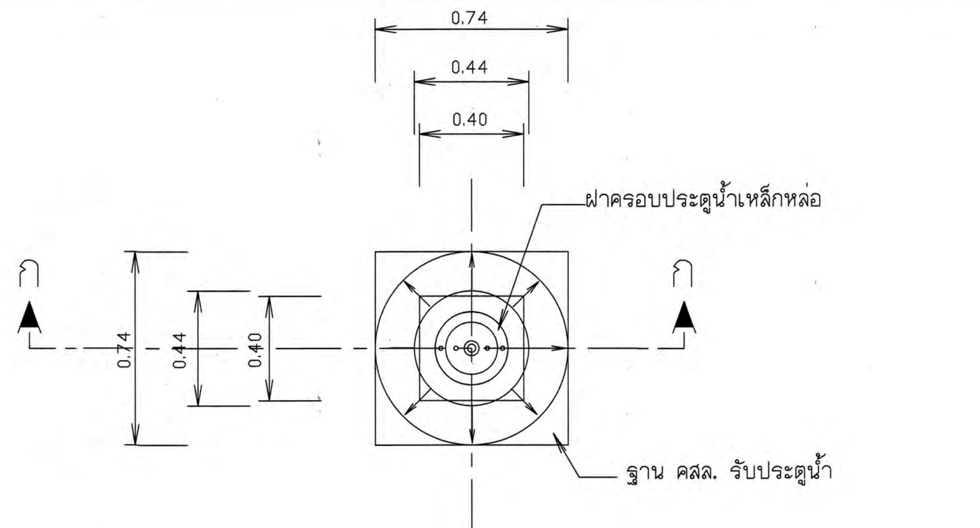
แปลนแสดงจุดติดตั้งประตูกวควบคุมท่อจ่ายน้ำ ขนาด 315 มม.
