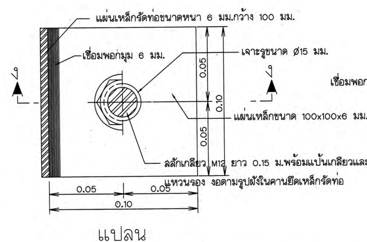
รายละเอียดแผ่นเหล็กยัดท่อ
