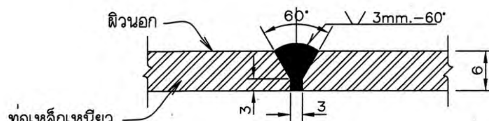
รูปขยายรอยเชื่อมท่อ ไม่แสดงมาตรฐาน
