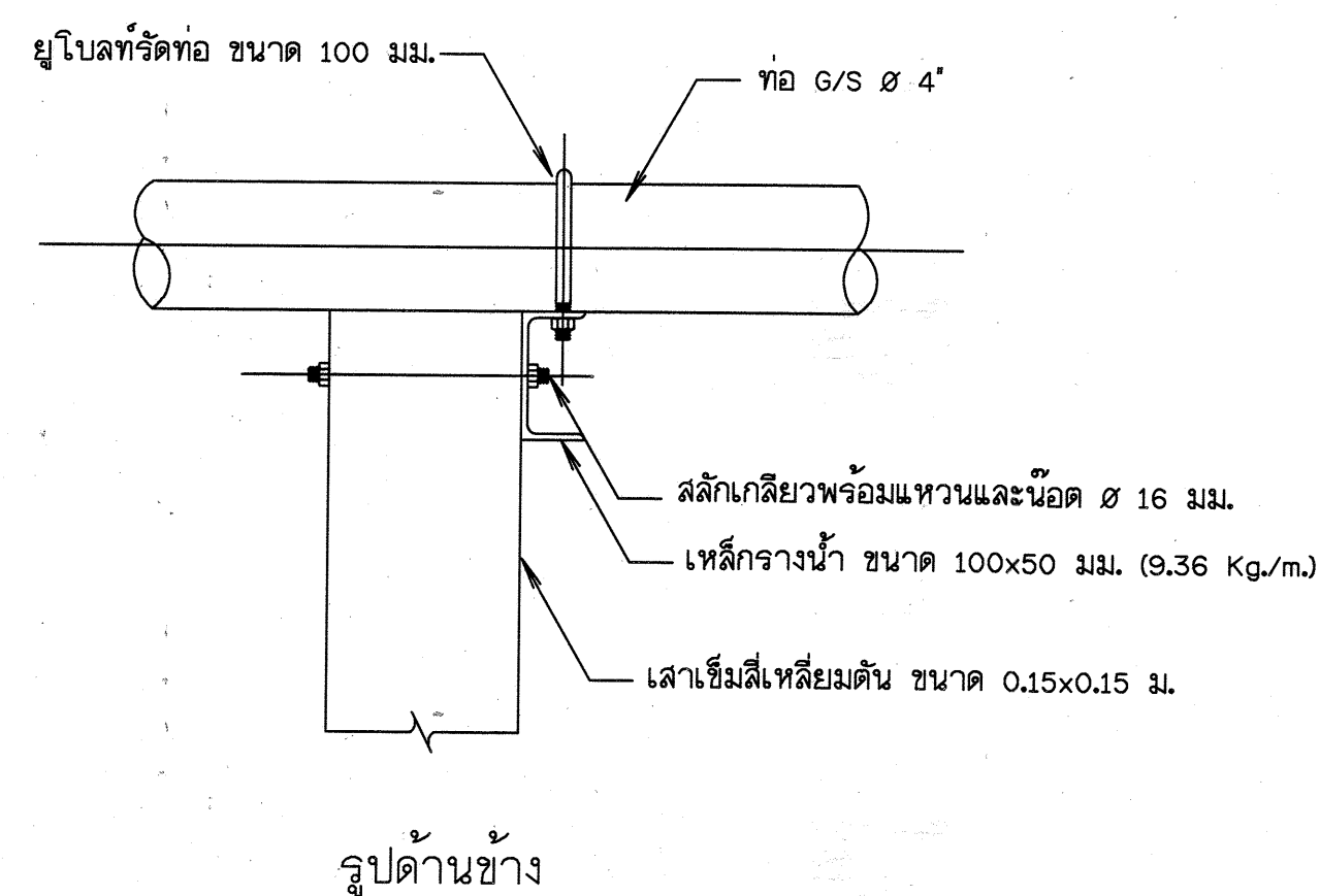
13. เสาค้ำรองรับท่อวัด และแบบขยายอุปกรณ์วัดท่อ ไม่แสดงมาตราส่วน
