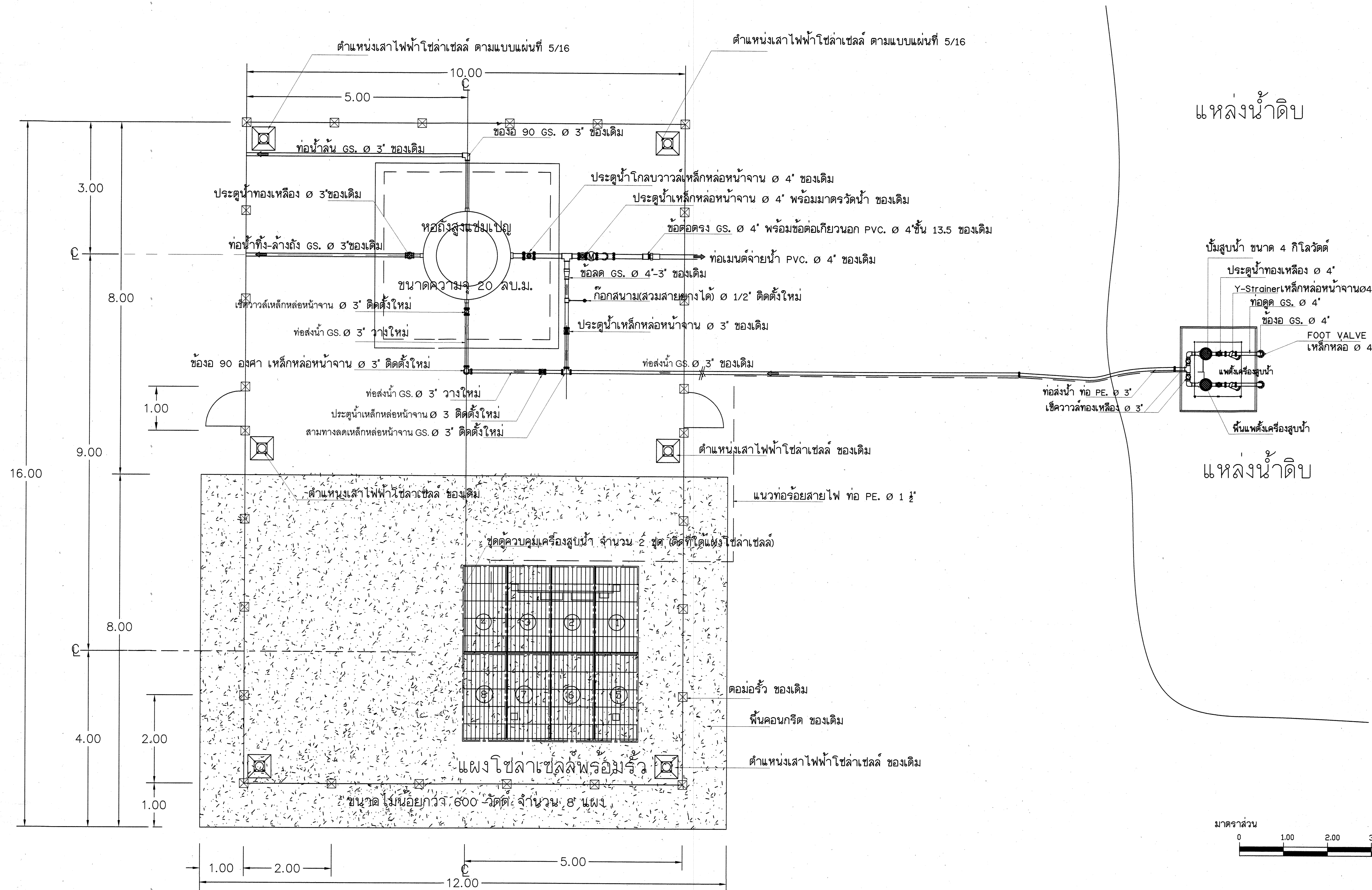
แบบแสดงผังตำแหน่งสิ่งก่อสร้างและการประสานท่อภายในระบบ Scale 1:100
