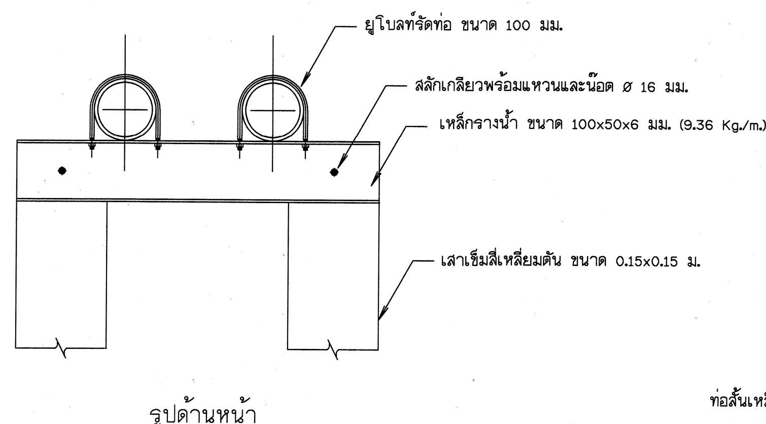
13. เสาคอมมูริบท่อดูด และแบบขยายอุปกรณ์รัดท่อ ไม่แสดงมาตราส่วน
