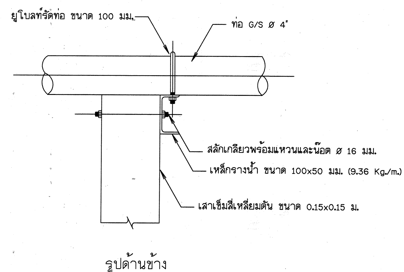
13. เสาคอมมูริบท่อดูด และแบบขยายอุปกรณ์รัดท่อ ไม่แสดงมาตราส่วน
