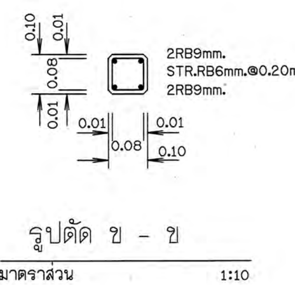
รูปตัด ข - ข มาตราส่วน 1:10
