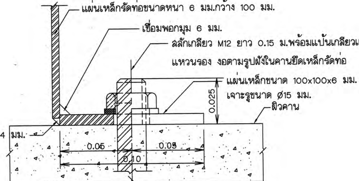
รูปตัด ง-ง
