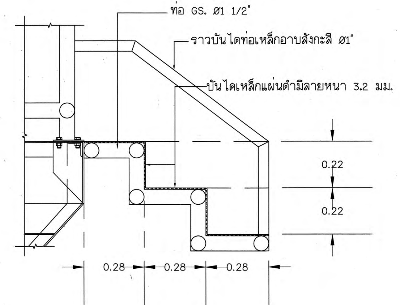
รูปขยายบันได ไม่แสดงมาตราส่วน
