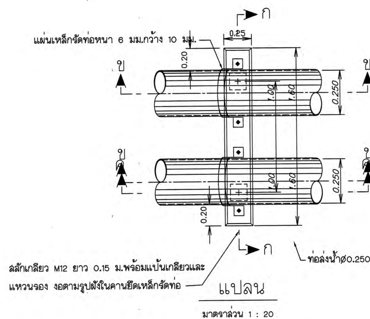
แบบแปลน
