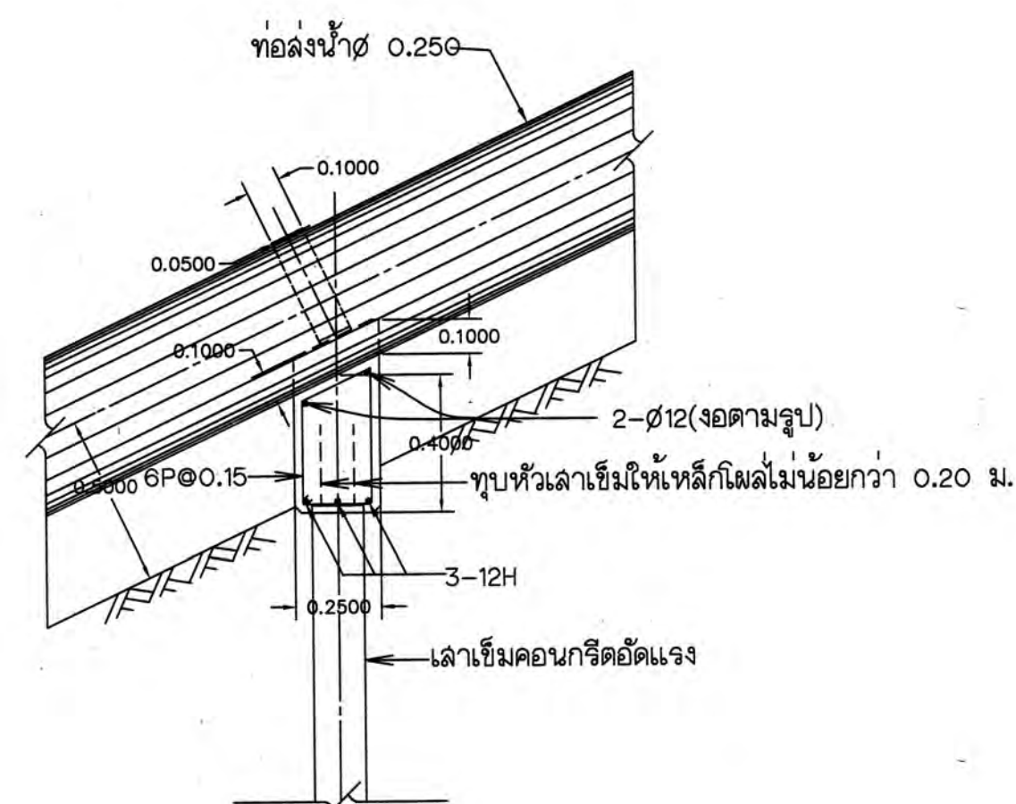
รูปตัด ข-ข
