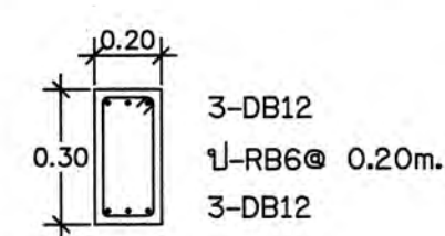
แบบขยายโครงสร้างคานรั้ว (BE)
