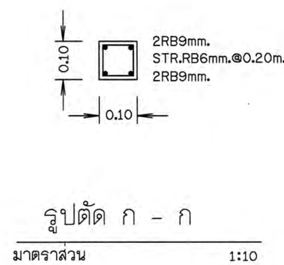
รูปตัด ก - ก มาตราส่วน 1:10
