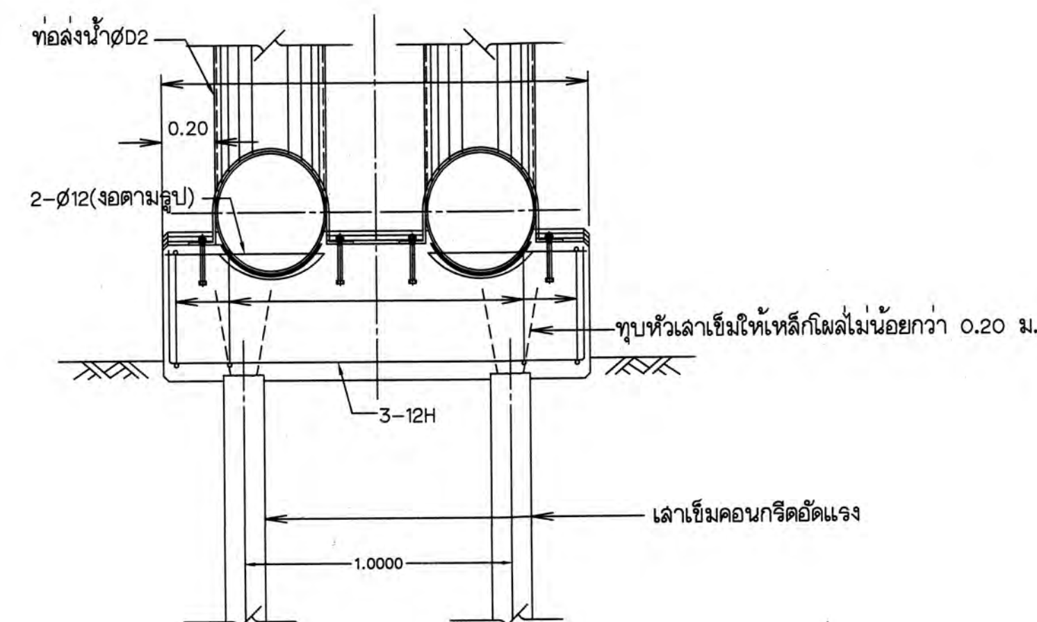
รูปตัด ก-ก
