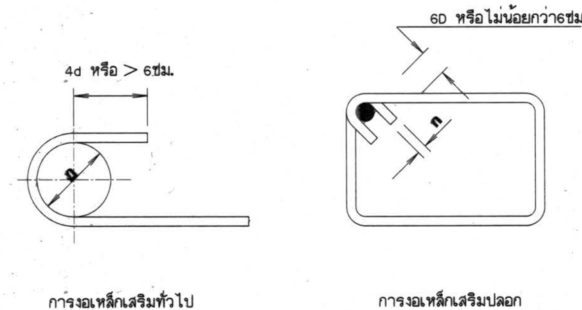
แสดงการติดตั้งเหล็กเสริม มาตราส่วน 1:20
