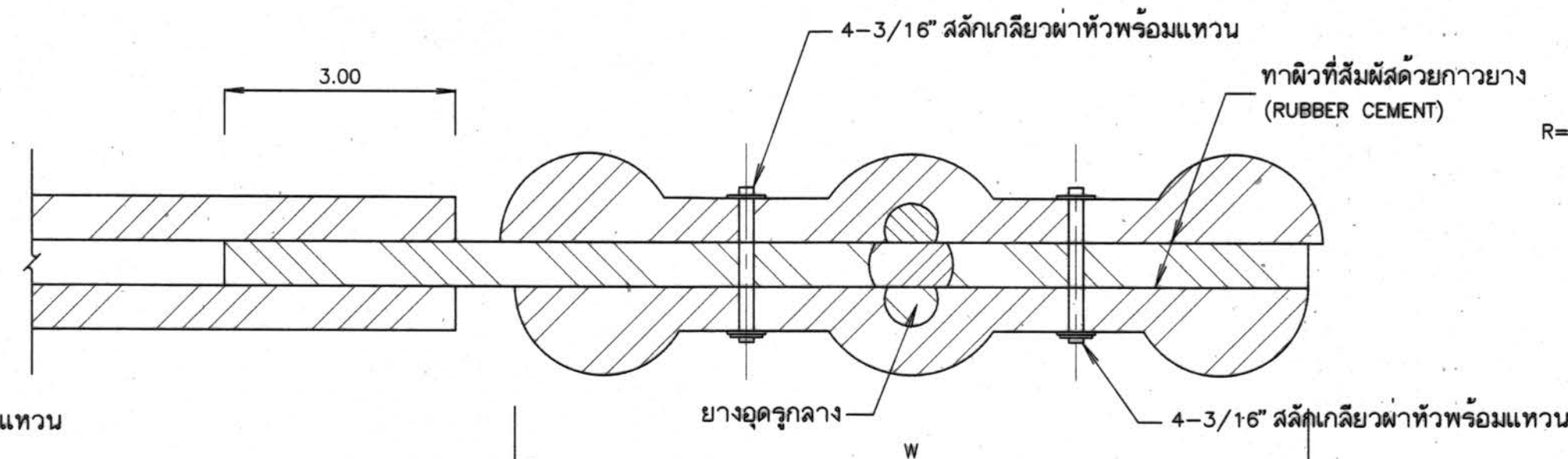
รูปตัด น-น ไม่แสดงมาตราส่วน
