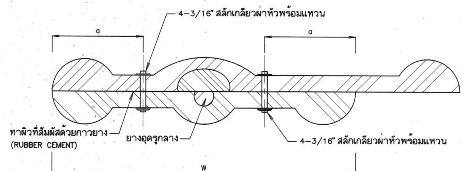
รูปตัด ท-ท ไม่แสดงมาตราส่วน
