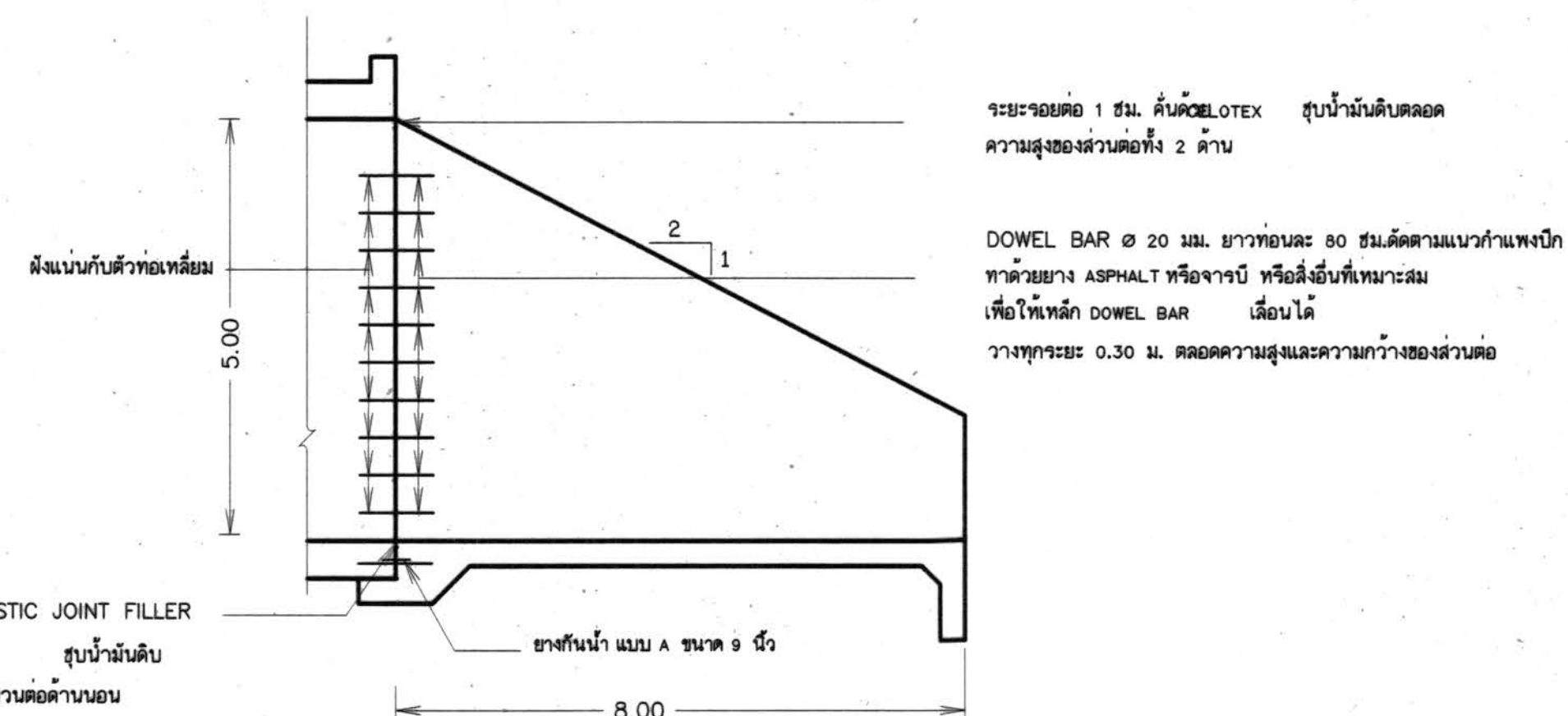
แบบขยายรอยต่อ เสริมเหล็กเดือย 1:75
