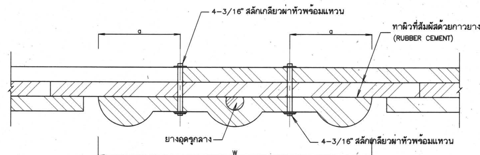
รูปตัด บ-บ ไม่แสดงมาตราส่วน
