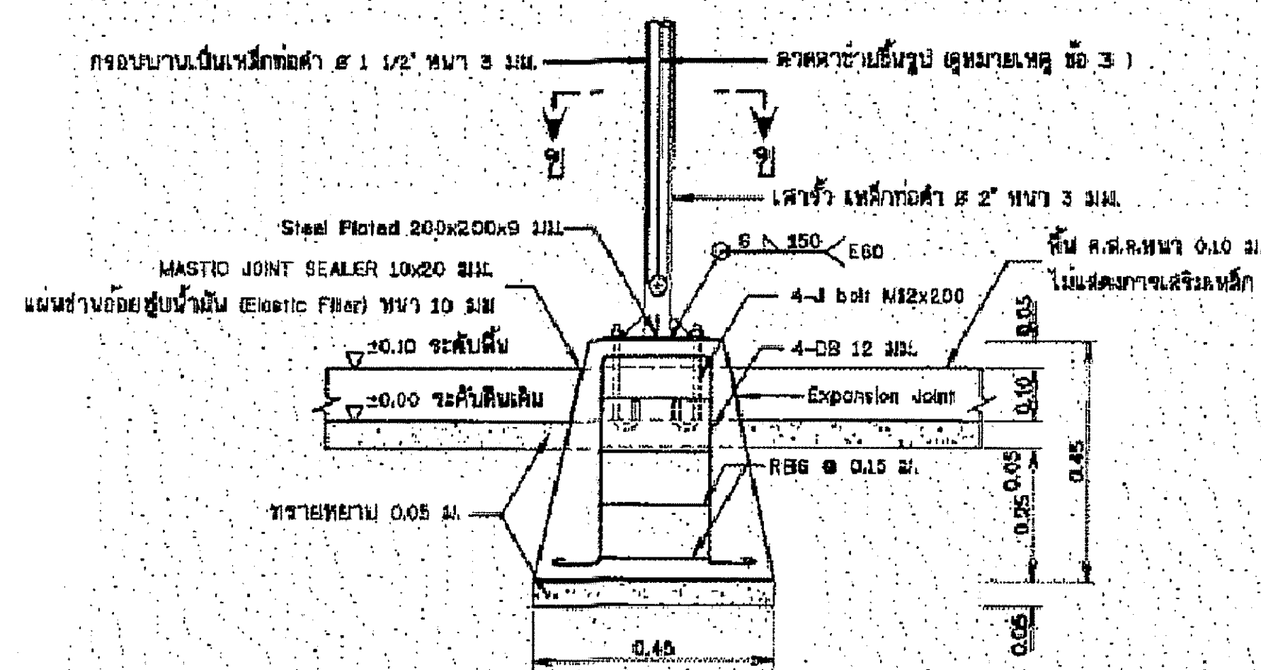
รูปขยายฐานจากโครงสร้างรับแผง F1 (คานา คสล. ท่อดำรับรูปหล่อคานาดัง) ไม่แสดงมาตราส่วน
