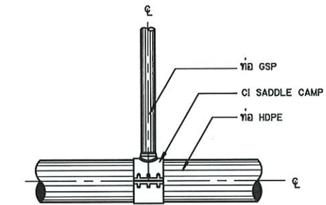
การบรรจุท่อสามทาง HDPE กับท่อ GSP แบบ CI SADDLE CLAMP (สำหรับอาคารจุดปล่อยน้ำ อาคารประจําขยะตอน อาคารระบายอากาศ กรณีท่อส่งน้ำขนาดเส้นผ่าศูนย์กลางน้อยกว่าหรือเท่ากับ 315 มม.)
