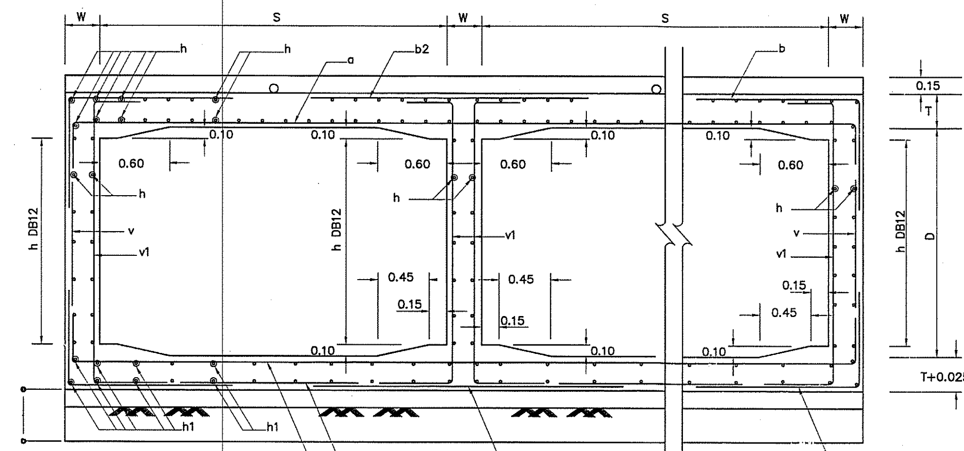
รูปตัด (ก) - (ก) NOT TO SCALE
