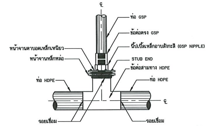
การบรรจุท่อสามทาง HDPE กับท่อ GSP แบบข้อต่อ (สำหรับอาคารจุดปล่อยน้ำ อาคารประจําขยะตอน อาคารระบายอากาศ กรณีท่อส่งน้ำขนาดเส้นผ่าศูนย์กลางมากกว่า 315 มม.)
