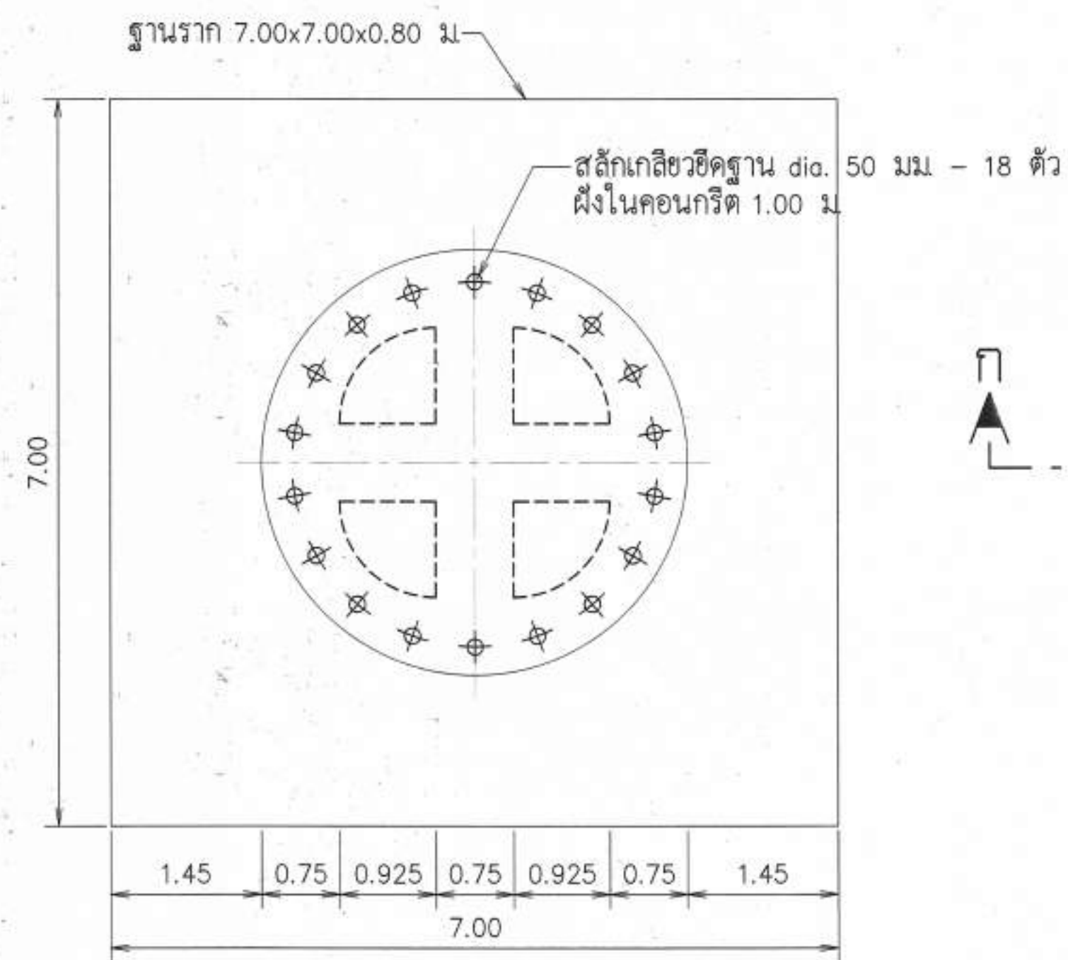
แปลนฐานรากหอดึงสูง (แบบเสาเข็ม) ไม่แสดงมาตราส่วน
