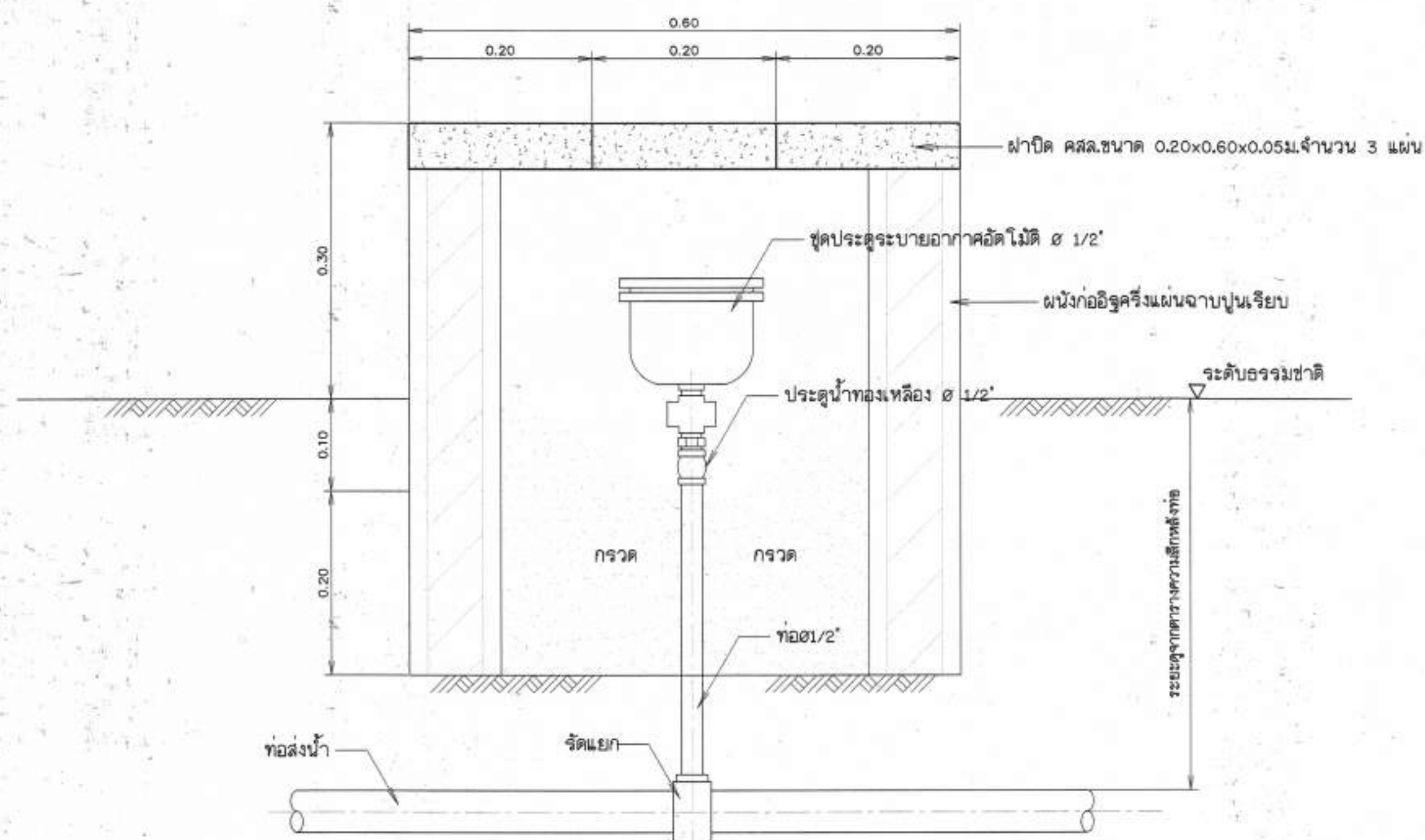
12 การติดตั้งประตูประบายอากาศอัตโนมัติ มาตราส่วน 1:5
