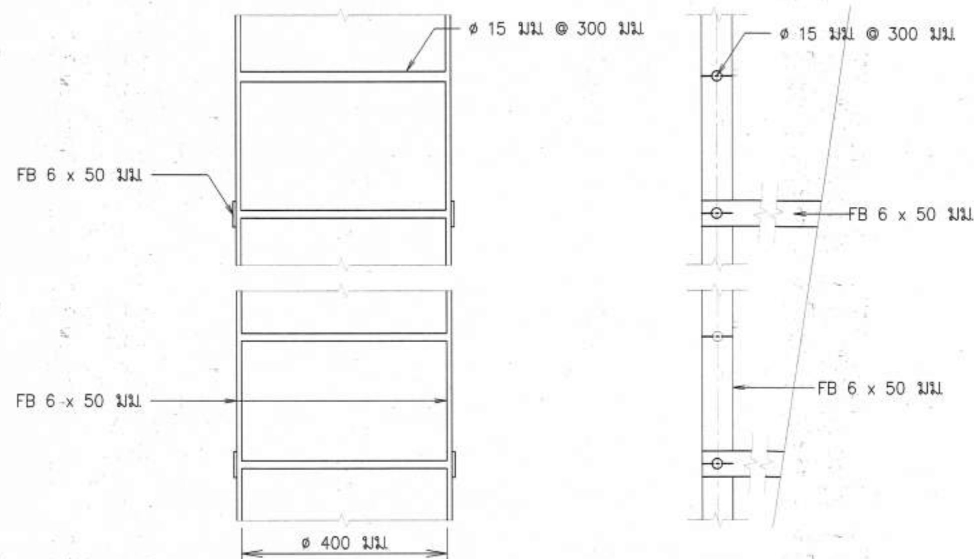
ภาพขยายบันได "1" ภายในห้องถึงเหล็กเก็บน้ำ ไม่แสดงมาตราส่วน
