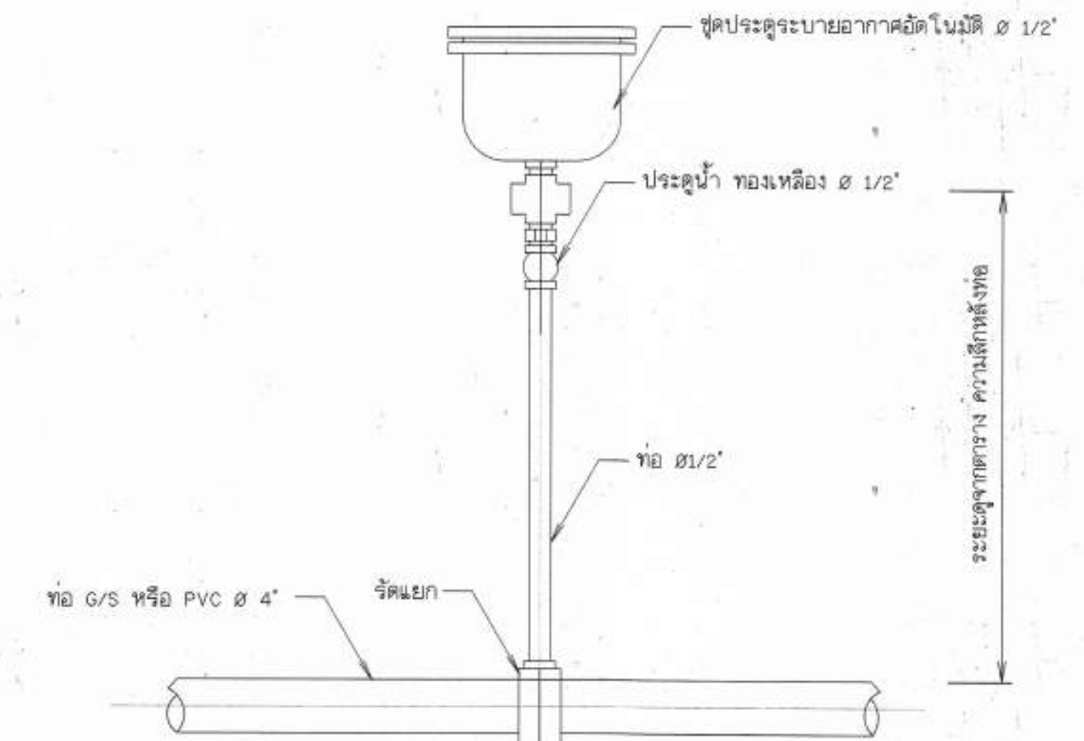
12. การติดตั้งประตูประบายอากาศอัตโนมัติ ไม่แสดงมาตราส่วน
