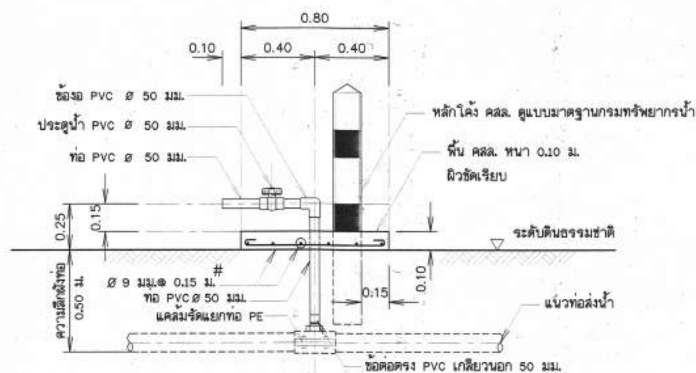
รูปตัด ก - ก แสดงการติดตั้งประตูจุดปล่อยน้ำ มาตราส่วน 1:20
