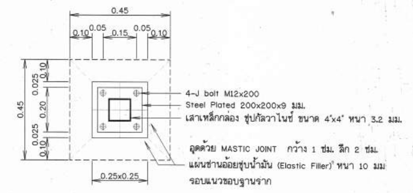
รูปตัด ก-ก ไม่แสดงขนาดราวล้วน
