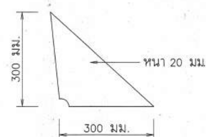
ภาพขยายหูช้าง จำนวน 12 ชิ้น โดยแบ่งระยะในการติดตั้งให้เท่ากัน
