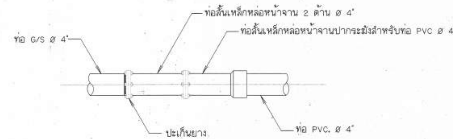
8. การบรรจุบล็อกลูกกลิ้ง G/S กับท่อ PVC. ไม่แสดงมาตราส่วน
