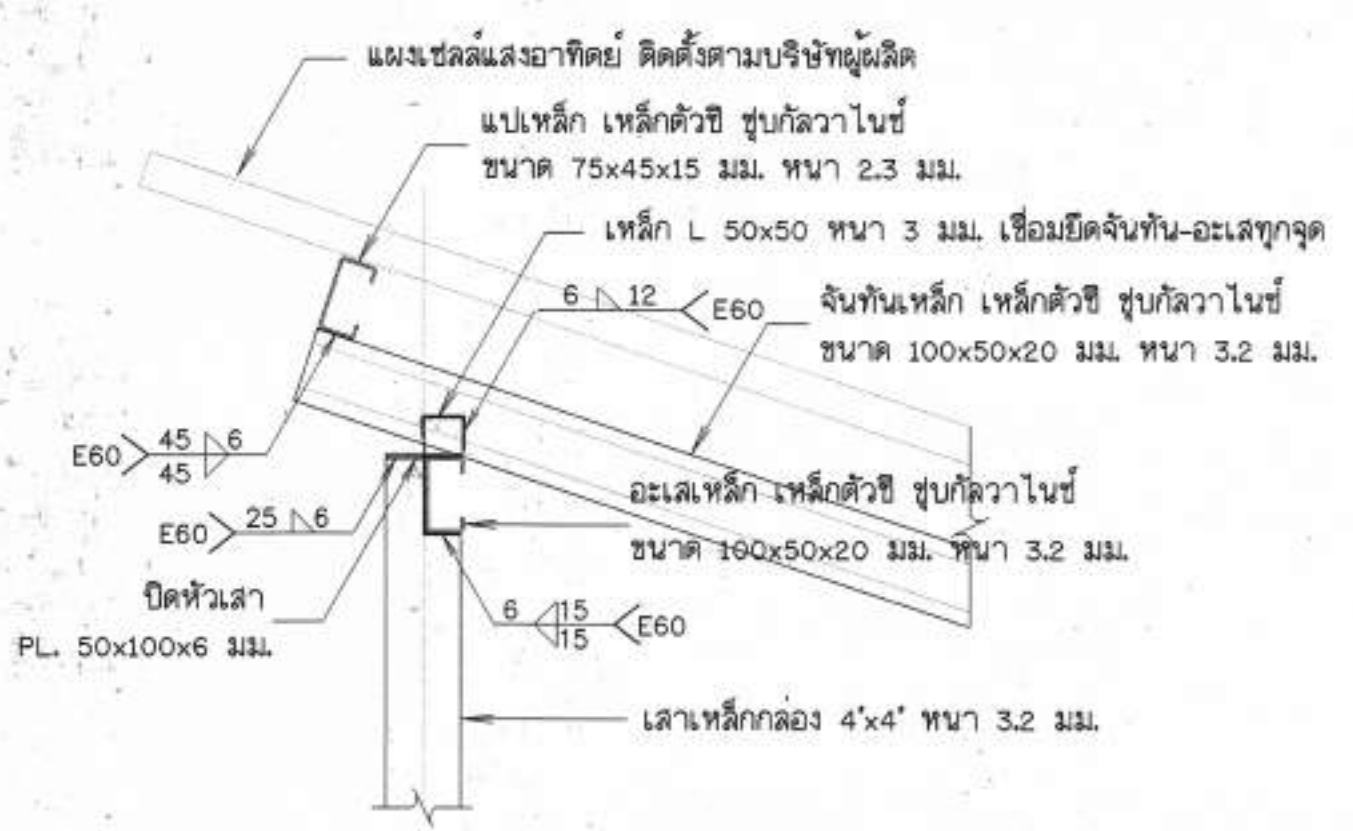
รูปขยาย การติดตั้งโครงหลังคา ไม่แสดงขนาดราวล้วน
