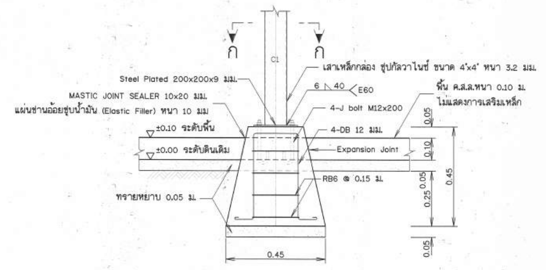
รูปขยายฐานรากโครงสร้างรับแฉ่ง F1 (ต่อม่อ คสล. หล่อสำเร็จรูปพร้อมติดตั้ง) ไม่แสดงขนาดราวล้วน
