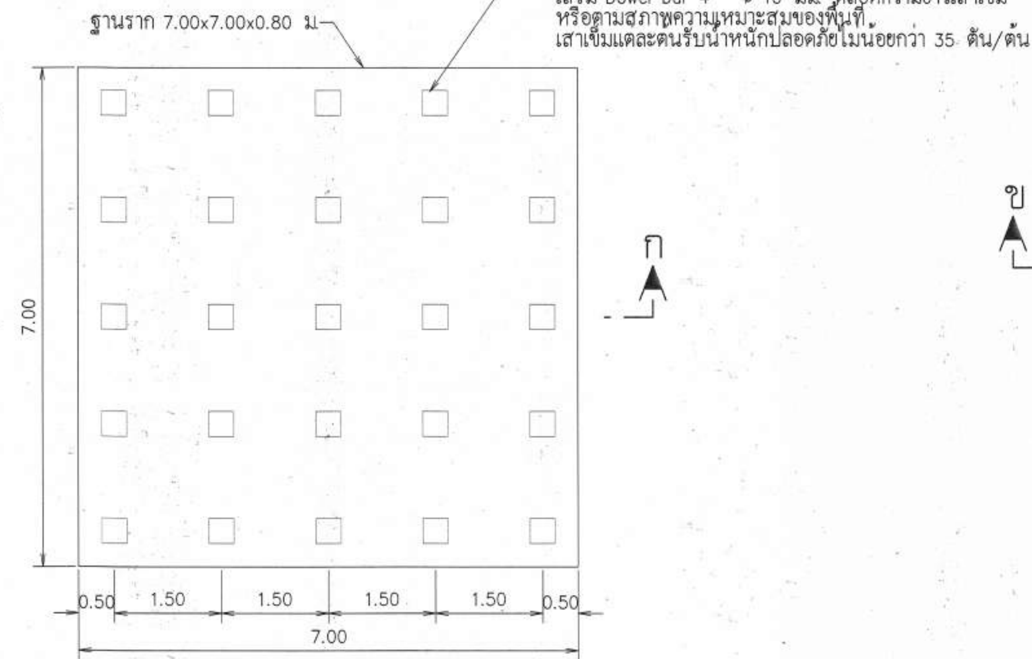
แปลนฐานรากหอดึงสูง (แบบเสาเข็ม) ไม่แสดงมาตราส่วน
