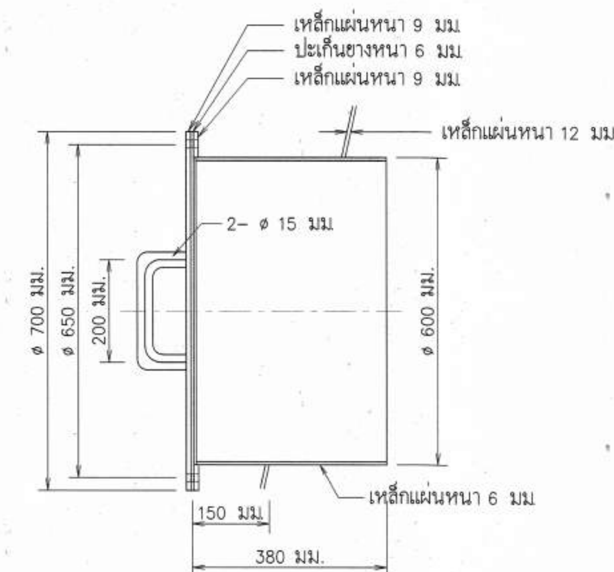
ภาพขยายทางคนเข้า-ออก "2" ไม่แสดงมาตราส่วน
