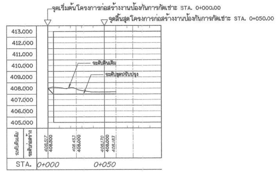
รูปตัดตามยาว ขนาดจาล้วน แนวนอน 1:1,000 แนวตั้ง 1:100
