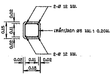
รูปตัด ข - ข ๙๐๙๑๑๐ 1:10
