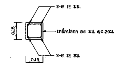
รูปตัด ก - ก ๙๐๙๑๑๐ 1:10
