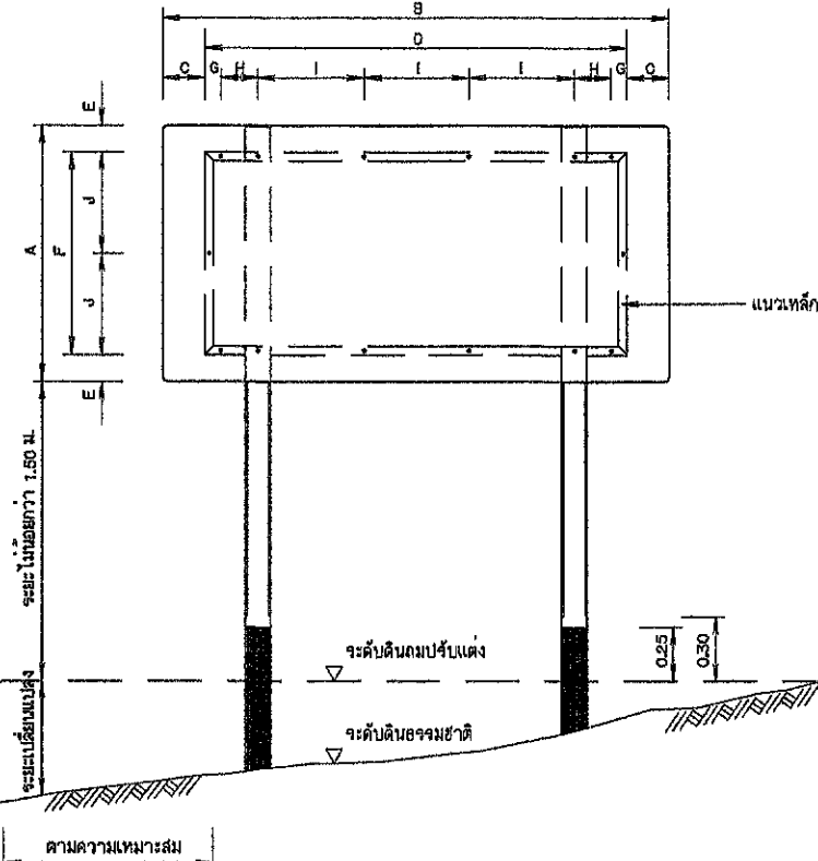
รูปแสดงการประกอบแผ่นป้าย ๙๐๙๑๑๐ 1:20
