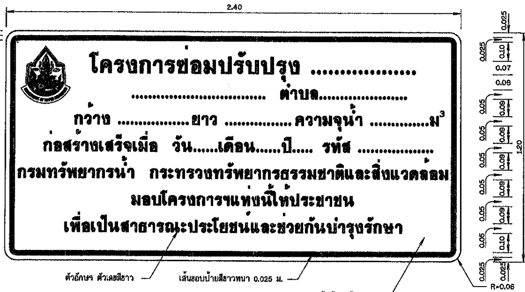
ป้ายโครงการ ๙๐๙๑๑๐ 1:10
