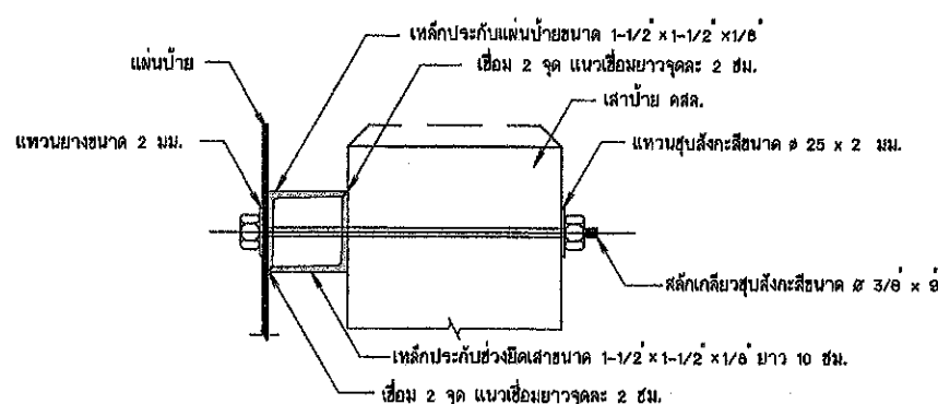
รูปตัดขยายการยึดแผ่นป้ายและเสา ๙๐๙๑๑๐ 1:20
