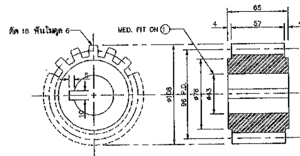
เฟืองเล็ก (เหล็กเหนียว)
