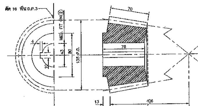
เฟืองดอกจอกเล็ก (เหล็กเหนียว)
