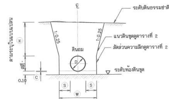
รูปตัดทั่วไปแสดงการวางท่อ มาตราส่วน 1:50
