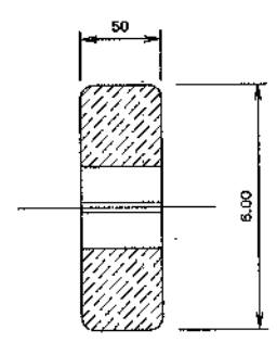
ล้อเหล็กหล่อ ASTM A 48 CLASS 30/MS G 5501 FC 20 มาตราส่วน 1:2.5
