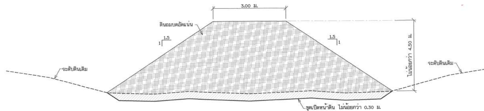
รูปแบบงานก่อสร้าง COFFERDAM ไม่แสดงมาตราส่วน
