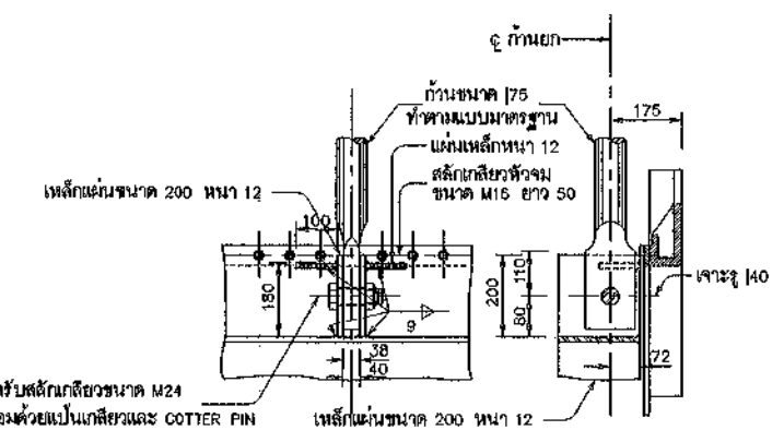
รูปตัด ค-ค มาตราส่วน 1:10
