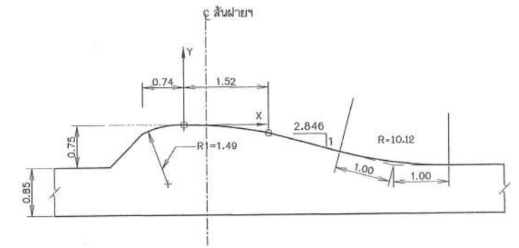
รูปขยายสัดส่วนสันฝายสูง 0.75 ม.
