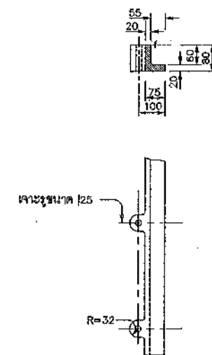
รูปขยายเหล็กนํ้าช่อง มาตราส่วน 1:10
