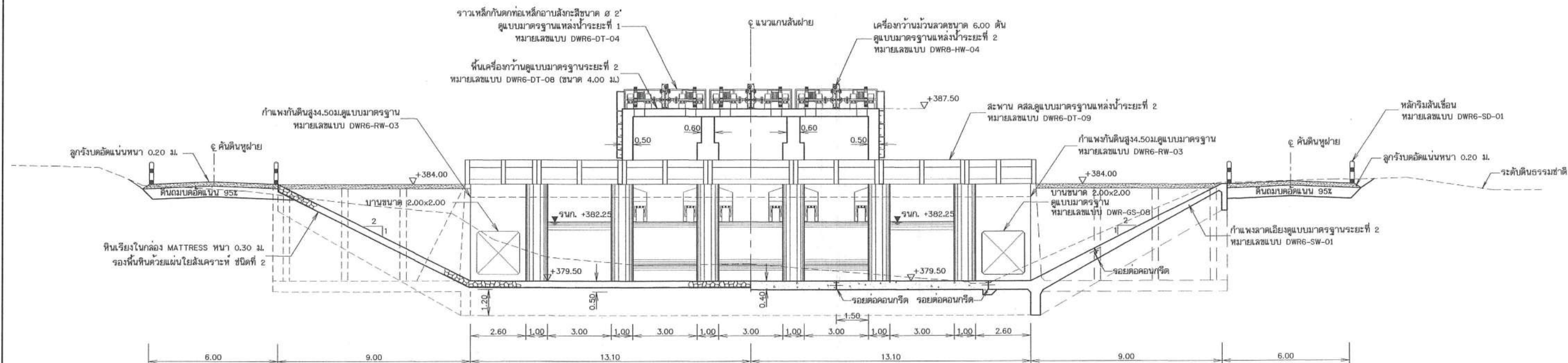
รูปตัด ค-ค
