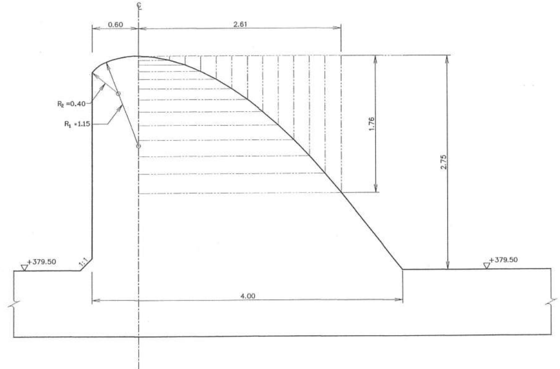
รูปขยายรายละเอียดโค้งฝายสันมนแบบไม่มีบานระบายควบคุม
