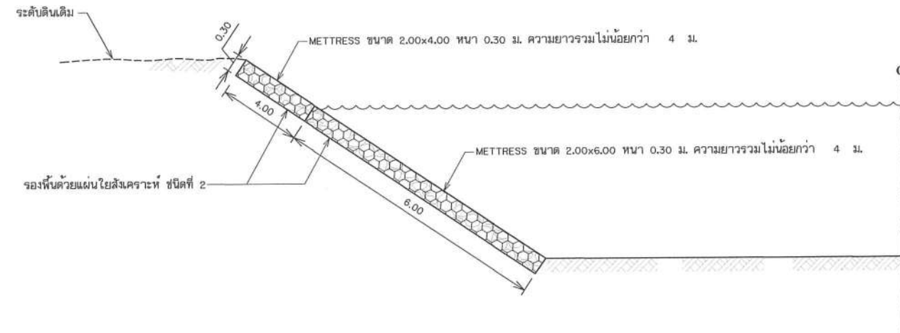
งานป้องกันการกัดเซาะท้ายฝาย ไม่แสดงมาตราส่วน
