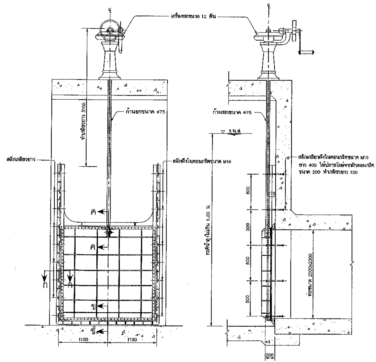
การประกอบ และติดตั้ง มาตราส่วน 1:25
