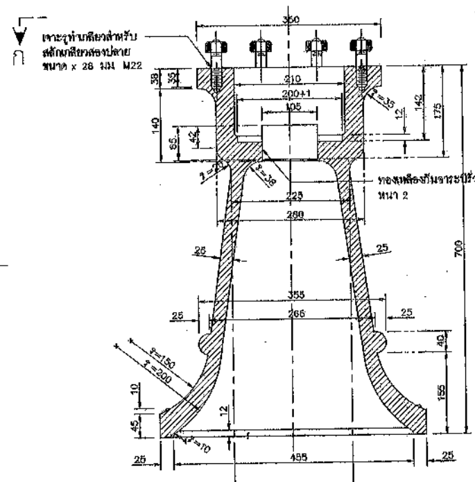
แท่น (เหล็กหล่อ)
