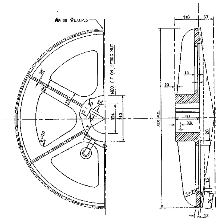
เฟืองดอกจอกใหญ่ (เหล็กหล่อ)
