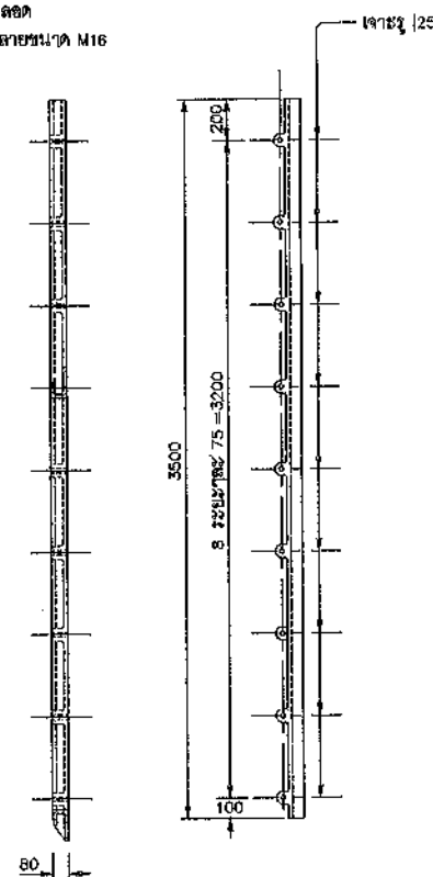
เหล็กหน้าร่อง เหล็กเหล็กรูป มาตราส่วน 1:20
