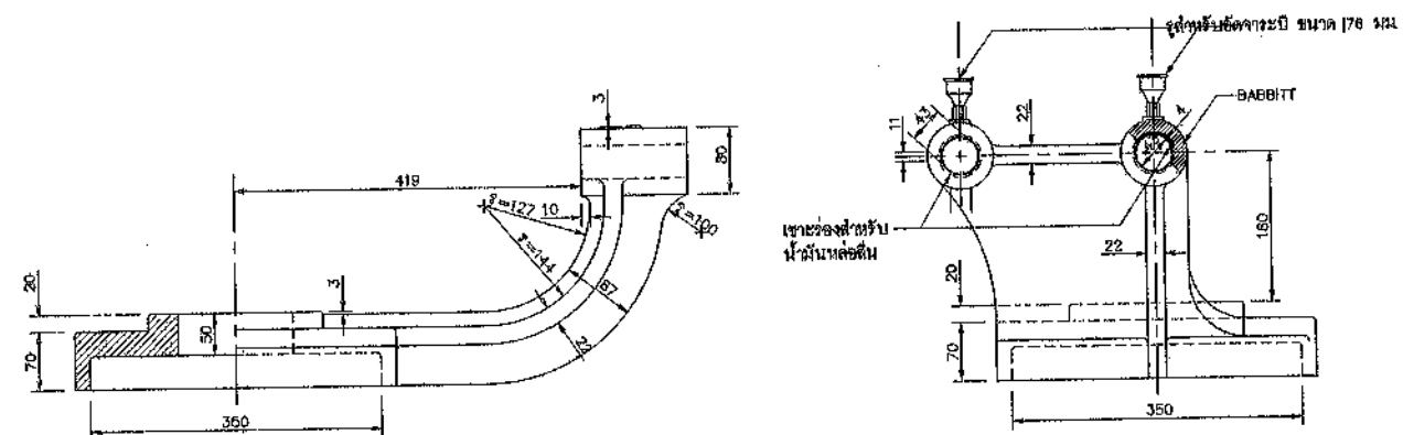
ฝาครอบและตุ๊กตา (เหล็กหล่อ)
