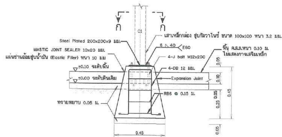
รูปขยายฐานรากโครงสร้างรับแผง F1 (ต่อม่อ คสล. หล่อสำเร็จรูปพร้อมติดตั้ง) ไม่แสดงขนาดบางส่วน
