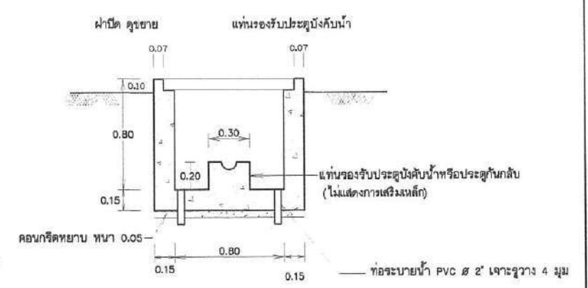
รูปตัด 1 - 1
