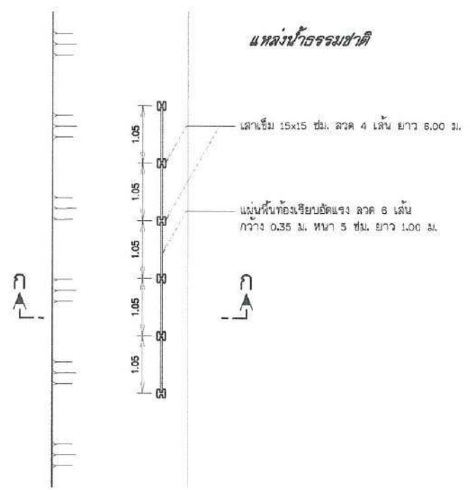
แปลนงานป้องกันดินพัง
