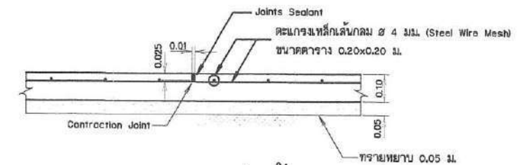
แบบขยายรอยต่อพื้น (Contraction Joint) ไม่แสดงขนาดบางส่วน
