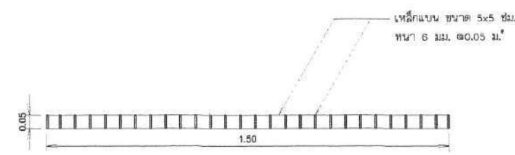
รูปตัด ข - ข
