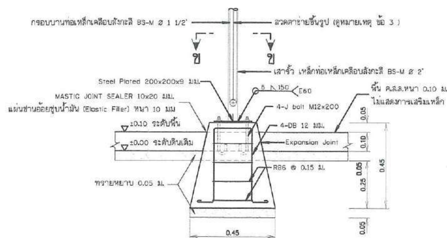
รูปขยายฐานรากโครงสร้างรับแผง F1 (เดอมอ คสล. หล่อสำเร็จรูปพร้อมติดตั้ง) ไม่แสดงมาตราส่วน
