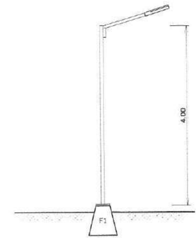
แบบเสาไฟ
