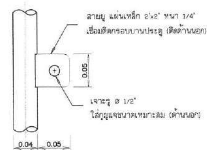
แบบขยายสายปู ไม่แสดงมาตราส่วน
