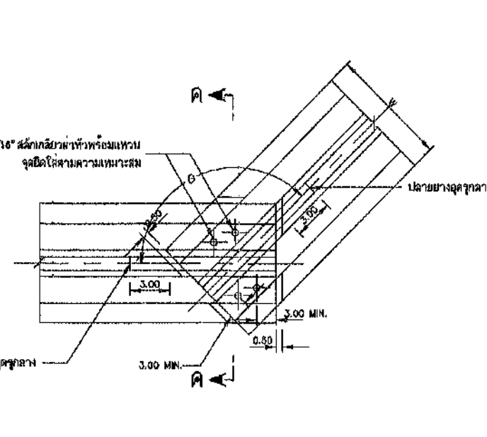
การต่อทำมุมกัน ไม่แสดงมาตราส่วน
