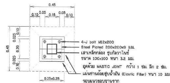
รูปตัด ก-ก ไม่แสดงขนาดบางส่วน
