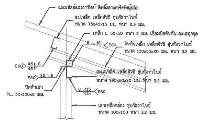
รูปขยาย การติดตั้งโครงหลังคา ไม่แสดงขนาดบางส่วน
