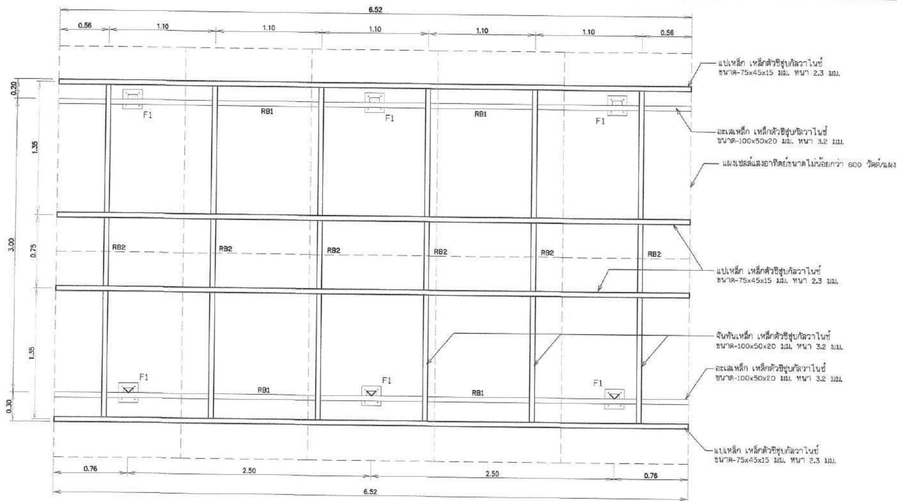
แปลนฐานรากและโครงหลังคา ไม่แสดงขนาดบางส่วน
