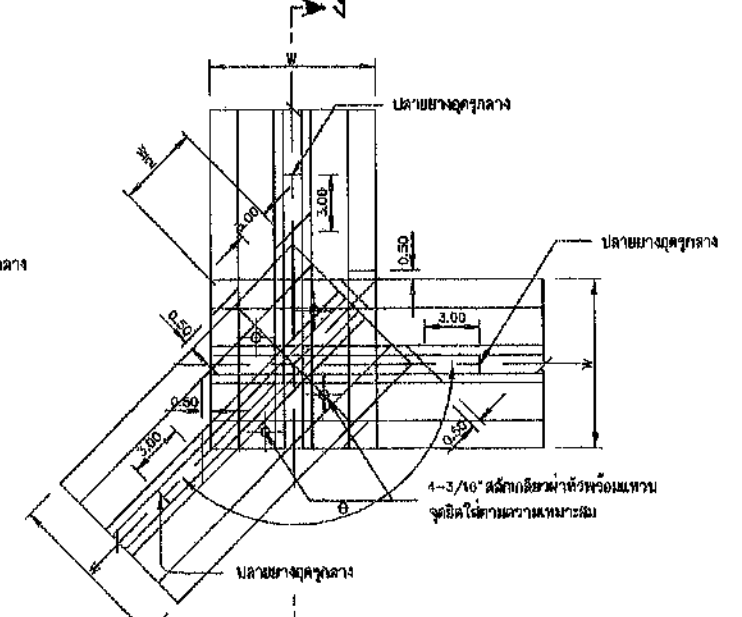
การต่อมุมกันทั้ง 3 ด้าน ไม่แสดงมาตราส่วน
