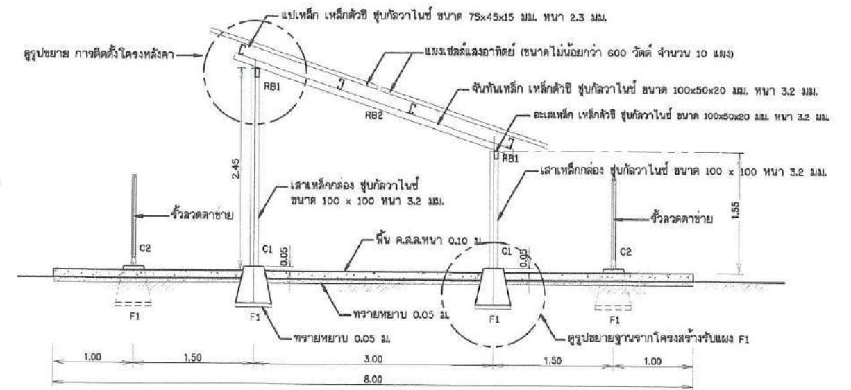
รูปด้านข้าง ไม่แสดงขนาดบางส่วน
