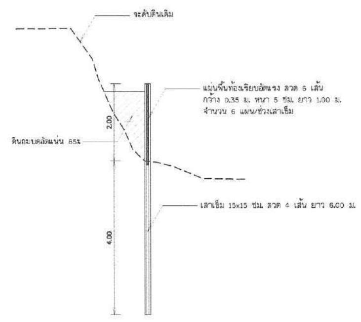
รูปตัด ก - ก
