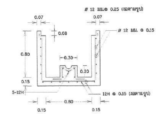
เหล็กเสริมบ่อประจุบึงคืบน้ำ
