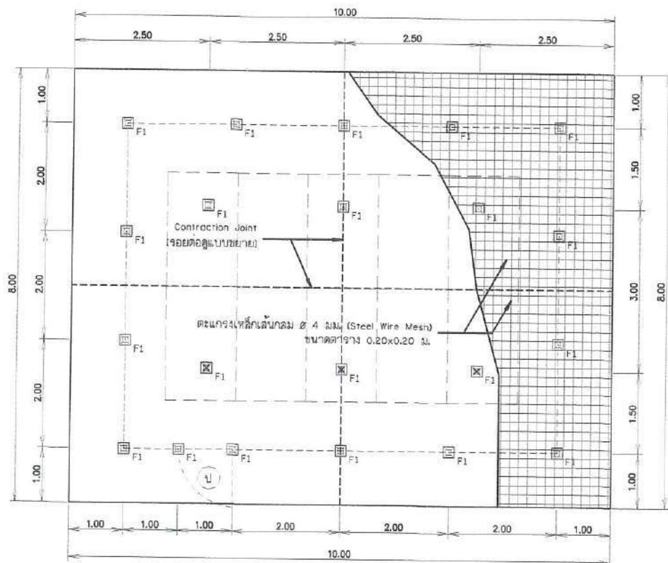
รูปขยายพื้นคอนกรีต ไม่แสดงขนาดบางส่วน
