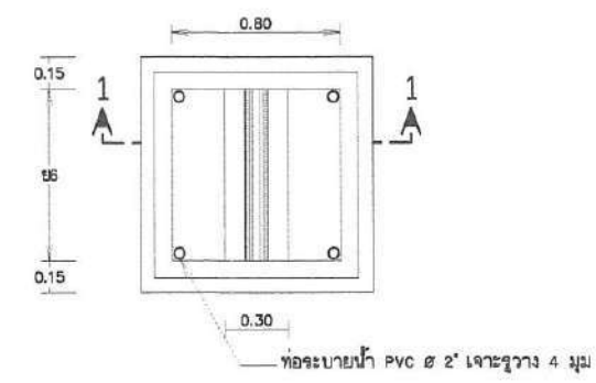
แปลนบ่อประจุบึงคืบน้ำ
