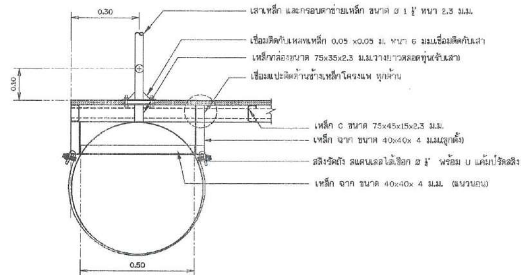
ขยายรูปด้านหน้าถึงเพลอย
