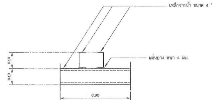
แบบขยายแท่นเครื่องสูบน้ำ
