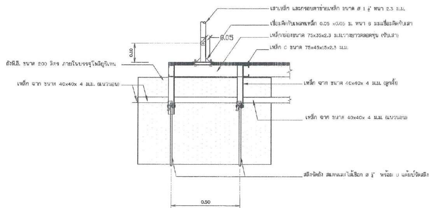
ขยายรูปด้านข้างถึงเพลอย
