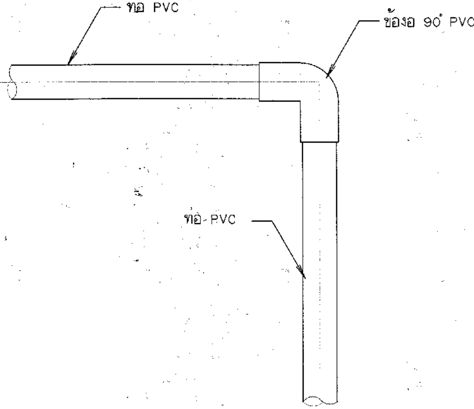
แบบการต่อข้อต่อ 90° PVC ไม่แสดงมาตราส่วน
