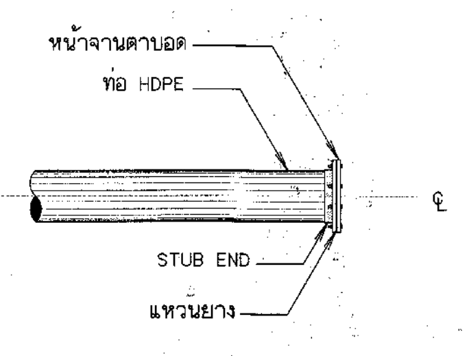
การปิดปลายท่อ ไม่แสดงมาตราส่วน
