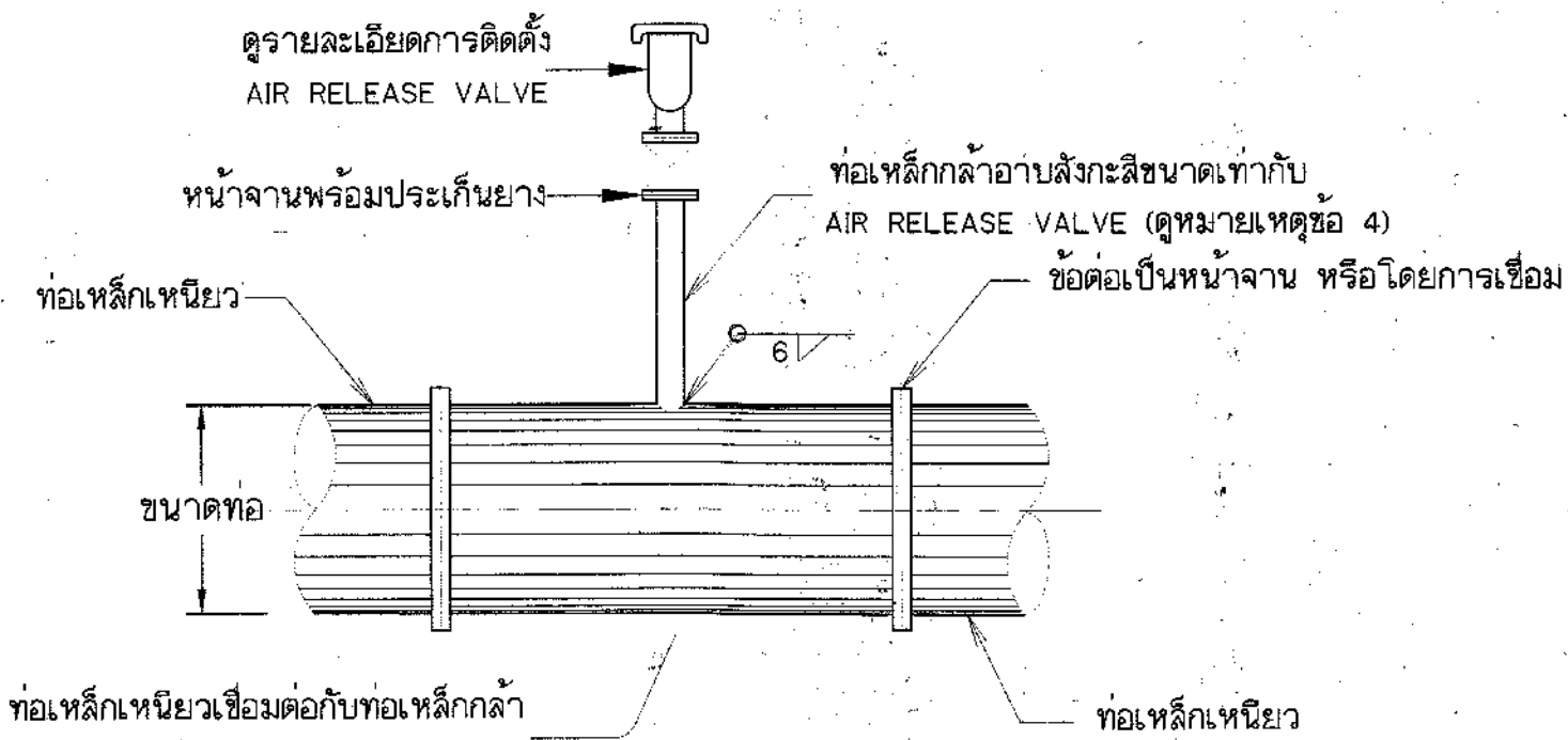
รายละเอียดข้อต่อแบบที่ 1 (กรณีท่อส่งน้ำเป็นท่อเหล็กเหนียว) ไม่แสดงมาตราส่วน
