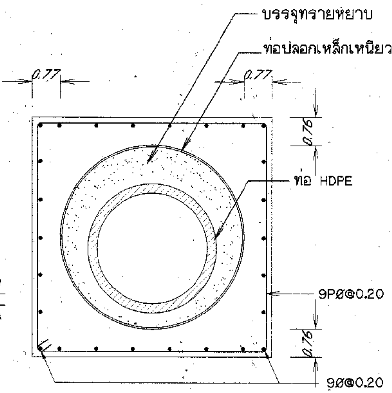
รูปตัด ก-ก มาตราส่วน 1:20
