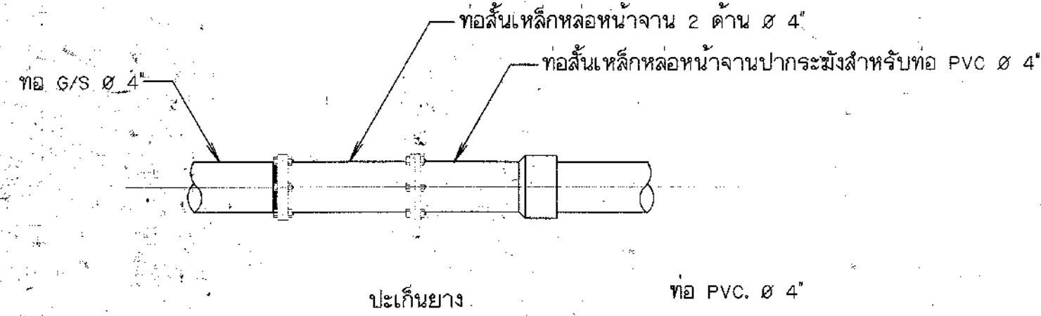
การบรรจุท่อเหล็กกล้าปลิงกลี G/S กับท่อ PVC. ไม่แสดงมาตราส่วน
