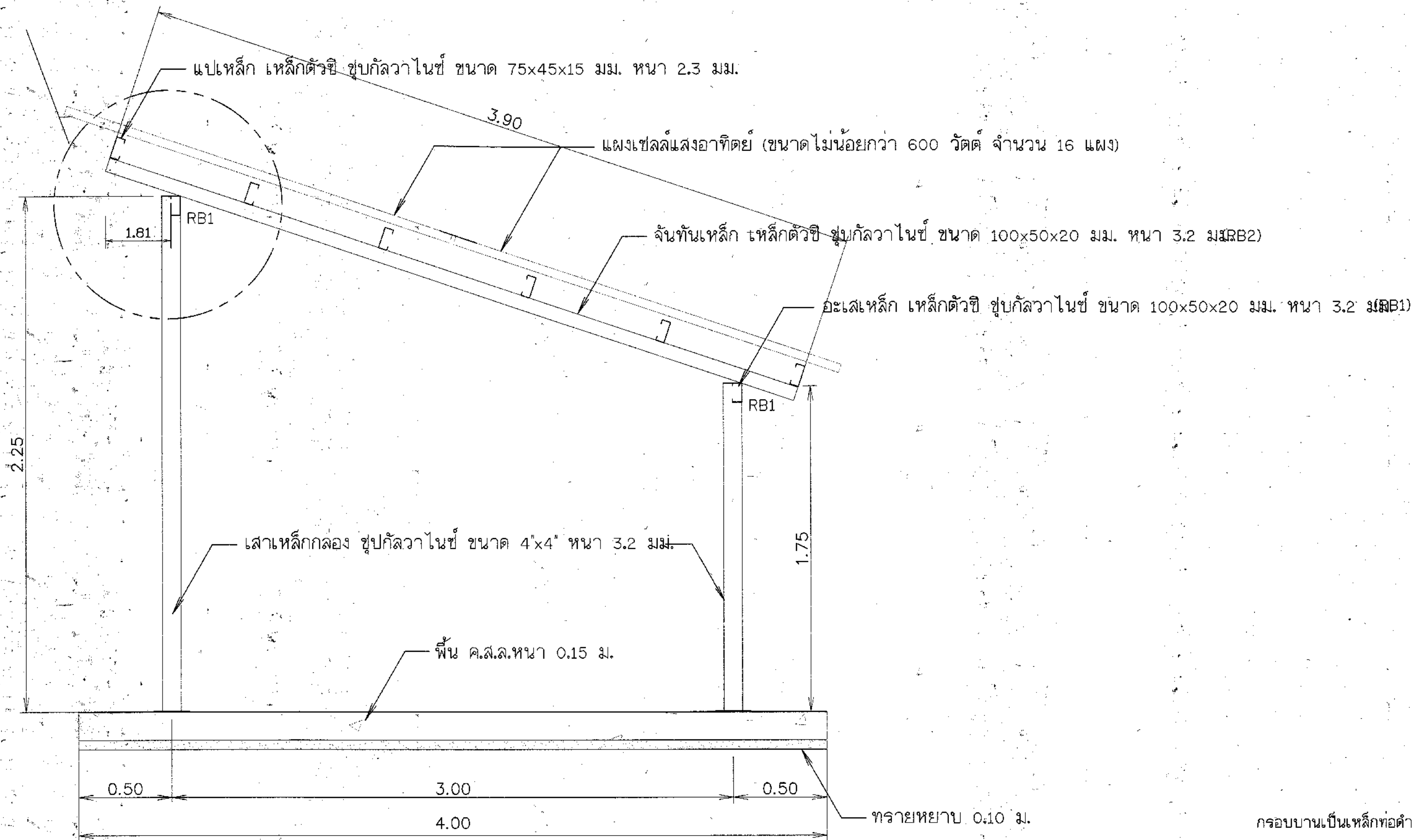
ดูรูปขยาย การติดตั้งโครงหลังคา
