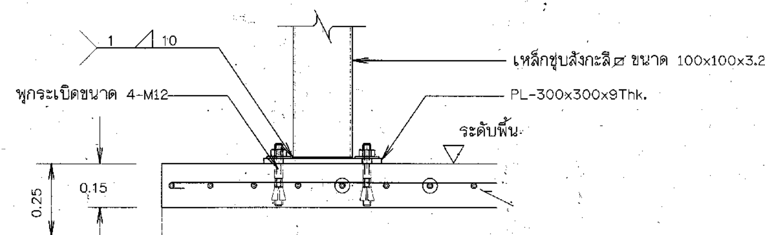
รูปตัด ก1 - ก1
