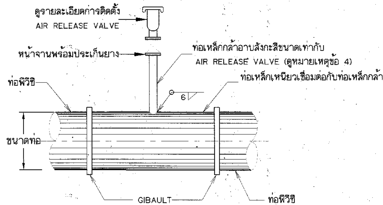
รายละเอียดข้อต่อแบบที่ 2 (กรณีท่อส่งน้ำเป็นท่อพีวีซี) ไม่แสดงมาตราส่วน
