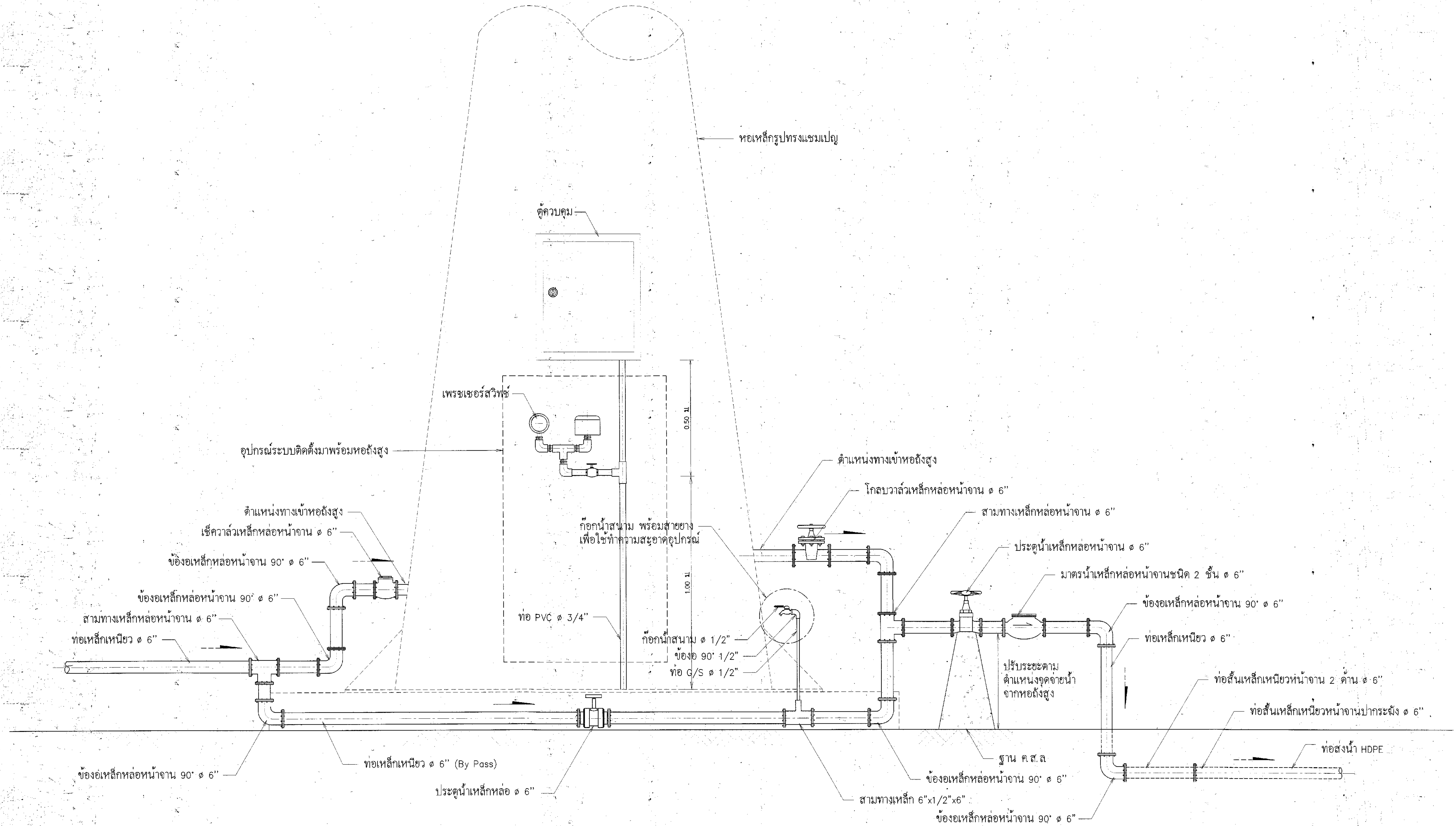
รูปแสดงรายละเอียดการต่อท่อและอุปกรณ์ออกจากถังเหล็กประพวงแฉลบ ไม่แสดงมาตราส่วน
