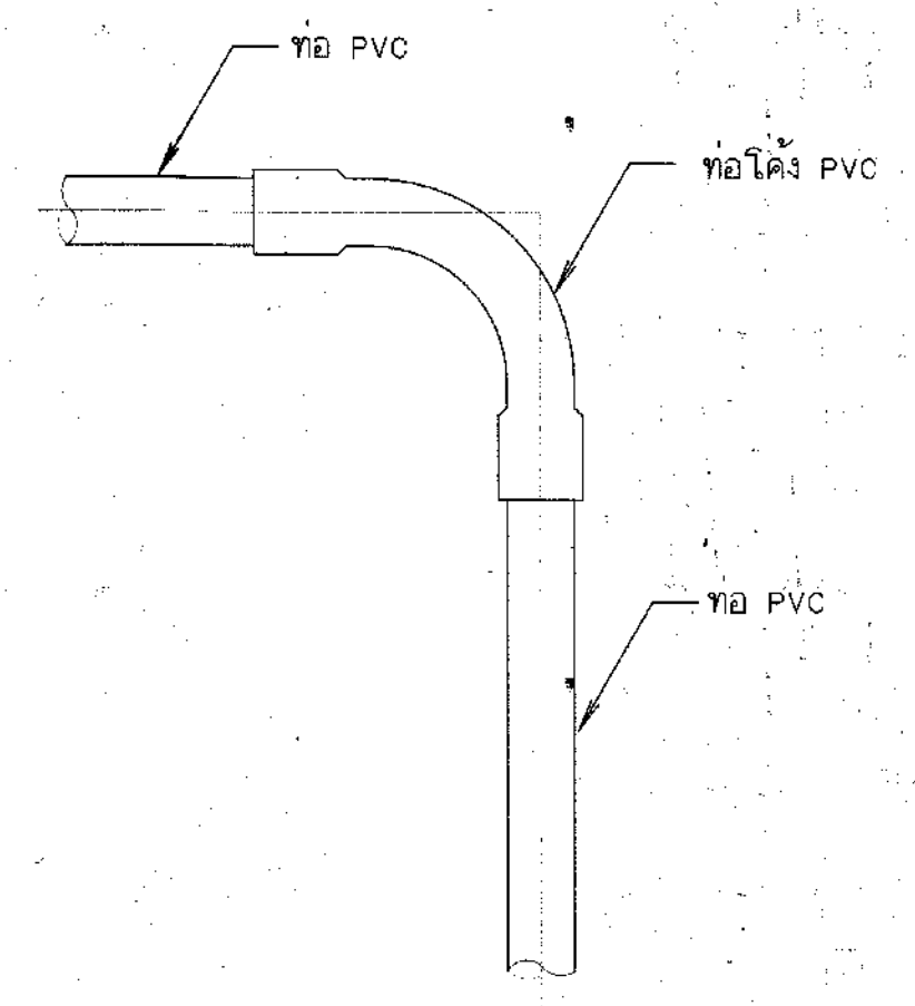
แบบการต่อข้อโค้ง 90° PVC ไม่แสดงมาตราส่วน
