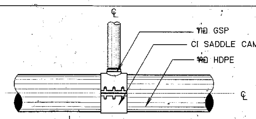
การบรรจุท่อสามทาง HDPE กับท่อ GSP แบบ CI SADDLE CLAMP (สำหรับอาคารจุดปล่อยน้ำ อาคารประตูดระบายตะกอน อาคารท่อระบายอากาศ กรณีท่อส่งน้ำขนาดเส้นผ่าศูนย์กลางน้อยกว่าหรือเท่ากับ 315 มม.) ไม่แสดงมาตราส่วน
