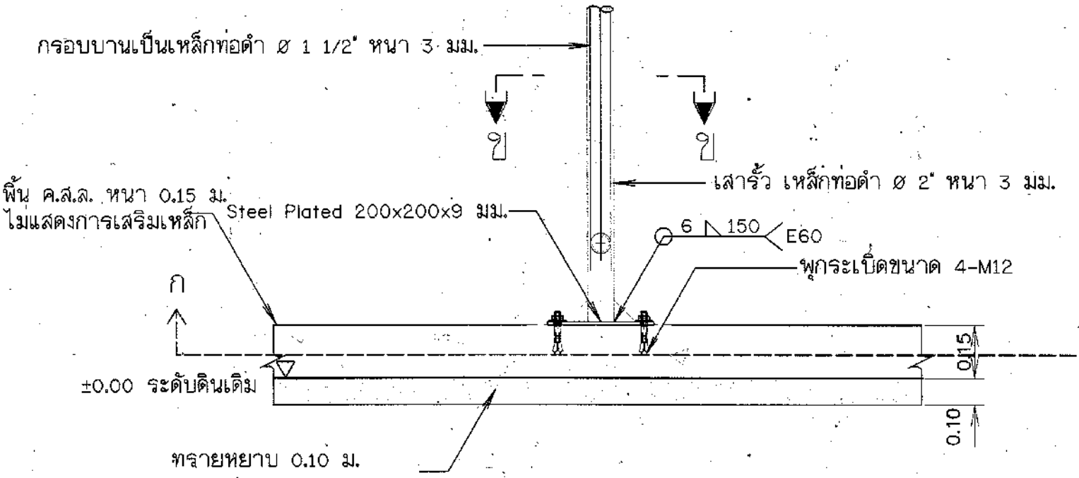
รูปขยายโครงสร้างรับแผง
