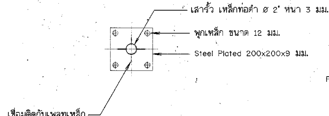
รูปตัด ข-ข
