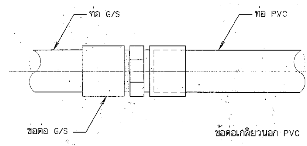
แบบการต่อท่อ G/S กับท่อ PVC ไม่แสดงมาตราส่วน
