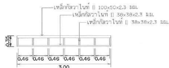
แบบขยาย T4 มาตราส่วน 1 : 100
