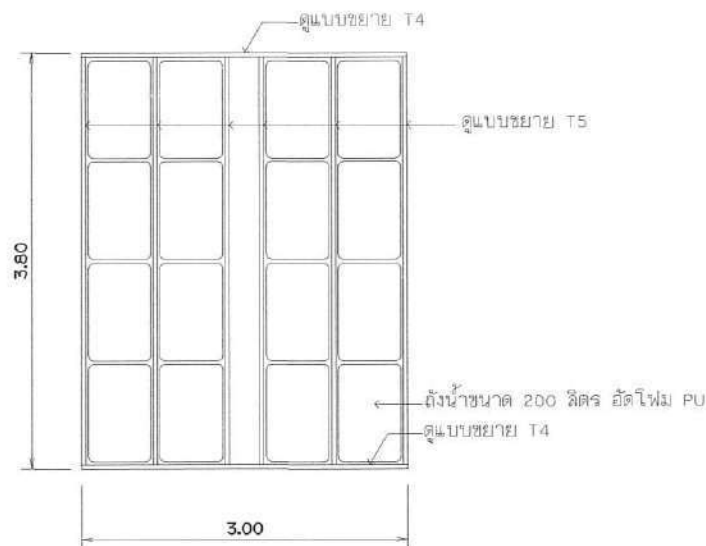
แบบขยายแพลอยสะพานช่วงที่ 2 มาตราส่วน 1 : 100
