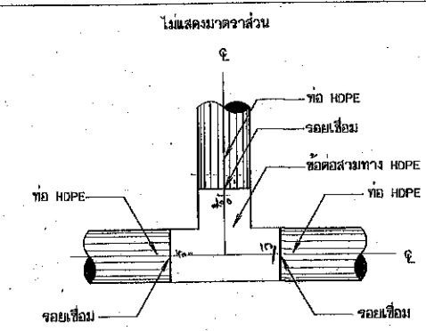
การบรรจุบ่อสามทาง HDPE กับท่อ HDPE ไม่แสดงมาตราส่วน
