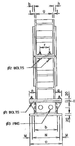
แบบแปลนข้าง (สำหรับท่อ Ø400 มม. - Ø1,000 มม.) ไม่แสดงขนาดบางส่วน
