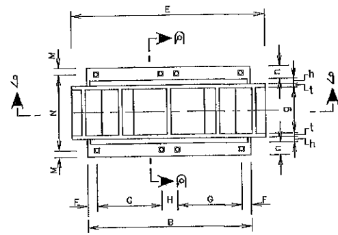
แบบแปลนตุ๊กตาจับท่อ (สำหรับท่อ Ø400 มม. - Ø1,200 มม.) ไม่แสดงขนาดบางส่วน
