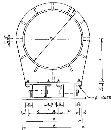
แบบแปลนหน้า (สำหรับท่อ Ø400 มม. - Ø1,000 มม.) ไม่แสดงขนาดบางส่วน
