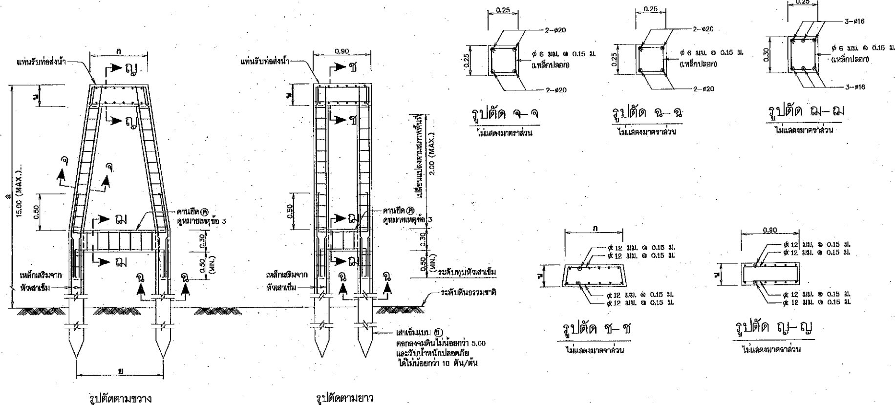
การเสริมเหล็กตอม่อรับท่อ แบบที่ 2
