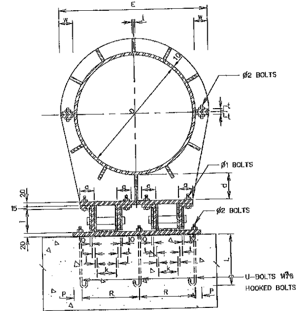
แบบแปลนหน้า (สำหรับท่อ Ø400 มม. - Ø1,000 มม.) ไม่แสดงขนาดบางส่วน
