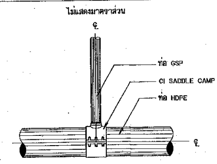
การบรรจุบ่อสามทาง HDPE กับท่อ GSP แบบ CI SADDLE CLAMP (สำหรับอาคารจุดปล่อยน้ำ อาคารประตูละบายตะกอน อาคารท่อระบายอากาศ กรณีท่อส่งน้ำขนาดเส้นผ่าศูนย์กลางน้อยกว่าหรือเท่ากับ 315 มม.)
