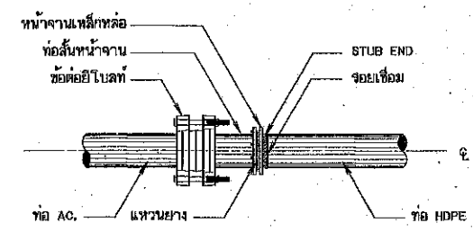
การบรรจุบ่อ AC. กับท่อ HDPE ไม่แสดงมาตราส่วน
