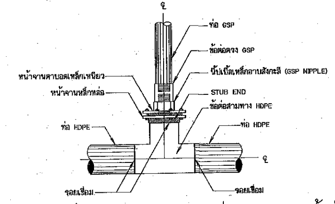
การบรรจุบ่อสามทาง HDPE กับท่อ GSP แบบข้อต่อ (สำหรับอาคารจุดปล่อยน้ำ อาคารประตูละบายตะกอน อาคารท่อระบายอากาศ กรณีท่อส่งน้ำขนาดเส้นผ่าศูนย์กลางมากกว่า 315 มม.)
