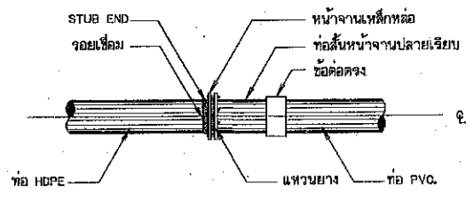
การบรรจุบ่อ HDPE กับท่อ PVC. ไม่แสดงมาตราส่วน
