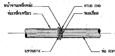
การบรรจุบ่อเหล็กเหนียวกับท่อ HDPE ไม่แสดงมาตราส่วน
