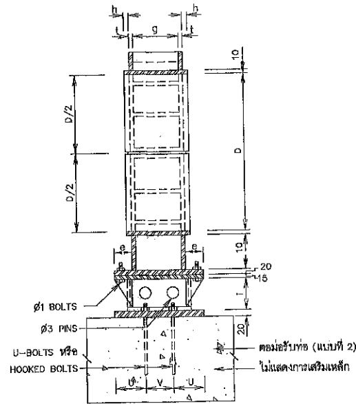
แบบแปลนข้าง (สำหรับท่อ Ø400 มม. - Ø1,000 มม.) ไม่แสดงขนาดบางส่วน
