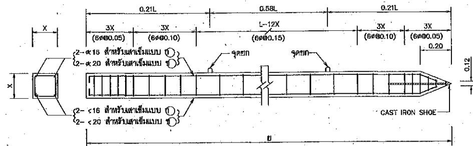
เส้าเข็ม ค.ส.ด. ไม่แสดงมาตราส่วน
