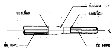
การบรรจุบ่อ HDPE กับข้อต่อ HDPE ไม่แสดงมาตราส่วน
