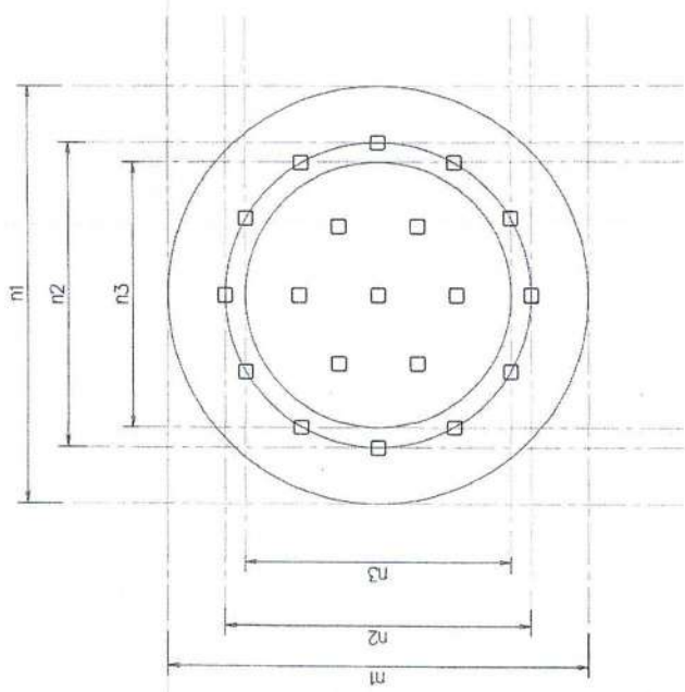
แผ่นฐานเดิม ถังเก็บน้ำ Fusion Bonded Epoxy (FBE) ขนาด 300 มม. มาตราส่วน 1:100
