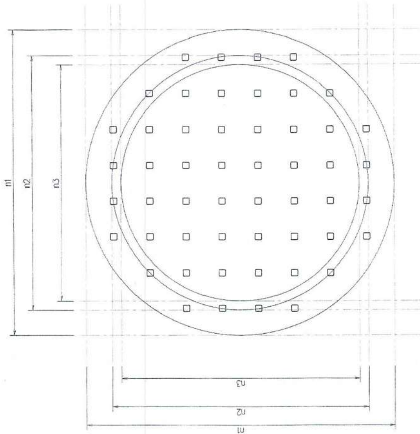
แผ่นฐานเดิม ถังเก็บน้ำ Fusion Bonded Epoxy (FBE) ขนาด 1,100 มม. มาตราส่วน 1:100
