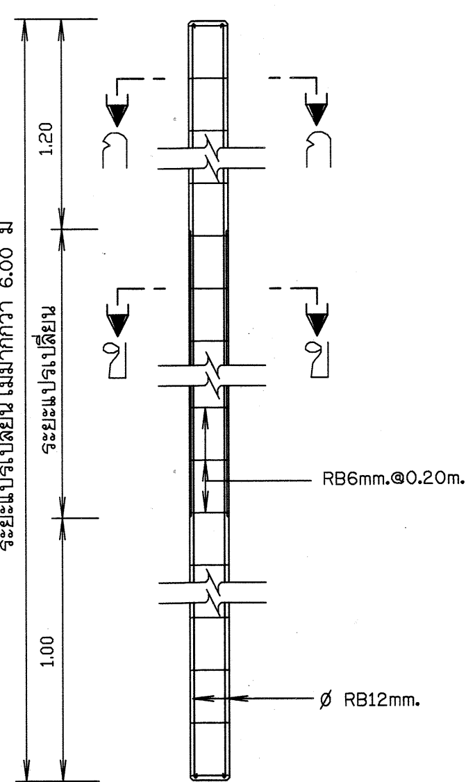
รายละเอียดเสาป้าย คสล. มาตรฐาน 1:20
