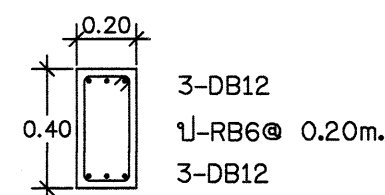
แปลนขยายโครงสร้างคาน BA SCALE 1:100
