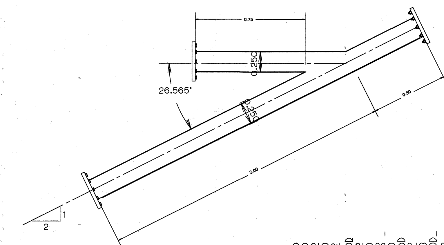
รายละเอียดทอริมดิ่ง ลาด 1:2 มาตราส่วน 1 : 100
