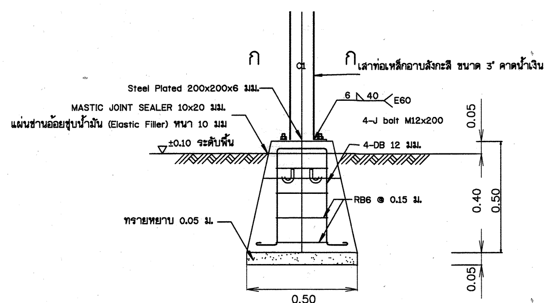
รูปขยายต่อม่อชุดกล้องวงจรปิด (ตาม คส. หรือรูปจริงพร้อมติดตั้ง) ไม่แสดงมาตราส่วน
