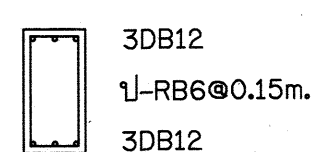
คาน Bx (0.20x0.40 m.) มาตราส่วน 1:25
