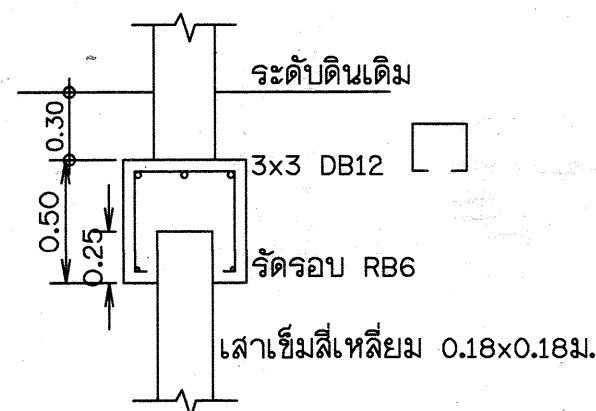
FA(0.50x0.50x0.50) แบบขยายฐานรากอาคารควบคุม มาตราส่วน 1:100
