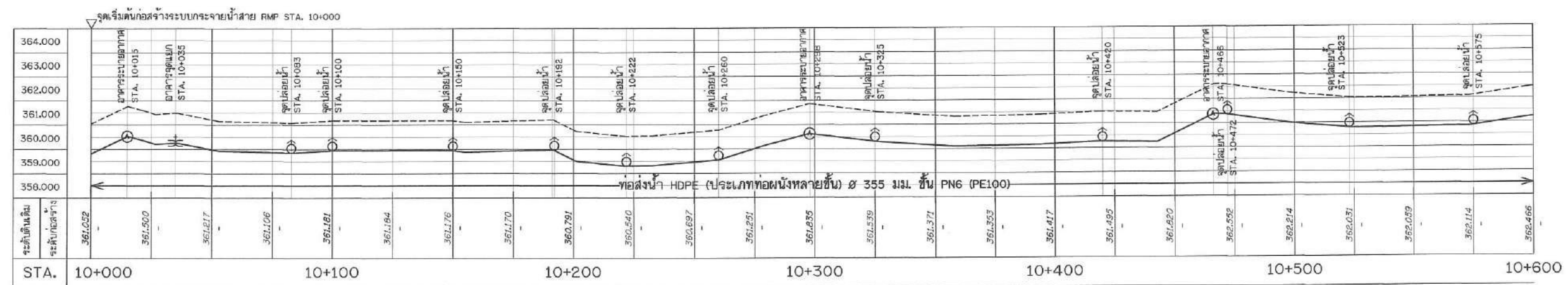
รูปตัดตามแนวยาวระบบกระจายน้ำ สาย 1L-1R-LMP STA. 10+000 - 10+600
