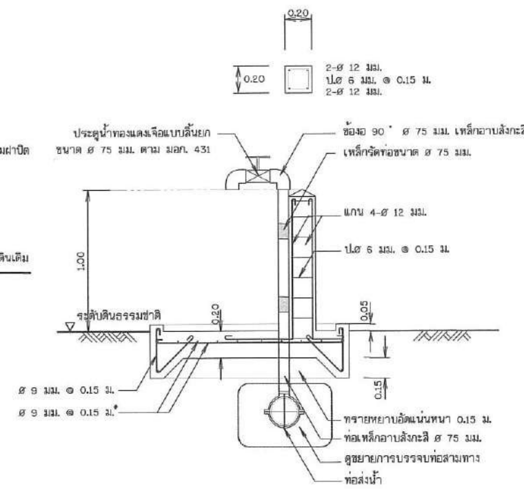
รูปตัด ค - ค
