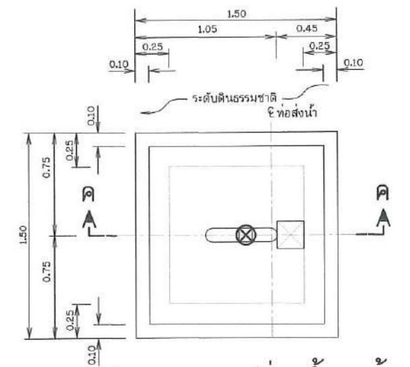
แปลนอาคารจุดปล่อยน้ำ 1 ด้าน
