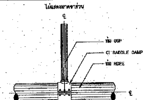
การบรรจุท่อสามทาง HDPE กับท่อ GSP แบบข้อต่อ สำหรับอาคารชลประทาน อาคารประสูตน้ำชลประทาน อาคารชลประทานอาคาร กรณีท่อส่งน้ำขนาดเส้นผ่าศูนย์กลางมากกว่า 315 มม.
