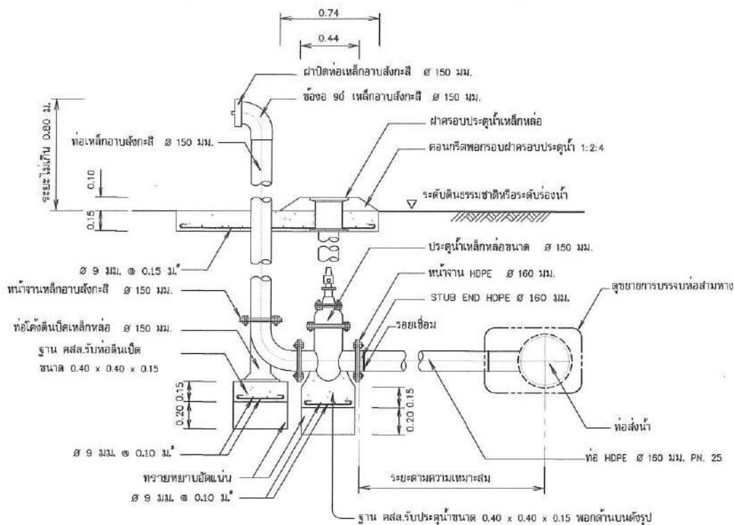
รูปตัด ก - ก แสดงการติดตั้งประตูระบายตะกอน
