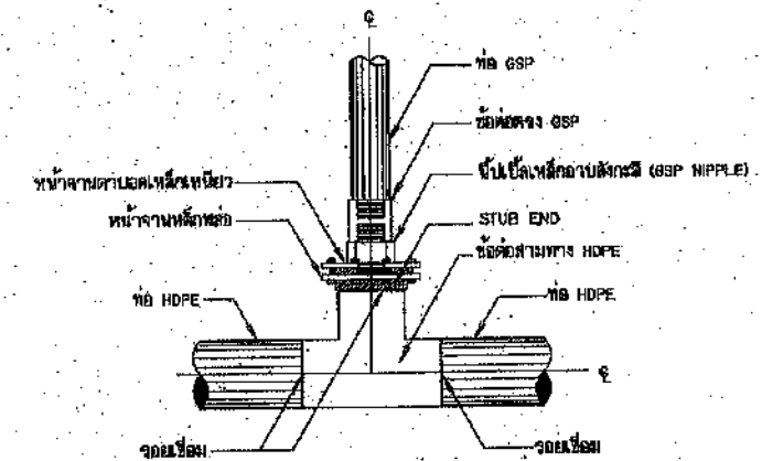
การบรรจุท่อสามทาง HDPE กับท่อ GSP แบบข้อต่อ สำหรับอาคารชลประทาน อาคารประสูตน้ำชลประทาน อาคารชลประทานอาคาร กรณีท่อส่งน้ำขนาดเส้นผ่าศูนย์กลางมากกว่า 315 มม.
