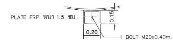
แบบขยาย ขายึดดึง SCALE 1 : 25
