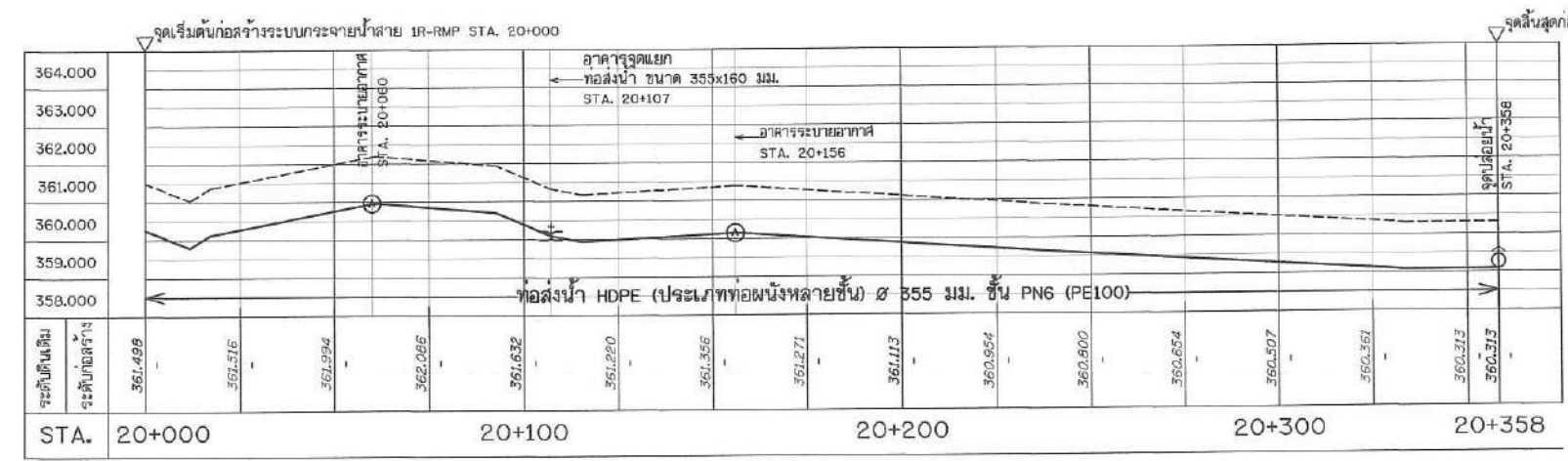
รูปตัดตามแนวยาวระบบกระจายน้ำ สาย 1R-1L-1R-LMP STA. 20+000 - 20+358 มาตรฐาน 1:1,000
