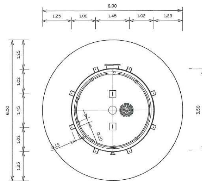
ตำแหน่ง ขายึดดึง SCALE 1 : 100
