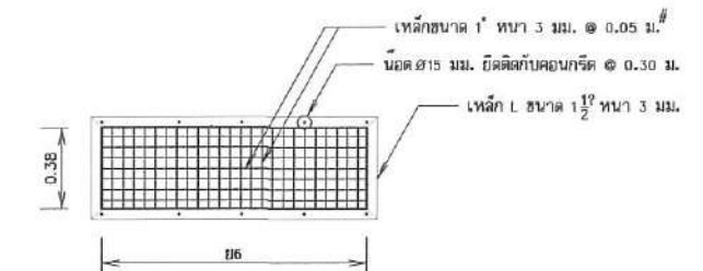
แปลนตะแกรงเหล็กกันลว
