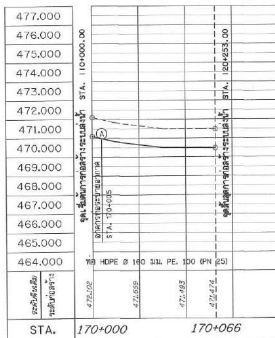
รูปตัดตามแนวยาว STA. 170+000 - 170+066 มาตรฐาน 1:200 แนวตั้ง 1:1,000
