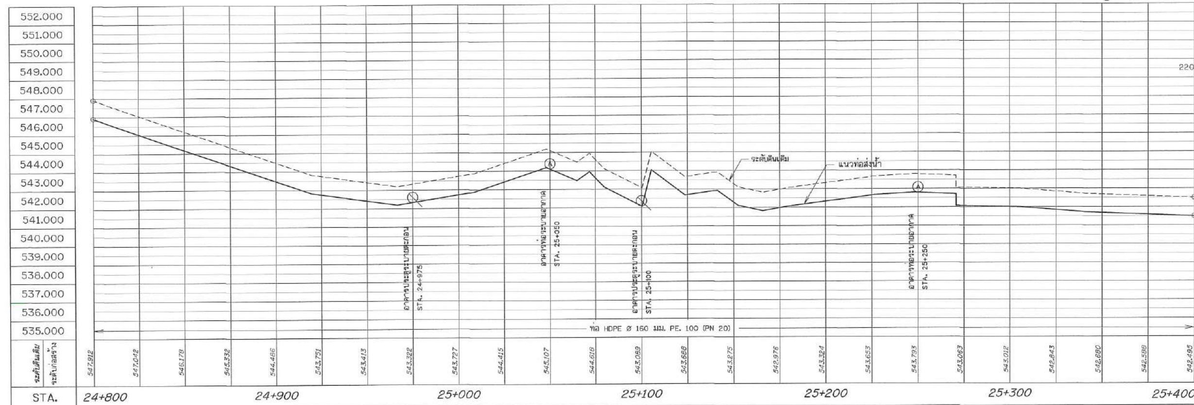
รูปตัดตามแนวยาว STA. 24+800 - 25+400 , STA. 50+000 - 50+046
