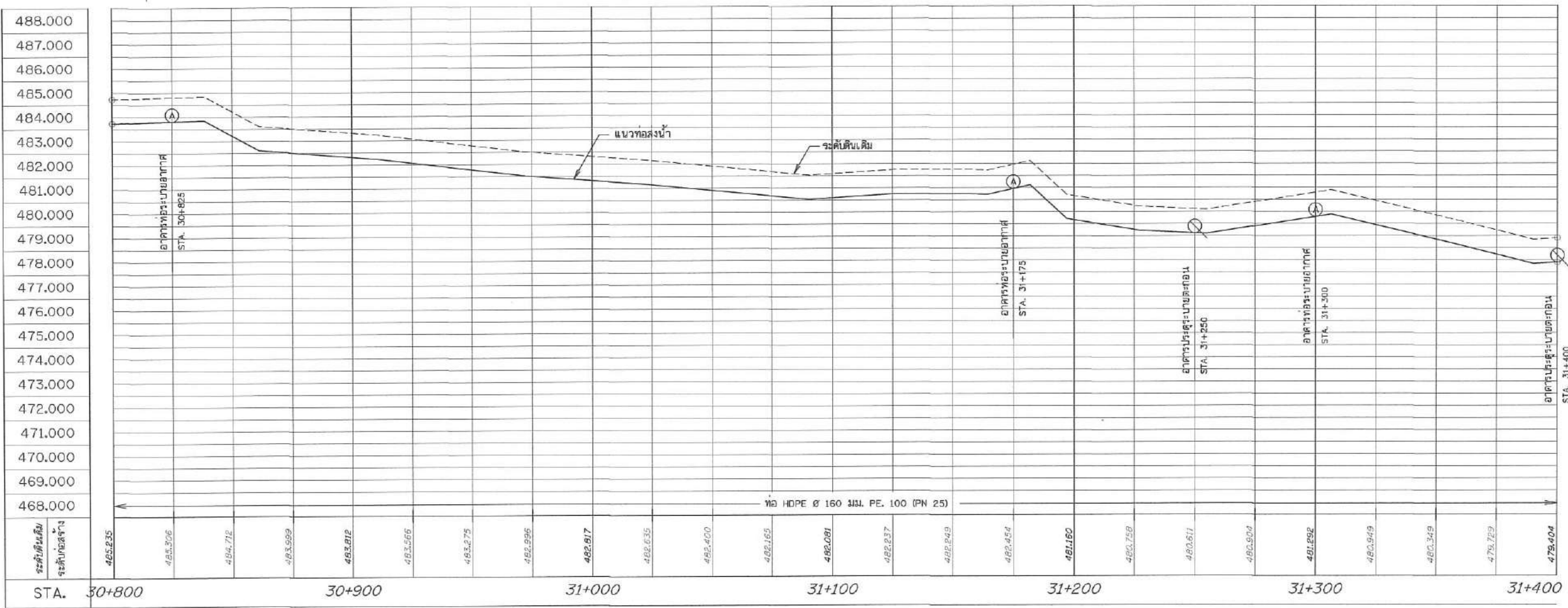
รูปตัดตามแนวยาว STA. 30+800 - 31+400
