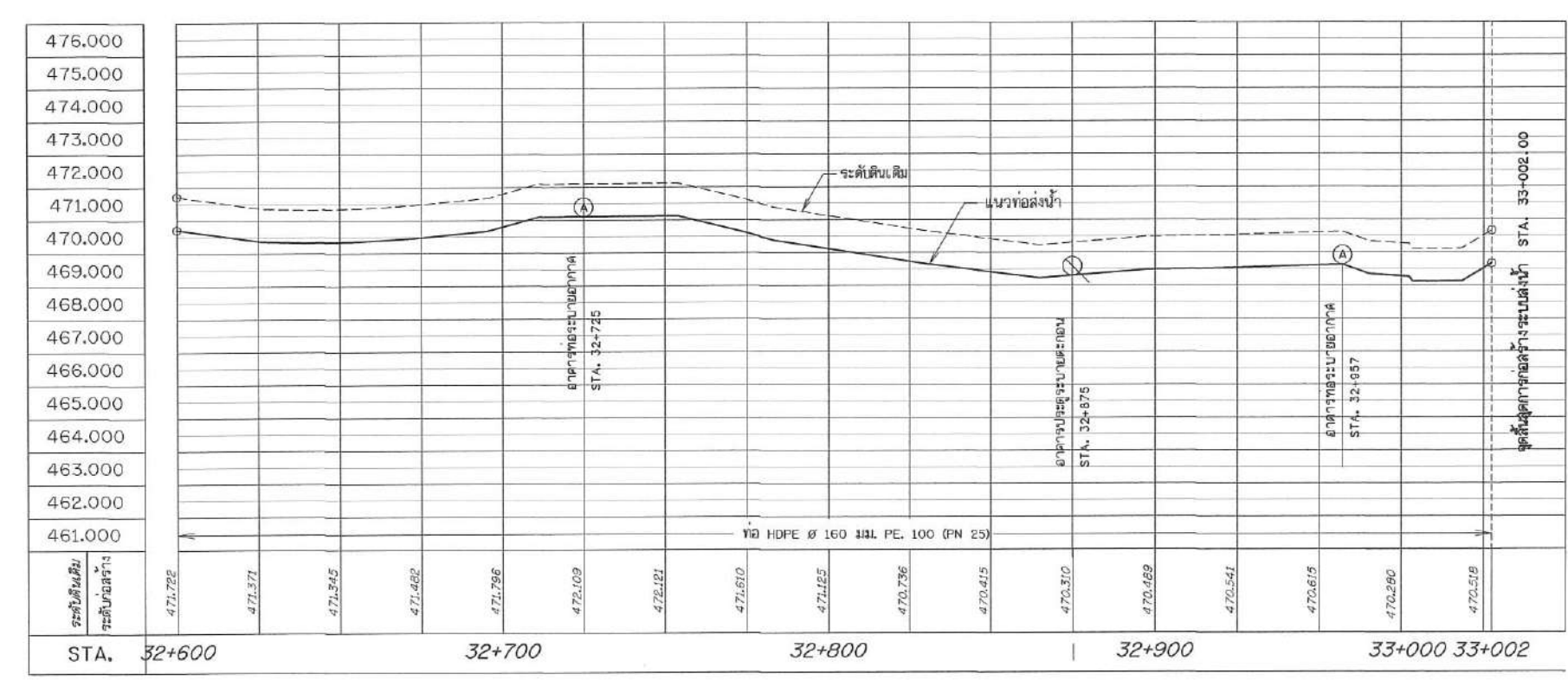
รูปตัดตามแนวยาว STA. 32+600 - 33+002
