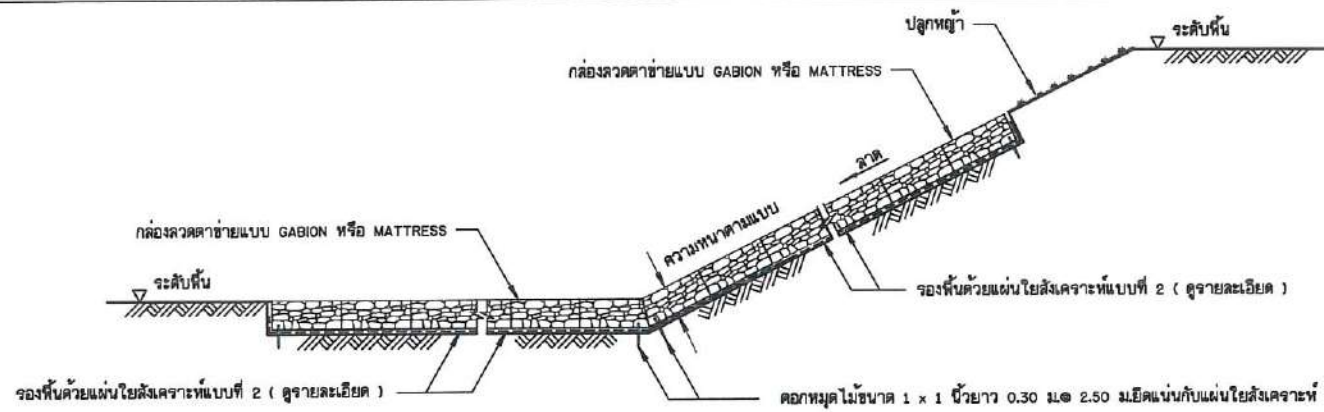
รูปตัดแสดงการวางกล่องลวดตาข่าย ( แผ่นใยสังเคราะห์รองพื้น )
