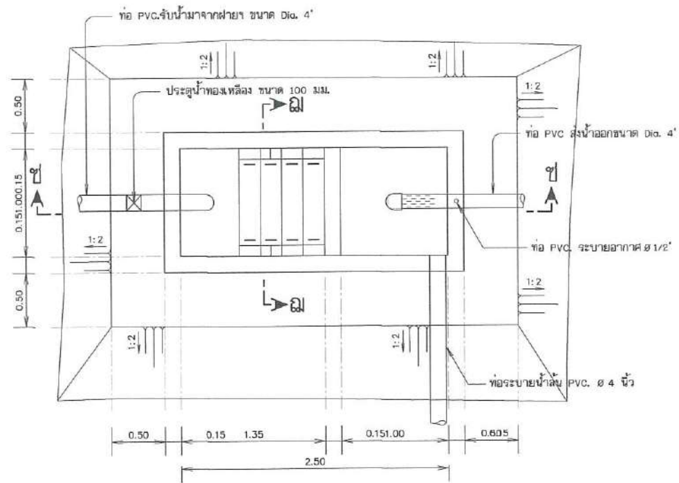
แปลนบ่อดักตะกอน
