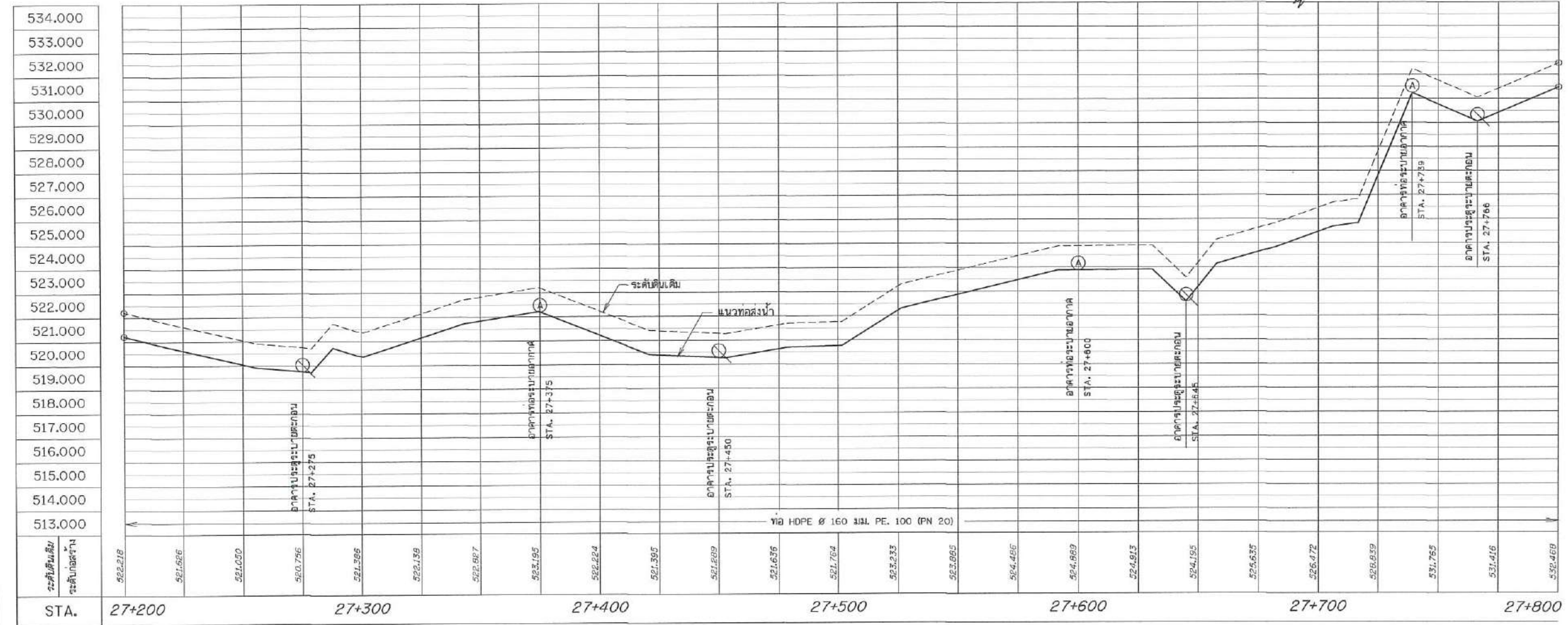
รูปตัดตามแนวยาว STA. 27+200 - 27+800 , STA. 70+000 - 70+057
