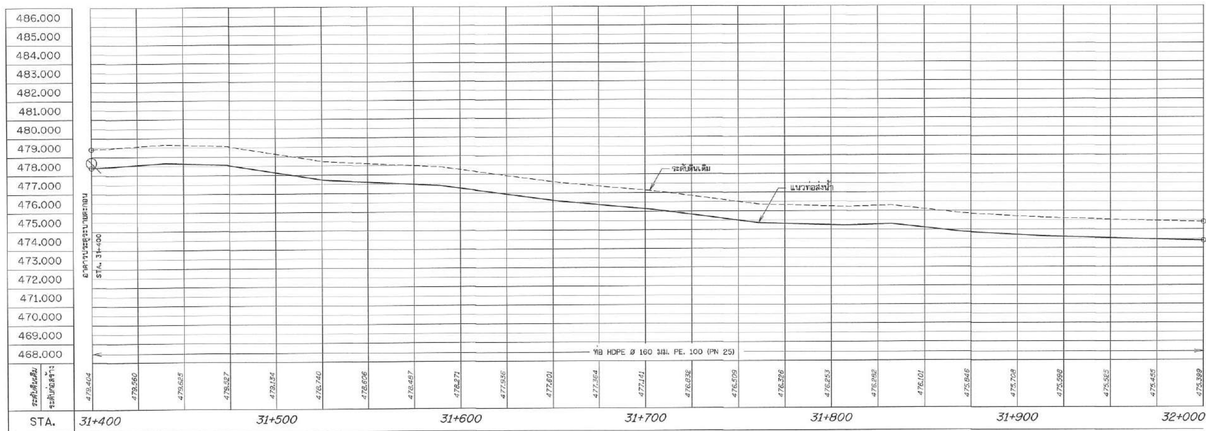
รูปตัดตามแนวยาว STA. 31+400 - 32+000
