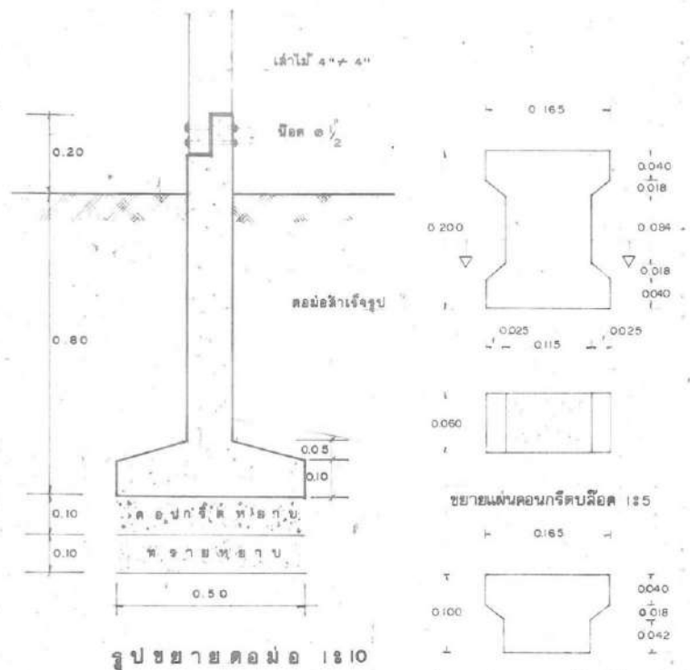
ขยายแผ่นคอนกรีตบล็อครีจแน่ม 185
