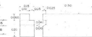
ขยายคั่นคอนกรีต 1810
