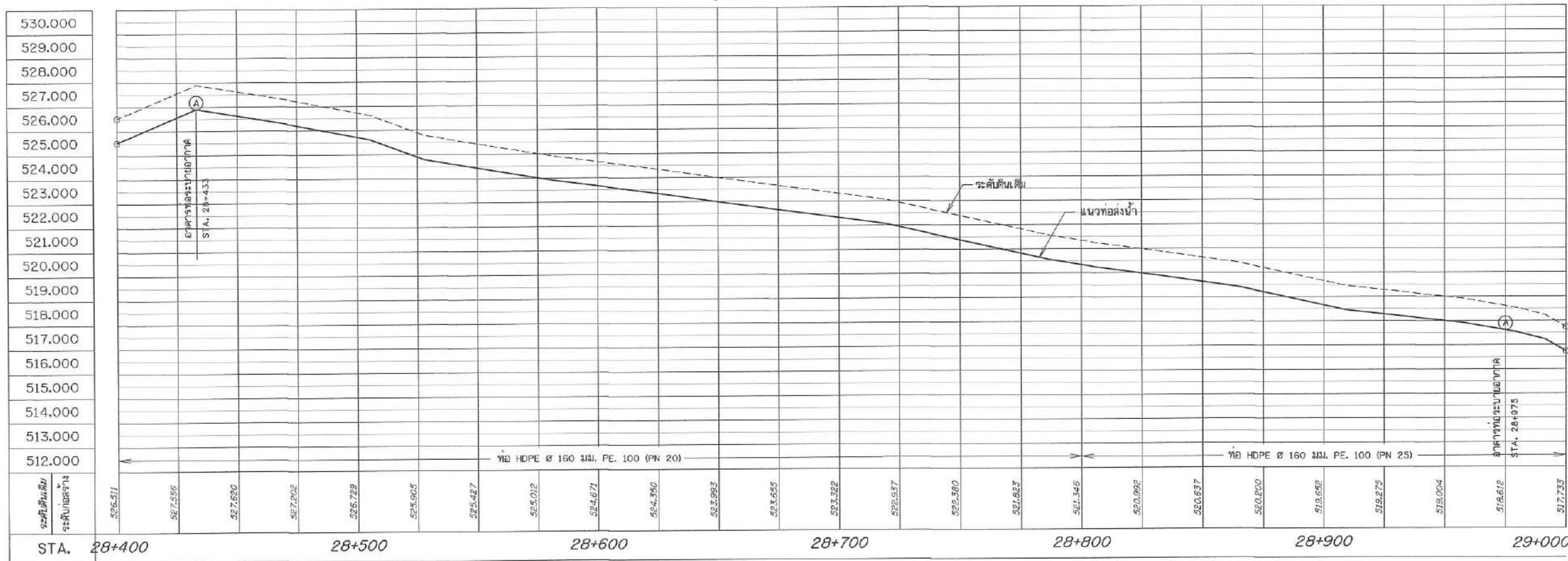
รูปตัดตามแนวยาว STA. 28+400 - 29+000
