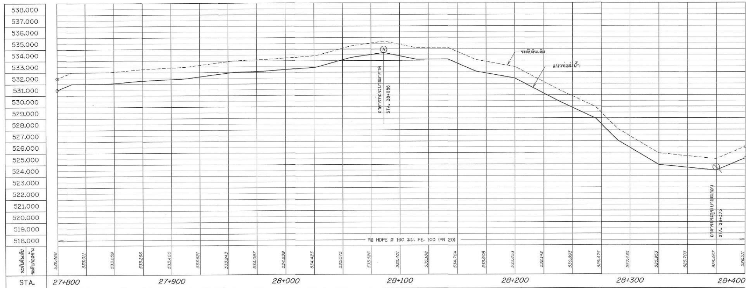
รูปตัดตามแนวยาว STA. 27+800 - 28+400
