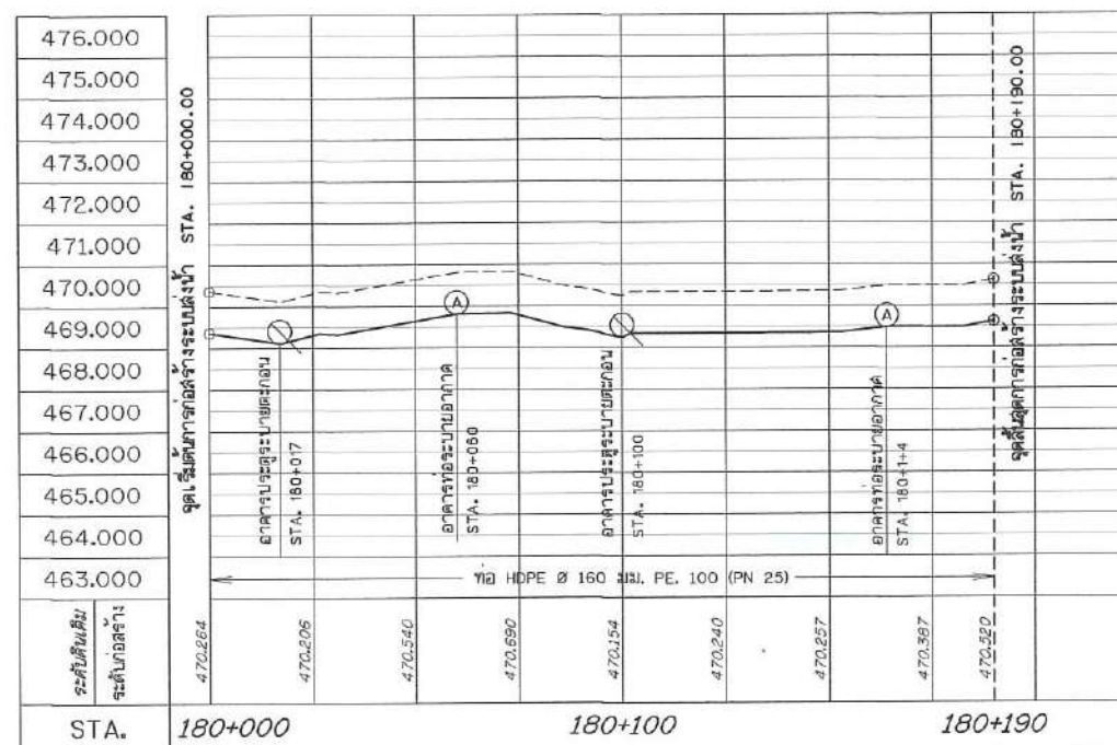
รูปตัดตามแนวยาว STA. 180+000 - 180+190 มาตรฐาน 1:200 แนวตั้ง 1:1,000
