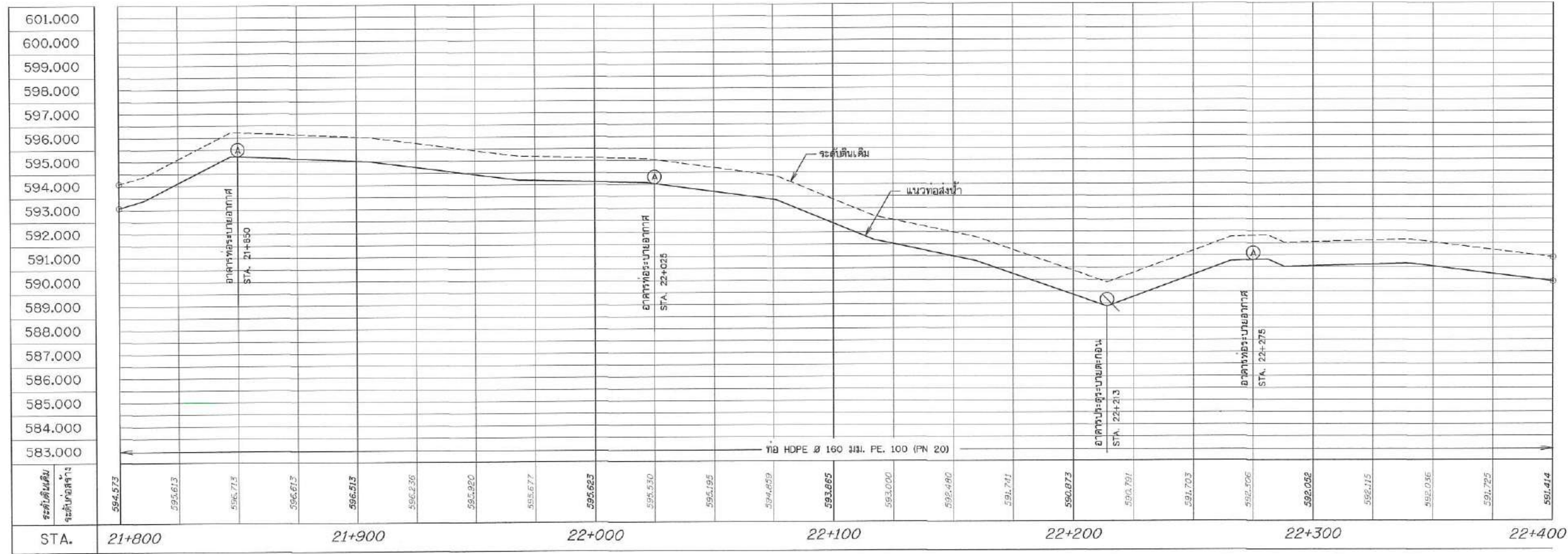
รูปตัดตามแนวยาว STA. 21+800 - 22+400 , STA. 30+000 - 30+035
