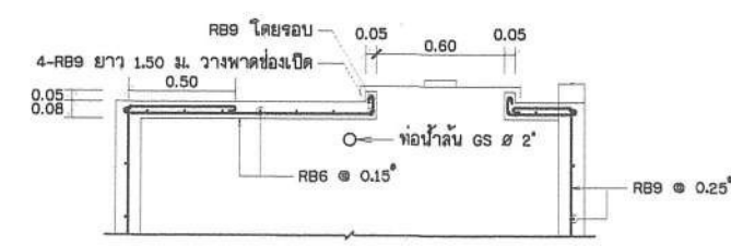
แสดงการเสริมเหล็กฝาถัง มาตราส่วน 1:20
