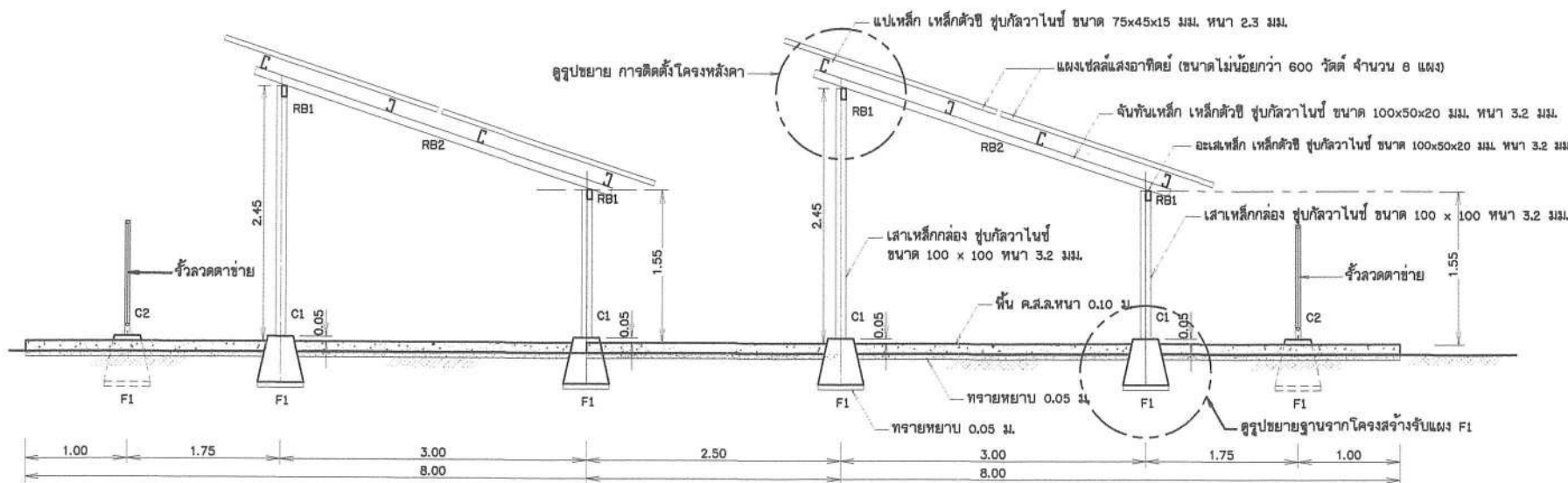
รูปด้านข้าง
