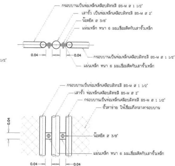
แบบขยายรายละเอียดแสดงการยึดระหว่างรื้อกับเสา
