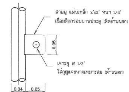
แบบขยายสาย โรงแสดงดนตรีส่วน
