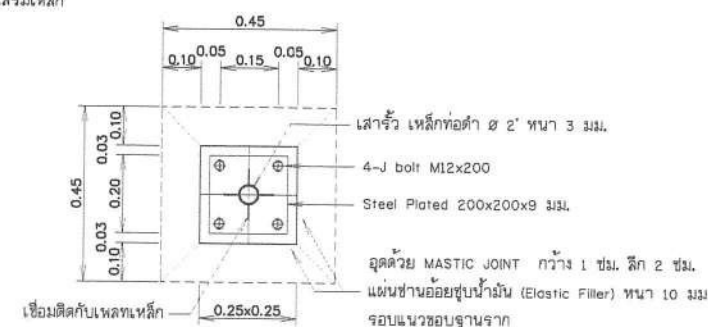
รูปตัด ข-ข ไม้เลื้อยมาดราส่วน
