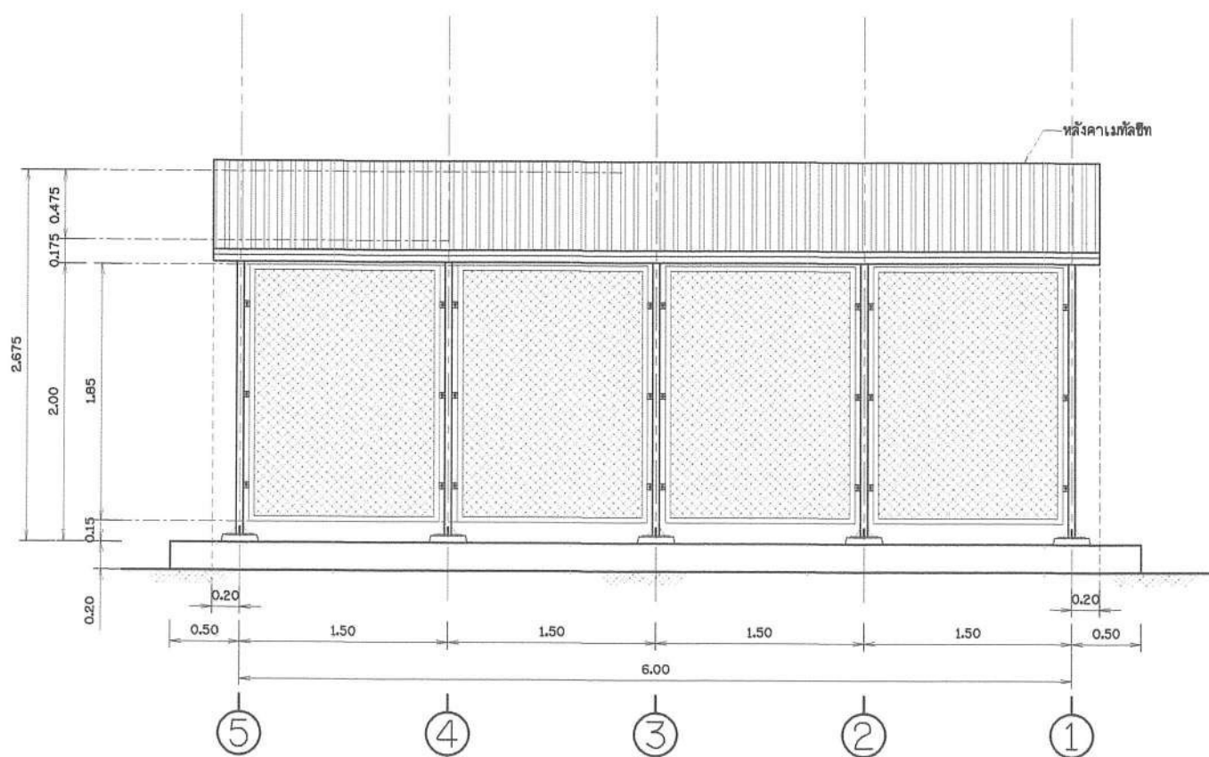
รูปด้าน 1 โมเมนต์มาตรฐาน
