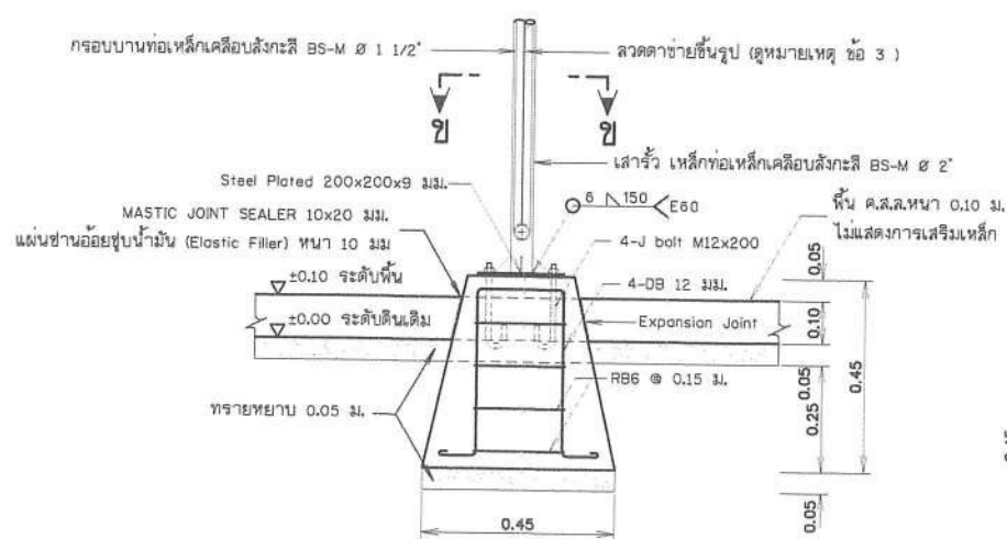
รูปขยายฐานรากโครงสร้างรับแผง F1 (ต่อมาอ. ศสส. ทลสอ.แจ้งสรุปพร้อมมติตั้ง) ไม่แสดงรายละเอียด
