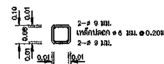
รูปตัด ข-ข มาตราส่วน 1:10
