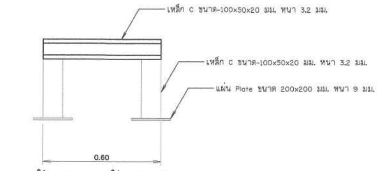
รูปด้านโครงสร้างรับท่อบนแพ ไม่แสดงมาตราส่วน
