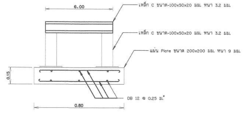
รูปด้านโครงสร้างรับท่อบนดิน ไม่แสดงมาตราส่วน
