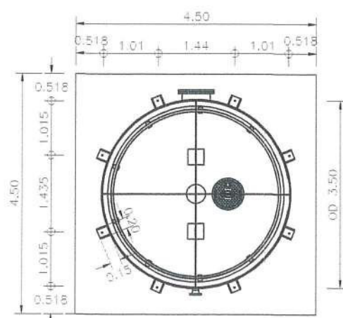
ตำแหน่ง ขายึดถัง SCALE 1 : 100
