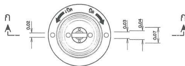
รายละเอียดแบบฝาคกรอบประตูน้ำเหล็กหล่อ
