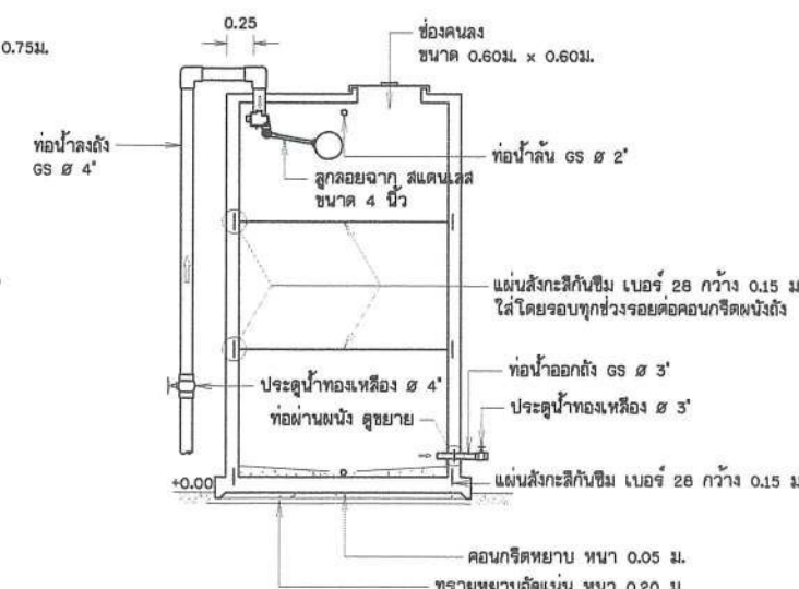
รูปตัด (1) มาตราส่วน 1:40
