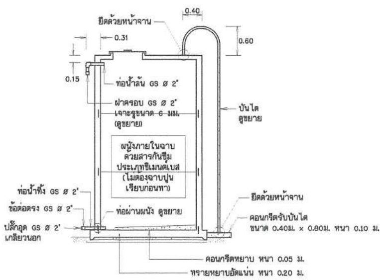
รูปตัด (2) มาตราส่วน 1:40
