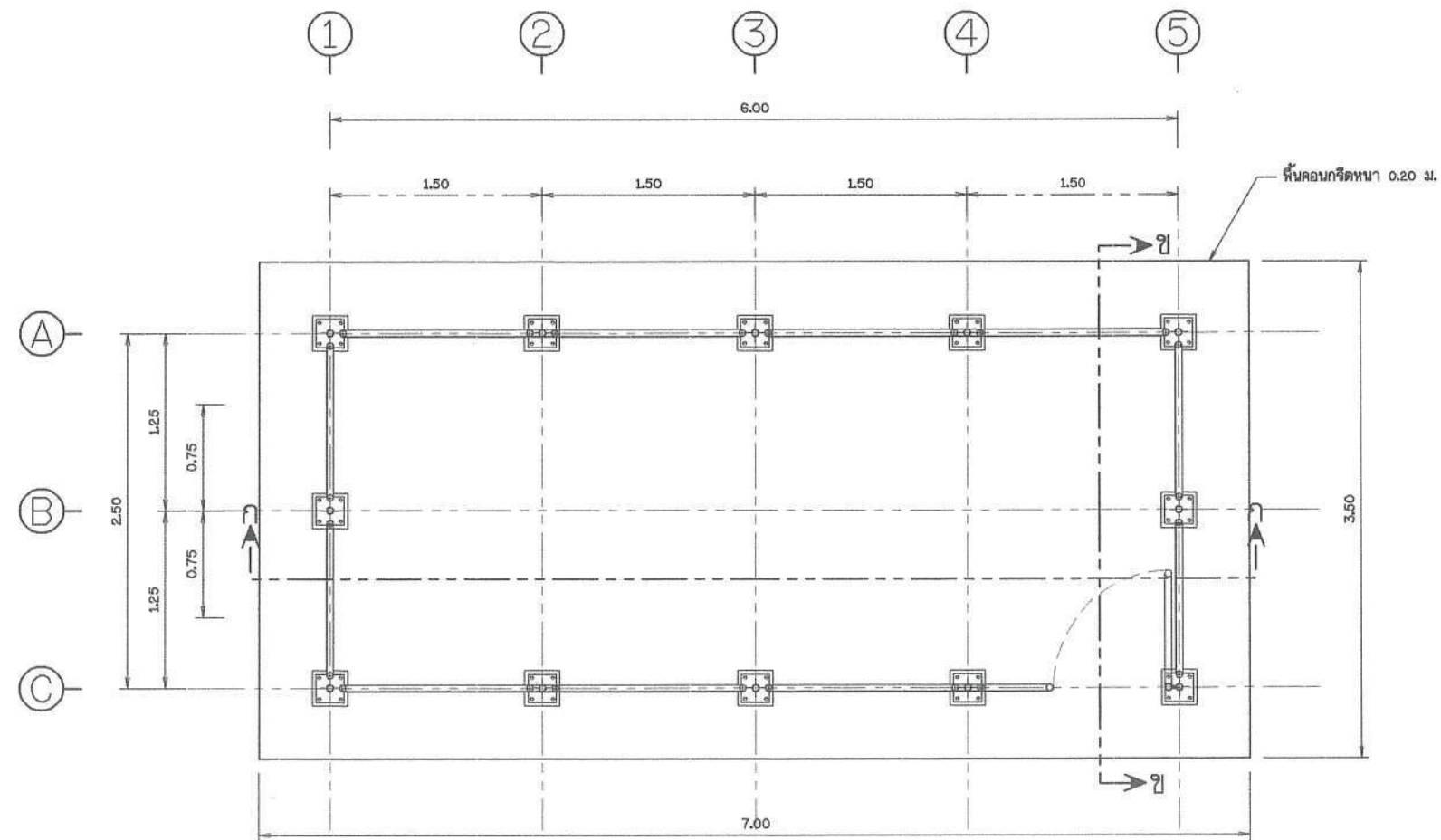
แปลนเสาและรั้ว ไม่แสดงขนาดราส่วน
