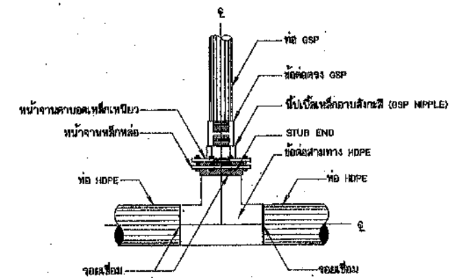
การบรรจุท่อสามทาง HDPE กับท่อ GSP แบบข้อต่อ สำหรับอาคารจุดปล่อยน้ำ อาคารประจวบประมาณ 100 เมตร อาคารท่าเรือประมาณ 100 เมตร กรณีท่อส่งน้ำขนาดเส้นผ่านศูนย์กลางน้อยกว่า 315 มม.
