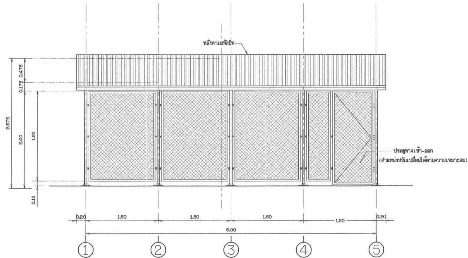
รูปด้าน 1 ไม่แสดงขนาดราวล้วน
