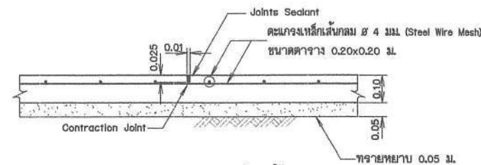
แบบขยายรอยต่อพื้น (Contraction Joint) ไม่แสดงมาตราส่วน
