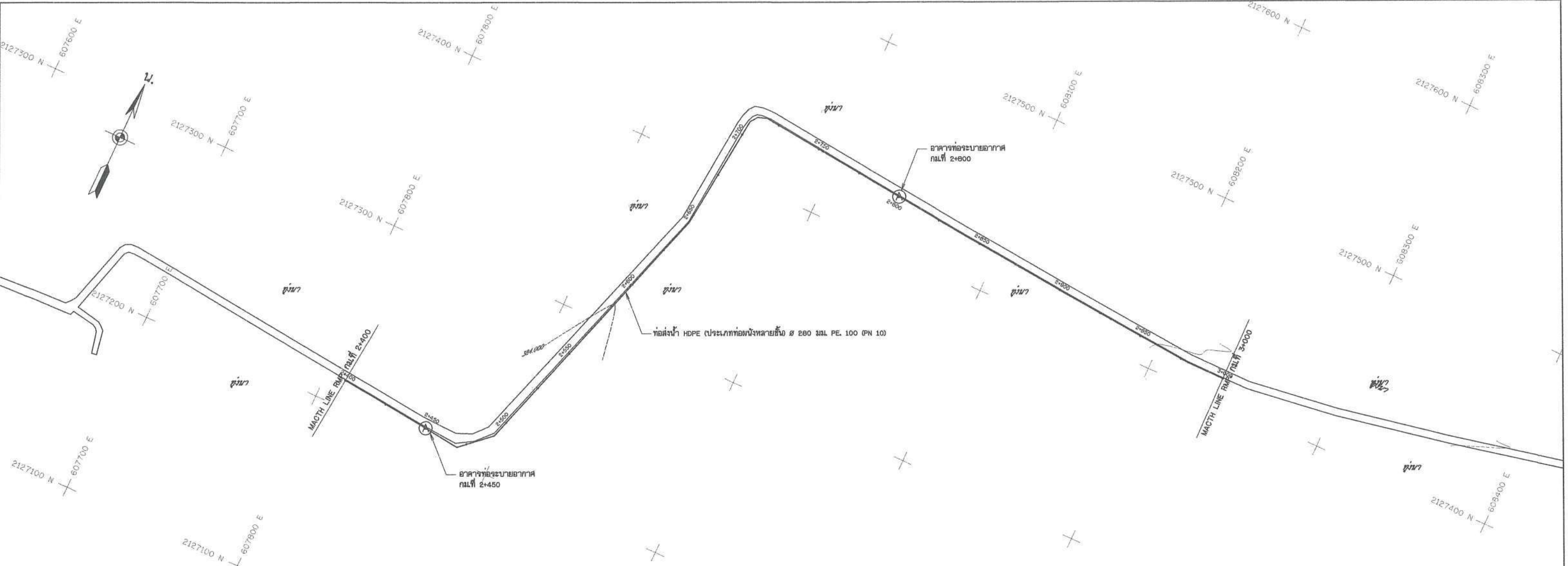
แปลนระบบส่งน้ำ สาย RMP. STA. 2+400 - 3+000 มาตราส่วน 1:1,000
