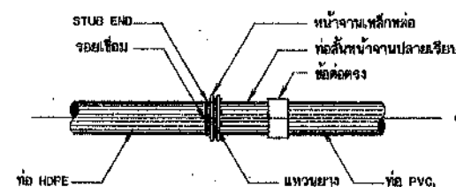
การบรรจุท่อ HDPE กับท่อ PVC. ไม่แสดงขนาดคร่าวๆ
