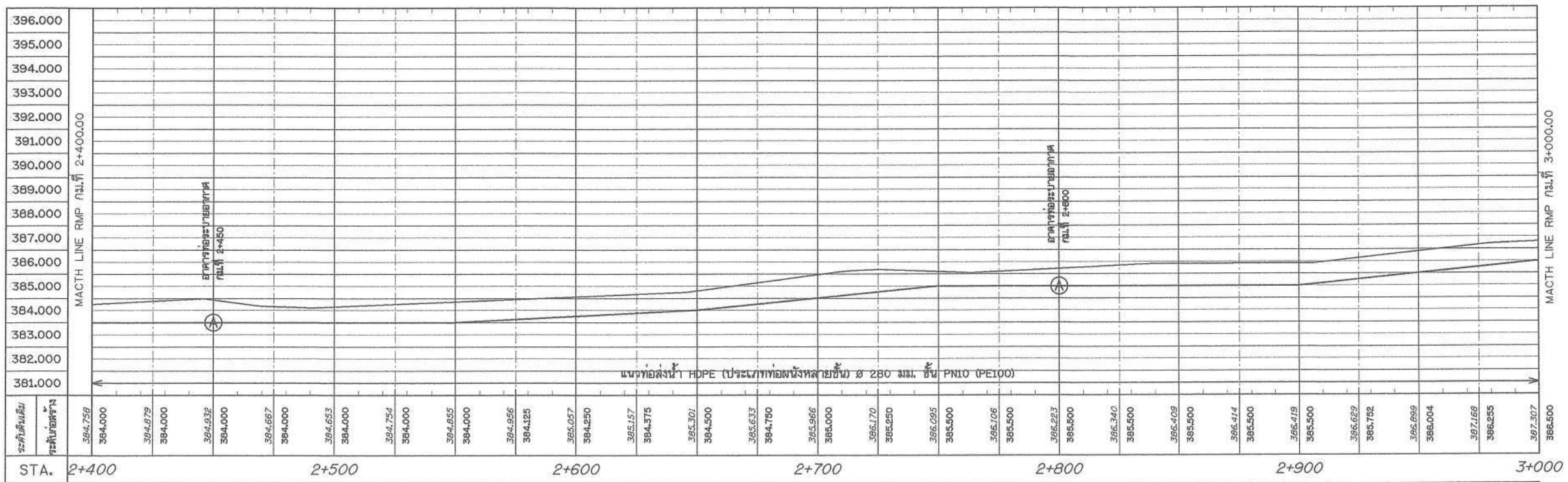
รูปตัดตามแนวยาว มาตราส่วน แนวตั้ง 1:500 แนวนอน 1:1,000
