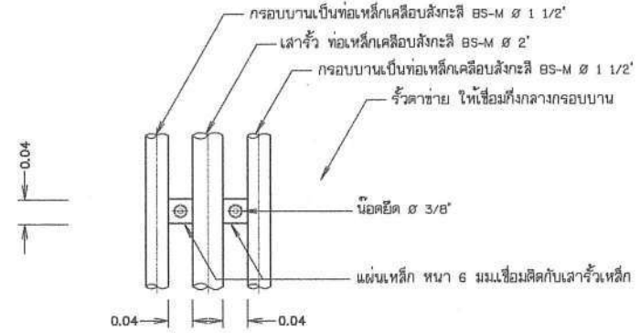
แบบขยายรายละเอียดแสดงการยึดระหว่างจั่วกับเสา
