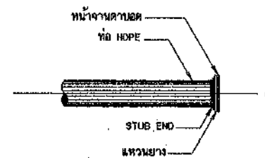
การปิดปลายท่อ ไม่แสดงขนาดคร่าวๆ
