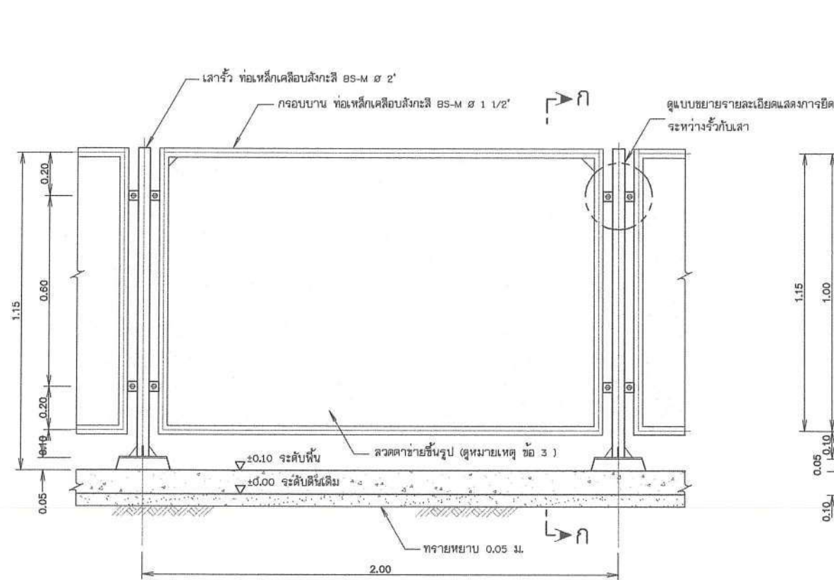
แบบขยายรั้วลวดด้าย
