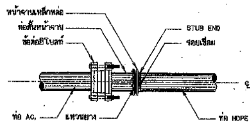
การบรรจุท่อ AC. กับท่อ HDPE ไม่แสดงขนาดคร่าวๆ
