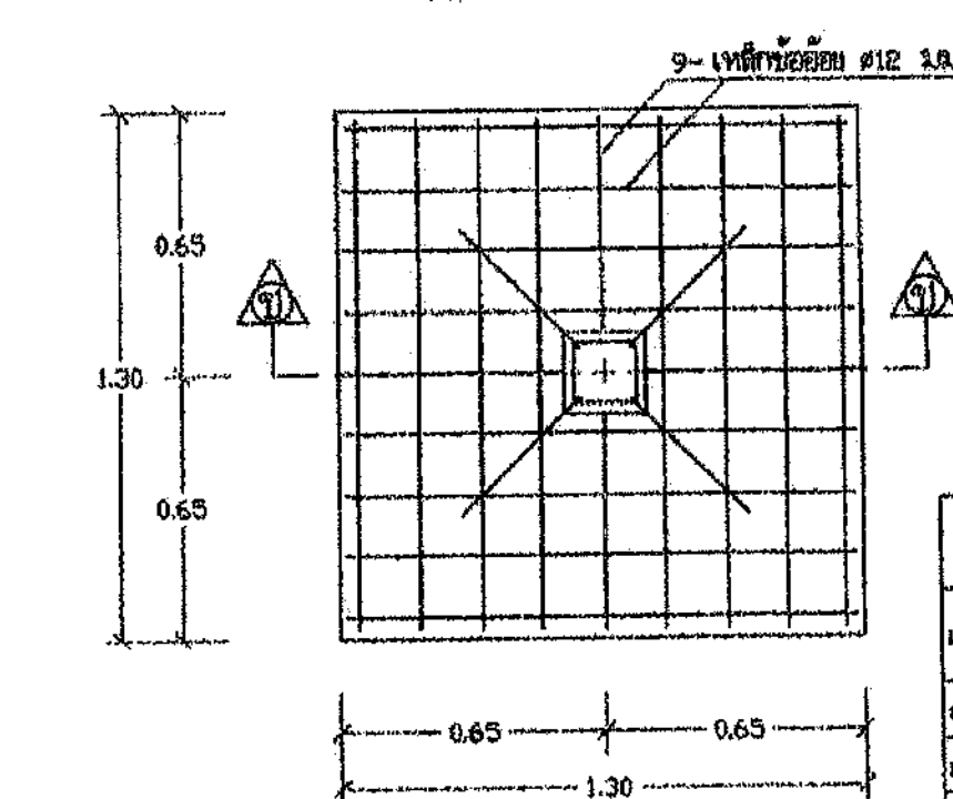
แบบขยายฐานราก F 2 (แบบตอกเข็ม) 1:20
