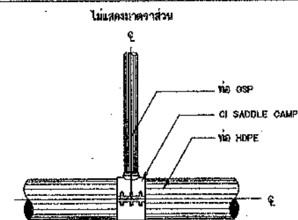
การบรรจุท่อสามทาง HDPE กับท่อ GSP แบบ CI SADDLE CLAMP สำหรับอาคารจุดปล่อยน้ำ อาคารประจวบประมาณ 100 เมตร อาคารท่าเรือประมาณ 100 เมตร กรณีท่อส่งน้ำขนาดเส้นผ่านศูนย์กลางน้อยกว่าหรือเท่ากับ 315 มม.
