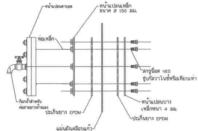
แบบขยายหน้าแปลนตาบอด scale NTC.
