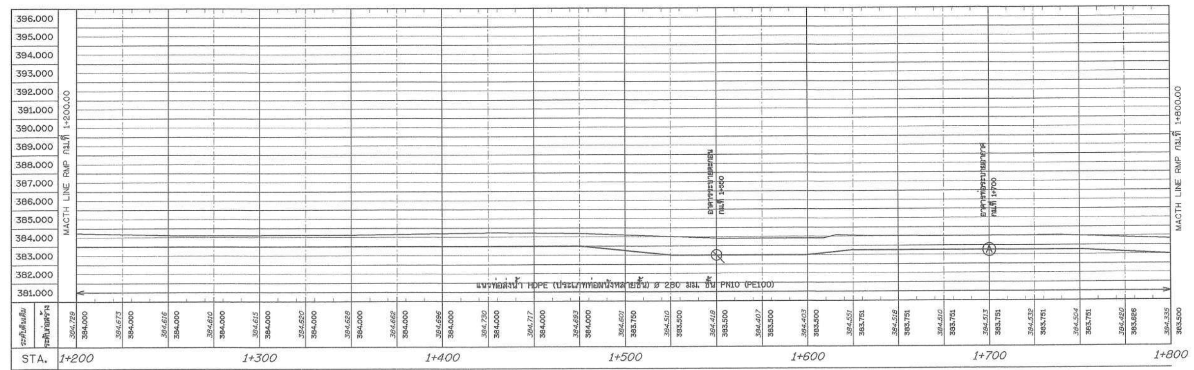
รูปตัดตามแนวยาว มาตราส่วน 1:500 แนวราบ 1:1,000
