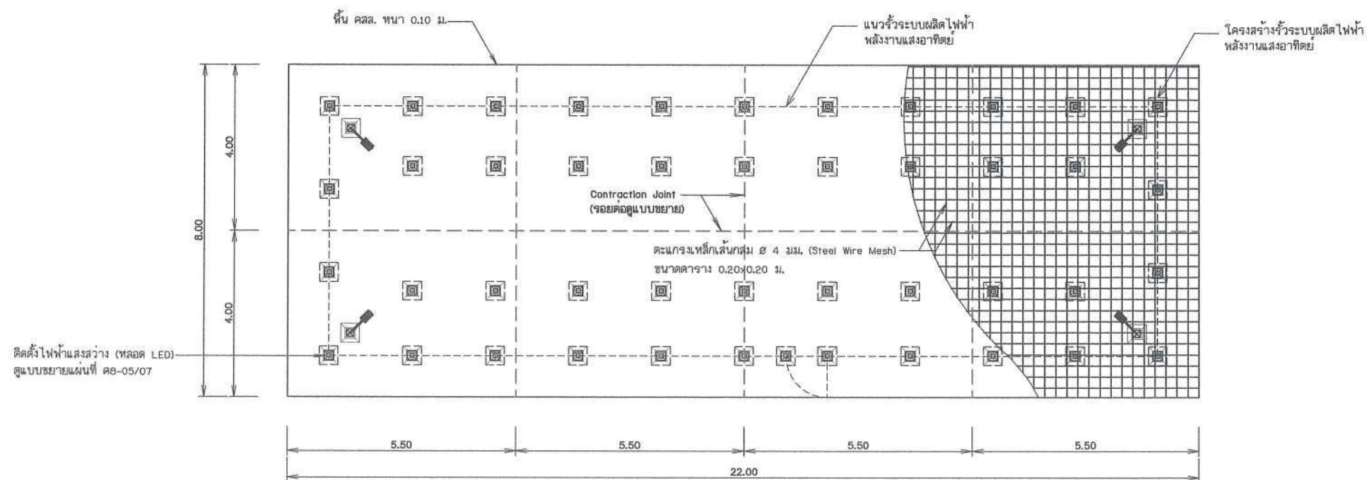
รูปขยายพื้นคอนกรีต ไม่มีมาตราส่วน
