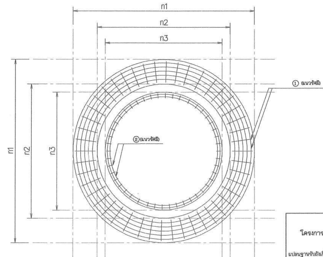
แปลนเหล็กเสริมขอบ รับถังเก็บน้ำ Fusion Bonded Epoxy (FBE)
