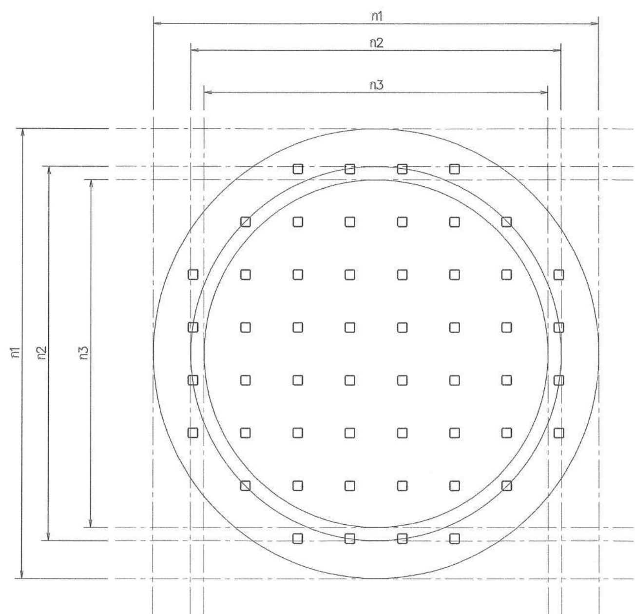
แปลนเสาเข็ม ถังเก็บน้ำ Fusion Bonded Epoxy (FBE) ขนาด 1,100 ลบ.ม. มาตราส่วน 1:100
