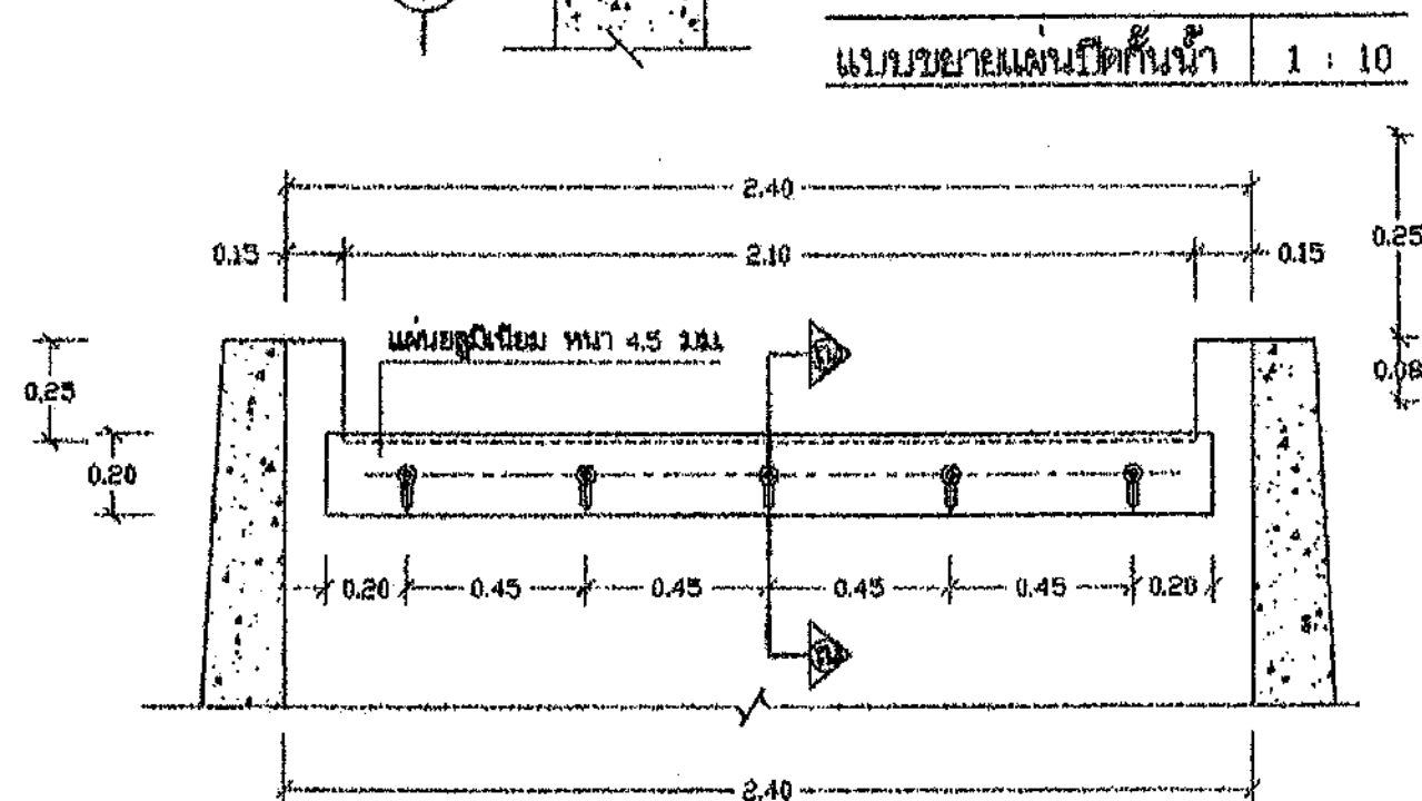
แบบขยายแผนปรับปรุงต้นน้ำ 1 : 20
