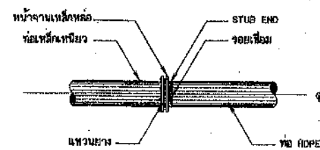
การบรรจุท่อเหล็กเหนียวกับท่อ HDPE ไม่แสดงขนาดคร่าวๆ
