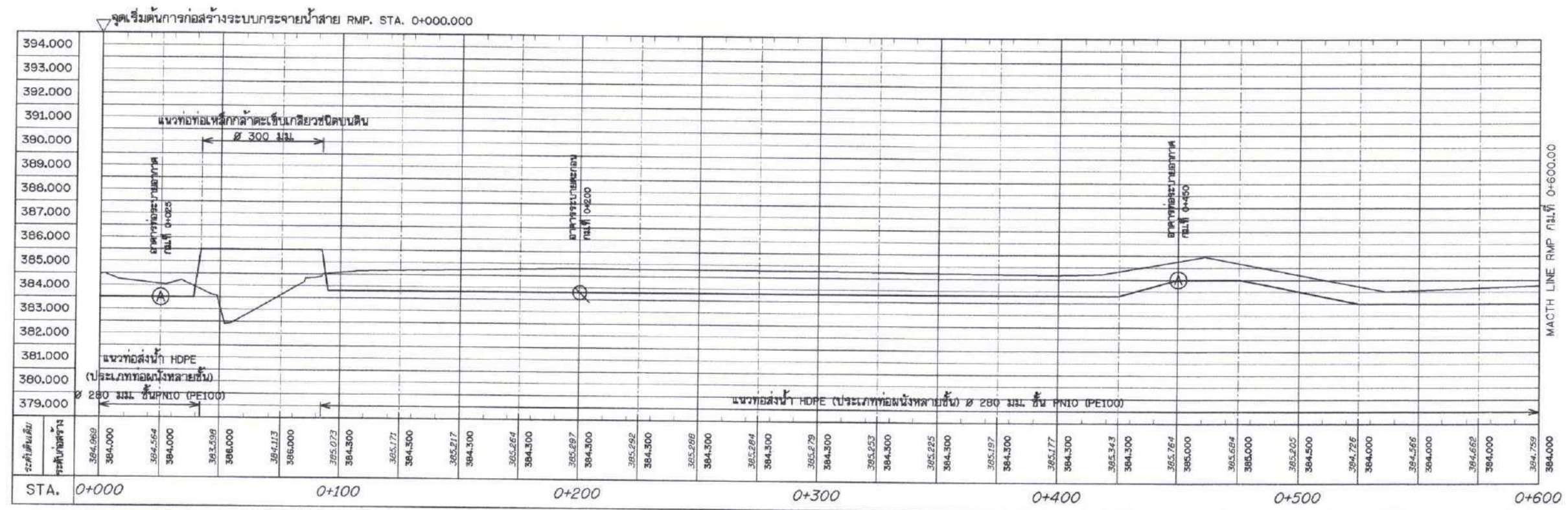
รูปตัดตามแนวยาว มาตราส่วน 1:500 แนวดิ่ง 1:500 แนวราบ 1:1,000
