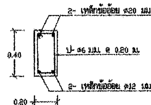
รูปตัด (ฎ) - (ฎ) 1:20
