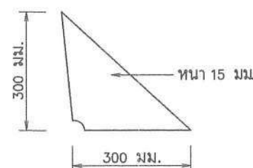
ภาพขยายหูช้าง จำนวน 12 ชิ้น โดยแบ่งระยะในการติดตั้งเท่ากัน
