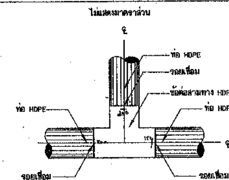
การบรรจุท่อสามทาง HDPE กับท่อ HDPE ไม่แสดงขนาดคร่าวๆ
