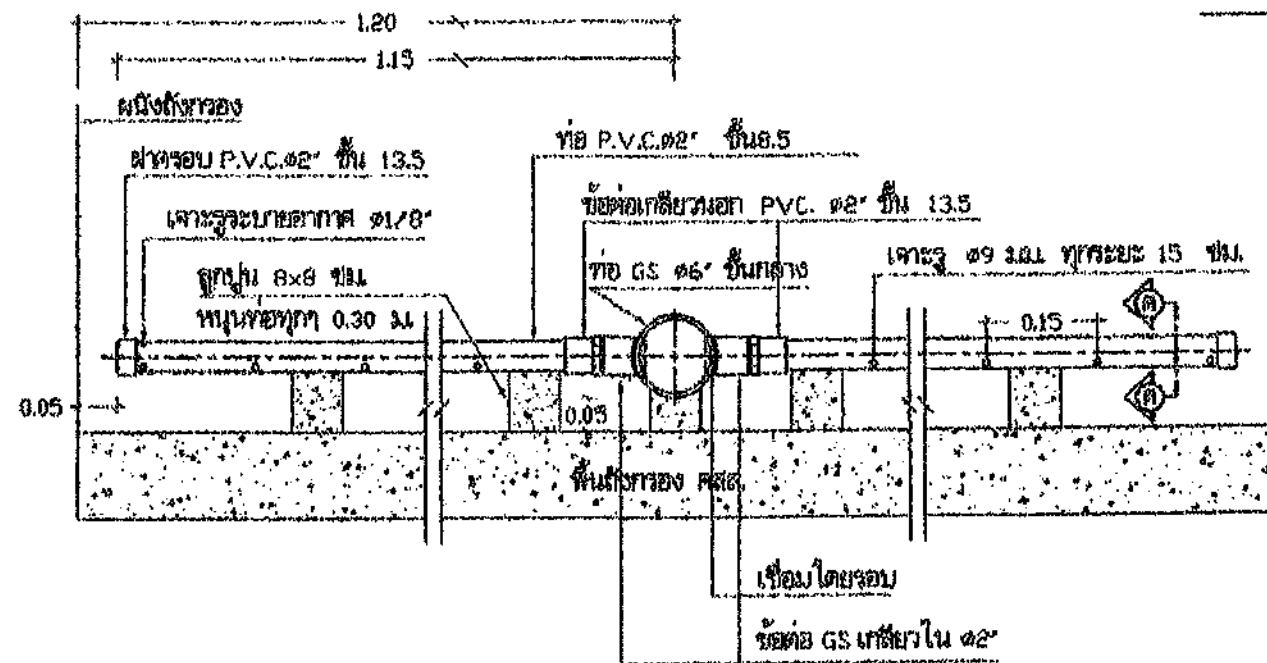
แบบขยายท่อทางปลา 1:20
