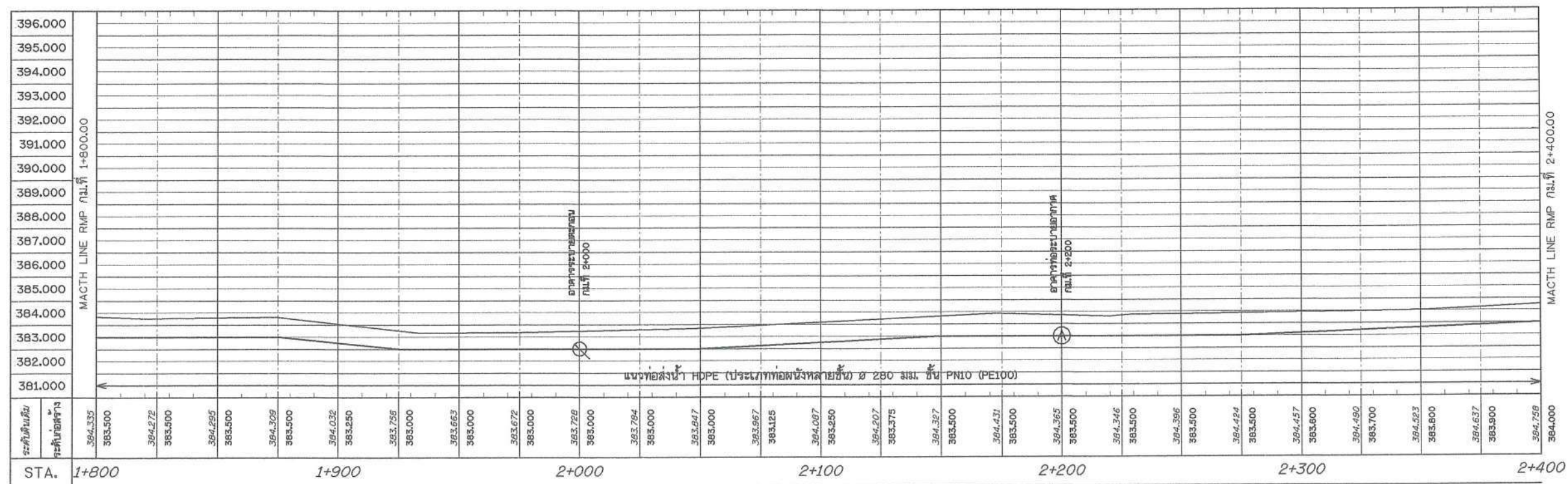
รูปตัดตามแนวยาว มาตราส่วน 1:500 แนวดิ่ง 1:500 แนวราบ 1:1,000
