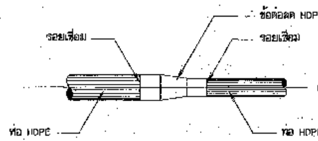
การบรรจุบ่อ HDPE กับข้อต่อเชื่อม HDPE
