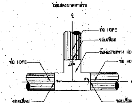
การบรรจุท่อสามทาง HDPE กับท่อ HDPE ไม่แสดงขนาดบางส่วน
