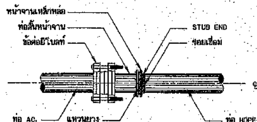
การบรรจุท่อ AC กับท่อ HDPE ไม่แสดงขนาดบางส่วน
