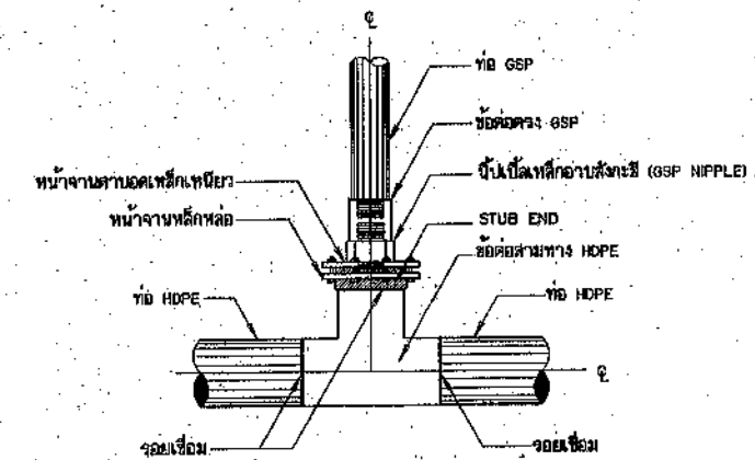
การบรรจุท่อสามทาง HDPE กับท่อ GSP แบบข้อต่อ (สำหรับอาคารชลประทาน อาคารประสูตประปา อาคารระบายน้ำเสีย) กรณีท่อส่งน้ำขนาดเส้นผ่านศูนย์กลางมากกว่า 315 มม.
