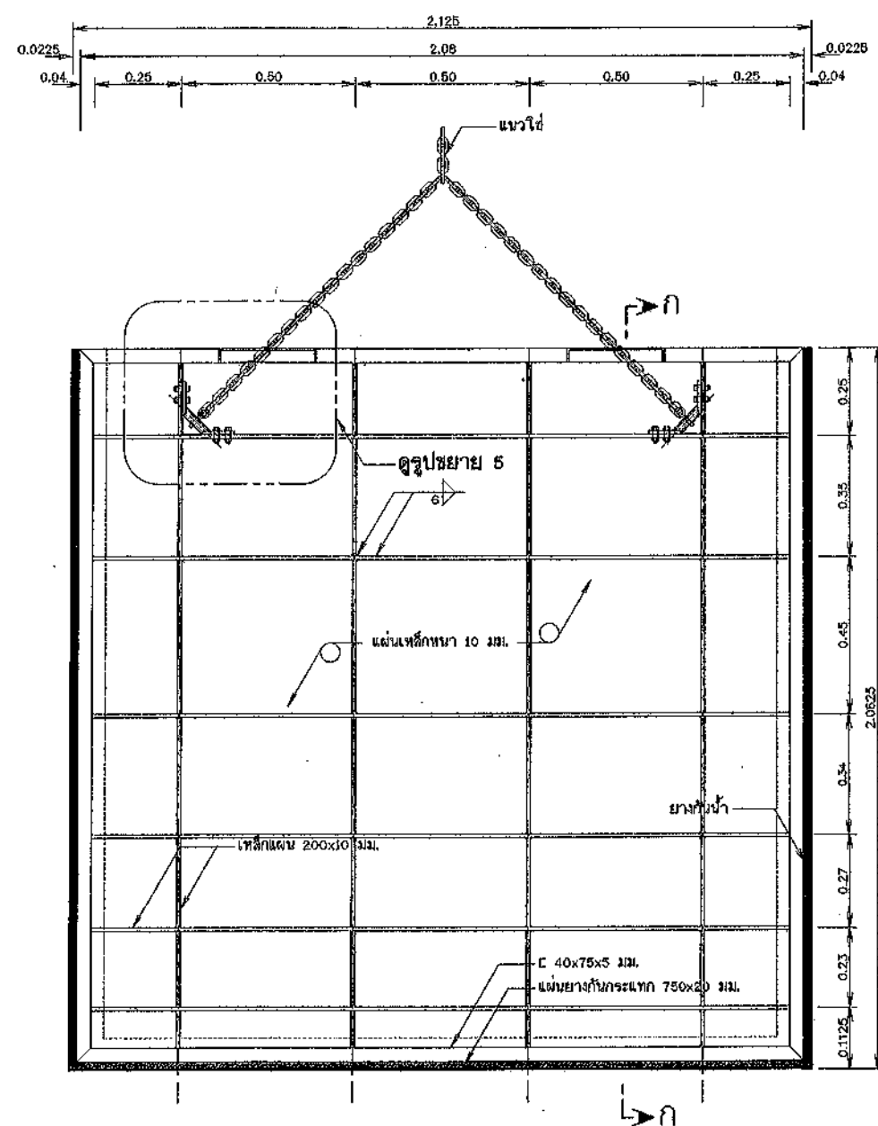
รูปด้านหลังบานประตูระบายทราย
