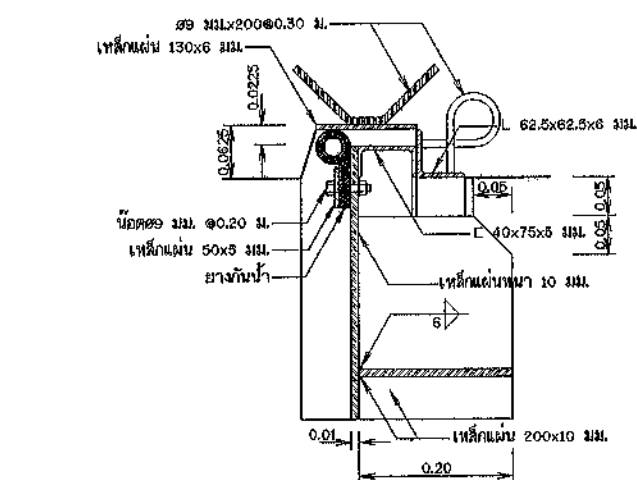
รูปขยายบานระบายด้านติดกำแพง
