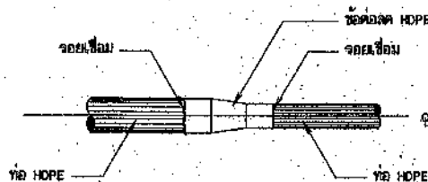
การบรรจุท่อ HDPE กับข้อต่อ HDPE ไม่แสดงขนาดบางส่วน
