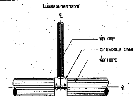
การบรรจุท่อสามทาง HDPE กับท่อ GSP แบบ CI SADDLE CLAMP (สำหรับอาคารชลประทาน อาคารประสูตประปา อาคารระบายน้ำเสีย) กรณีท่อส่งน้ำขนาดเส้นผ่านศูนย์กลางน้อยกว่าหรือเท่ากับ 315 มม.
