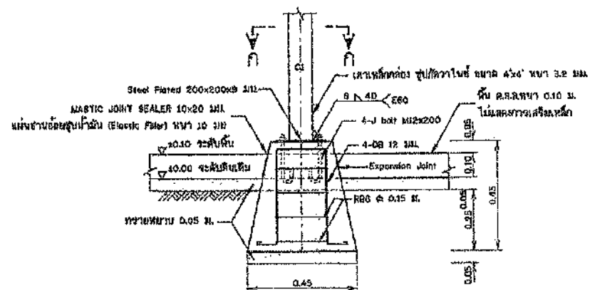
รูปขยายฐานรากโครงสร้างรับแรง F1 ตามแปลน คสล. ยกเว้นรูปหล่อคอนกรีต
