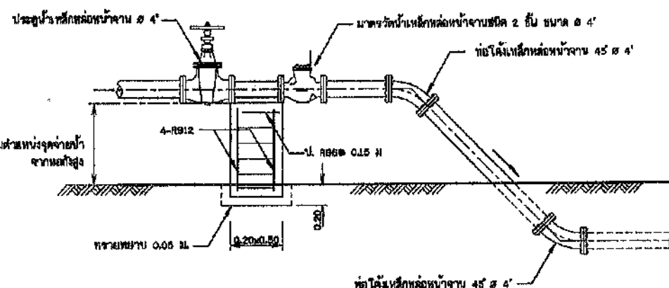
14. การติดตั้งมาตรวัดน้ำบนพื้นดิน ๔" ไม่แสดงขนาดส่วน
