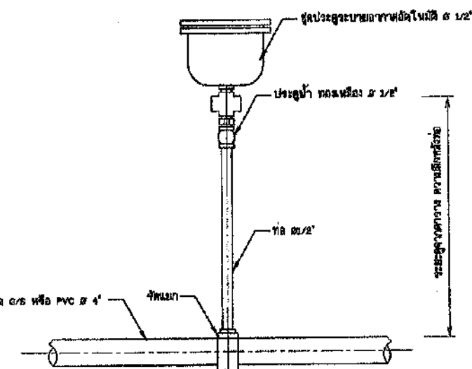
12. การติดตั้งประตูละบายอากาศอัตโนมัติ ไม่แสดงขนาดส่วน
