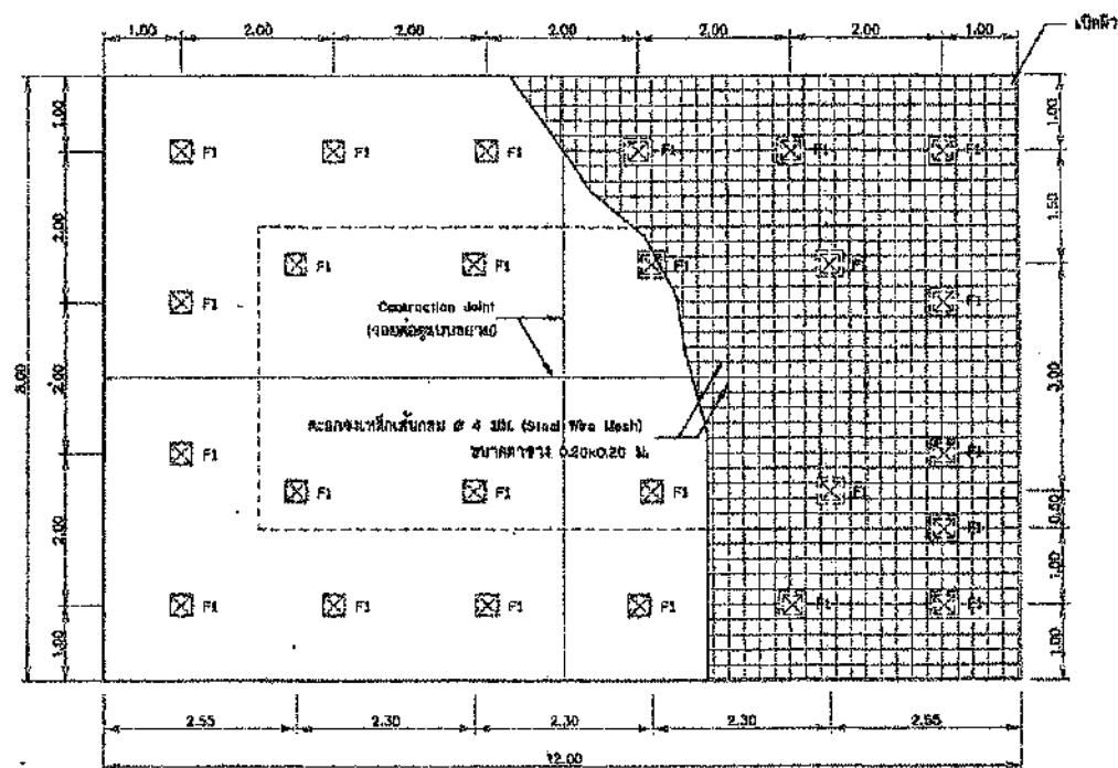
รูปขยายพื้นคอนกรีต ไม่แสดงขนาดฐาน
