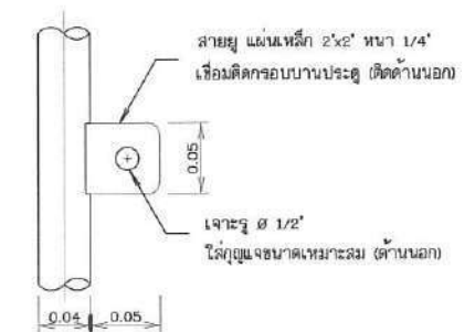
แบบขยายสายผูก ไม่แสดงมาตราส่วน
