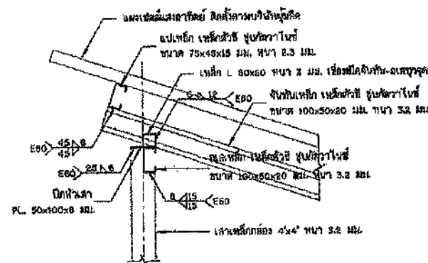
รูปขยาย การติดตั้งโครงหลังคา ไม่แสดงขนาดฐาน
