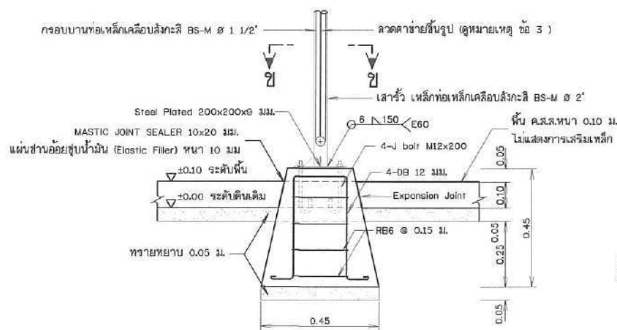
รูปขยายฐานรากโครงสร้างรับแผง F1 (ต่อมอด คสล. หล่อสำเร็จรูปพร้อมติดตั้ง) ไม่แสดงมาตราส่วน
