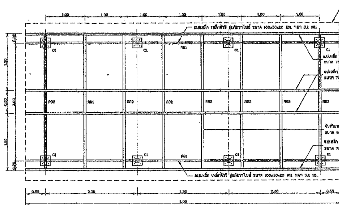
แปลนฐานรากและโครงหลังคา ไม่แสดงขนาดฐาน
