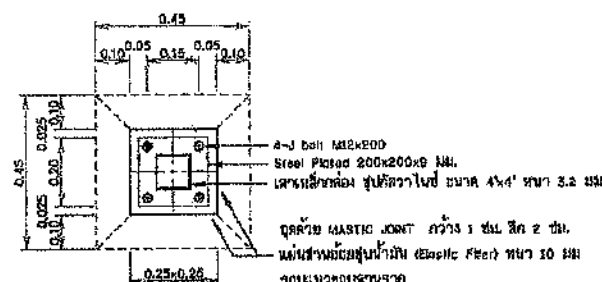
รูปตัด ก-ก ไม่แสดงขนาดฐาน
