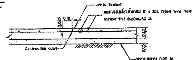
แบบขยายรอยต่อพื้น (Contraction Joint) ไม่แสดงขนาดฐาน
