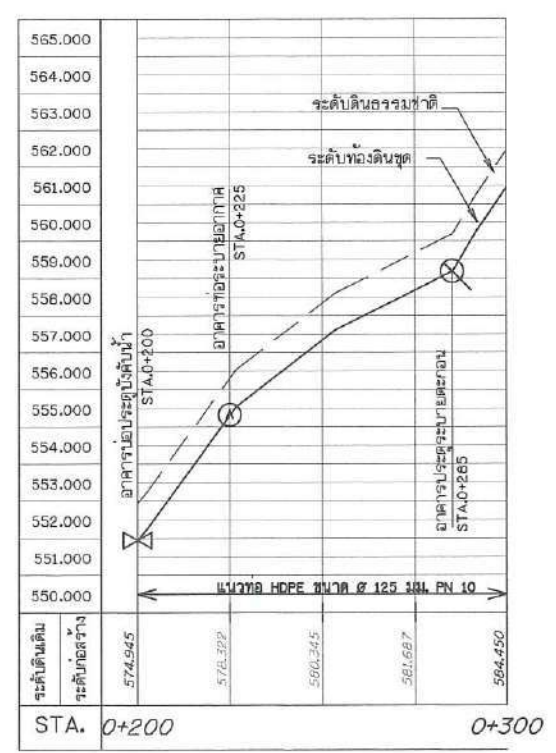
รูปตัดตามแนวยาว
