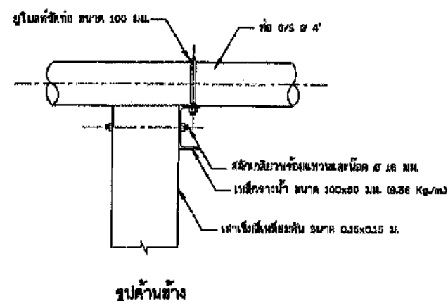
13. เสาต่อม่อรับท่อชุด และแบบขยายอุปกรณ์รั้วท่อ ไม่แสดงขนาดส่วน
