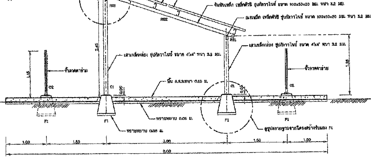
รูปด้านข้าง ไม่แสดงขนาดฐาน
