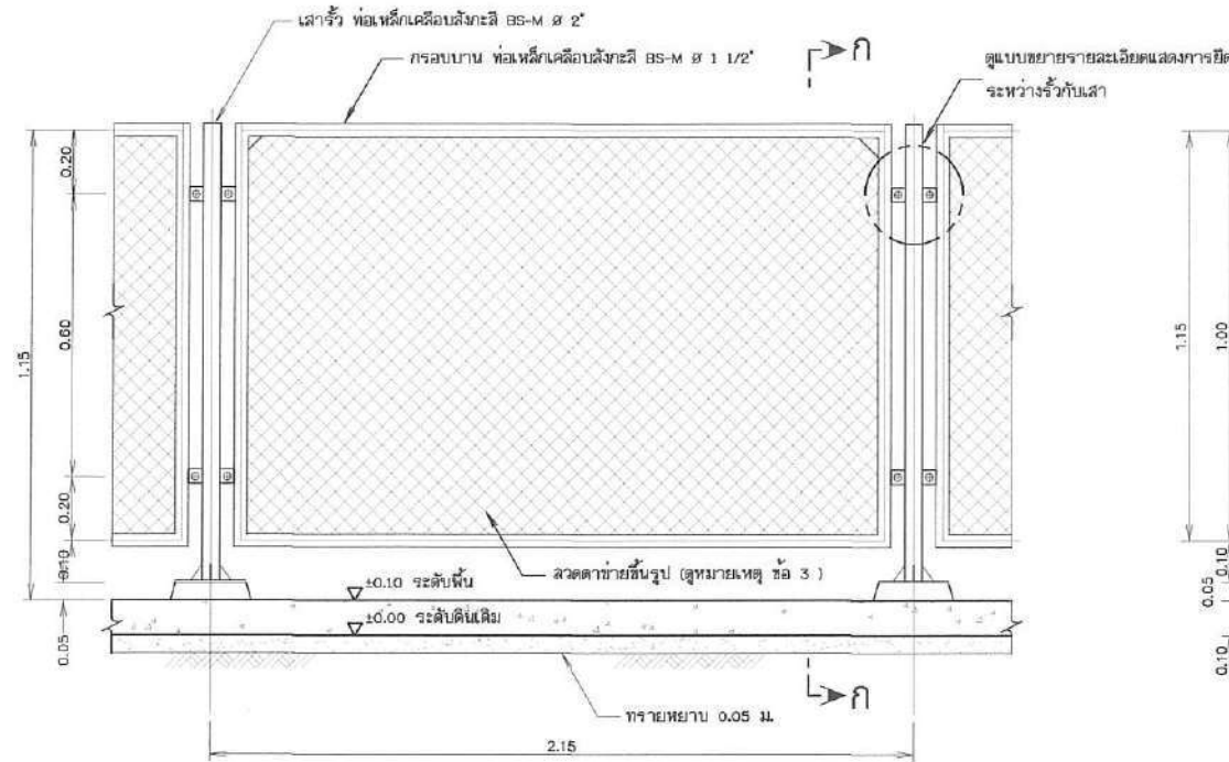
แบบขยายหัวลวดตาข่าย ไม่แสดงมาตราส่วน
