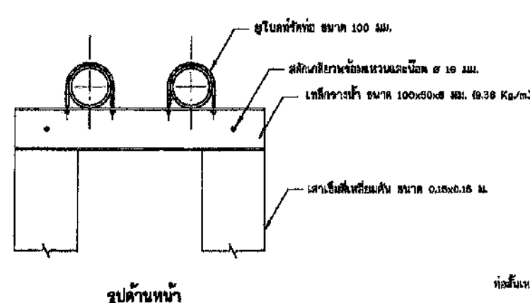
13. เสาต่อม่อรับท่อชุด และแบบขยายอุปกรณ์รั้วท่อ ไม่แสดงขนาดส่วน
