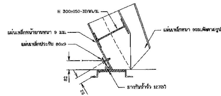
รูปขยายยางกันน้ำรั่วใต้บ้าน มาตราส่วน 1:10
