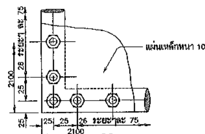
รูปขยาย 1 มาตราส่วน 1:4
