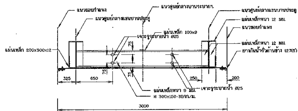
รูปตัด ข - ข มาตราส่วน 1:20
