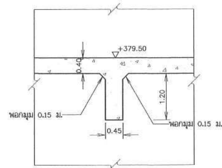
รูปขยาย 2
