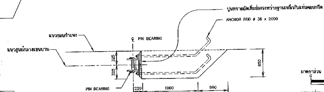
รูปตัด ข - ข
