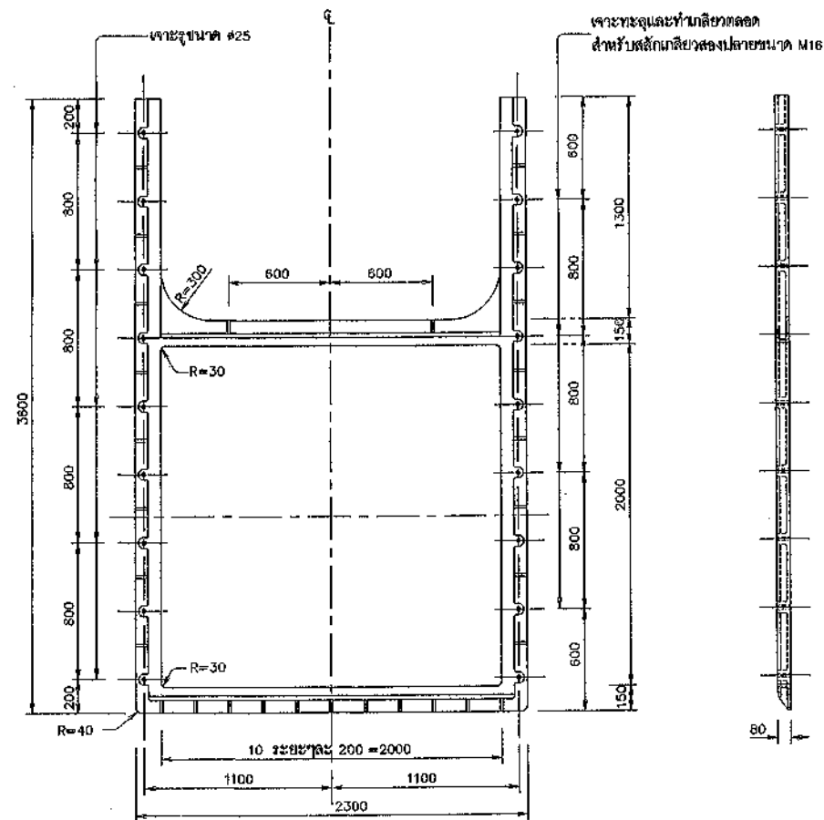
กรอบบาน เหล็กหล่อ มาตราส่วน 1:20
