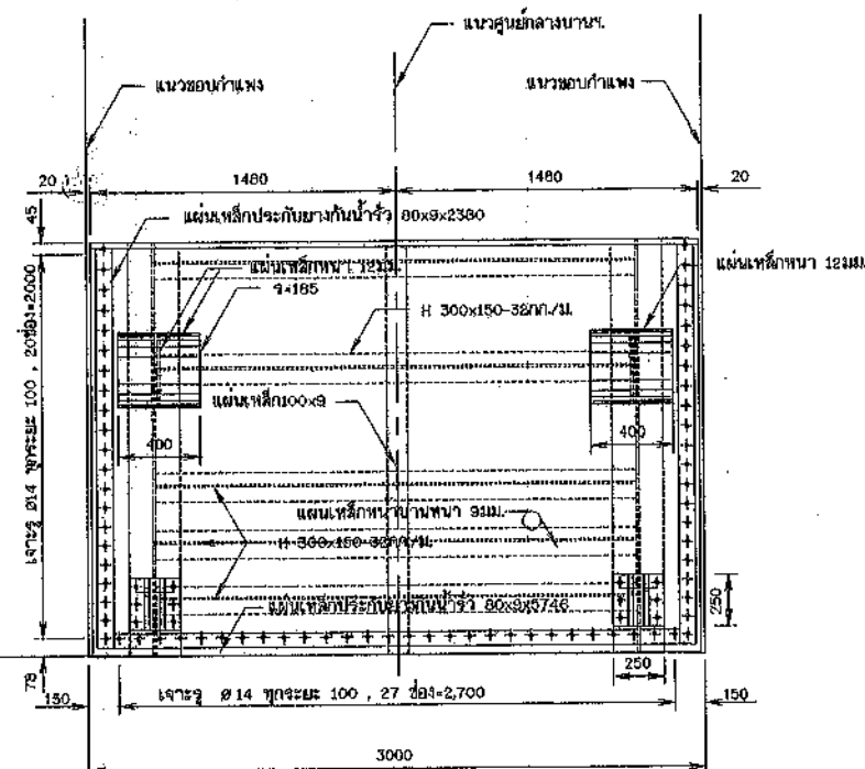
บานระบายด้านเหนือ
