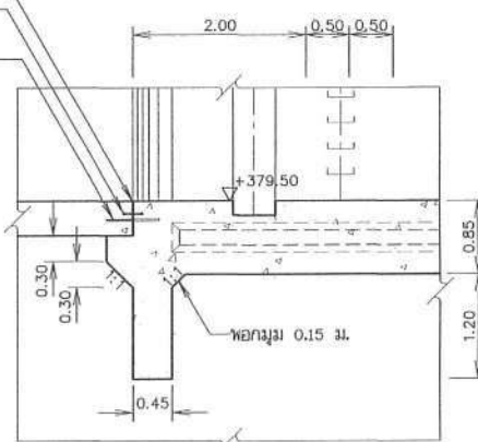
รูปขยาย 3
