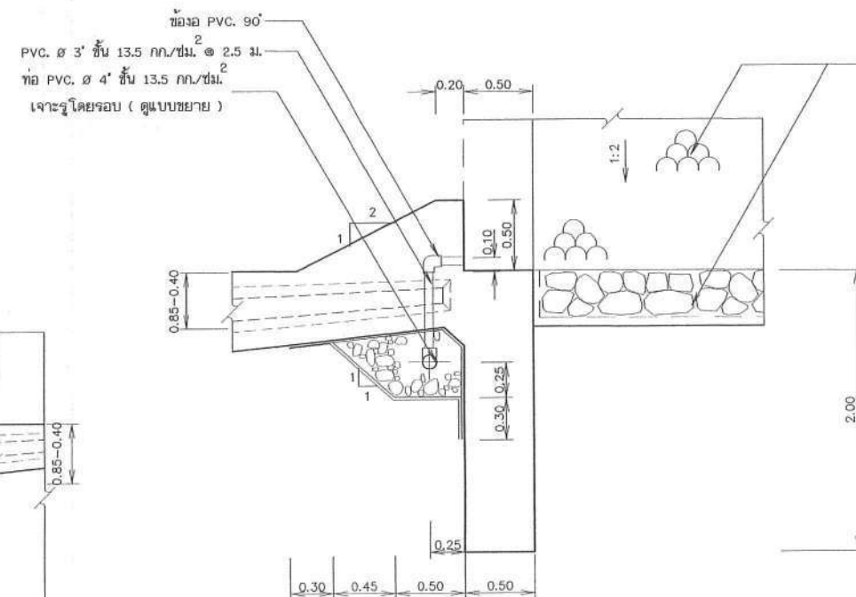
รูปขยาย 5
