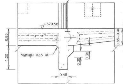
รูปขยาย 4
