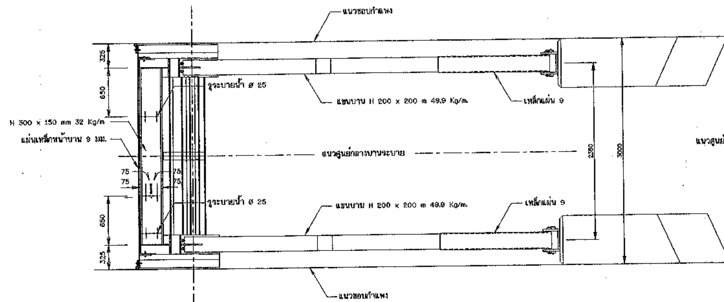
แปลนขนาน
