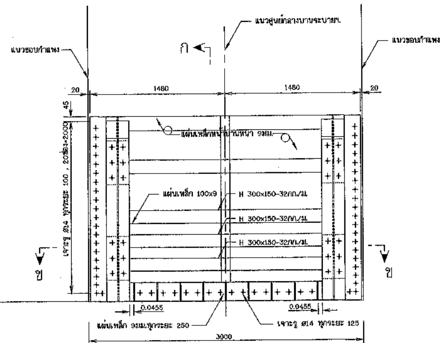
บ้านระบายด้านท้ายน้ำ มาตราส่วน 1:20
