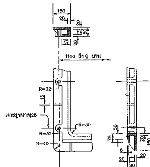
รูปขยายกรอบบาน มาตราส่วน 1:10
