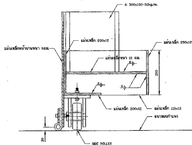
รูปตัดแสดงการติดตั้งล้อด้านข้าง
