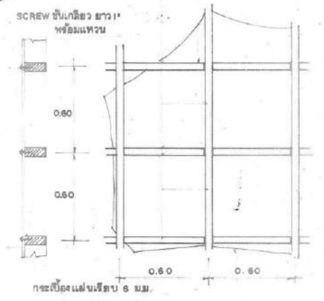
รูปขยายโครงฝ้า 18 20
