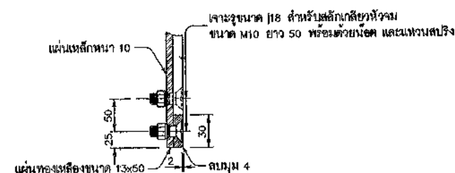
รูปขยาย 2 มาตราส่วน 1:4
