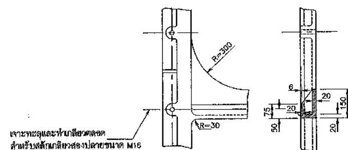
กรอบบาน เหล็กหล่อ มาตราส่วน 1:20
