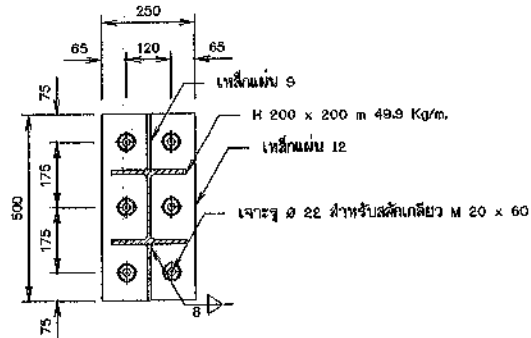
รูปตัด ก - ก
