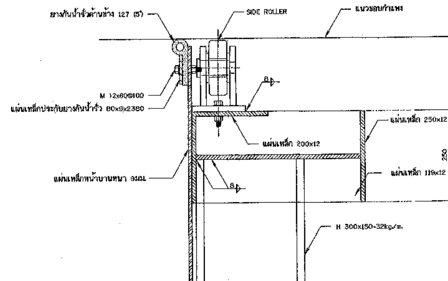
การติดตั้งยางกันน้ำรั่วด้านข้างและ SIDE ROLLER
