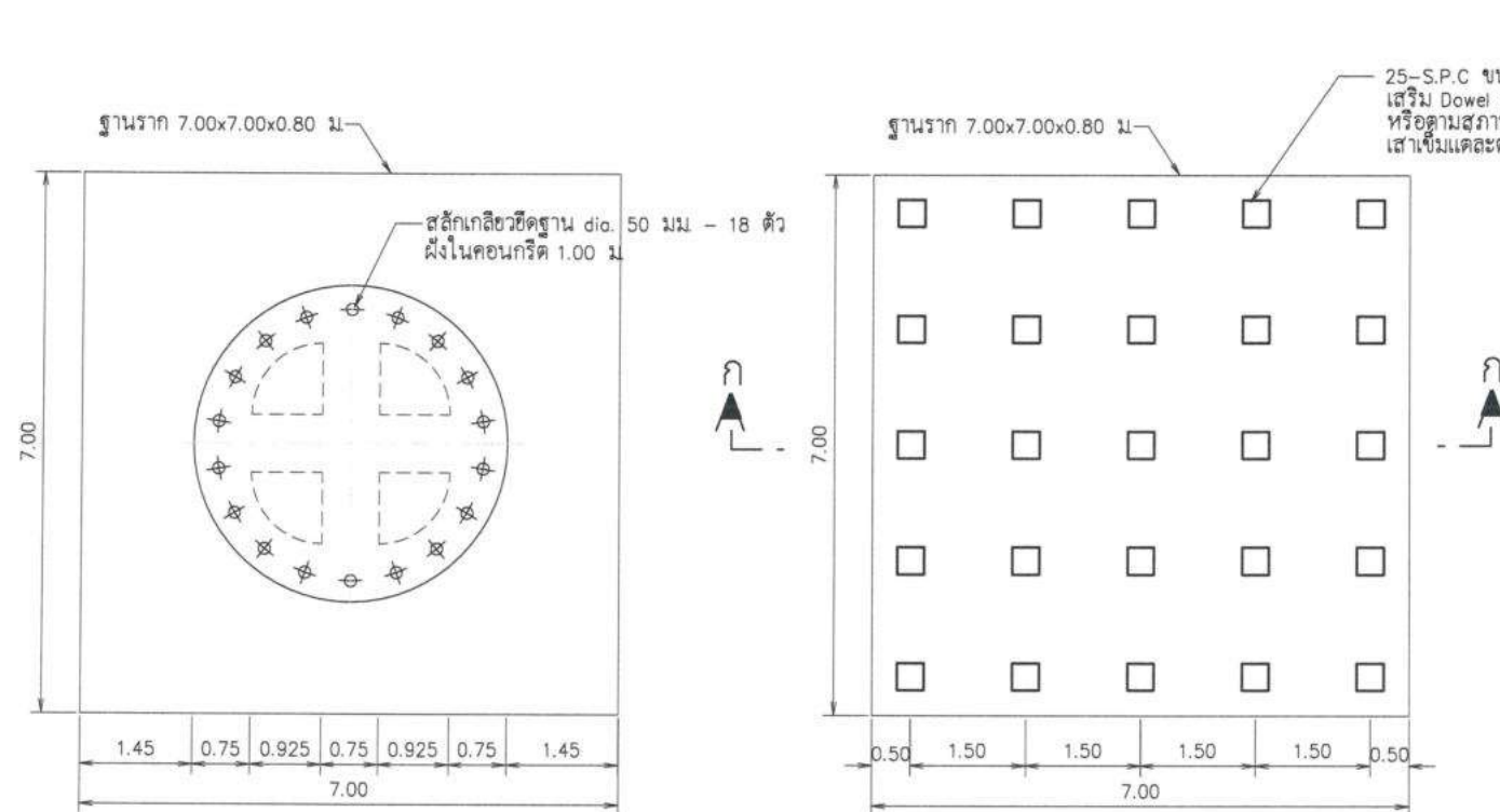
แปลนฐานรากหอดึงสูง (แบบเสาเข็ม)
