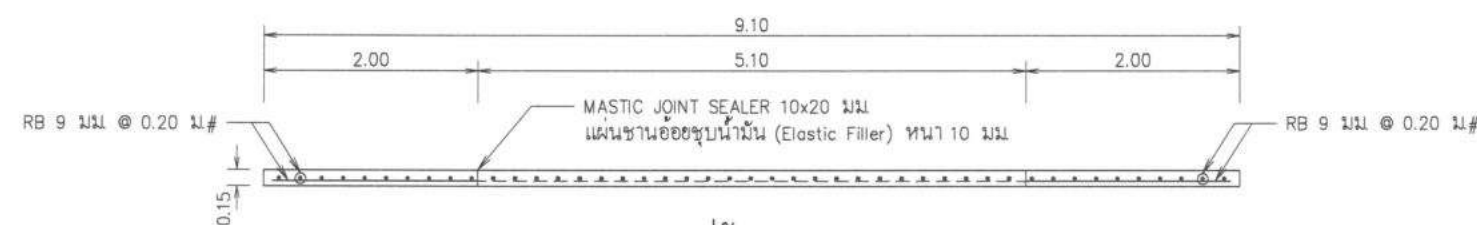
รูปตัด ข-ข
