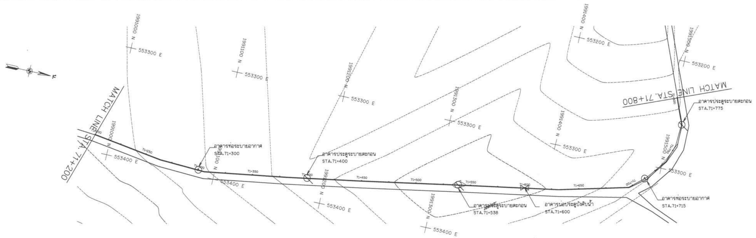
แปลนทั่วไป STA. 71+200 - 71+800
