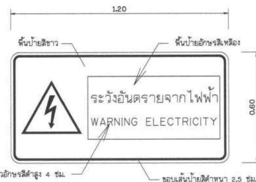
แบบขยายป้ายแจ้งเตือน มาตราส่วน No Scale
