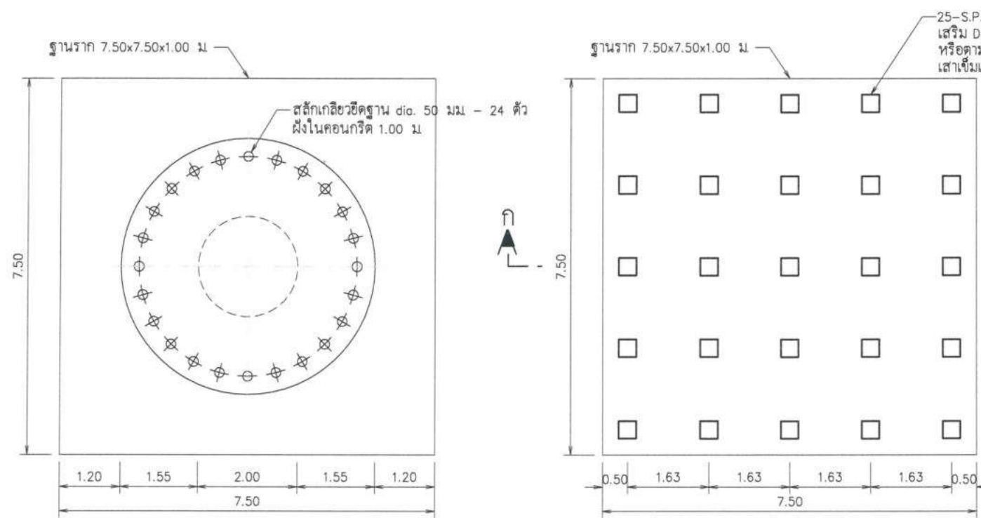
แปลนฐานรากหอดึงสูง (แบบเสาเข็ม)
