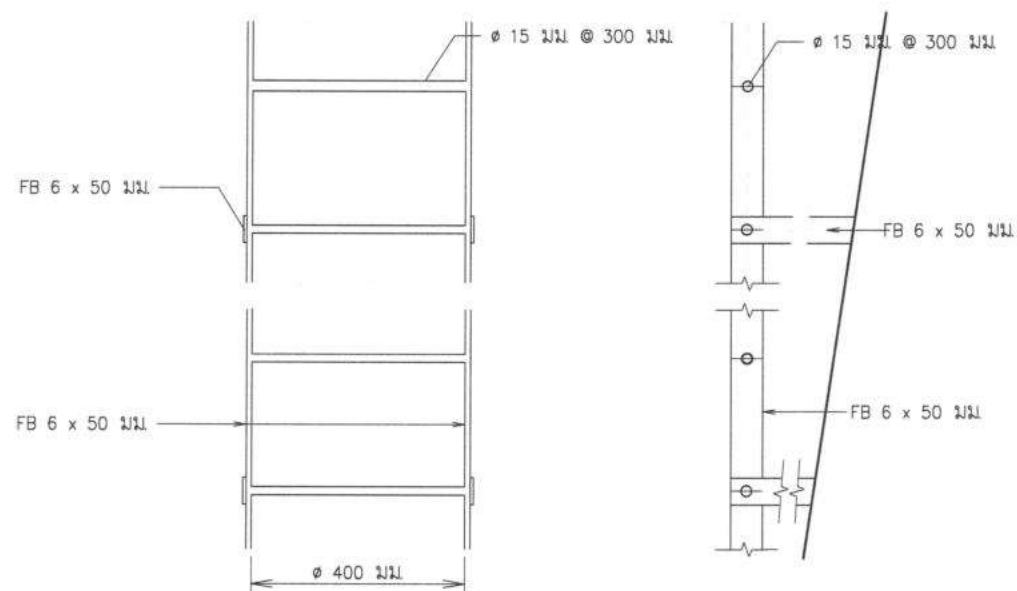
ภาพขยายบันได "1" ภายในห้องเหล็กเก็บน้ำ ไม่แสดงมาตราส่วน
