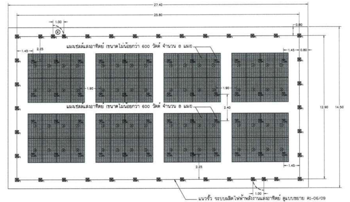
แปลนการติดตั้งแผงเซลล์แสงอาทิตย์ ขนาด 22 กิโลวัตต์ พร้อมรั้ว
