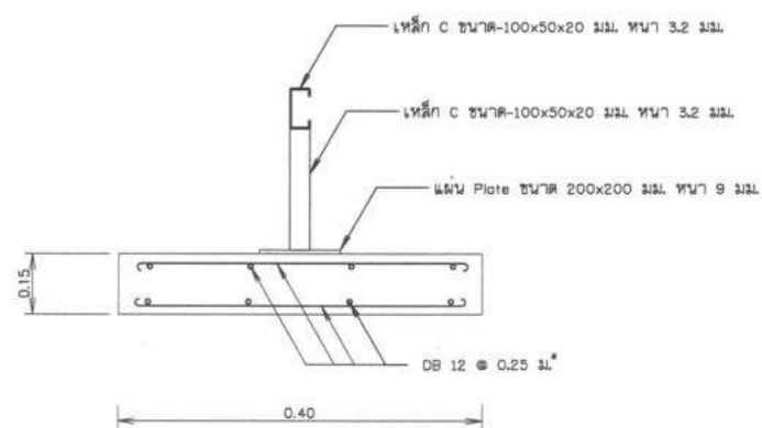
รูปด้านโครงสร้างรับท่อ ไม่แสดงมาตราส่วน
