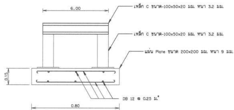
รูปด้านโครงสร้างรับท่อน้ำดิน ไม่แสดงมาตราส่วน
