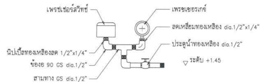
แบบขยายสวิทช์ควบคุมและแจ้งความดัน ไม่แสดงมาตราส่วน
