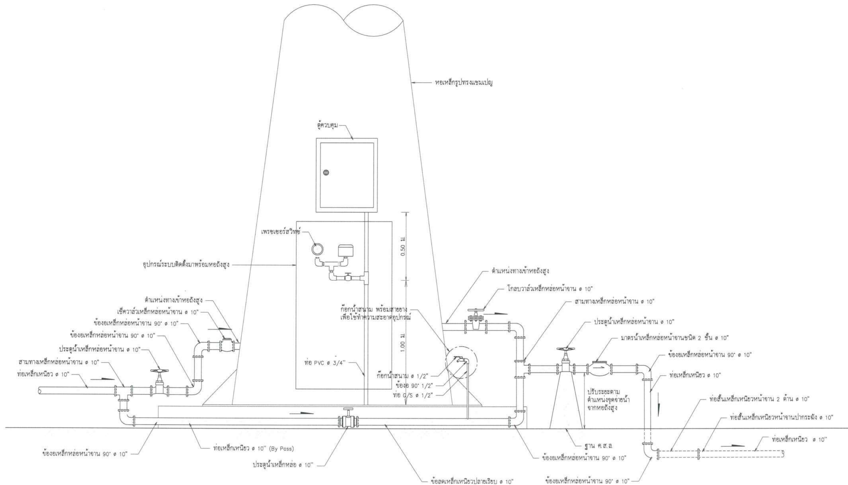
รูปแสดงรายละเอียดการต่อท่อและอุปกรณ์ออกจากถังเหล็กรูปทรงแฉะแปญ
