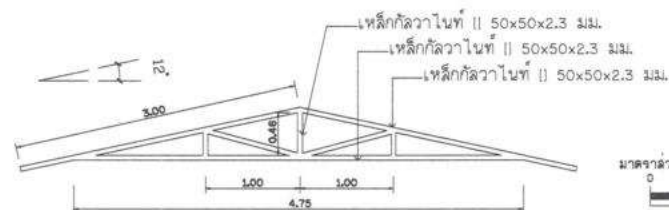
แบบขยาย T3 มาตราส่วน 1 : 100
