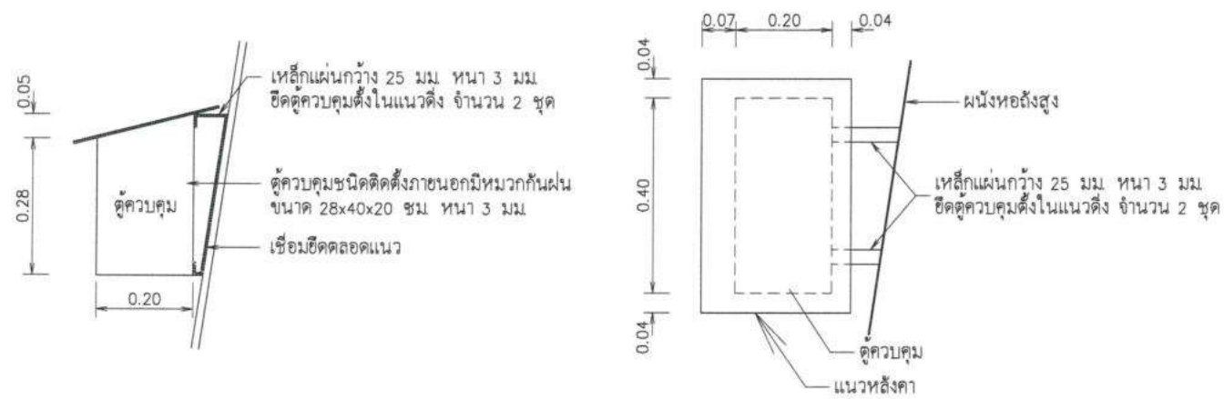
แบบขยายตัวควบคุม ไม่แสดงมาตราส่วน
