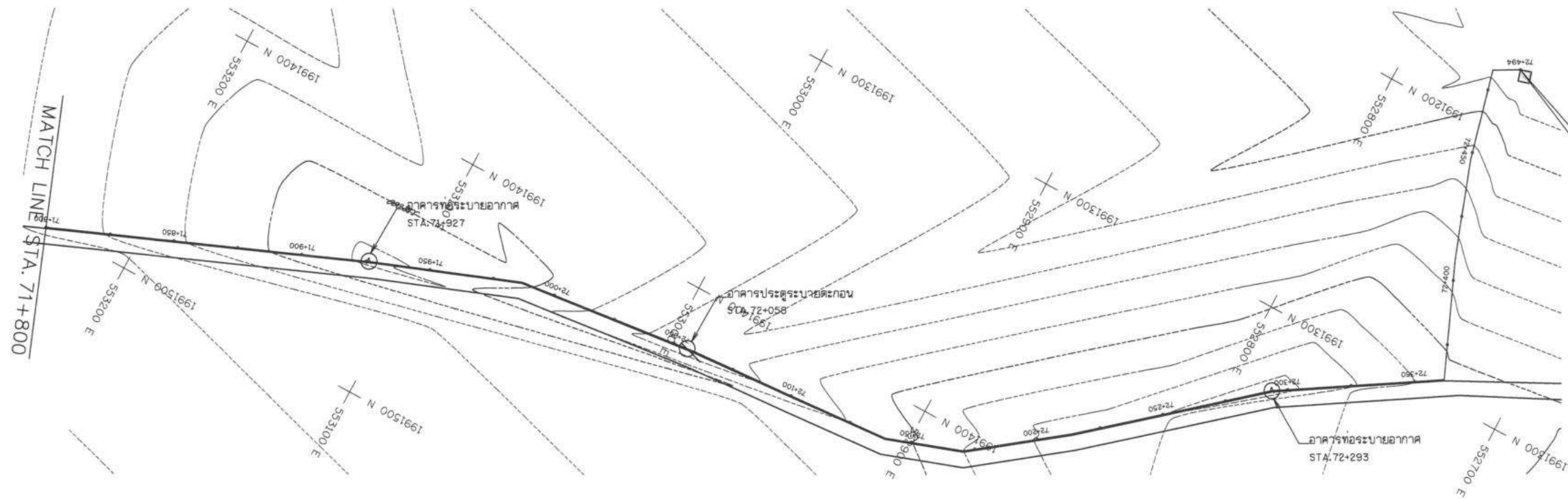
แปลนทั่วไป STA. 71+800 - 72+494
