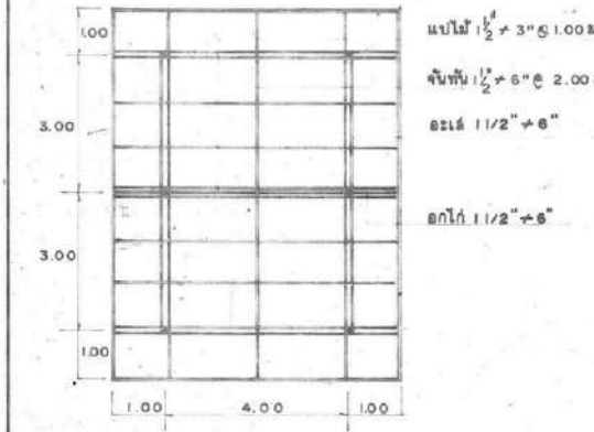
แปลนโครงเหล็ก 18100
