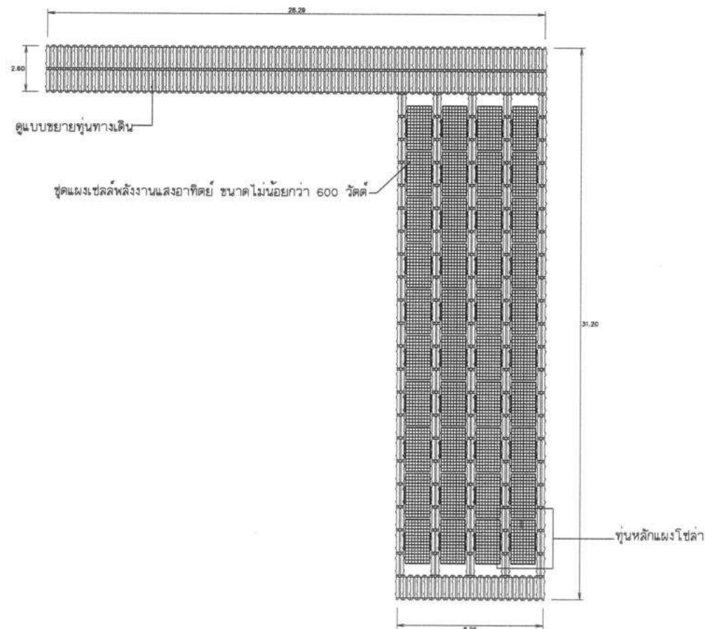
ระบบกระจายน้ำพลังงานแสงอาทิตย์ ขนาด 15 กิโลวัตต์
