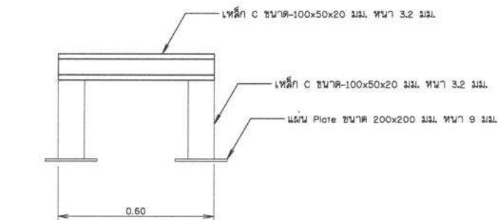
รูปด้านโครงสร้างรับท่อน้ำ ไม่แสดงมาตราส่วน
