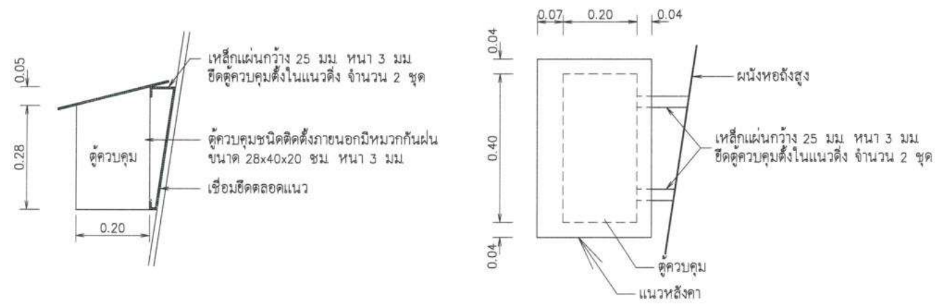
แบบขยายตุ้ควคุม ไม่แสดงมาตราส่วน
