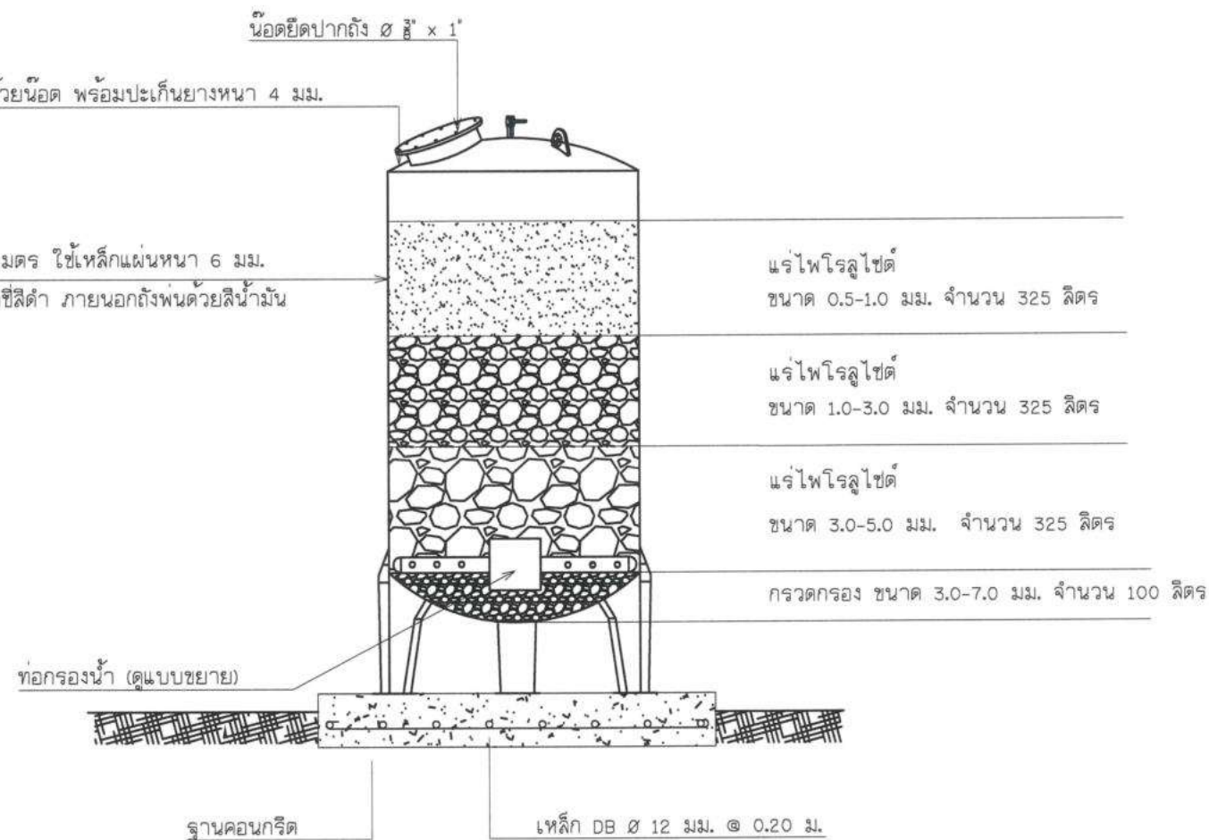
แบบแสดงฐานรากและส่วนประกอบสารกรองถังกรองน้ำ
