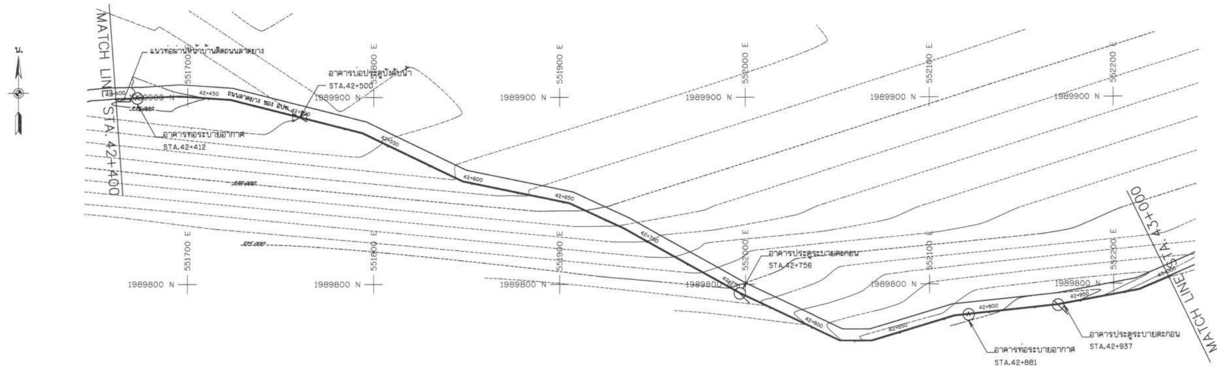
แปลนทั่วไป STA. 42+400 - 43+000
