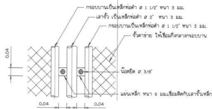
แบบขยายรายละเอียดแสดงการยึดระหว่างหัวกับเสา ไม่แสดงมาตราส่วน
