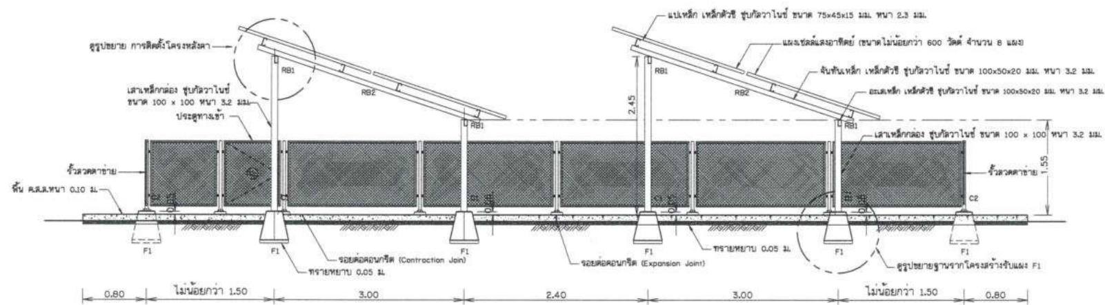
รูปด้านข้าง
