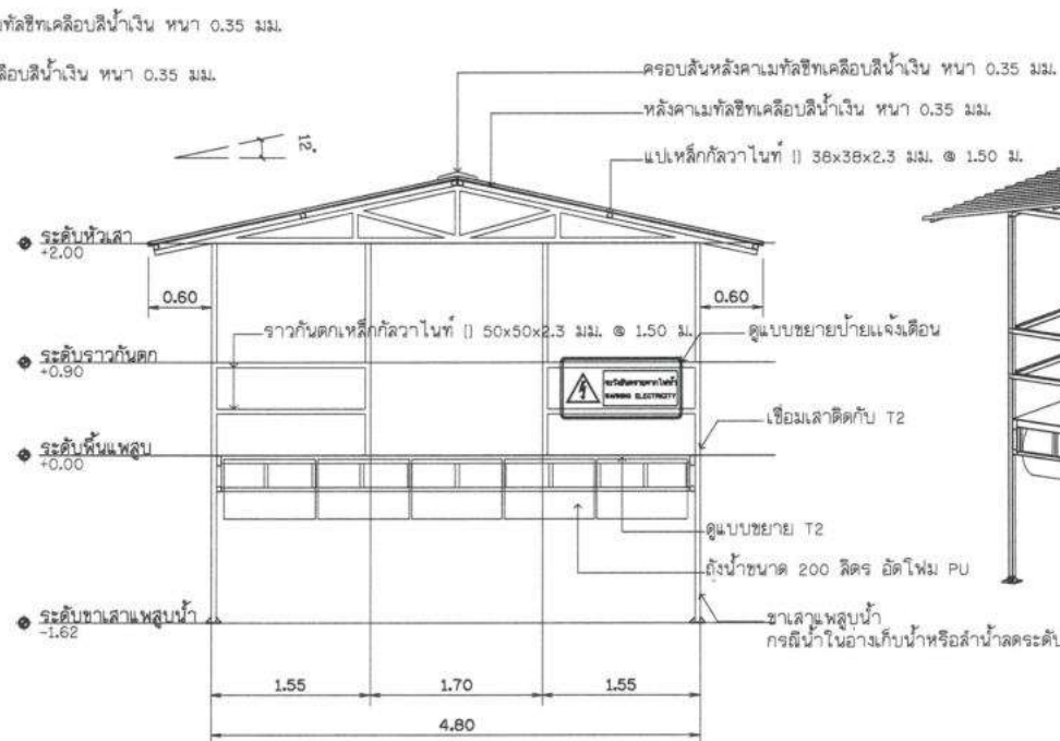
รูปด้าน 1 มาตราส่วน 1 : 100
