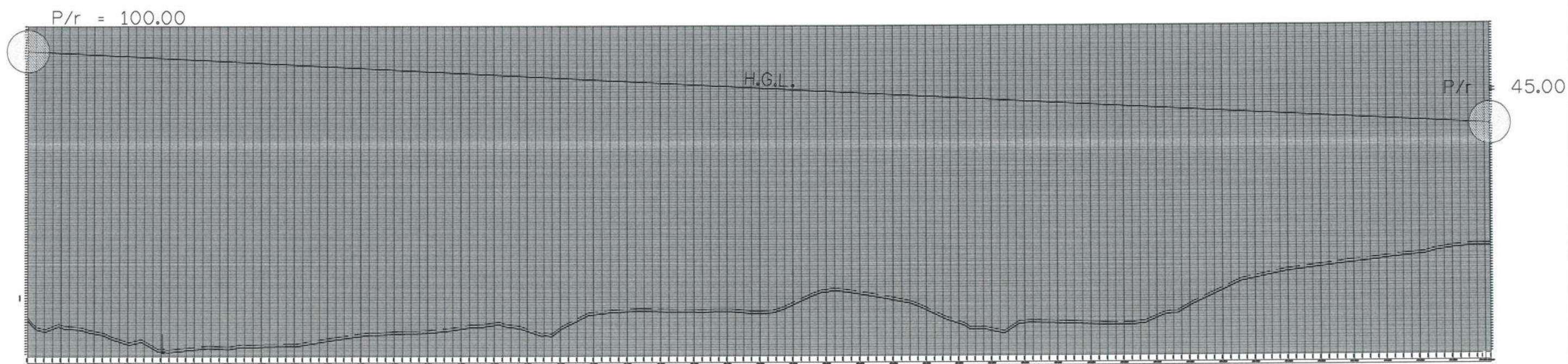
รูปตัด H.G.L. STA. 20+000 - 22+337 มาตรฐาน 1:1,000
