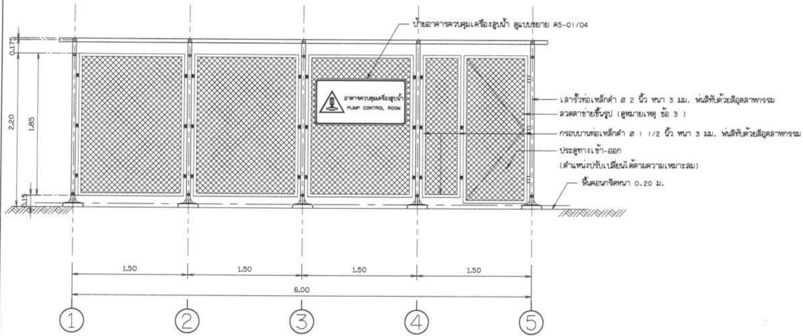
แบบขยายรูป 1 ไม่แสดงมาตราส่วน
