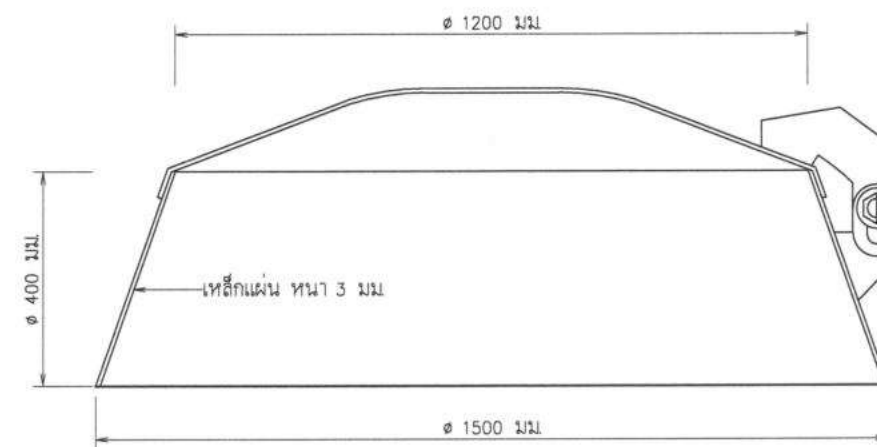
ภาพขยายทางคนเข้า-ออก "1" ไม่แสดงมาตราส่วน
