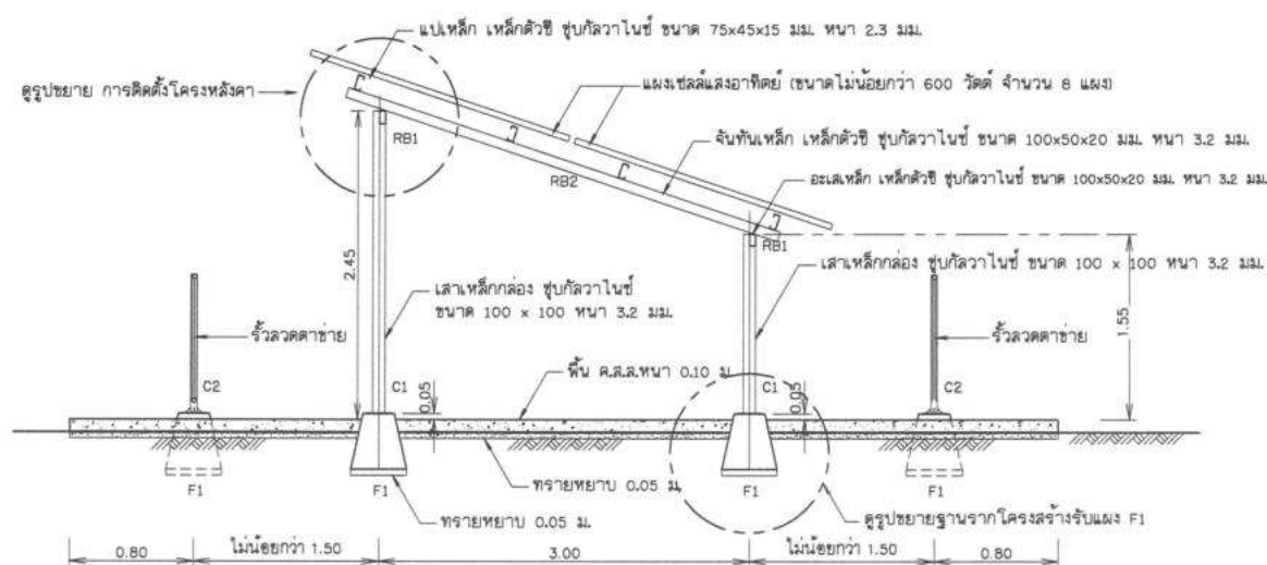
รูปด้านข้าง
