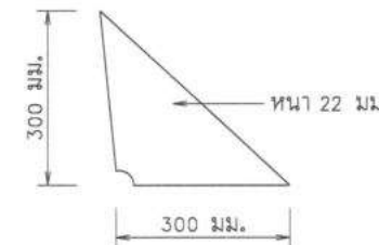
ภาพขยายหูช้าง จำนวน 12 ชิ้น โดยแบ่งระยะในการติดตั้งให้เท่ากัน
