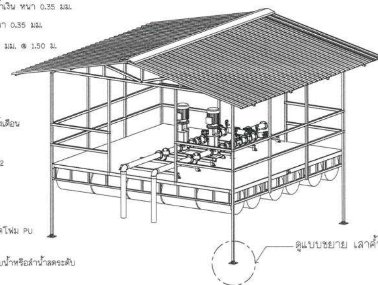
ISOMETRIC มาตราส่วน 1 : 100
