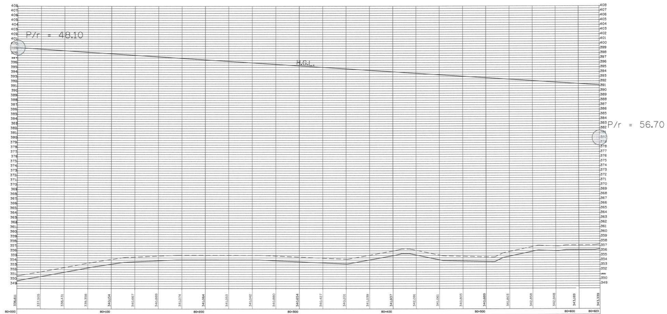
รูปตัด H.G.L. STA. 80+000 - 80+623 มาตราส่วน 1:1,000
