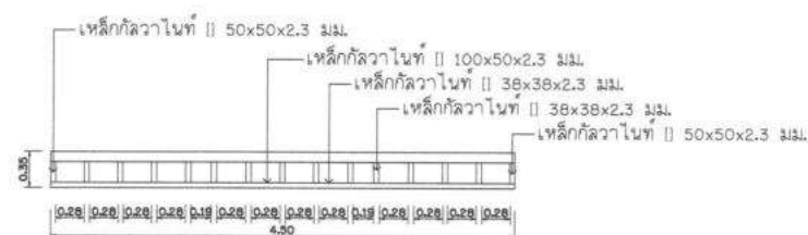
แบบขยาย T1 มาตราส่วน 1 : 100
