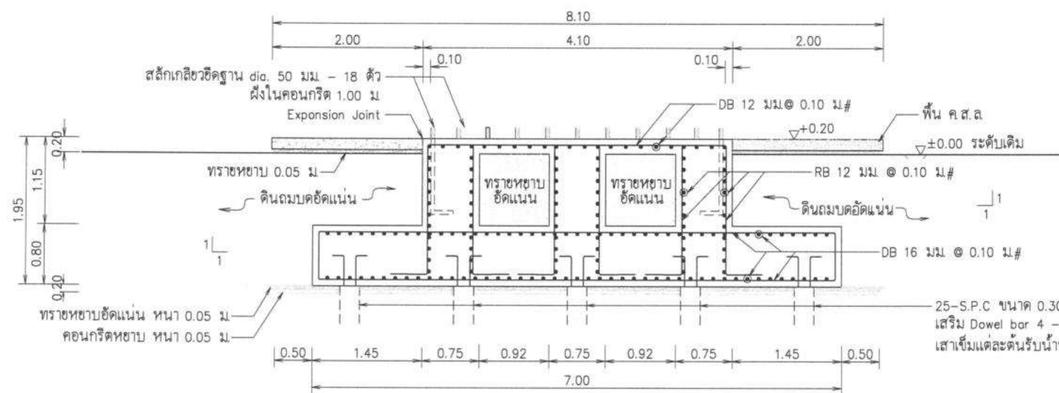
รูปตัด ก-ก
