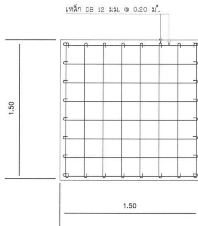
ฐานรากถังกรอง
