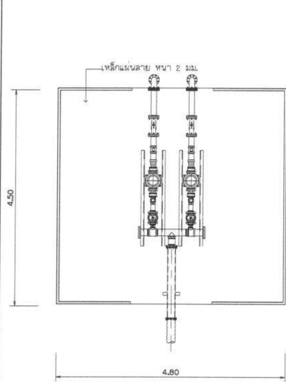
แปลนพื้นอาคาร มาตราส่วน 1 : 100
