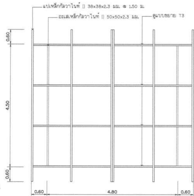
แปลนโครงหลังคา มาตราส่วน 1 : 100
