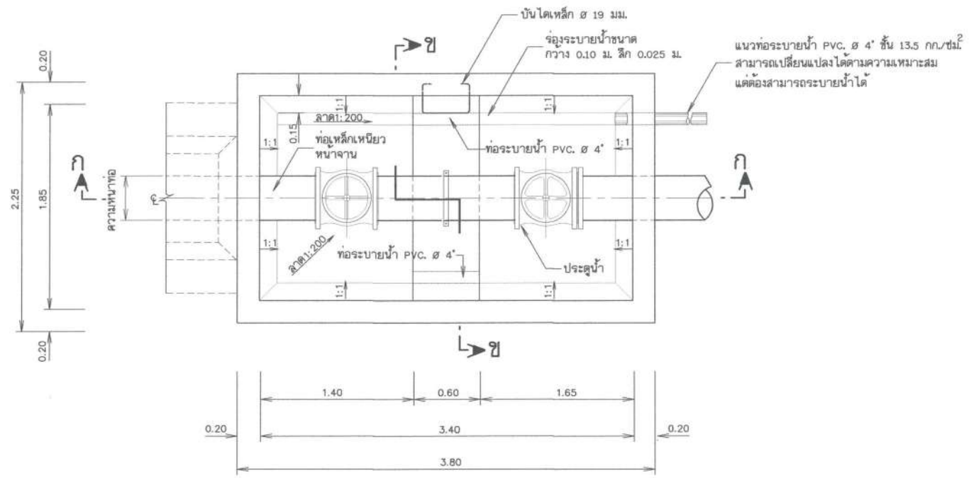
แปลนอาคารบังคับน้ำด้านท้ายน้ำ มาตราส่วน 1:25
