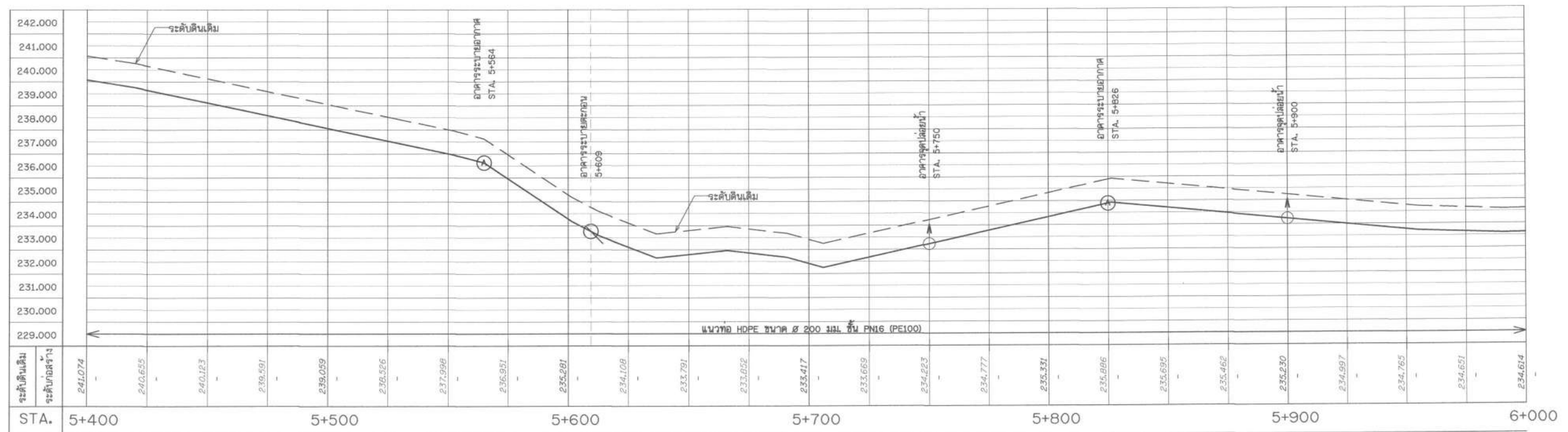
รูปตัดตามแนวยาว กม. 0+000 STA. 5+400 - 6+000
