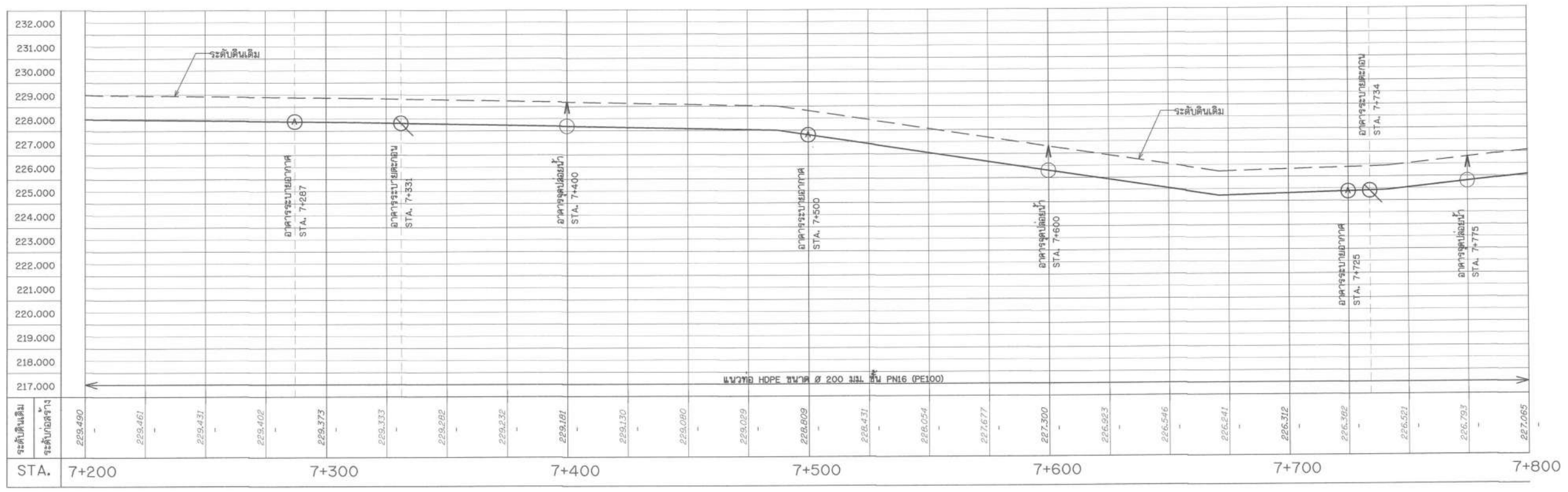
รูปตัดตามแนวยาว กม. 0+000 STA. 7+200 - 7+800 มาตรฐาน 1:1,000 แนวตั้ง 1:100
