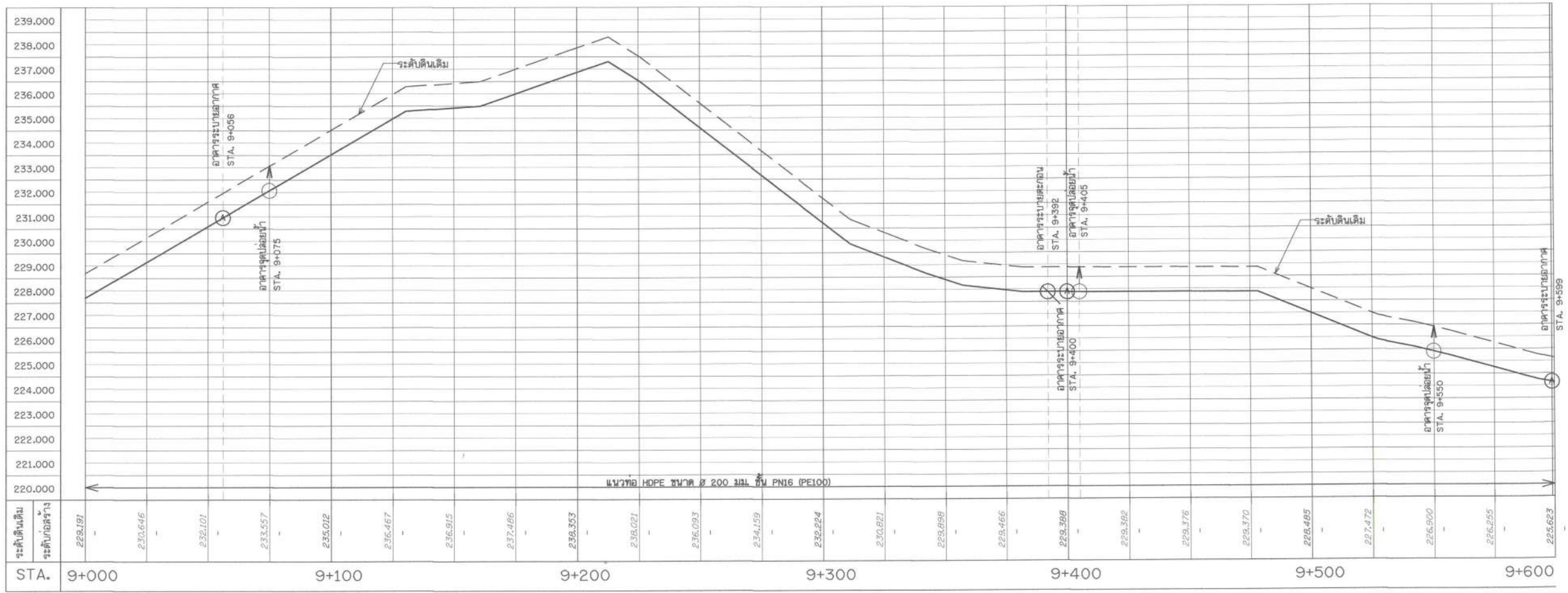
รูปตัดตามแนวยาว กม. 0+000 STA. 9+000 - 9+600 มาตรฐาน 1:1,000
