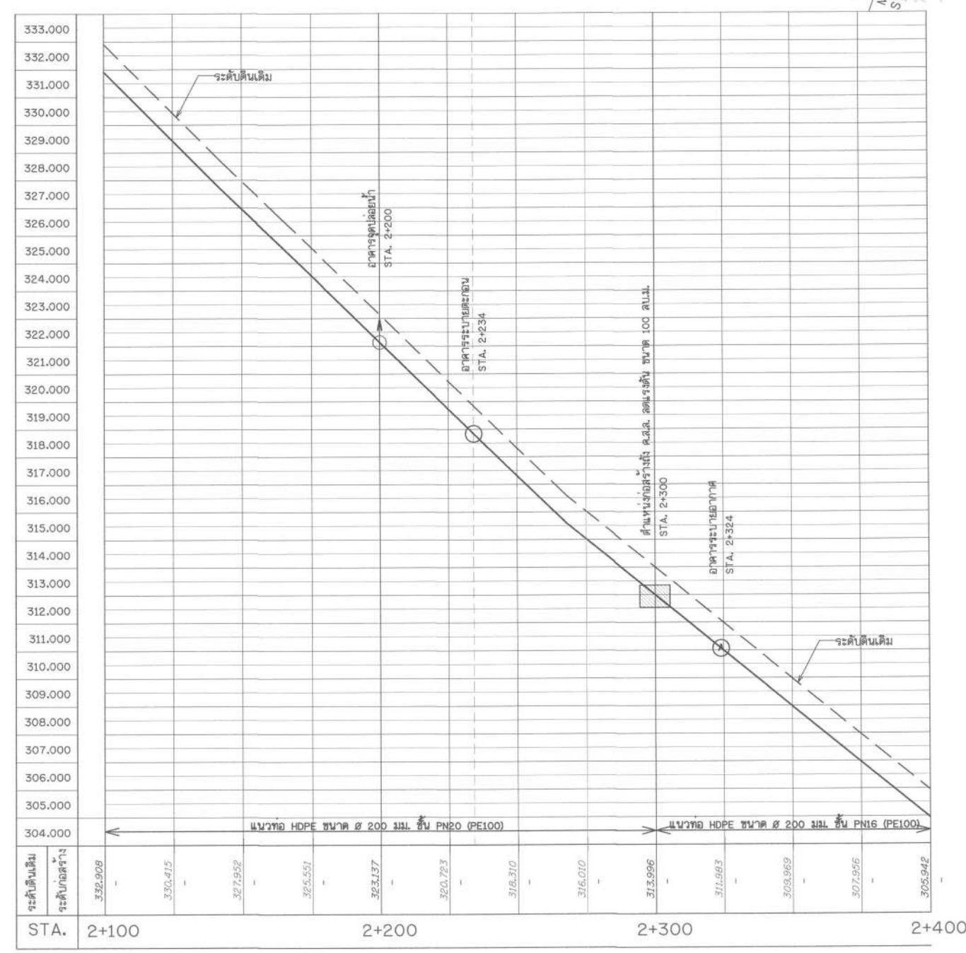
รูปตัดตามแนวยาว กม. 0+000 STA. 1+800 - 2+400 มาตราส่วน แนวบน 1:1,000 แนวตั้ง 1:100
