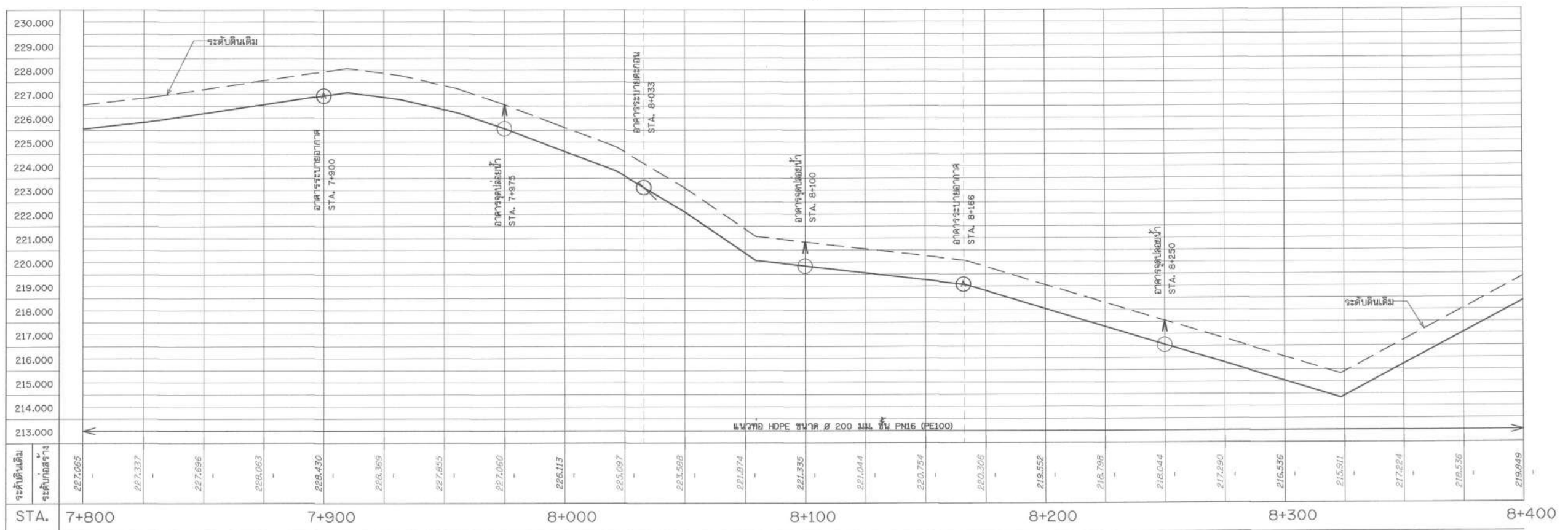
รูปตัดตามแนวยาว กม. 0+000 STA. 7+800 - 8+400
