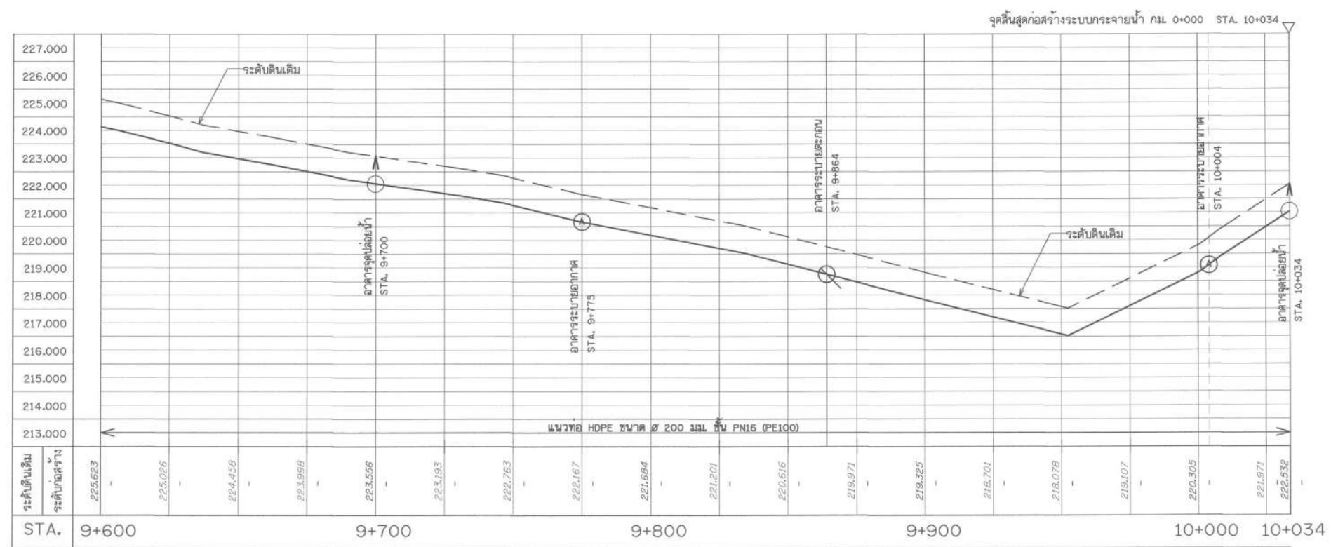
รูปตัดตามแนวยาว กม. 0+000 STA. 9+600 - 10+034 มาตราส่วน 1:1,000 แนวตั้ง 1:100
