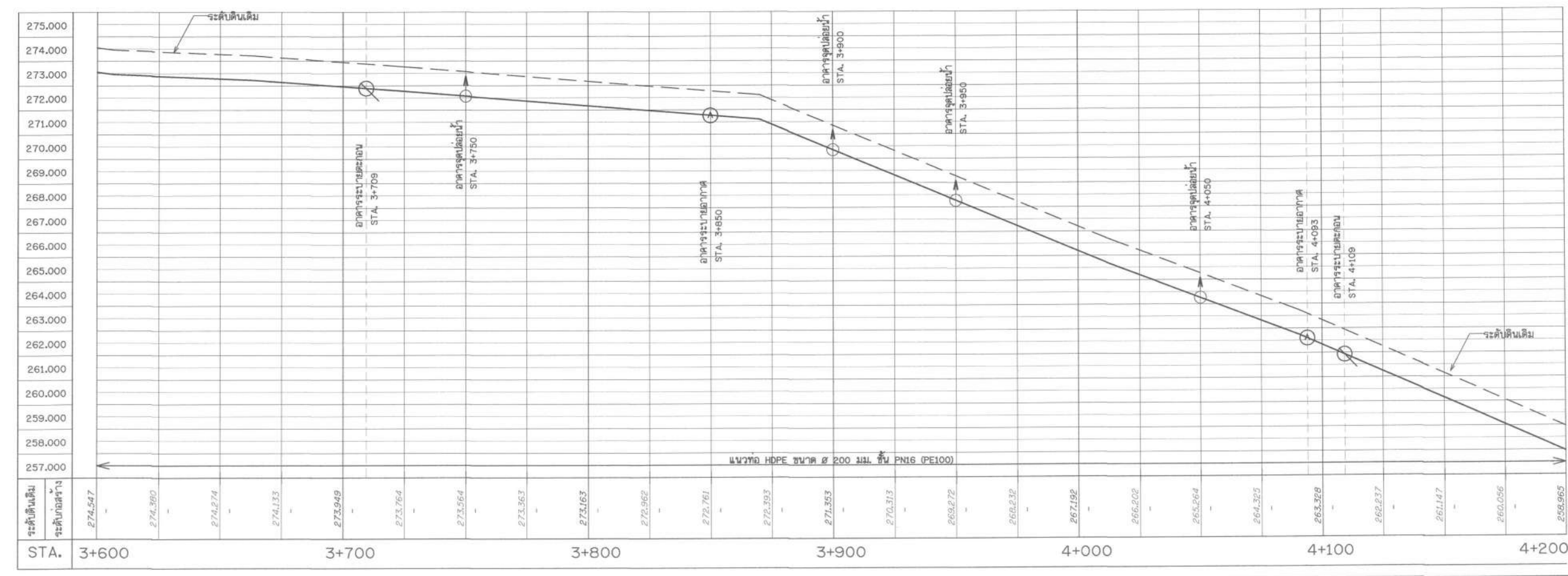
รูปตัดตามแนวยาว กม. 0+000 STA. 3+600 - 4+200 , กม. 20+000 STA. 20+000 - 20+148 มาตราส่วน แนวนอน 1:1,000 แนวตั้ง 1:100
