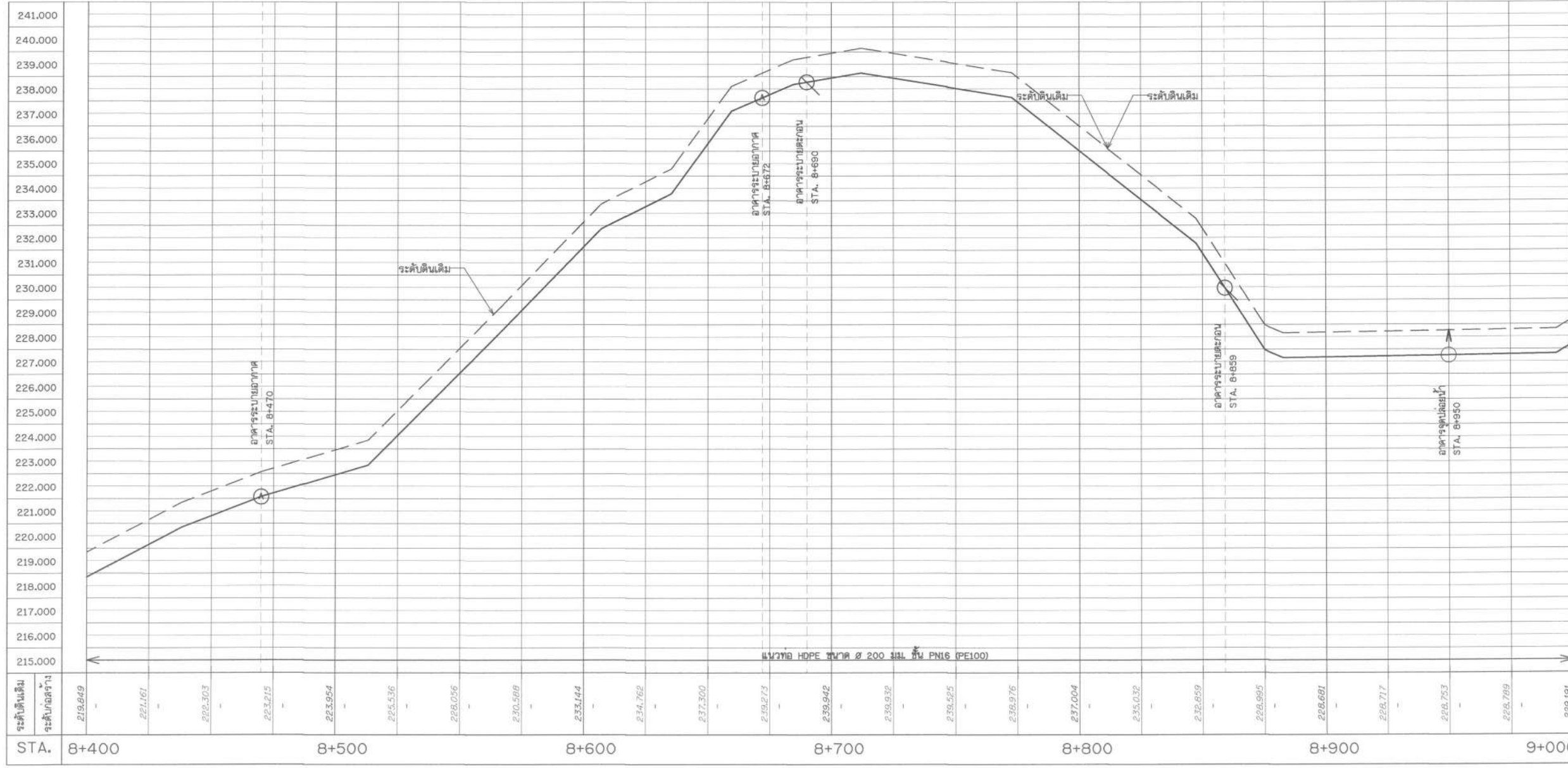
รูปตัดตามแนวยาว กม. 0+000 STA. 8+400 - 9+000
