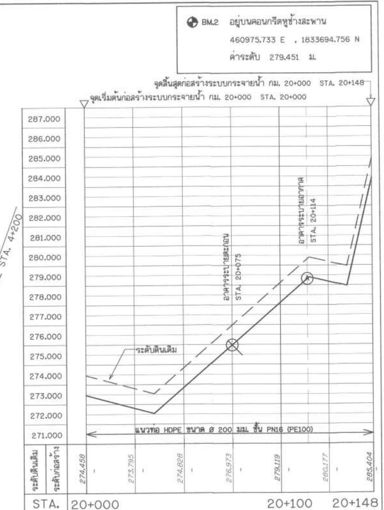
รูปตัดตามแนวยาว กม. 0+000 STA. 3+600 - 4+200 , กม. 20+000 STA. 20+000 - 20+148 มาตราส่วน แนวนอน 1:1,000 แนวตั้ง 1:100
