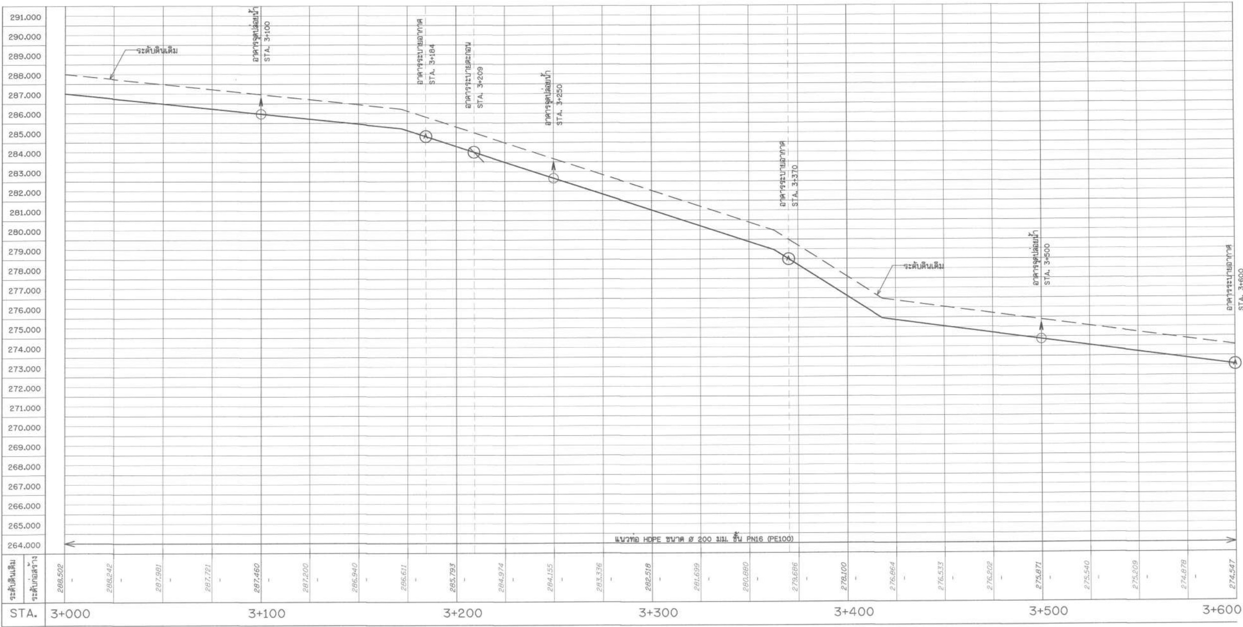
รูปตัดตามแนวยาว กม. 0+000 STA. 3+000 - 3+600
