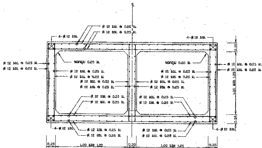
รูปตัดขวางแสดงการเสริมเหล็กท่อนเหลี่ยม (ท่อนขนาด 1.00 x 1.00 ม. และท่อนขนาด 1.25x1.25 ม.)
