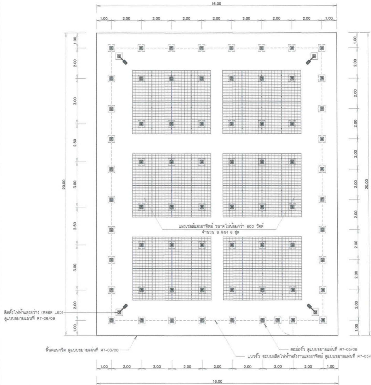
แผ่นการติดตั้งแผงเซลล์แสงอาทิตย์ พร้อมรั้ว
