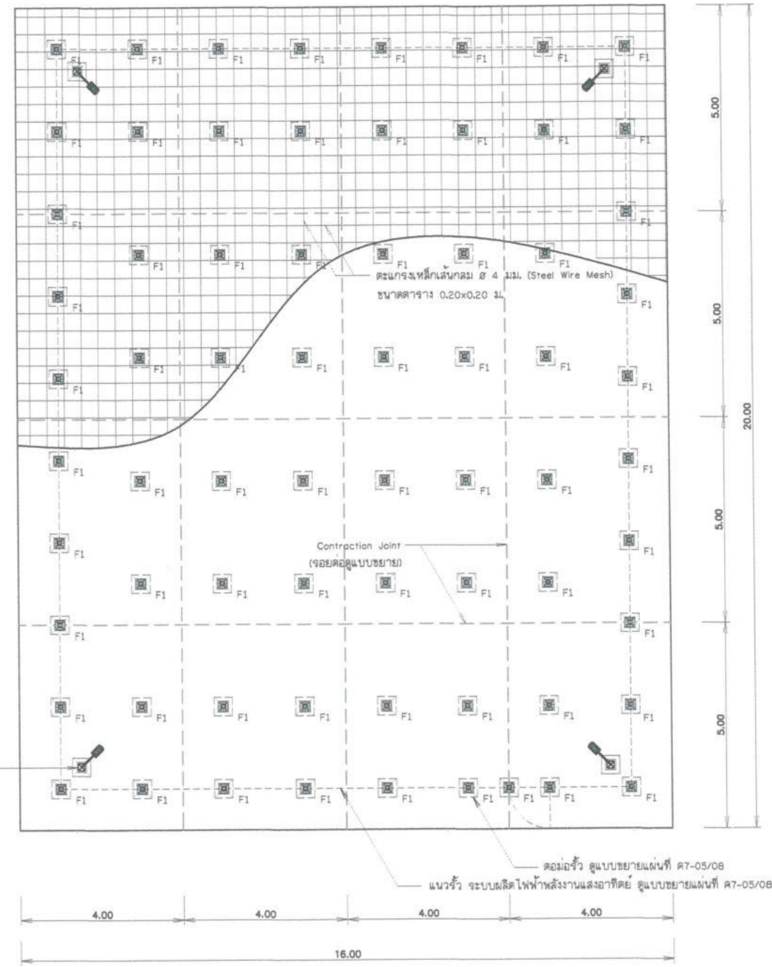
รูปขยายพื้นคอนกรีต
