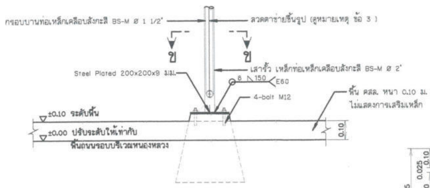
รูปขยายฐานรากโครงสร้างรับแผง F1 (ต่อมอ คสล. หล่อสำเร็จรูปพร้อมติดตั้ง) ไม่แสดงมาตราส่วน
