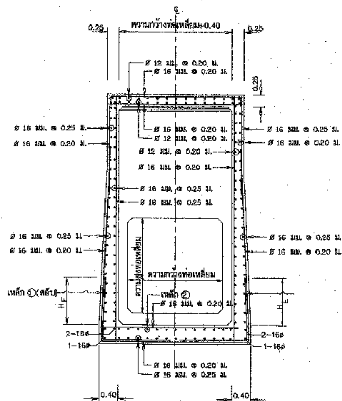
รูปตัด ก-ก โมเมนต์ตามยาวตามส่วน
