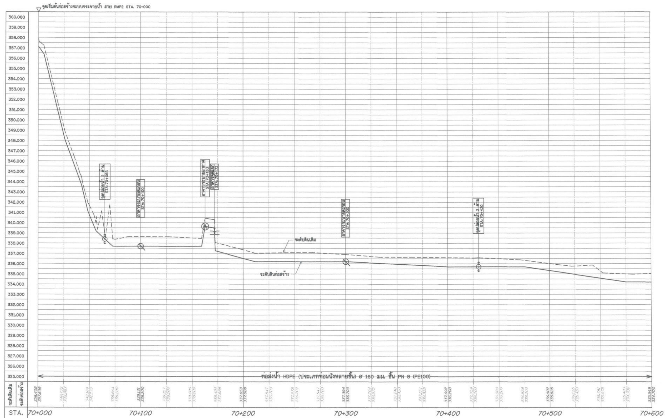
รูปตัดตามแนวสายระบบกระจายน้ำ สาย RMP2 STA. 70+000 - 70+600 มาตรฐาน แนวนอน 1:1,000 แนวตั้ง 1:100
