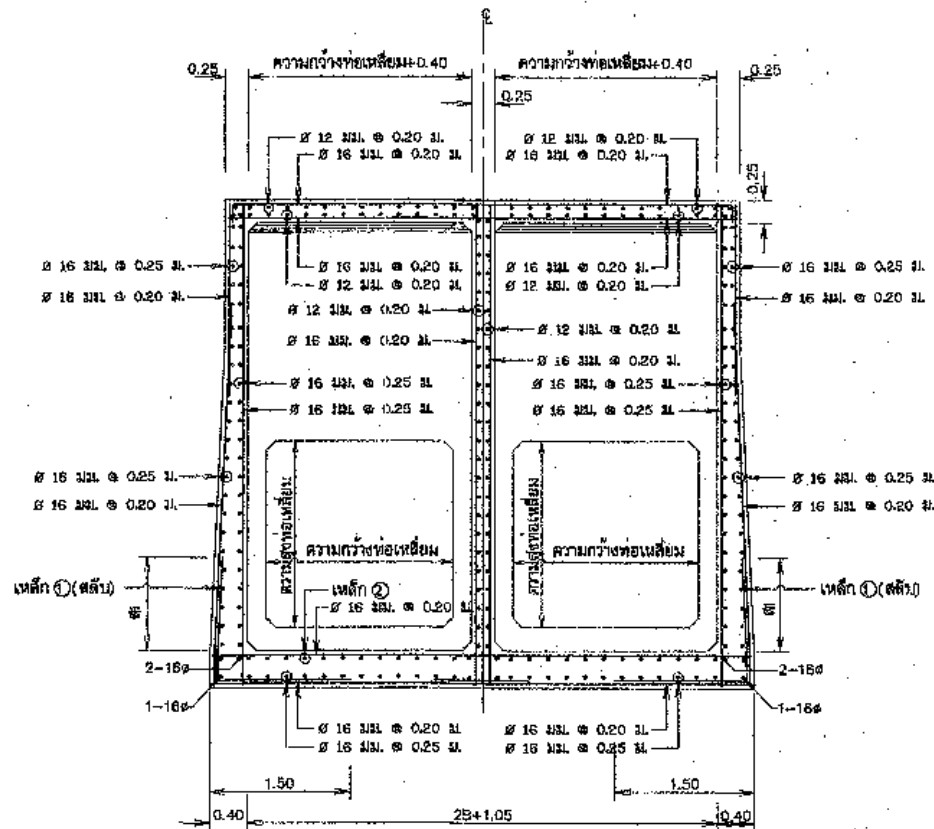
รูปตัด จ-จ
