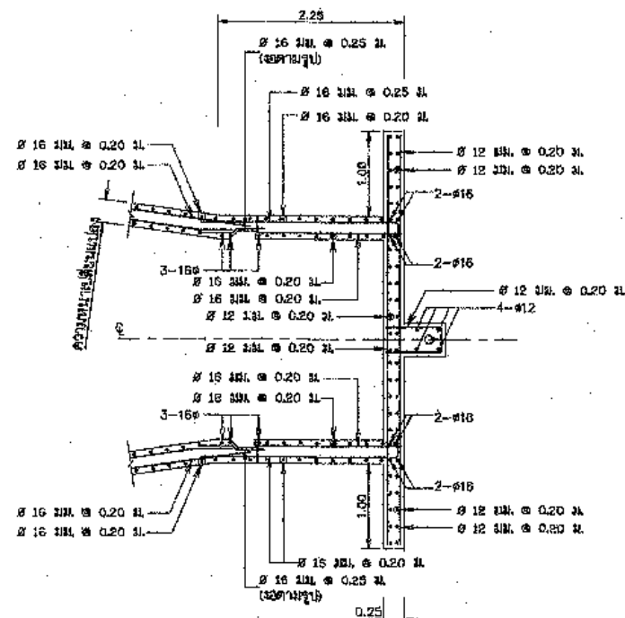
รูปตัด ก2-ก2 โมเมนต์ตามยาวตามส่วน
