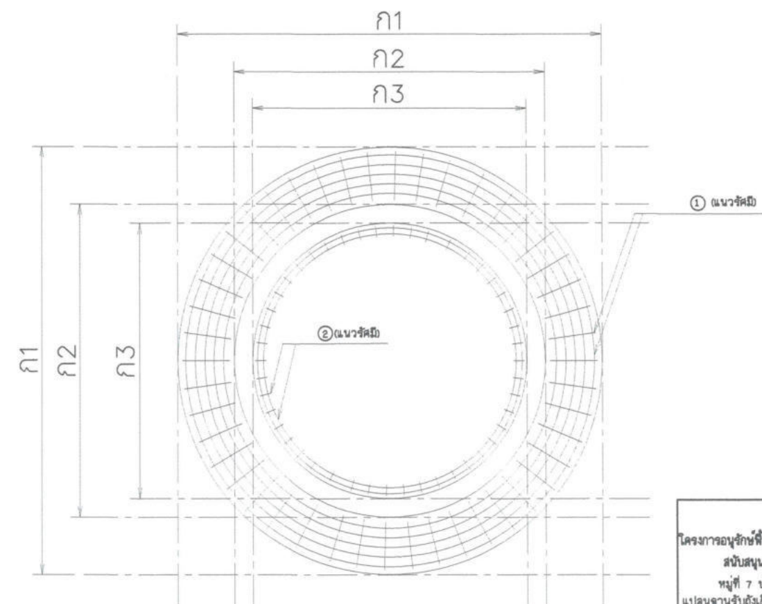
แผ่นเหล็กเสริมขอบ รับดึงเก็บน้ำ Fusion Bonded Epoxy (FBE)
