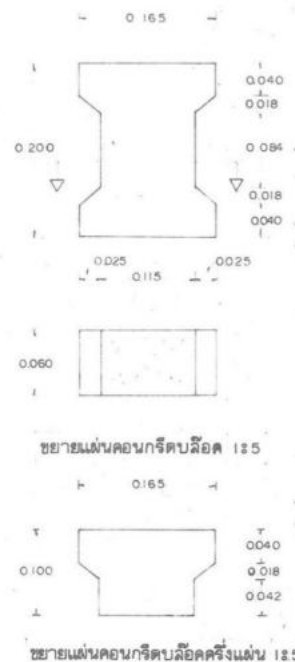
ขยายแผ่นคอนกรีตเสริมเหล็ก 1810
