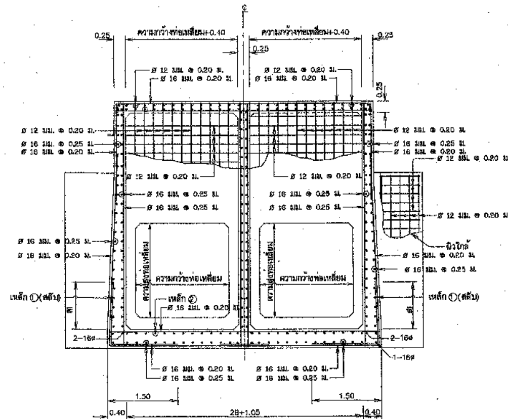
รูปตัด จ2-จ2
