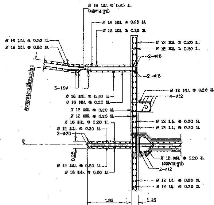
รูปตัด ก2-ก2
