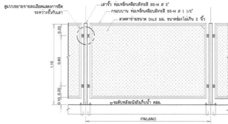
แบบขยายราวกันตก (สำหรับรั้วกับน้ำ คสล. แบบไม่มีฝ้าปิด)
