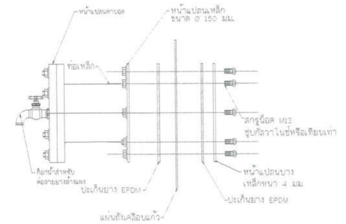
แบบขยายหน้าแปลนคานบอด scale NTC.
