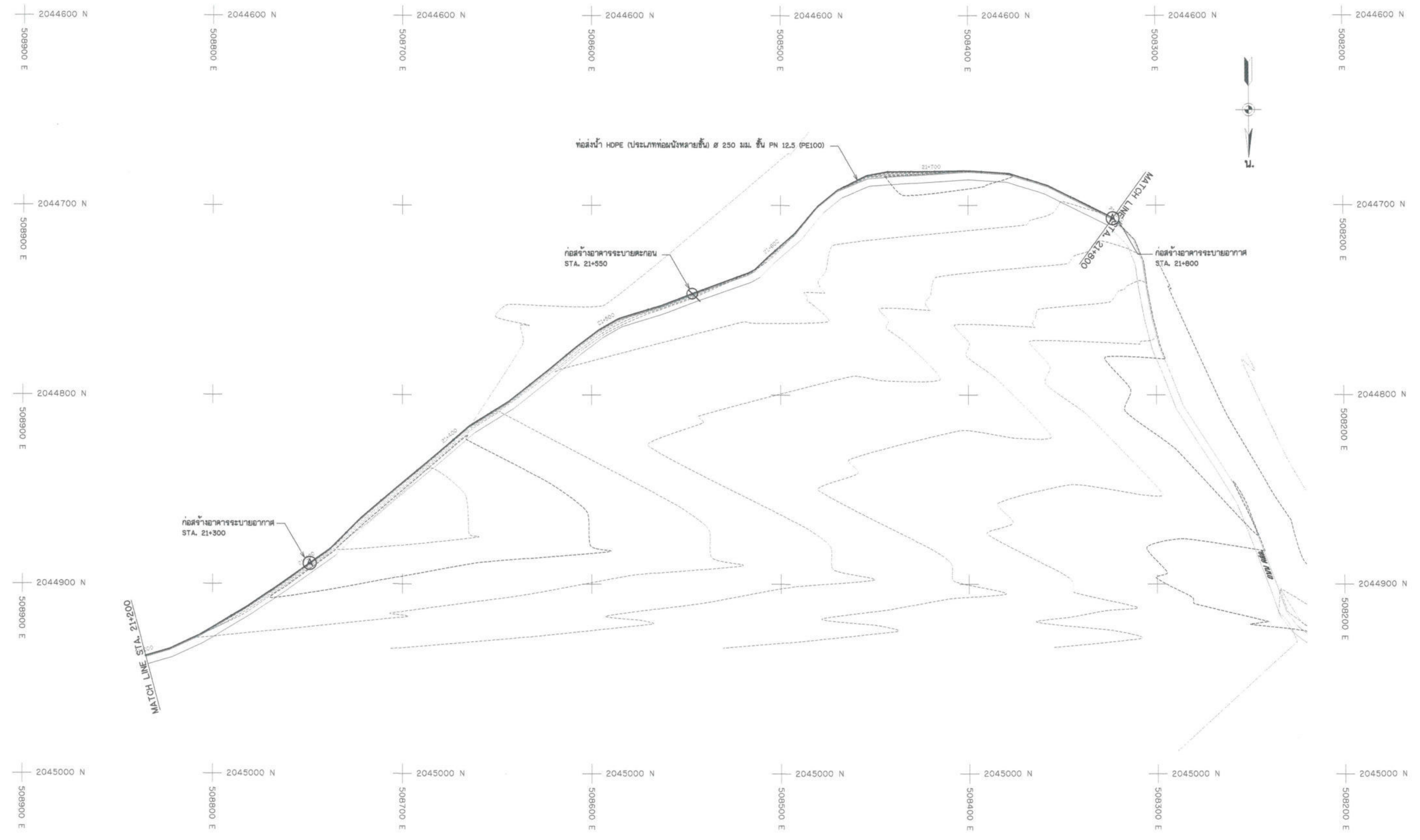
แปลนทั่วไประบบกระจายน้ำ สาย RMP STA. 21+200 - 21+800 มาตราส่วน 1:1,000
