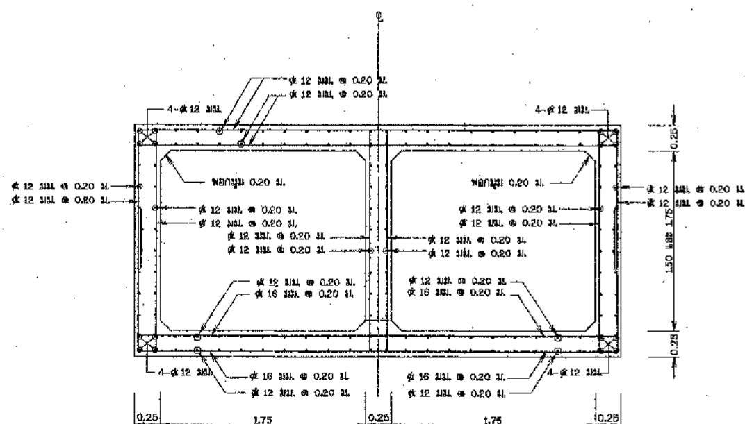
รูปตัดขวางแสดงการเสริมเหล็กท่อเหลี่ยม (ท่อขนาด 1.50 x 1.50 ม. และท่อขนาด 1.75x1.75 ม.)
