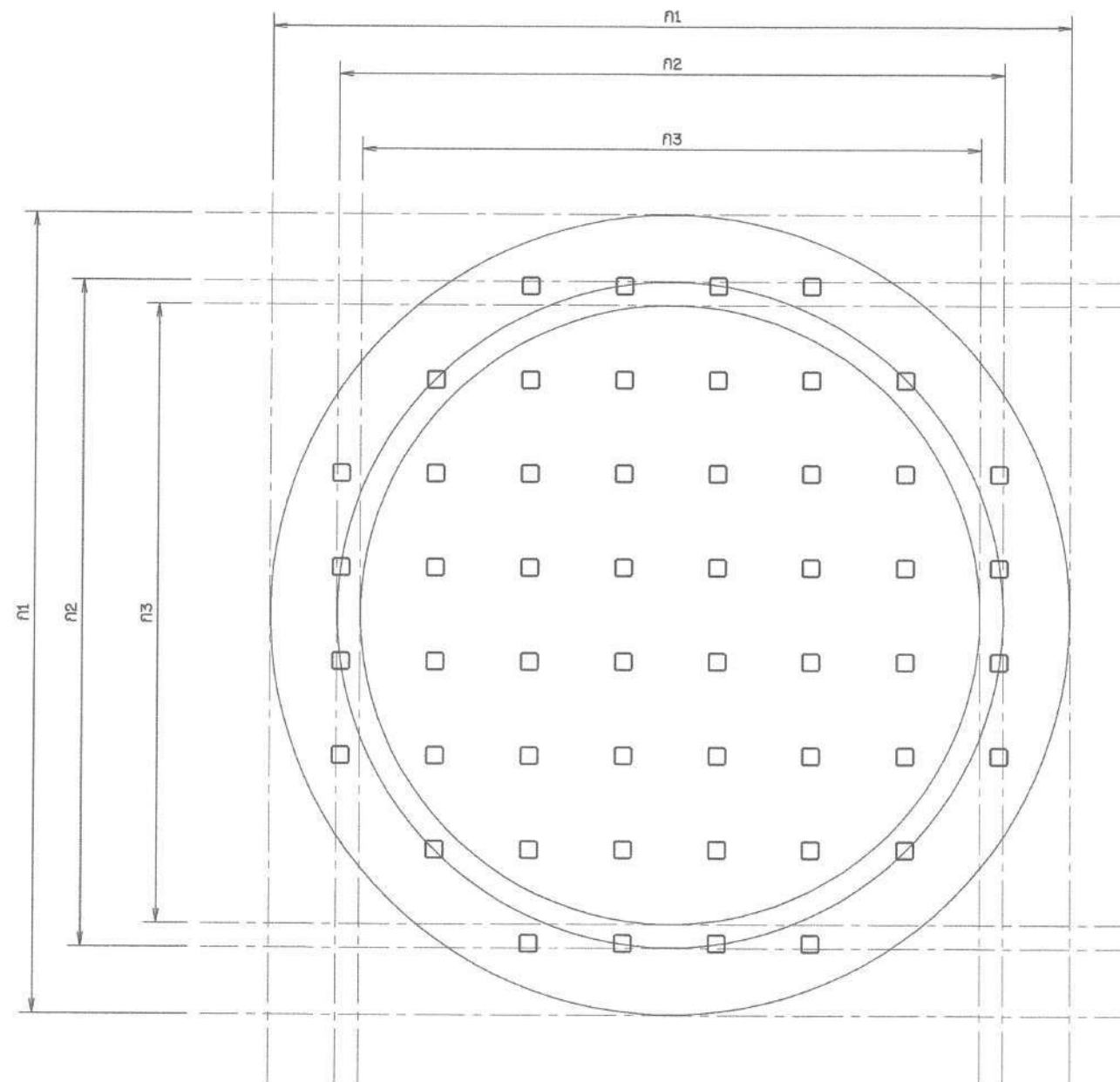
แพลนเสาสีม ถึงเก็บน้ำ Fusion Bonded Epoxy (FBE) ขนาด 1,100 ลบ.ม. มาตราส่วน 1:100
