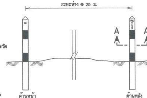
แสดงการวางหลักบ่อแกวท่อ มาตราส่วน 1:20
