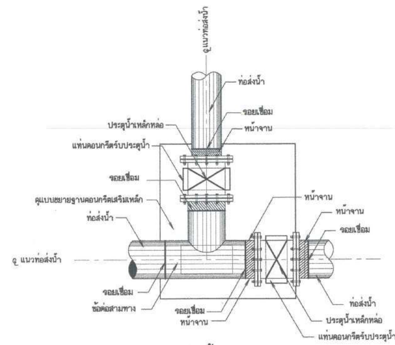
รูปขยายการติดตั้งอาคารจุดแยก
