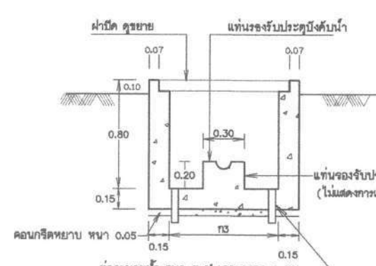
รูปตัด 1 - 1 มาตราส่วน 1:20
