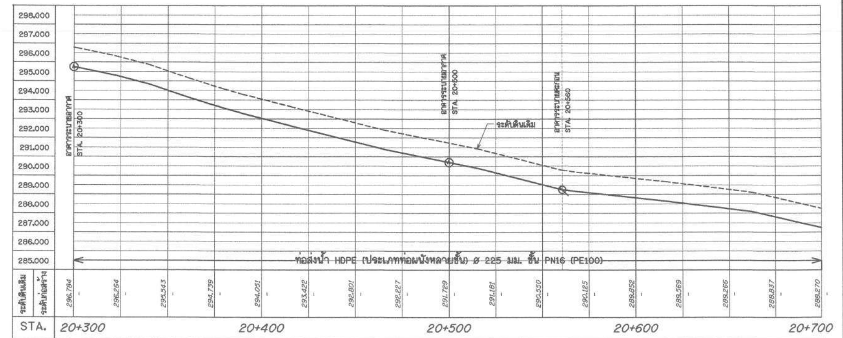
รูปตัดตามแนวยาวระบบกระจายน้ำ สาย RMP STA. 20+000 - 20+600 มาตราส่วน 1:1,000
