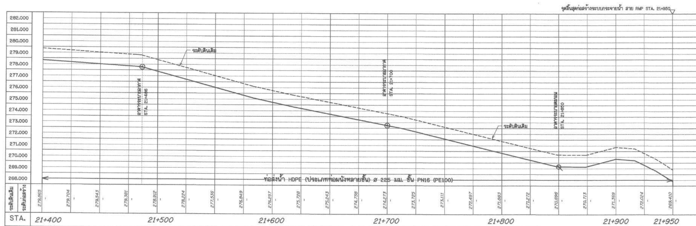
รูปตัดตามแนวสายระบบกระจายน้ำ สาย RMP STA. 21+400 - 21+950 มาตราส่วน 1:1,000
