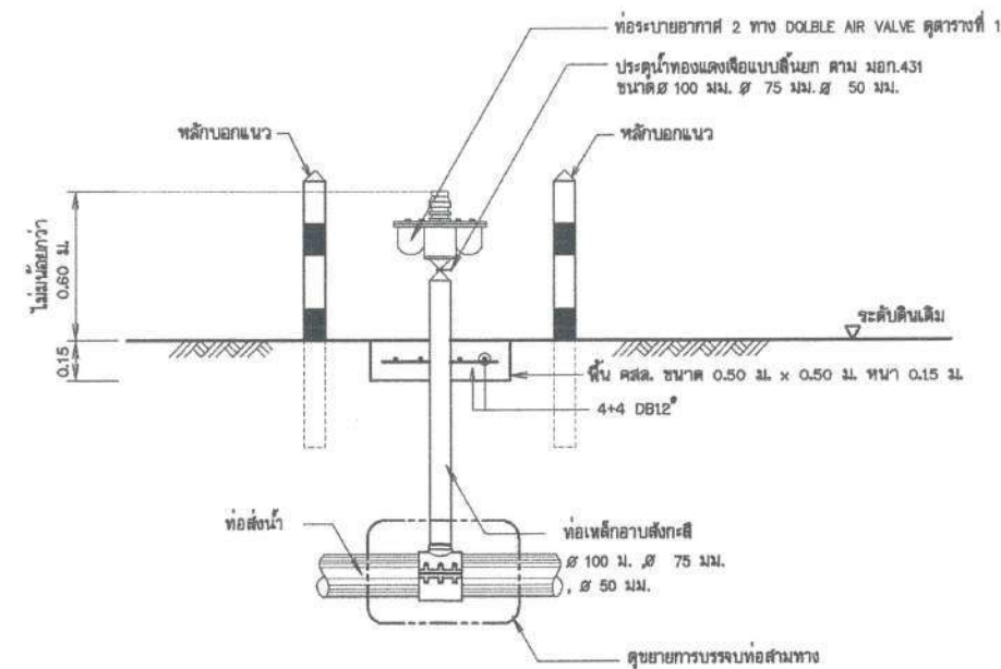
รูปตัด ข - ข แสดงการติดตั้งท่อระบายอากาศ
