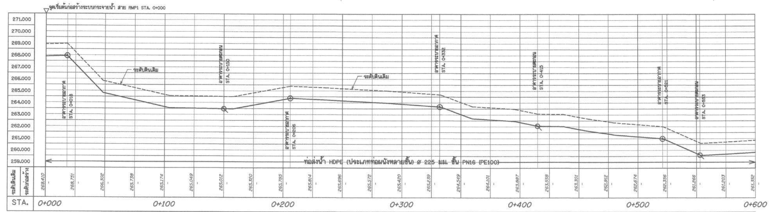
รูปตัดตามแนวยาวระบบกระจายน้ำ สาย RMP1 STA. 0+000 - 0+600 มาตราส่วน 1:1,000
