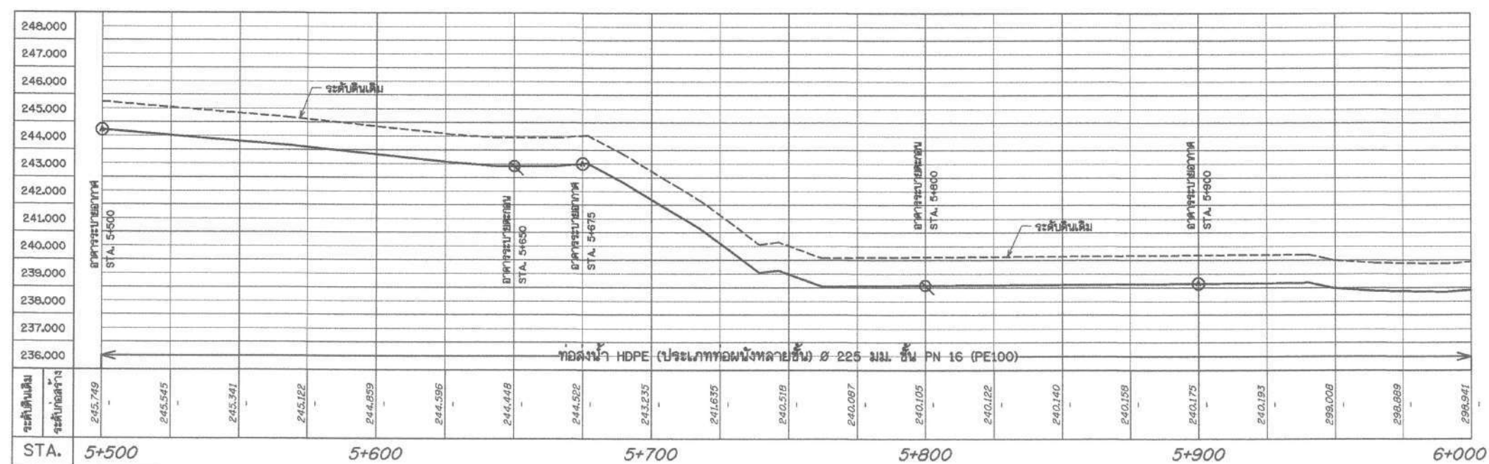
รูปตัดตามแนวสายระบบกระจายน้ำ สาย RMP1 STA. 5+500 - 6+000 มาตราส่วน 1:1,000
