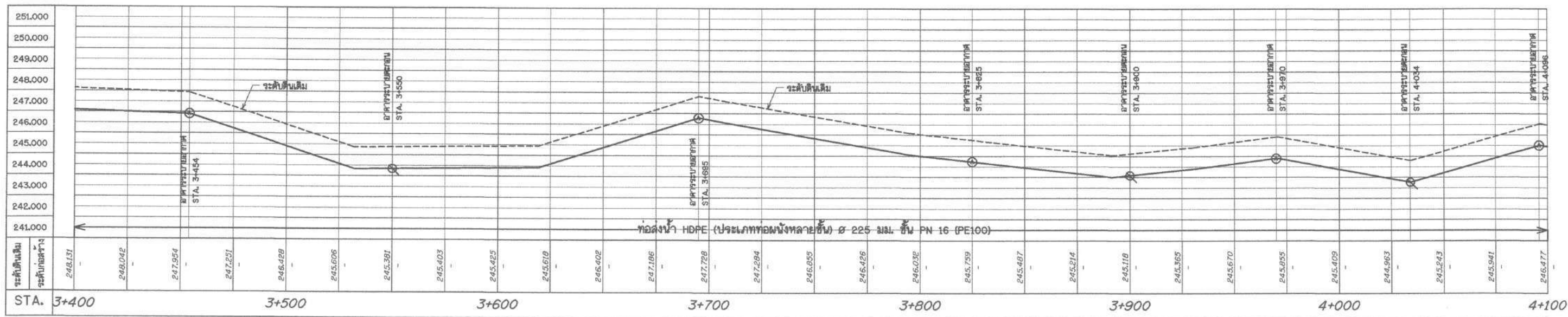
รูปตัดตามแนวาวระบบกระจายน้ำ สาย RMP1 STA. 3+400 - 4+100 มาตรฐาน 1:1,000
