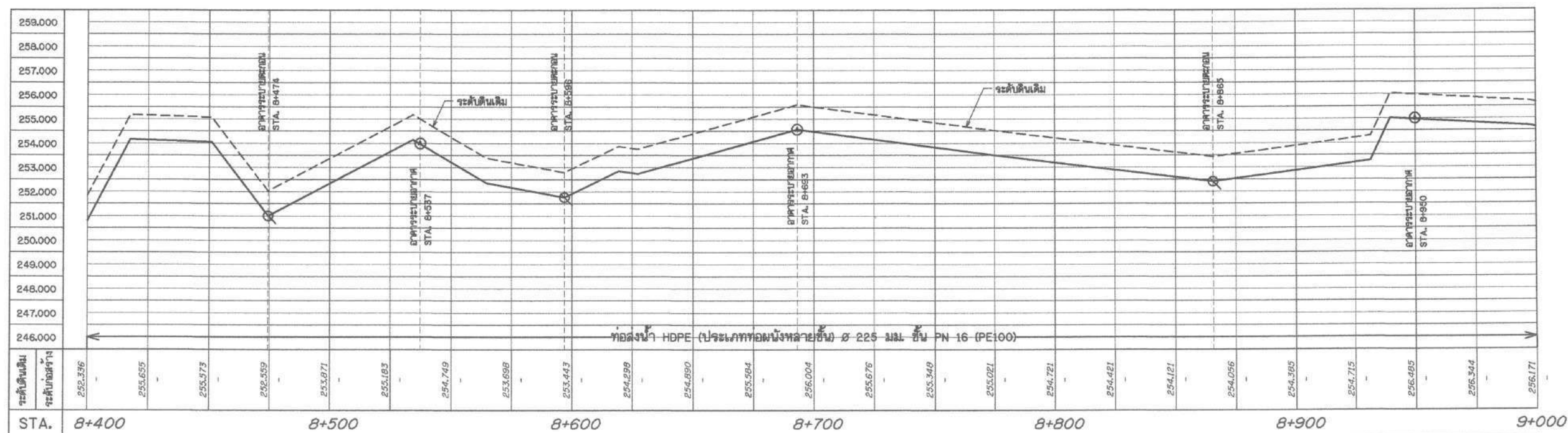
รูปตัดตามแนวยาวระบบกระจายน้ำ สาย RMP1 STA. 8+400 - 9+000
