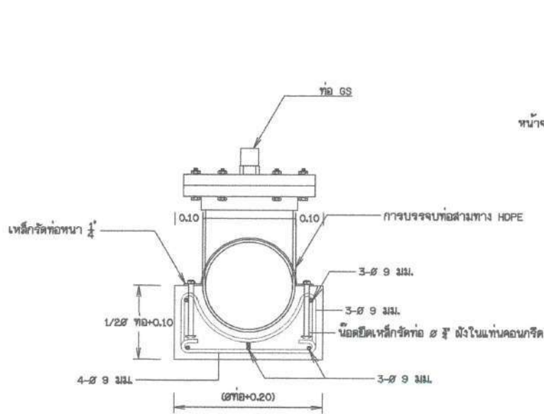
รูปตัดอาคารท่อระบายอากาศ Ø 25 มม. (ใช้สำหรับท่อส่งน้ำที่มีขนาดไม่เกิน 6 นิ้ว) มาตราส่วน 1:20
