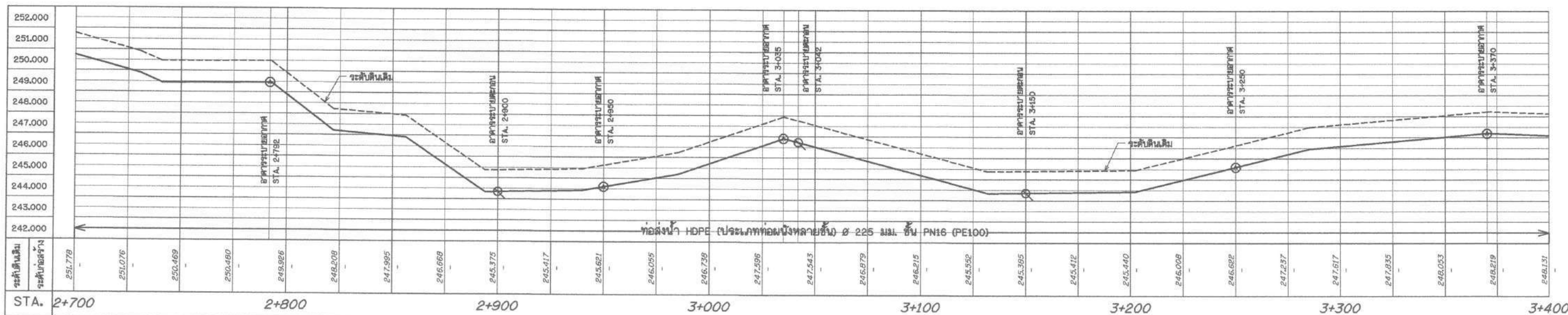
รูปตัดตามแนวยาวระบบกระจายน้ำ สาย RMP STA. 2+700 - 3+400
