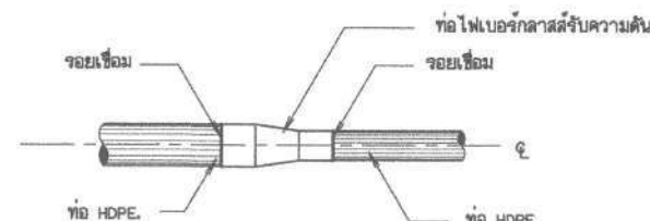
รูปตัดทั่วไปแสดงการวางท่อ มาตราส่วน 1:50
