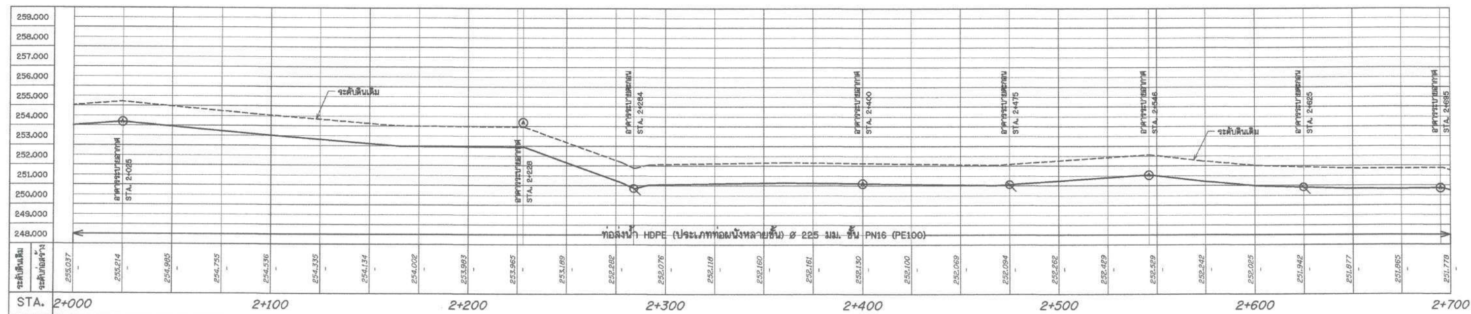
รูปตัดตามแนวยาวระบบกระจายน้ำ สาย RMP1 STA. 2+000 - 2+700
