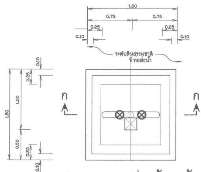
แปลนอาคารจุดปล่อยน้ำ 2 ด้าน
