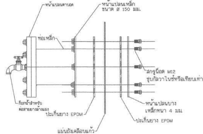
แบบขยายหน้าแปลนคานาอด scale NTC.
