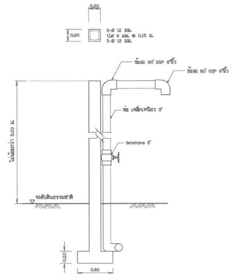
ท่อจุดปล่อยน้ำ ความสูงไม่น้อยกว่า 3.00 ม.
