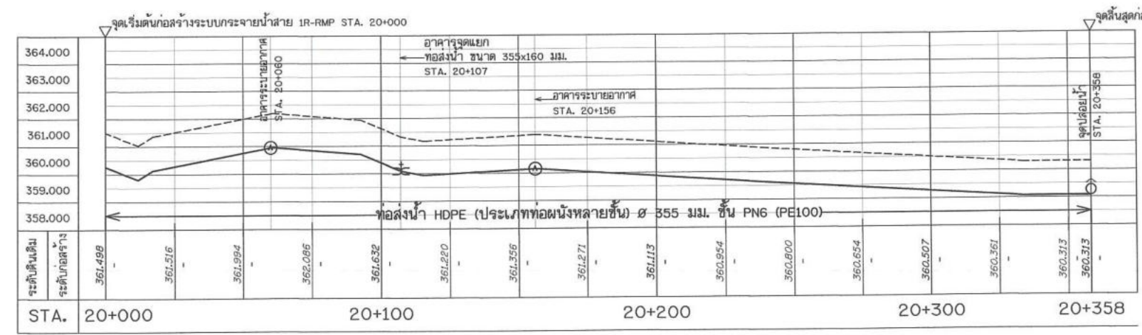
รูปตัดตามแนวยาวระบบกระจายน้ำ สาย 1R-1L-1R-LMP STA. 20+000 - 20+358 มาตรฐาน 1:1,000 แนวตั้ง 1:100
