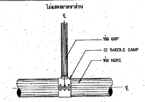
การบรรจุท่อสามทาง HDPE กับท่อ GSP แบบ CI SADDLE CLAMP (สำหรับอาคารจุดปล่อยน้ำ อาคารประจวบประจวบตอน อาคารท่อระบายอากาศ กรณีท่อส่งน้ำขนาดเส้นผ่าศูนย์กลางน้อยกว่าหรือเท่ากับ 315 มม.) ไม่แสดงมาตราส่วน
