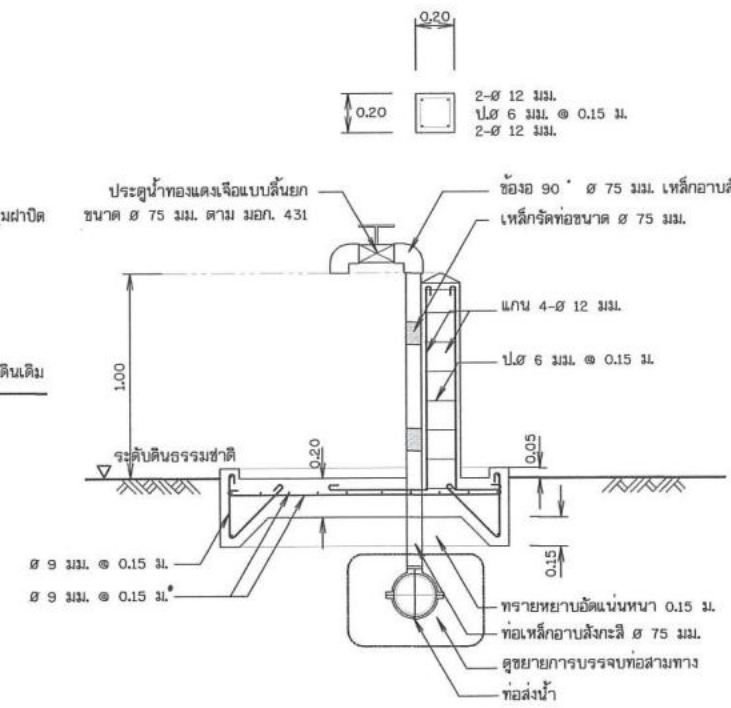
รูปตัด ค - ค
