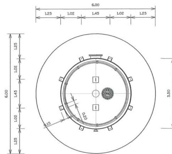
ตำแหน่ง ขายึดถัง SCALE 1 : 100
