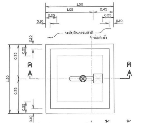
แปลนอาคารจุดปล่อยน้ำ 1 ด้าน
