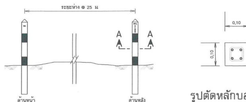
แสดงการวางหลักบอกแนวท่อ
