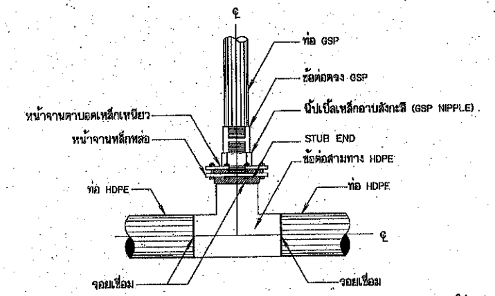
การบรรจุท่อสามทาง HDPE กับท่อ GSP แบบข้อต่อ (สำหรับอาคารจุดปล่อยน้ำ อาคารประจวบประจวบตอน อาคารท่อระบายอากาศ กรณีท่อส่งน้ำขนาดเส้นผ่าศูนย์กลางมากกว่า 315 มม.) ไม่แสดงมาตราส่วน
