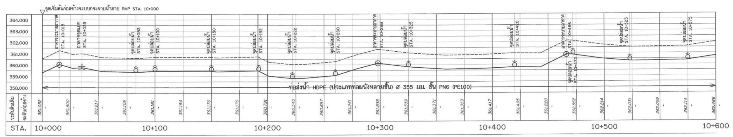
รูปตัดตามแนวยาวระบบกระจายน้ำ สาย 1L-1R-LMP STA. 10+000 - 10+600 มาตราส่วน 1:1,000 แนวตั้ง 1:100
