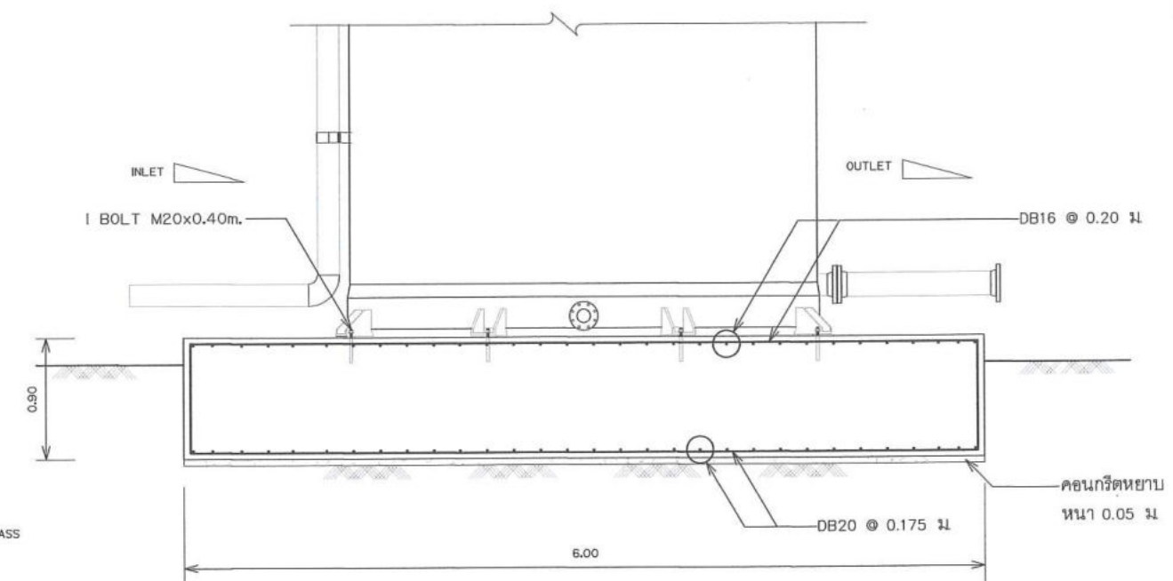
รูปขยายพื้นถัง มาตราส่วน 1:100
