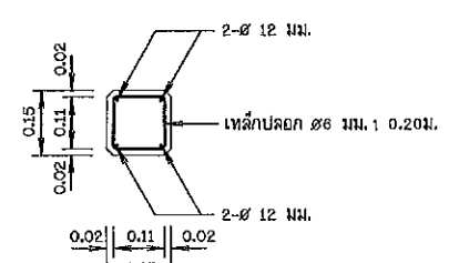
รายละเอียดการติดตั้งเสาป้าย มาตรฐาน 1:20
