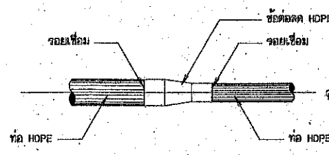
การบรรจุท่อ HDPE กับข้อต่อลดท่อ HDPE ไม่แสดงมาตราส่วน
