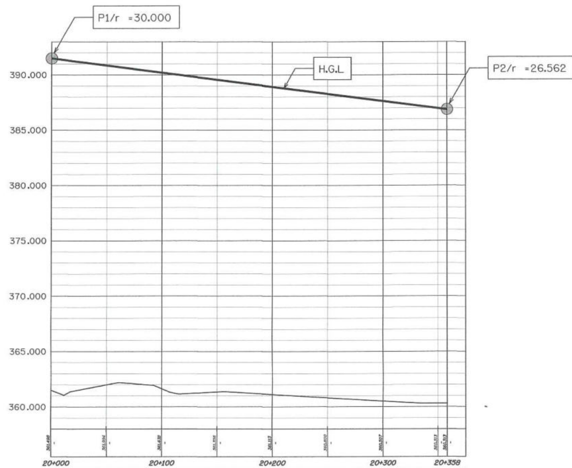
รูปตัดตามแนวยาวแสดง H.G.L. สาย 1L-1R-LMP ไม่แสดงมาตราส่วน
