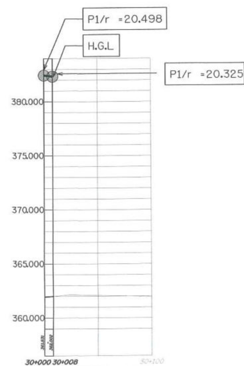
รูปตัดตามแนวยาวแสดง H.G.L. สาย 1L-2R-LMP ไม่แสดงมาตราส่วน
