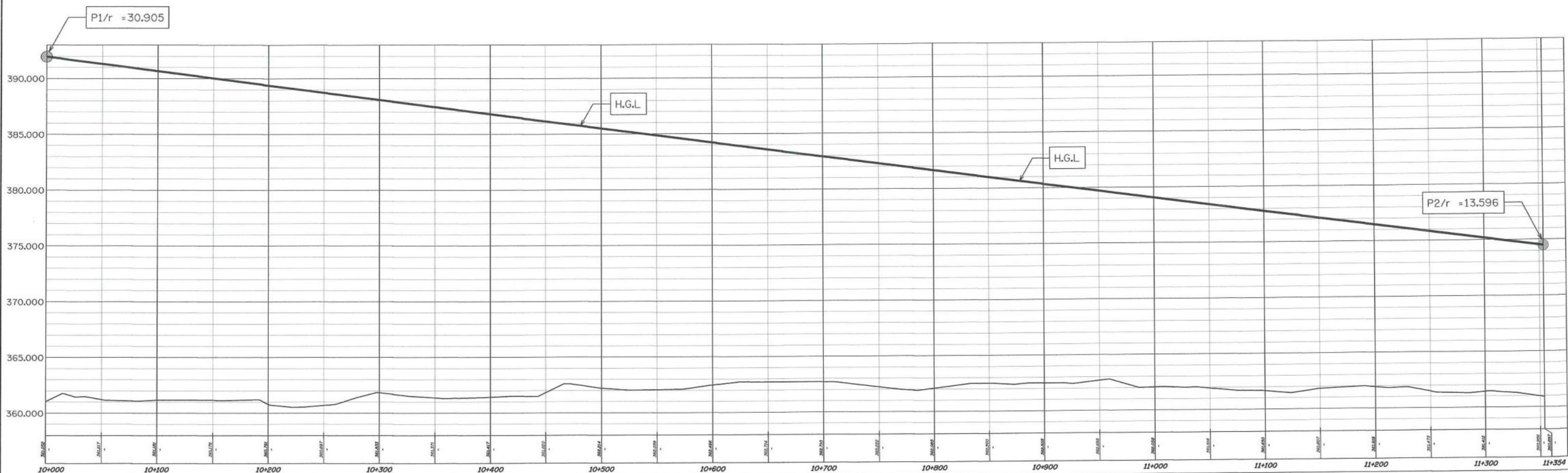
รูปตัดตามแนวยาวแสดง H.G.L. สาย 1L-1R-LMP ไม่แสดงมาตราส่วน
