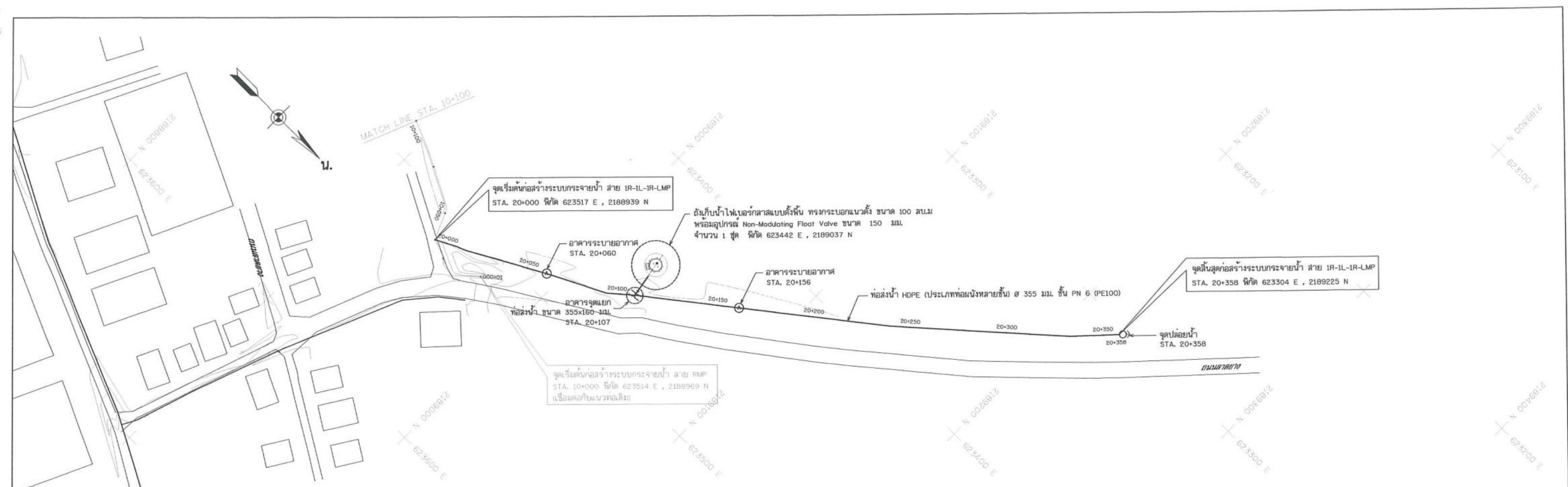
แปลนทั่วไประบบกระจายน้ำ สาย 1R-1L-1R-LMP STA. 20+000 - 20+358 มาตรฐาน 1:1,000
