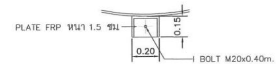
แบบขยาย ขายึดถัง SCALE 1 : 25
