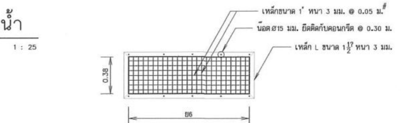
แปลนตะแกรงเหล็กกันล้น
