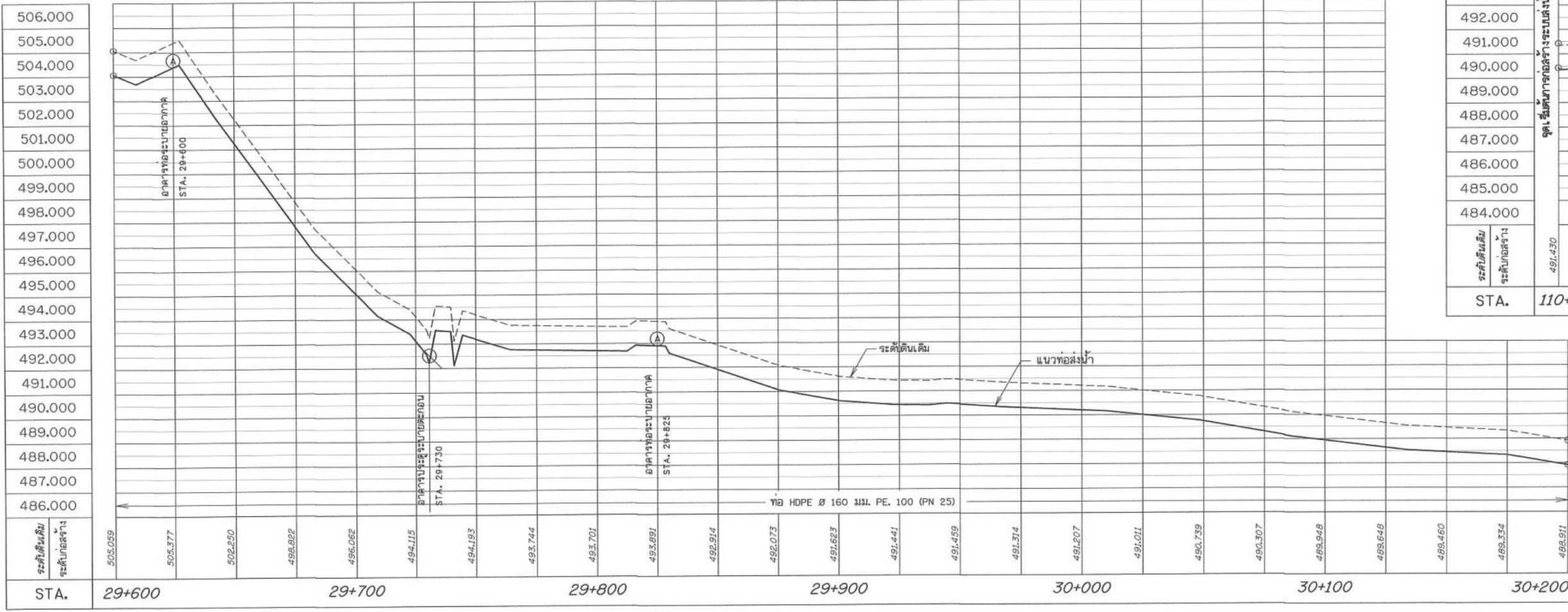
รูปตัดตามแนวยาว STA. 29+600 - 30+200 , STA. 110+000 - 110+115
