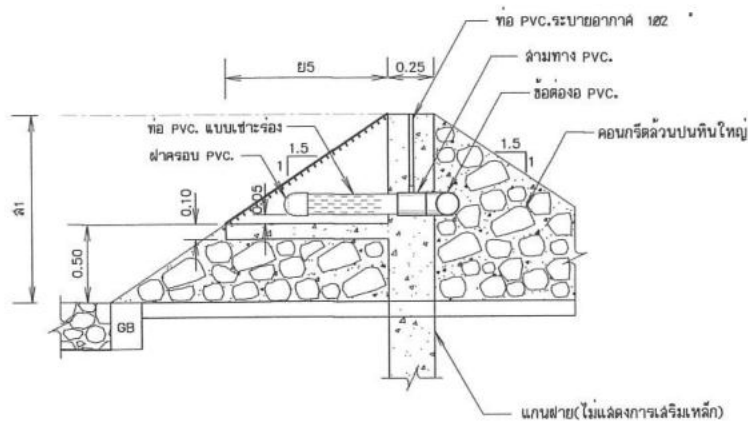
รูปตัด ช - ช
