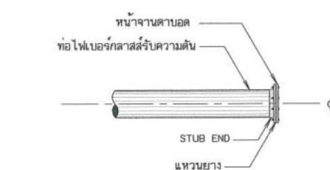
การปิดปลายท่อ
