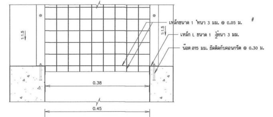
รูปตัด ช - ช
