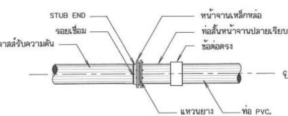
การบรรจุท่อไฟเบอร์กลาสส์ กับท่อ PVC.
