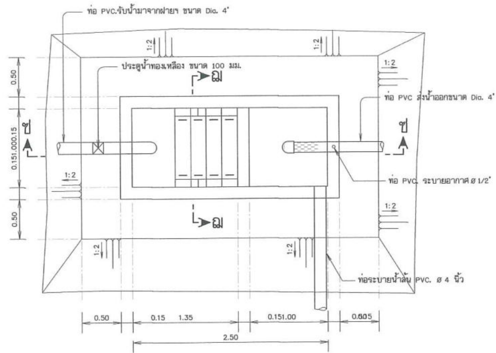
แปลนบ่อตกตะกอน
