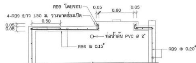
แสดงการเสริมเหล็กฝาถัง
