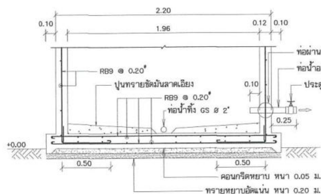
แสดงการเสริมเหล็กพื้นถัง
