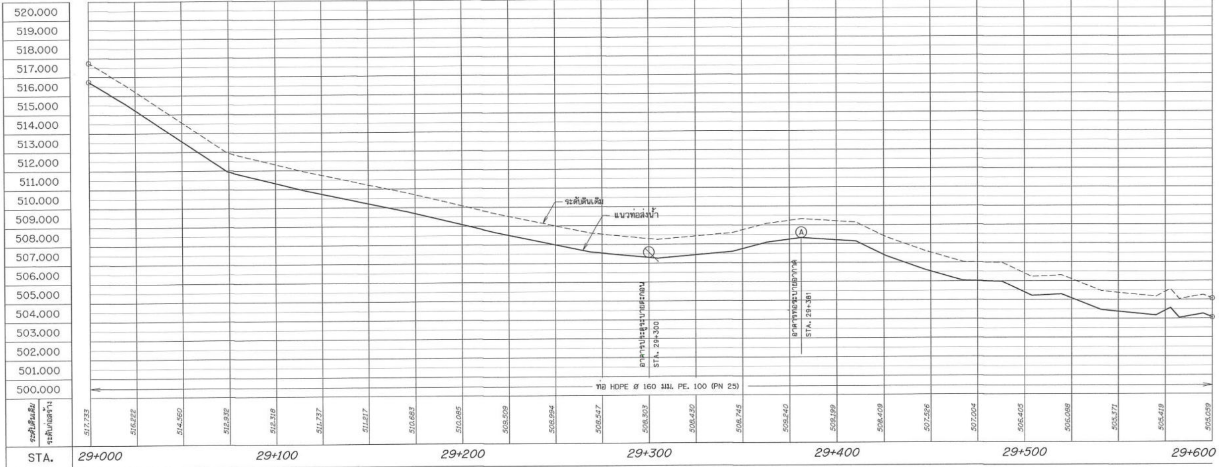
รูปตัดตามแนวยาว STA. 29+000 - 29+600
