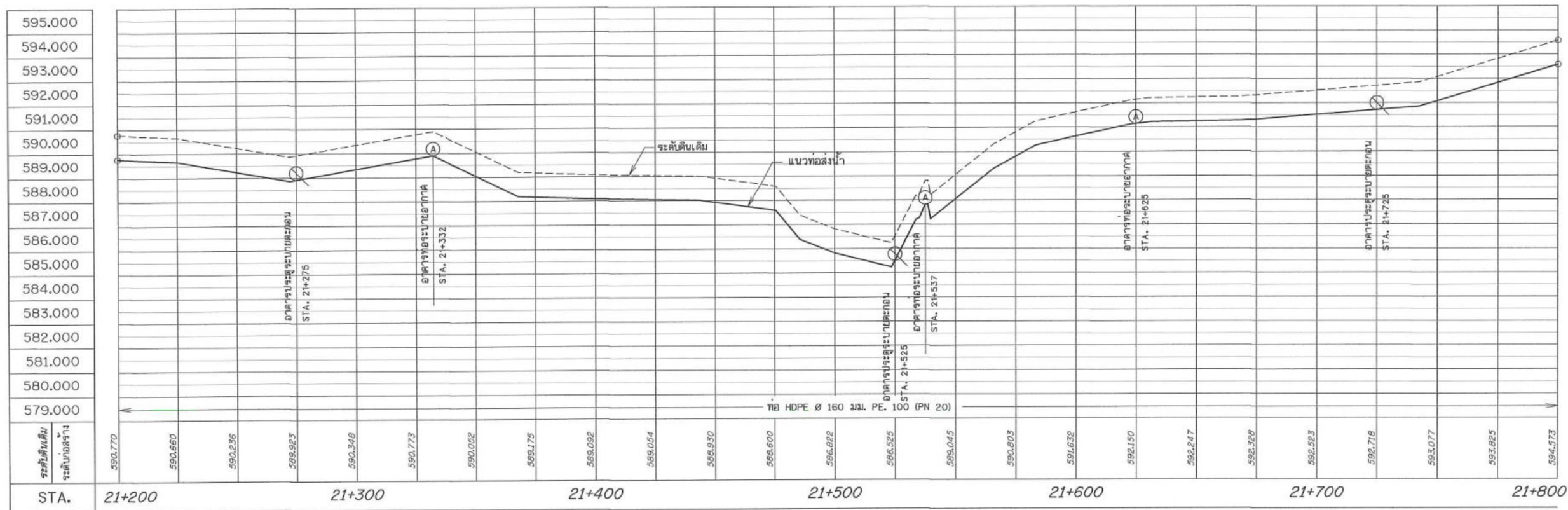
รูปตัดตามแนวยาว STA. 21+200 - 21+800
