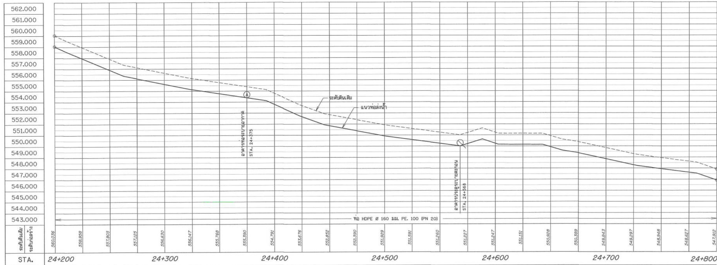
รูปตัดตามแนวยาว STA. 24+200 - 24+800
