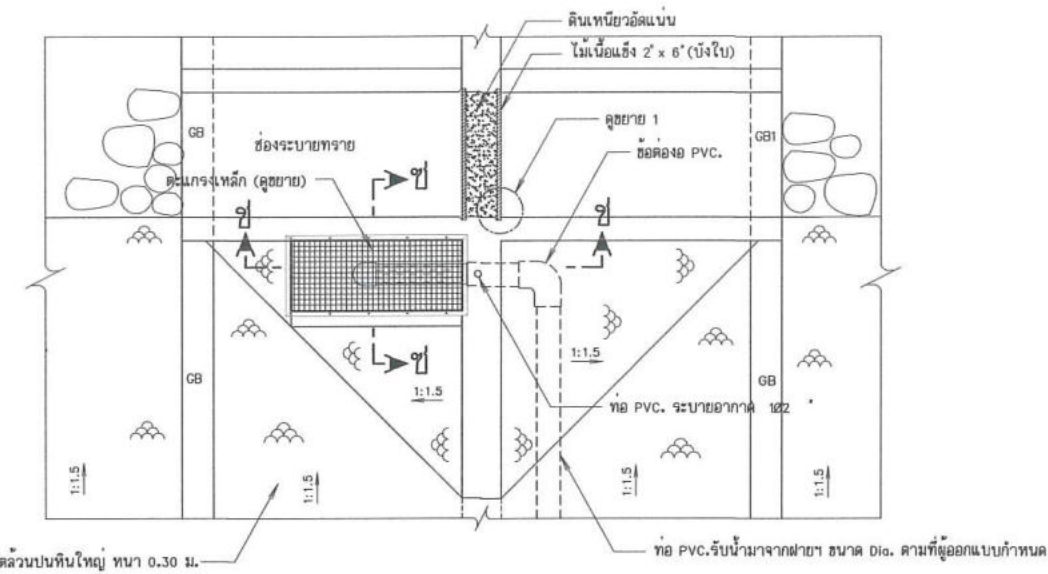
แปลนอาคารรับน้ำ
