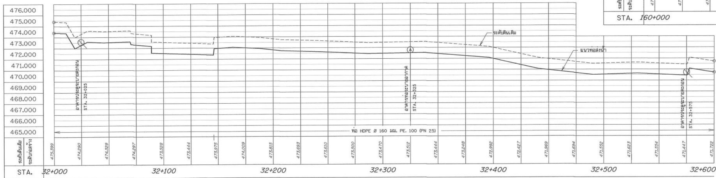
รูปตัดตามแนวยาว STA. 32+000 - 32+600 , STA. 160+000 - 160+151
