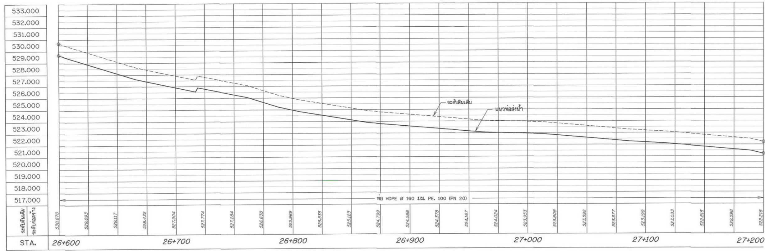
รูปตัดตามแนวยาว STA. 26+600 - 27+200
