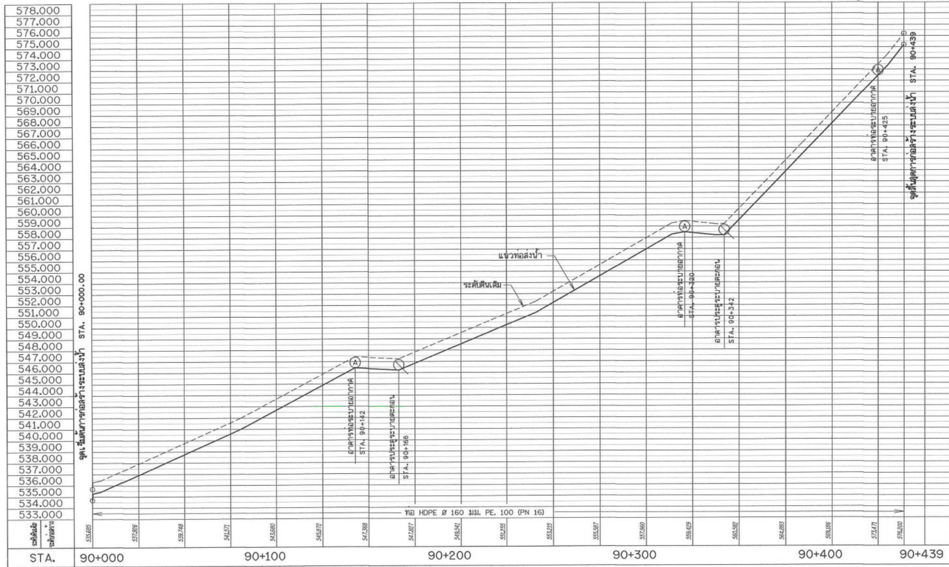
รูปตัดตามแนวยาว STA. 90+000 - 90+439
