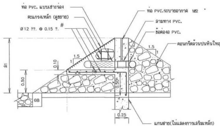
รูปตัด ช - ช (แสดงการเสริมเหล็ก)
