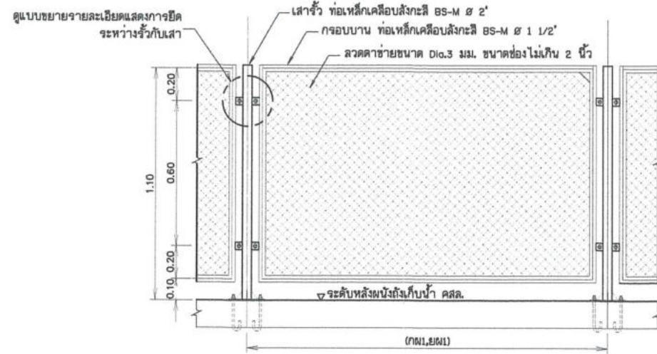
แบบขยายรอกันตก (สำหรับถังเก็บน้ำ คสล. แบบไม่มีฝาปิด)
