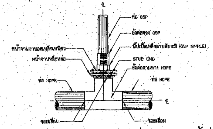
การบรรจุบดท่อสามทาง HDPE กับท่อ GSP แบบข้อต่อ สำหรับอาคารชลประทาน อาคารประจักษ์วิทยาเกษตร อาคารชลประทานอาคาร กรณีท่อส่งน้ำขนาดเส้นผ่าศูนย์กลางน้อยกว่า 315 มม.
