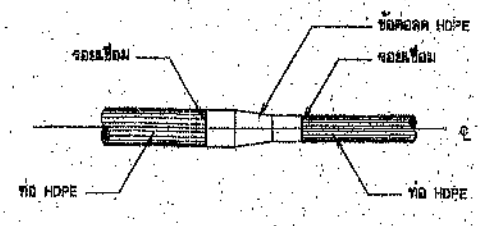
การบรรจุบดท่อ HDPE กับข้อต่อ HDPE ไม่แสดงขนาดบางส่วน
