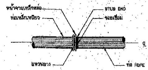
การบรรจุบดท่อเหล็กเหนียวกับท่อ HDPE ไม่แสดงขนาดบางส่วน
