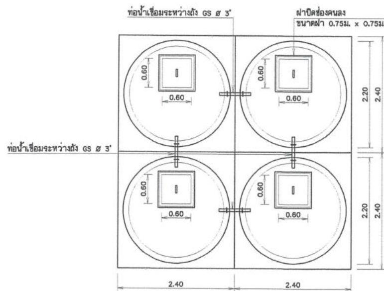
แปลนแบบ 4 ถึง มาตราส่วน 1:40
