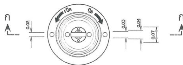
รายละเอียดแบบฝาคอบประตุน้ำเหล็กหล่อ
