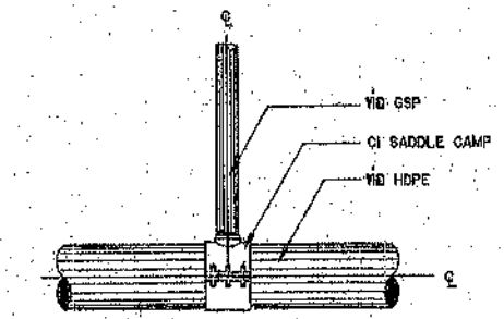
การบรรจุบดท่อสามทาง HDPE กับท่อ GSP แบบ CI SADDLE CLAMP สำหรับอาคารชลประทาน อาคารประจักษ์วิทยาเกษตร อาคารชลประทานอาคาร กรณีท่อส่งน้ำขนาดเส้นผ่าศูนย์กลางน้อยกว่า 315 มม.
