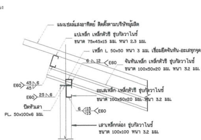
รูปขยาย การติดตั้งโครงหลังคา
