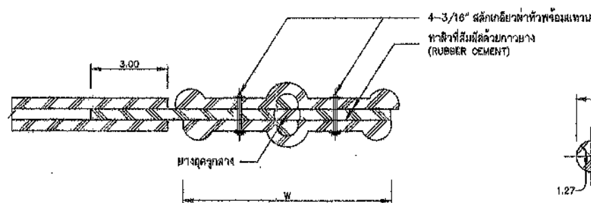
รูปตัด ง-ง ไม่แสดงขนาดส่วน
