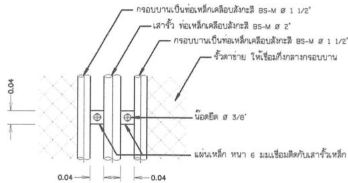
แบบขยายรายละเอียดแสดงการยึดระหว่างตัวกับเสา ไม่แสดงมาตราส่วน
