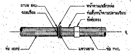
การบรรจุบดท่อ HDPE กับท่อ PVC. ไม่แสดงขนาดบางส่วน
