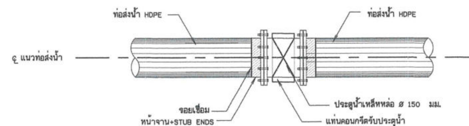
รูปขยายการติดตั้งอาคารควบคุมพลังงาน
