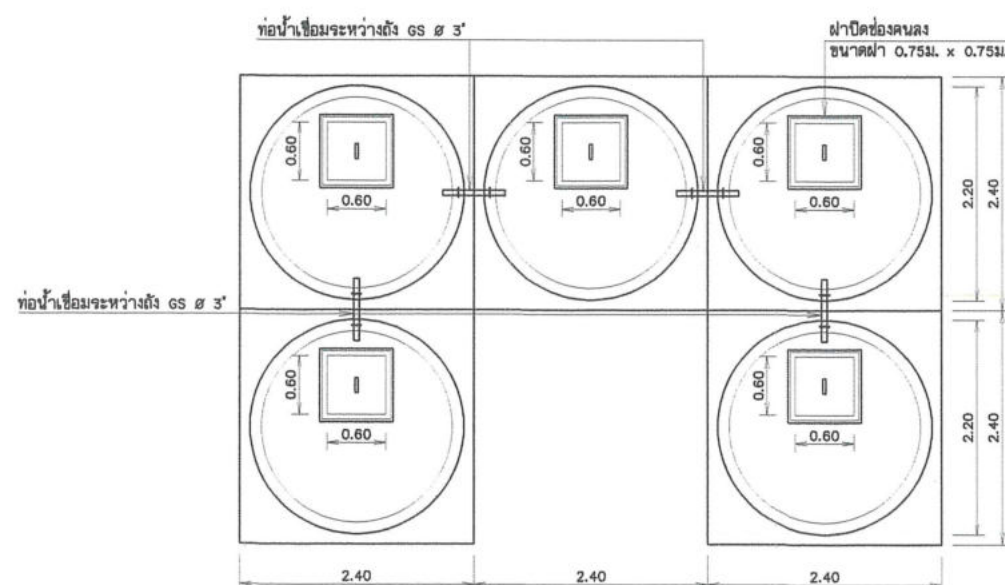
แปลนแบบ 5 ถึง มาตราส่วน 1:40
