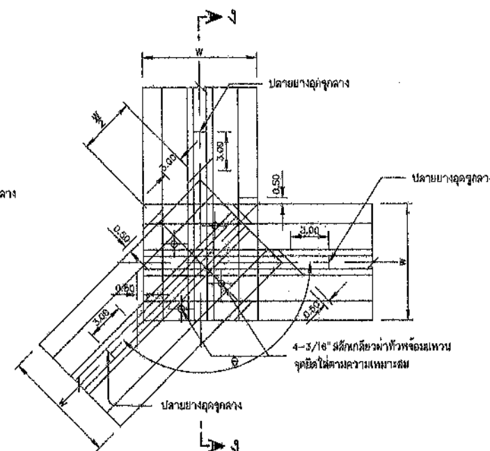
การต่อมุมกันทั้ง 3 ชั้น ไม่แสดงขนาดส่วน
