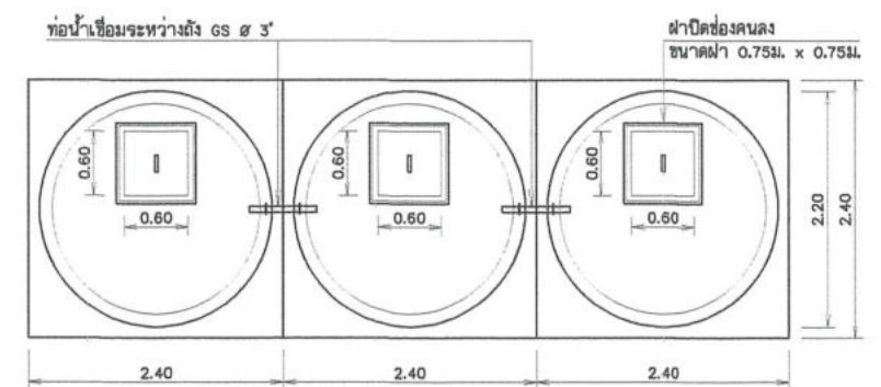
แปลนแบบ 3 ถึง มาตราส่วน 1:40
