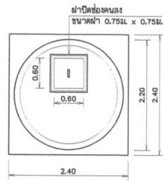
แปลนแบบ 1 ถึง มาตราส่วน 1:40
