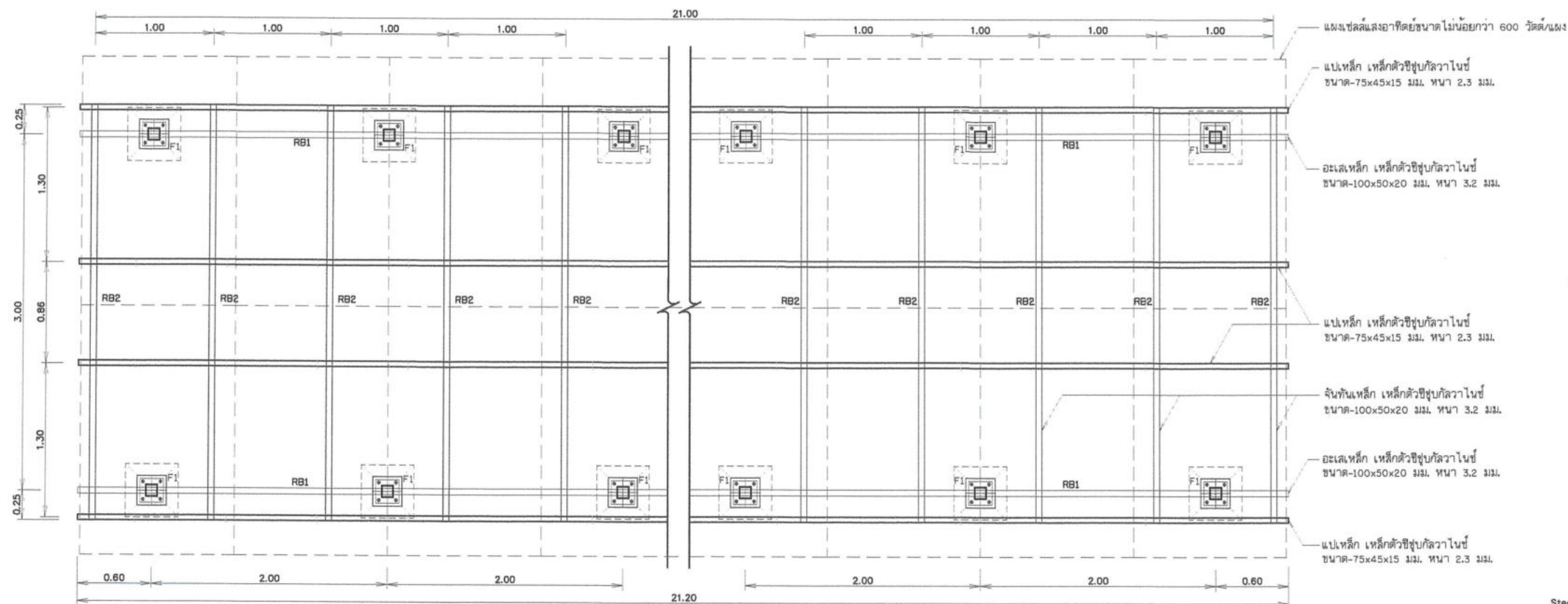
แปลนฐานรากและโครงหลังคา
