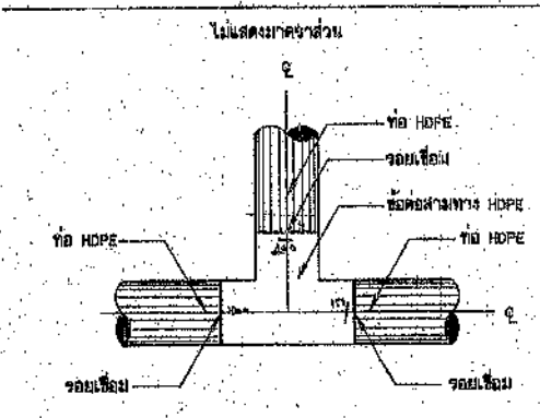
การบรรจุบดท่อสามทาง HDPE กับท่อ HDPE ไม่แสดงขนาดบางส่วน
