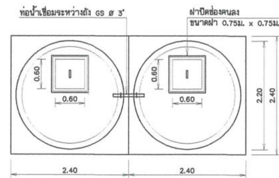
แปลนแบบ 2 ถึง มาตราส่วน 1:40
