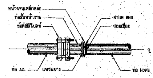
การบรรจุบดท่อ AC กับท่อ HDPE ไม่แสดงขนาดบางส่วน
