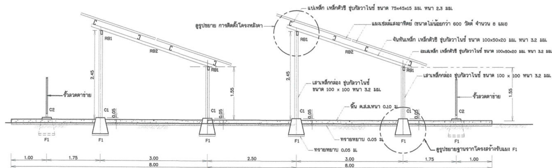
รูปด้านข้าง
