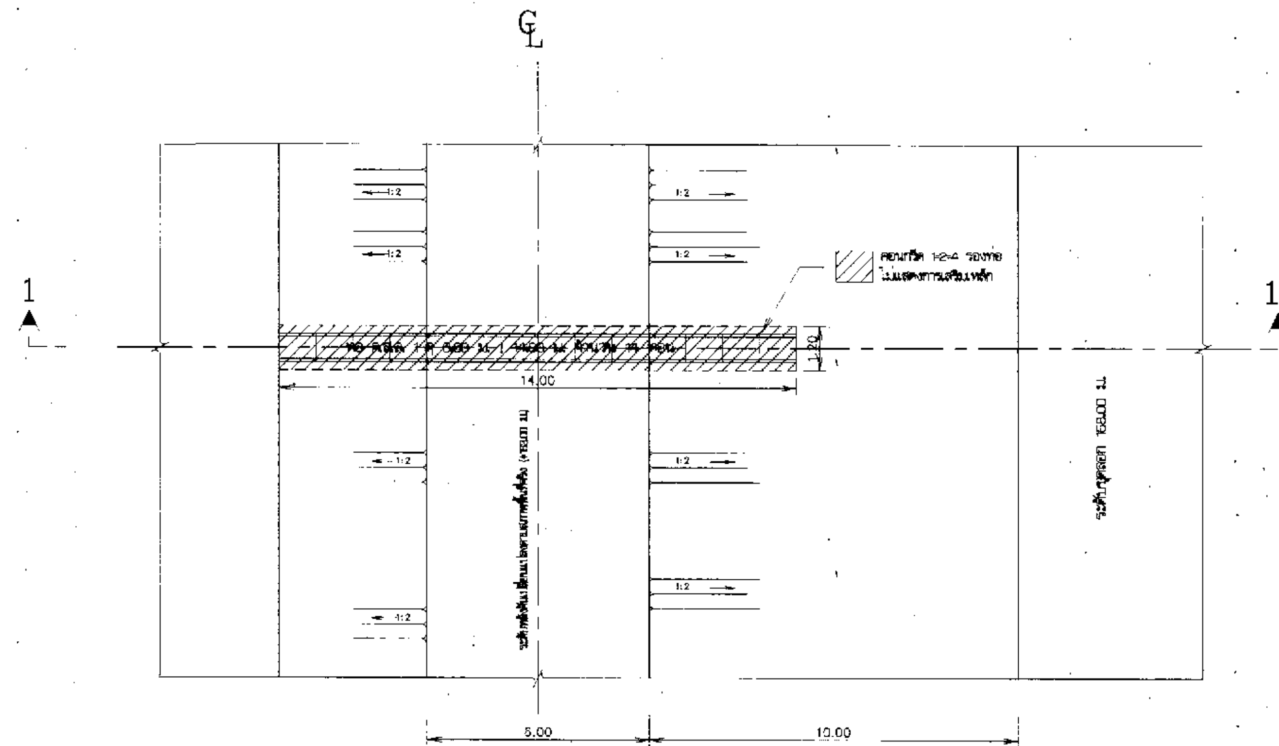
แปลนวางท่อทางน้ำเข้า คสล. ขนาด 1-Ø 0.60 ม. X 14.00 ม. มาตราส่วน 1:100
