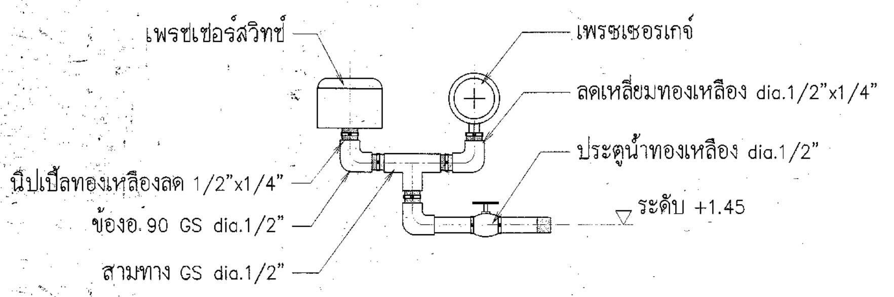
แบบขยายสวิตช์ควบคุมและแก้้ความดัน ไม่แสดงมาตราส่วน
