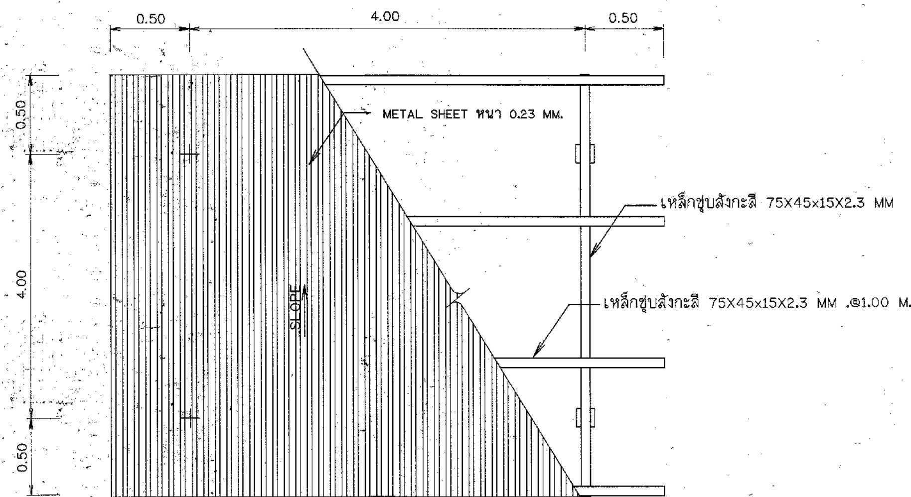
แปลนหลังคา
