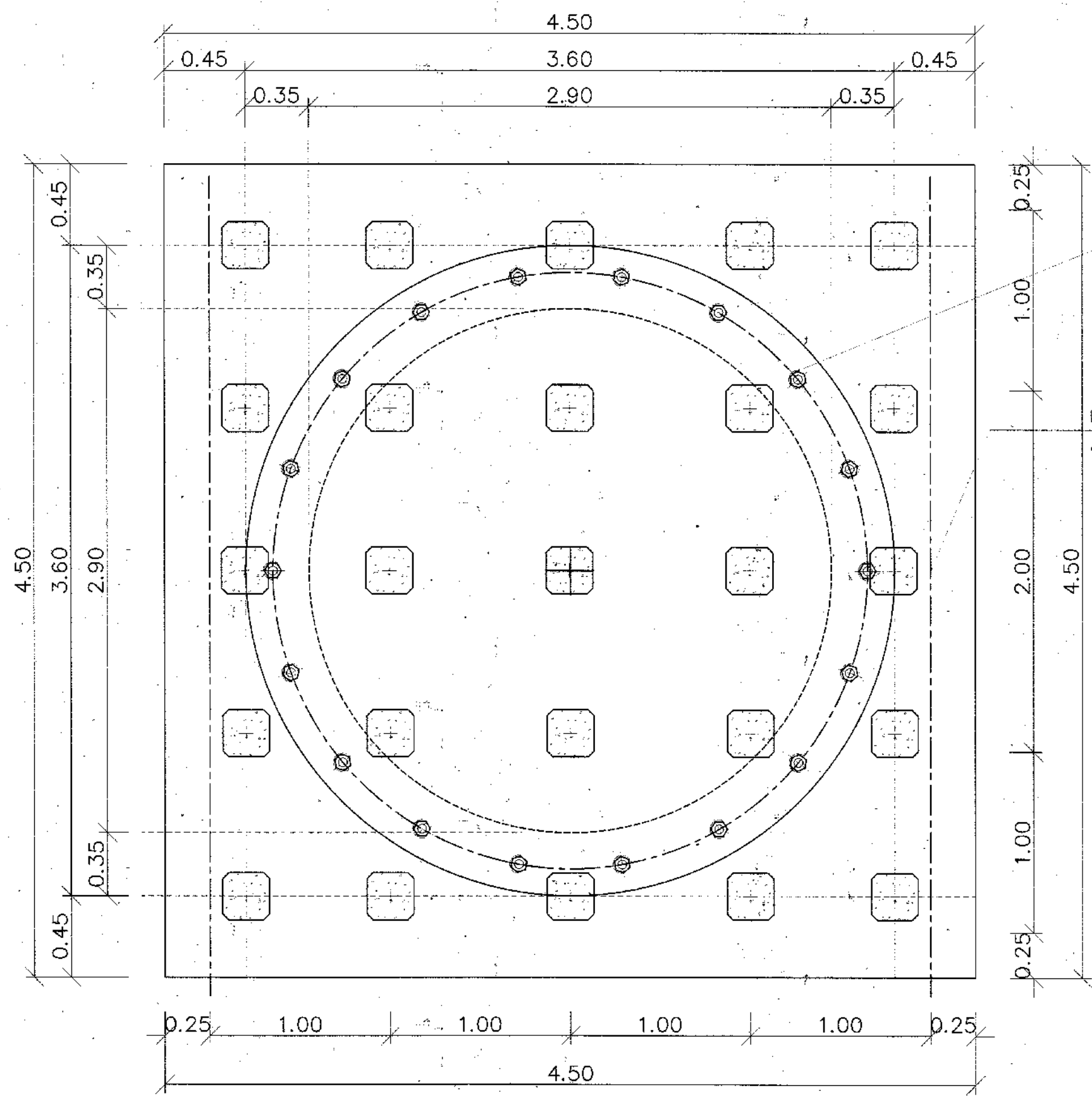
แบบขยายฐานรากหอดึงสูง (แบบเสาเข็ม)
