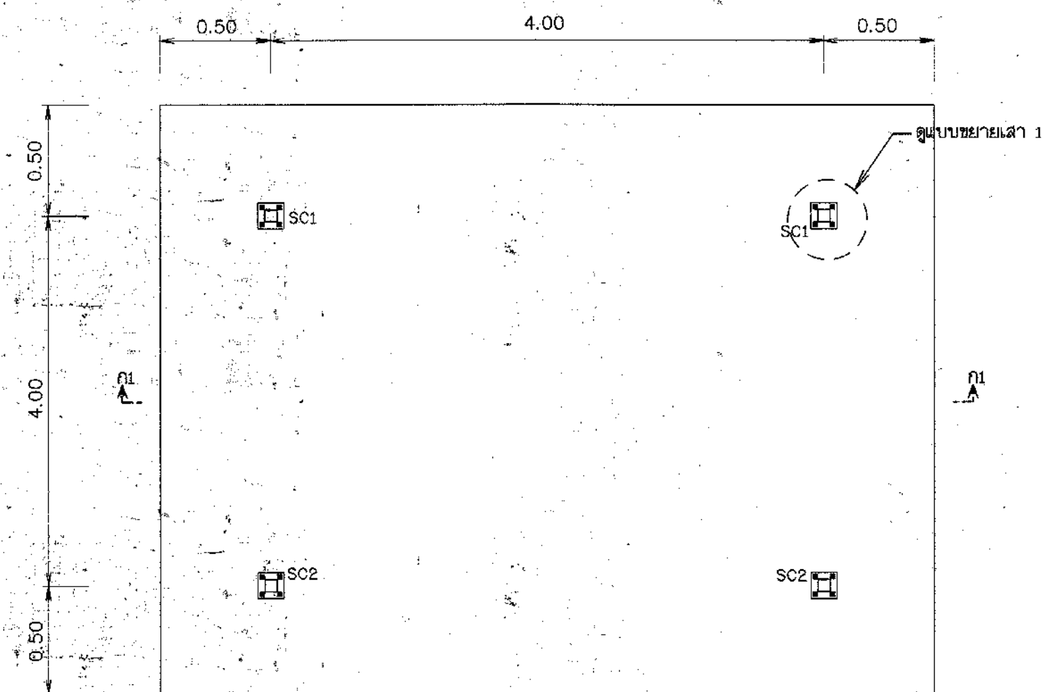
แปลนฐานอาคารวางปั๊ม
