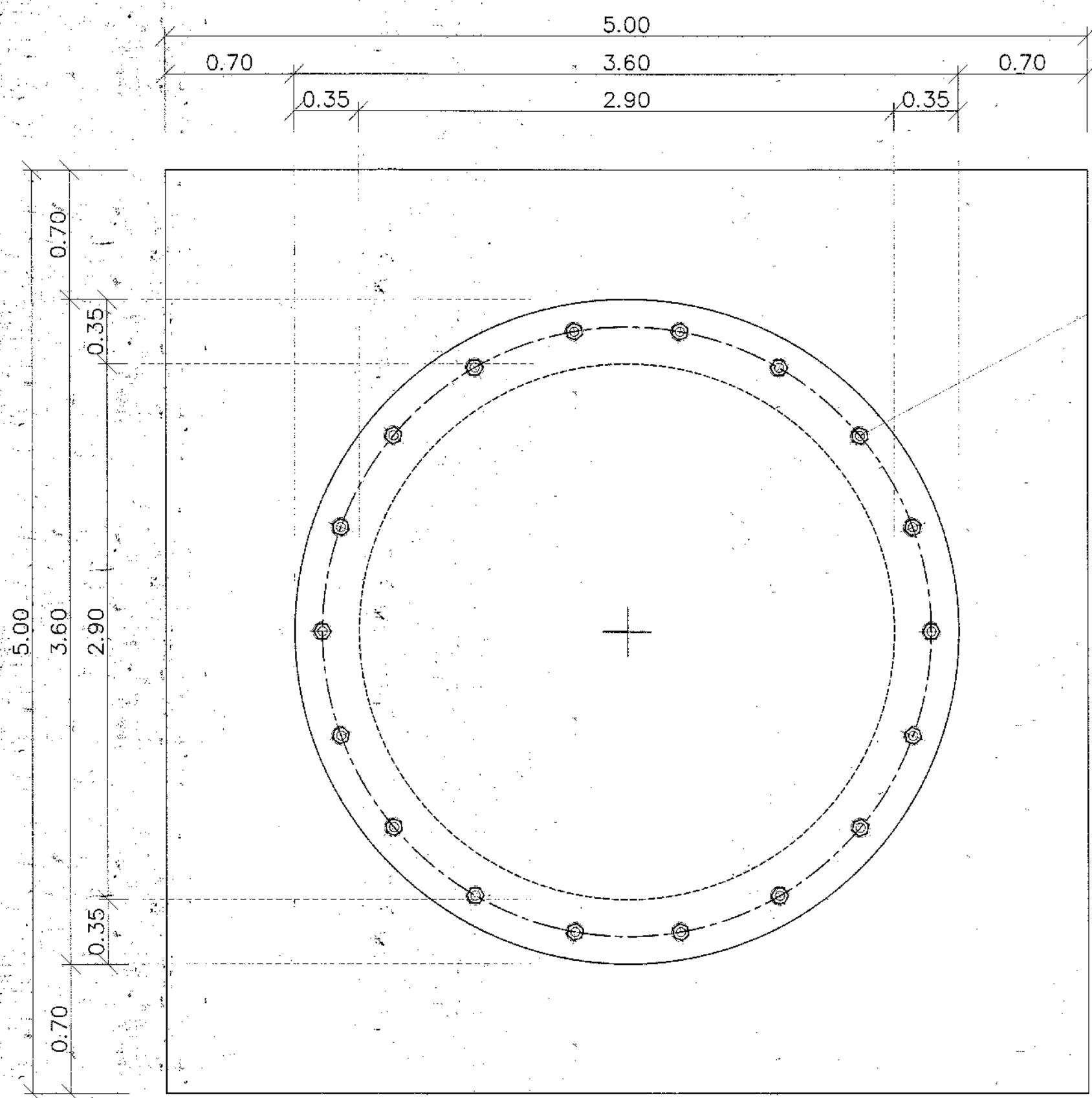
แบบขยายฐานรากหอดึงสูง (แบบฐานแฉ)
