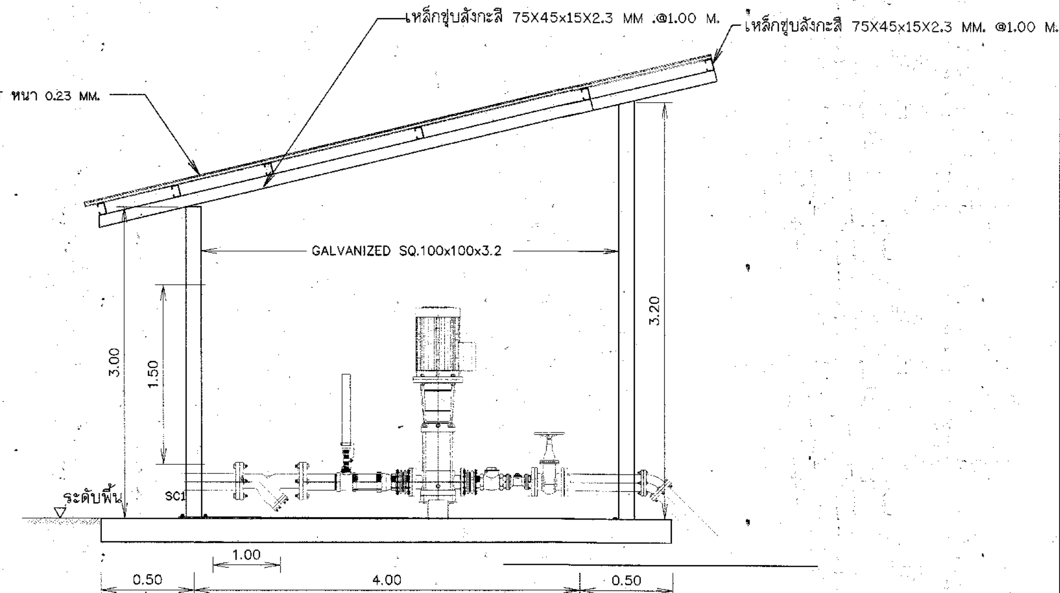
รูปด้าน 2
