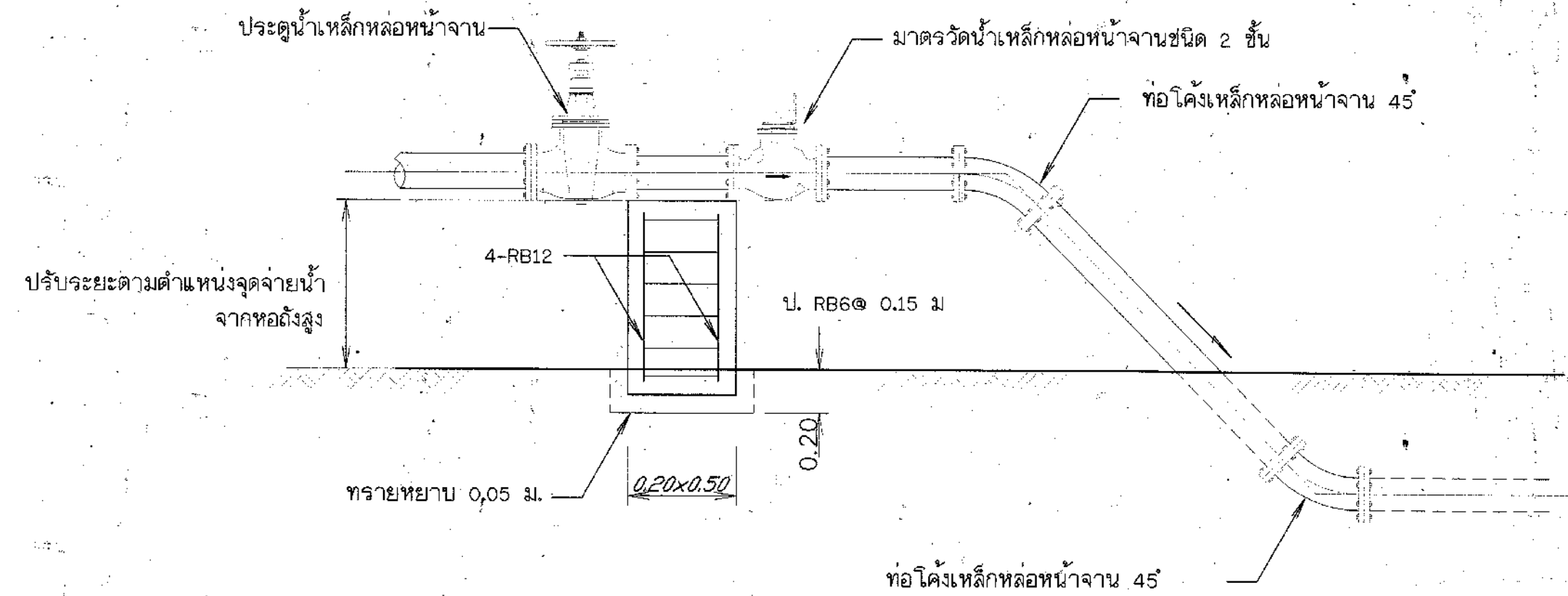
การติดตั้งมาตรวัดน้ำบนพื้นดิน
