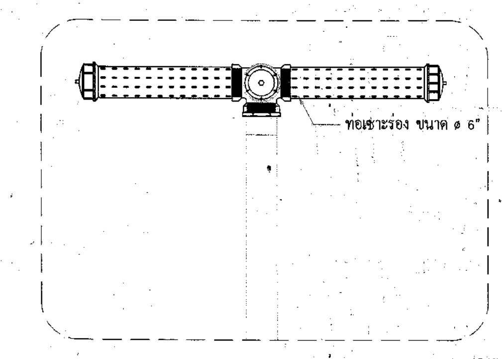
ภาพขยายการติดตั้งท่อระบายน้ำ HDPE หรือ PVC ไม่แสดงมาตราส่วน
