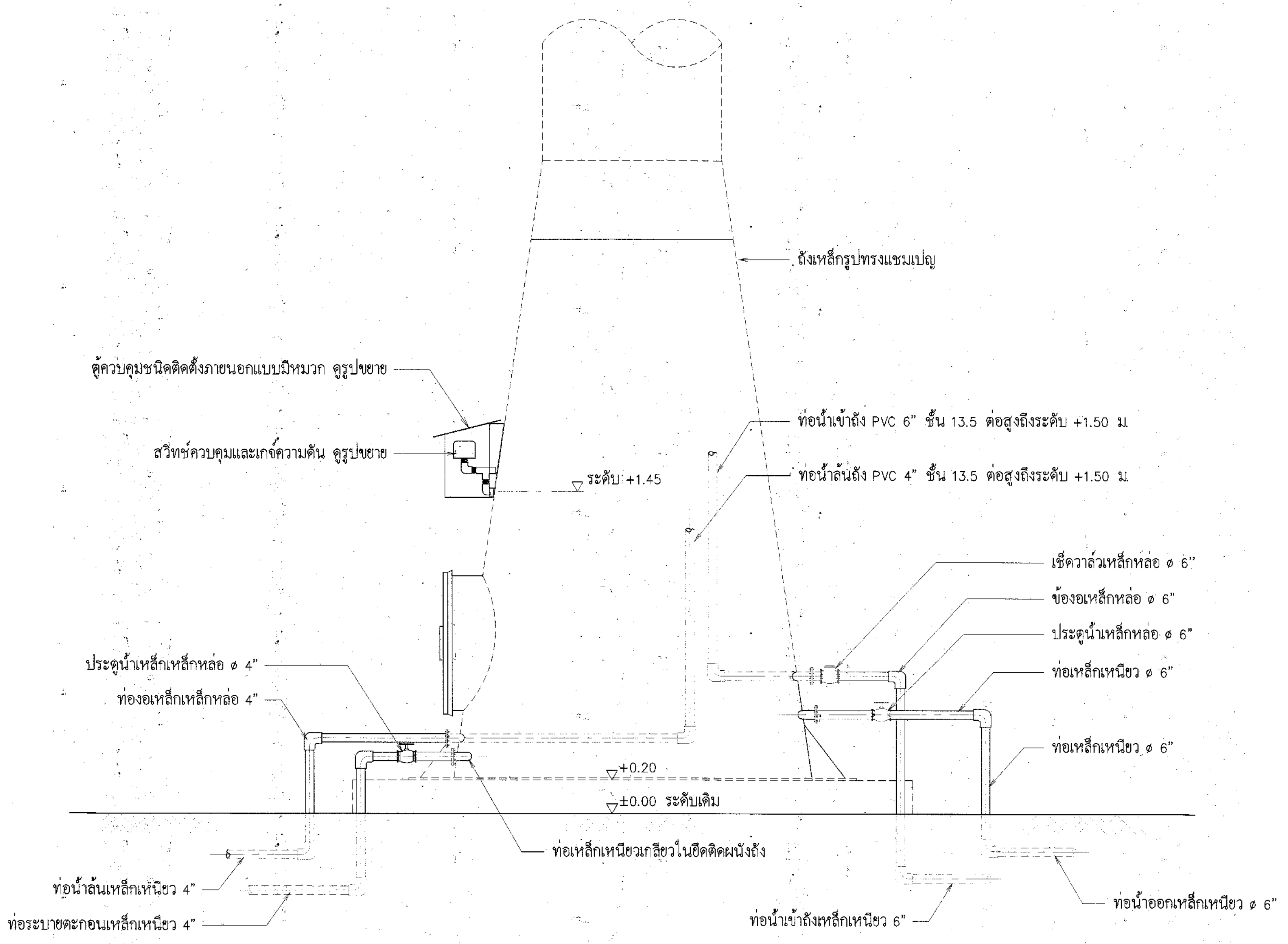
แบบแสดงการเดินท่อในหอถึงสูง ไม่แสดงมาตราส่วน
