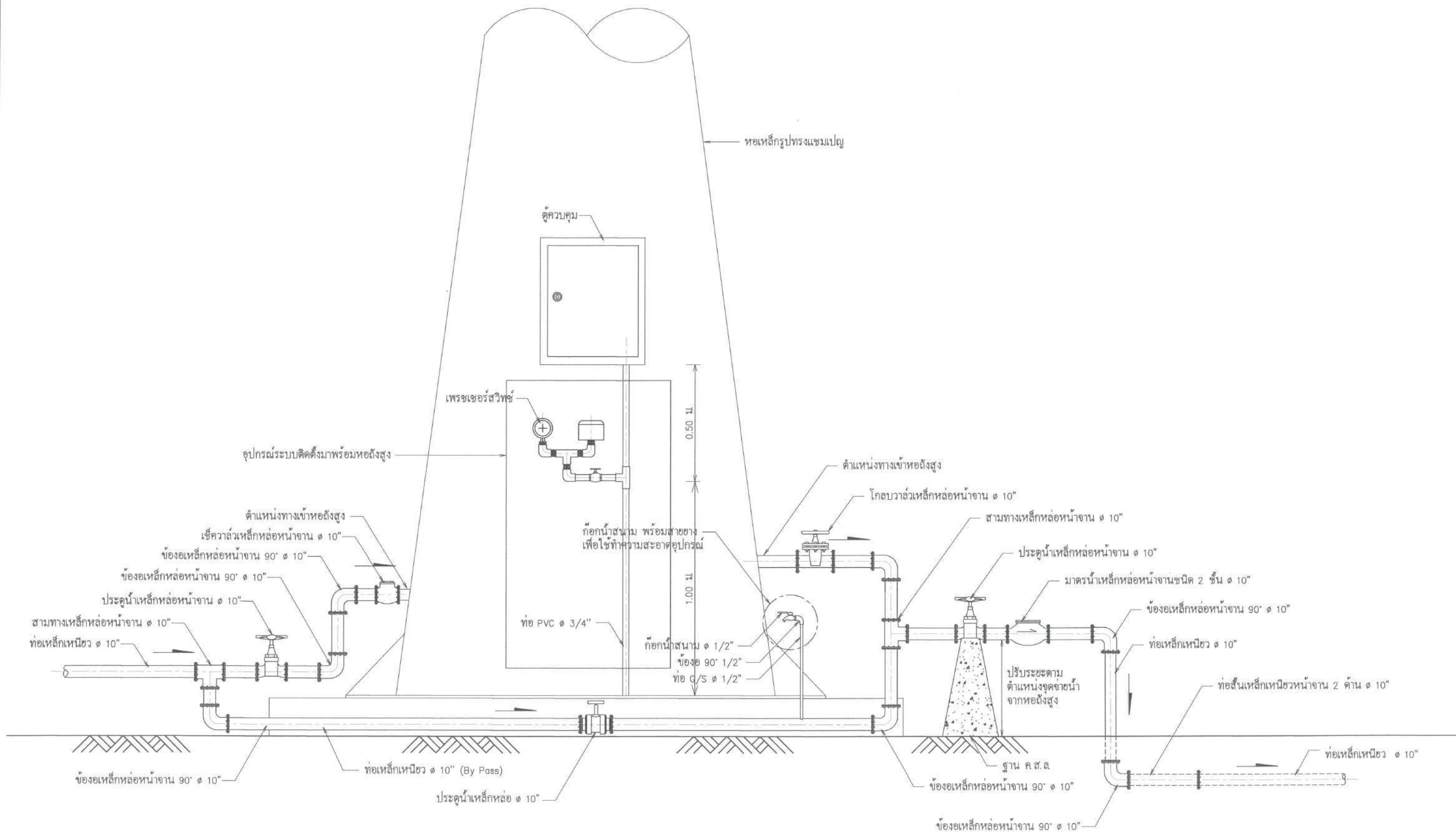
รูปแสดงรายละเอียดการต่อท่อและอุปกรณ์ออกจากถังเหล็กรูปทรงกลมแป้น
