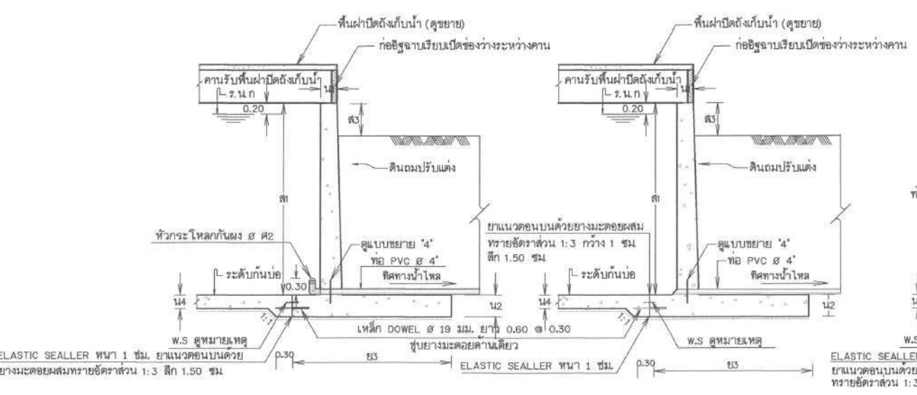
รูปตัดท่อส่งน้ำ
