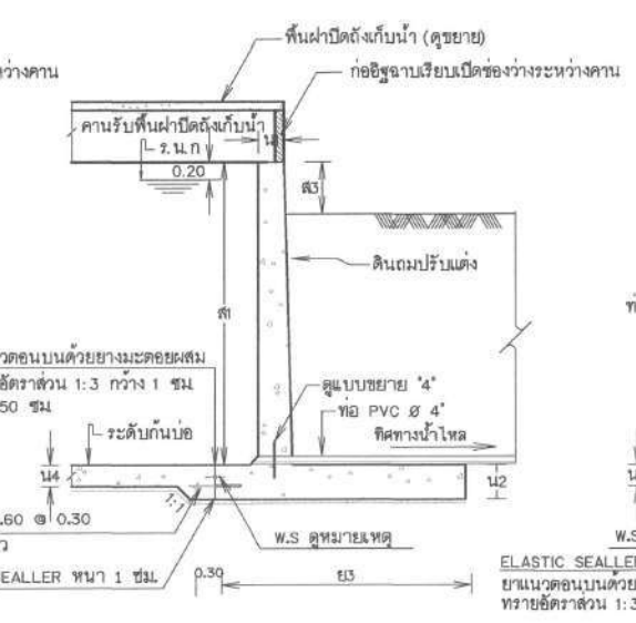
รูปตัดท่อระบายตะกอน
