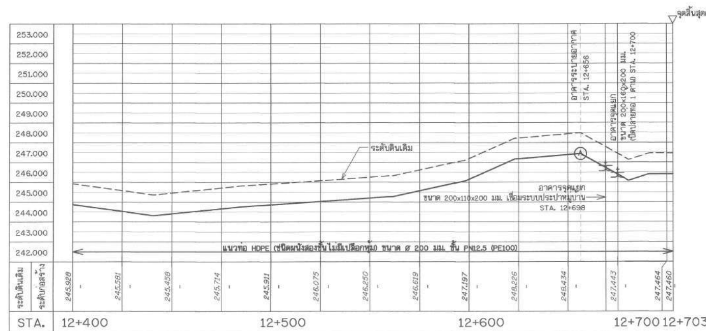
รูปตัดตามแนวยาว สาย 2RMP STA. 12+400 - 12+703
