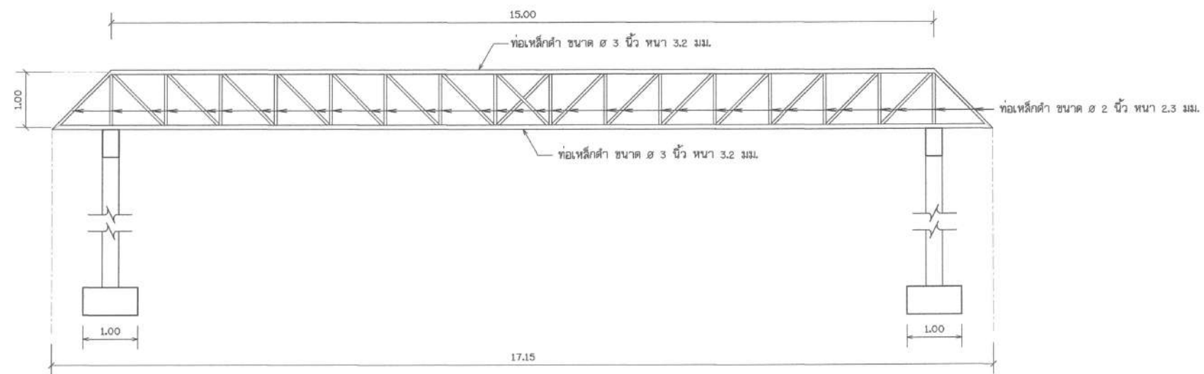
รูปด้านสะพานรับท่อส่งน้ำ
