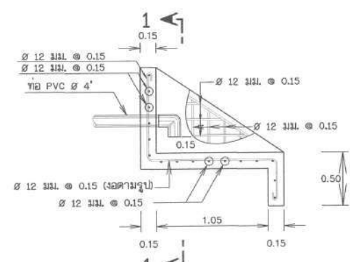
ขยายอาคารปลายท่อระบายน้ำ
