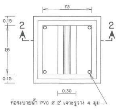
แปลนบ่อประจุบับน้ำ
