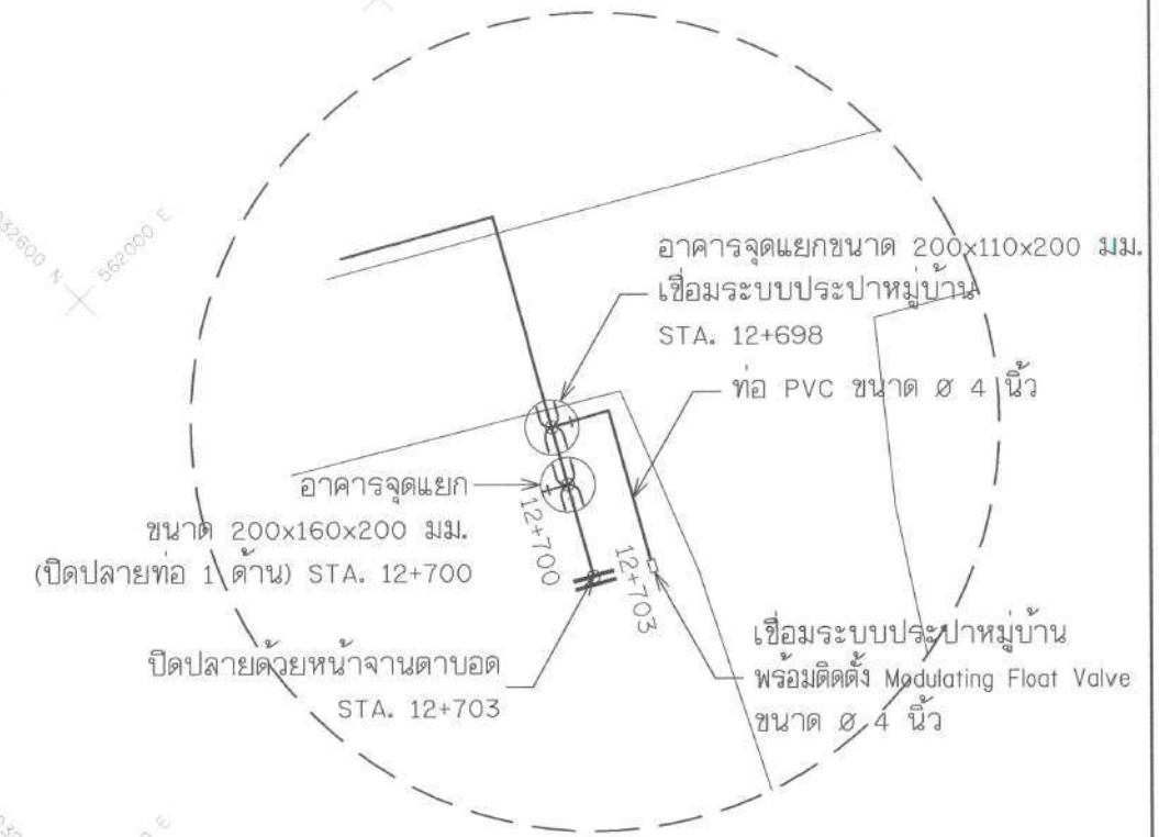
แบบขยาย 1
