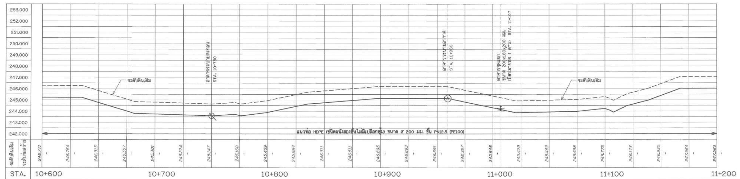
รูปตัดตามแนวยาว สาย 2RMP STA. 10+600 - 11+200
