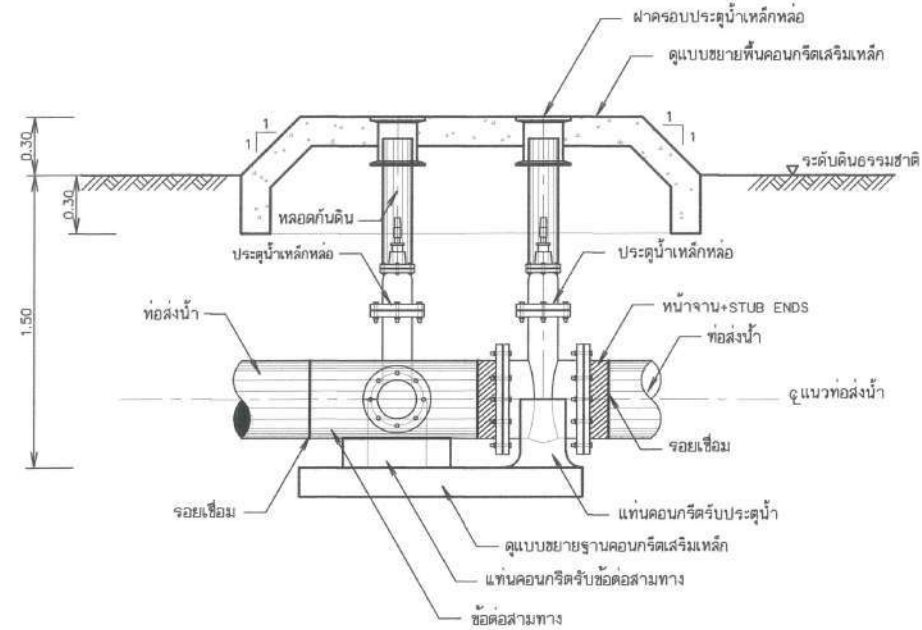
รูปตัดอาคารจุดแยก
