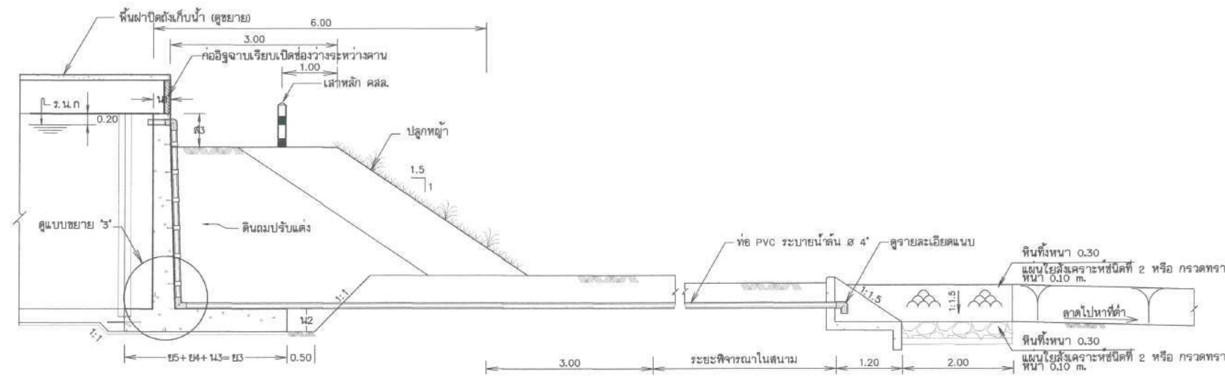
รูปตัด ข - ข
