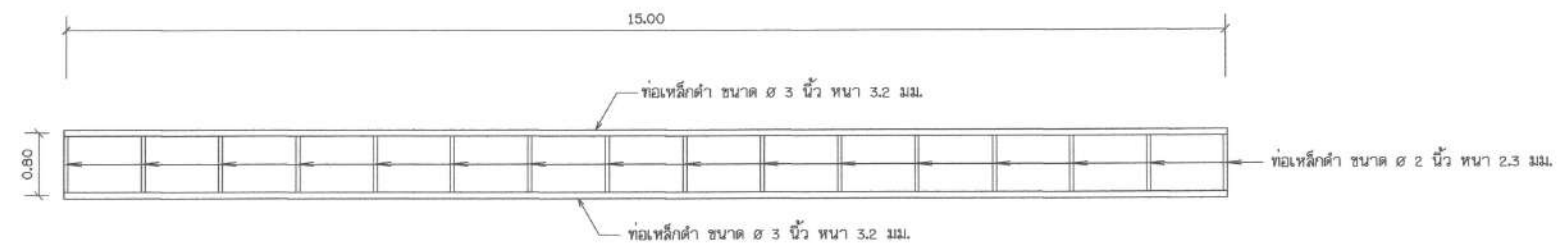
รูปด้านบนสะพานรับท่อส่งน้ำ
