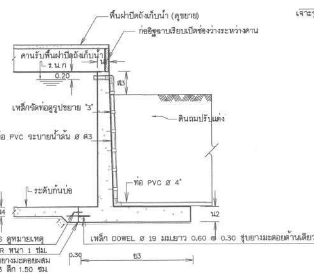
รูปตัดท่อรับน้ำหรือท่อระบายน้ำ
