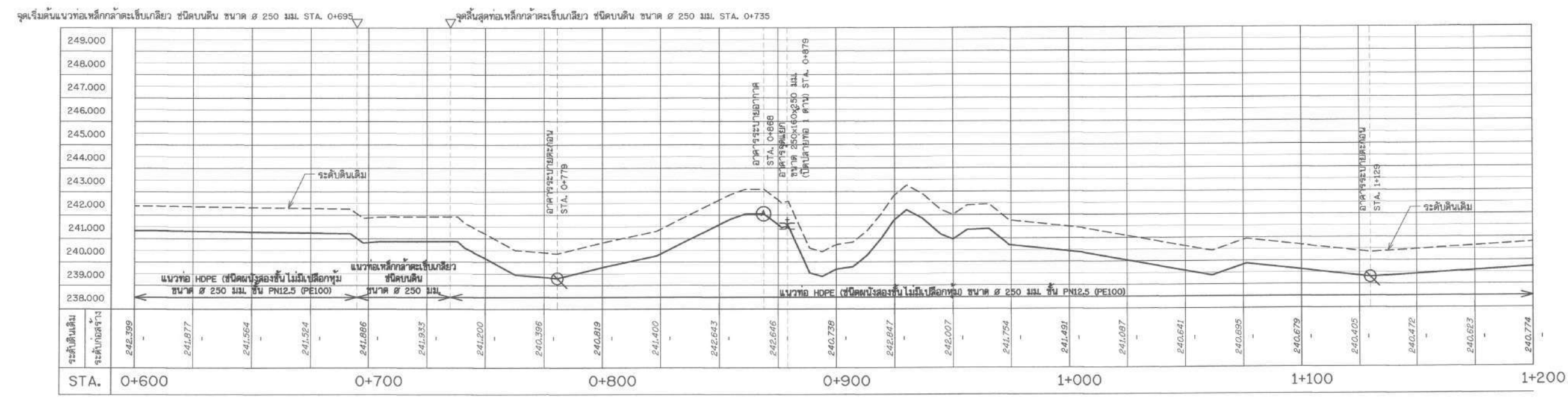
รูปตัดตามแนวยาว สาย 1RMP STA. 0+600 - 1+200 มาตราส่วน 1:1,000 แนวตั้ง 1:100
