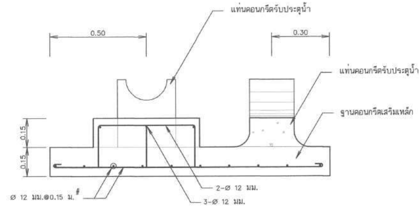
รูปตัด ก - ก
