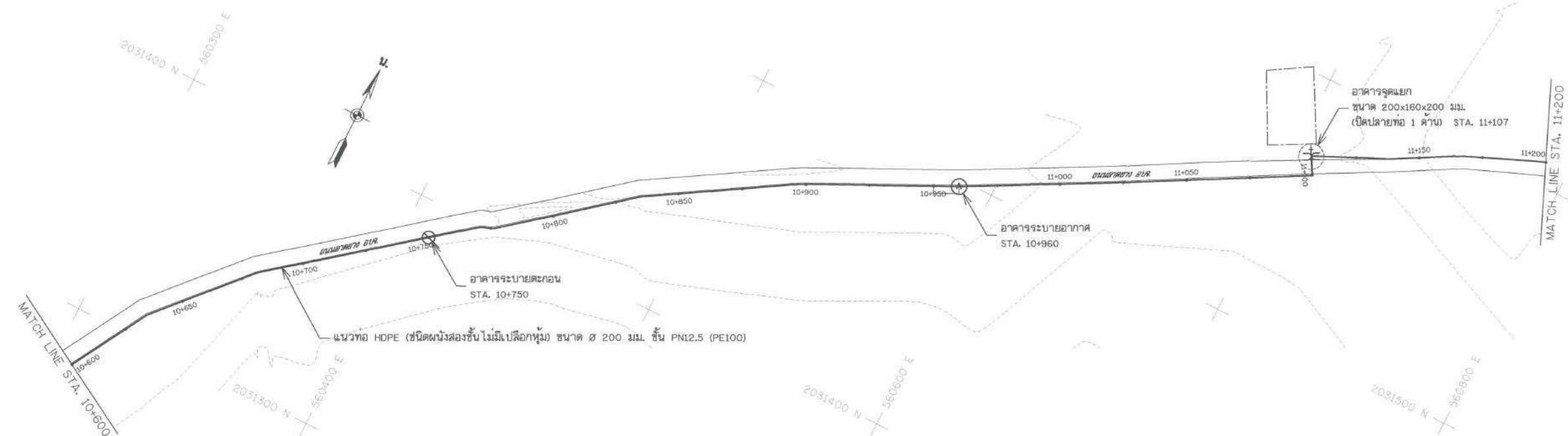
แปลนทั่วไป สาย 2RMP STA. 10+600 - 11+200
