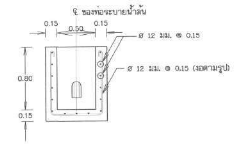
รูปตัดแนว 1 - 1
