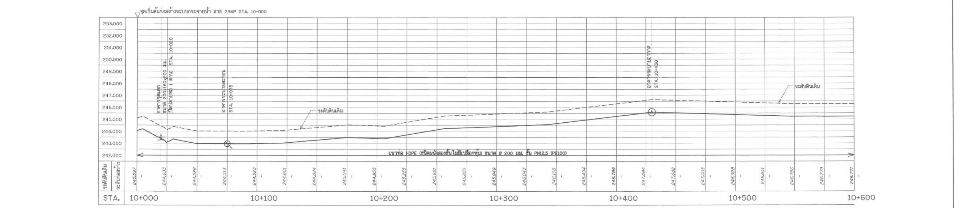
รูปตัดตามแนวยาว สาย 2RMP STA. 10+000 - 10+600
