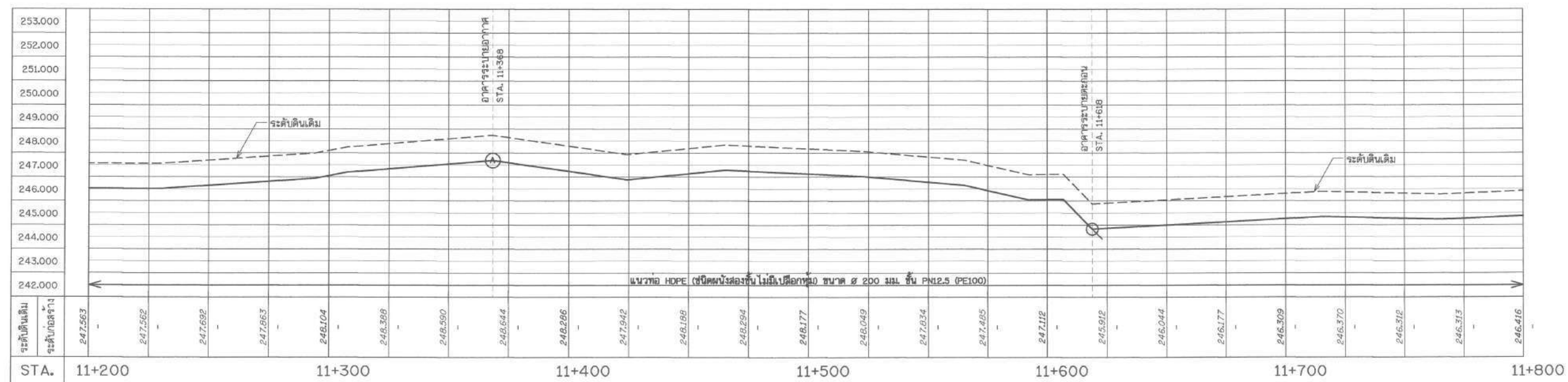
รูปตัดตามแนวยาว สาย 2RMP STA. 11+200 - 11+800
