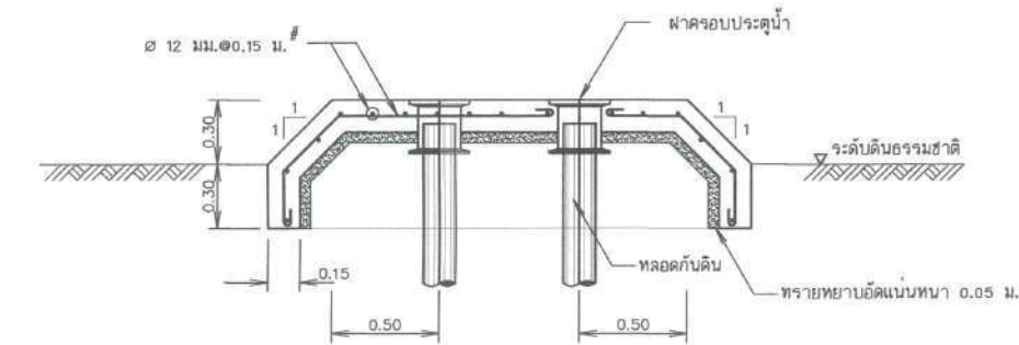
รูปขยายการเสริมเหล็กพื้นคอนกรีตเสริมเหล็ก
