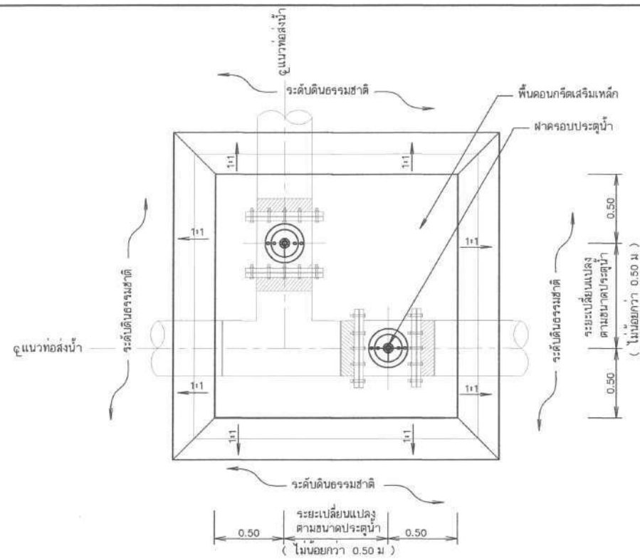
แปลนอาคารจุดแยก
