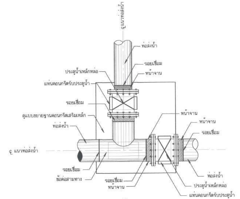
รูปขยายการติดตั้งอาคารจุดแยก
