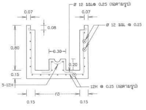
เหล็กเสริมบ่อประจุน้ำ
