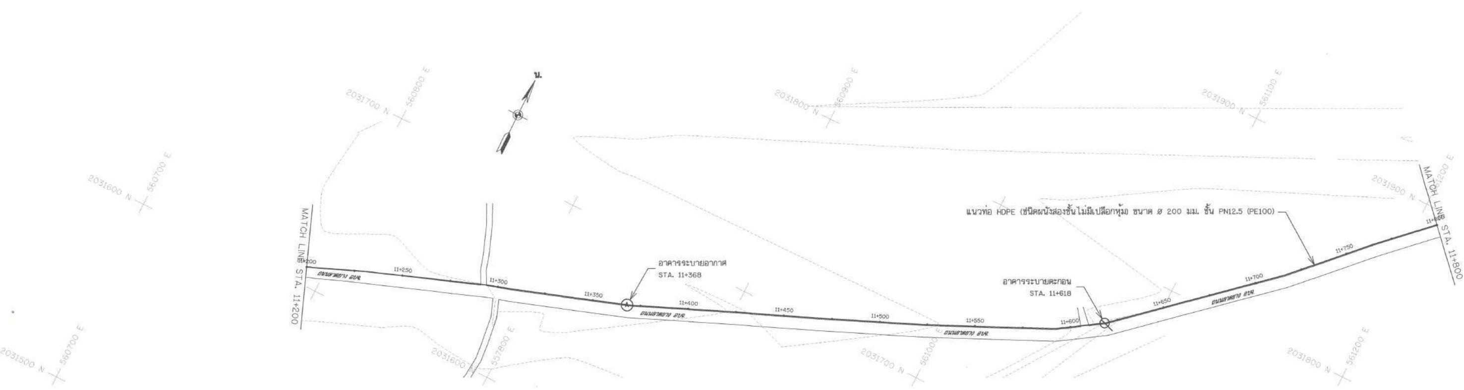
แปลนทั่วไป สาย 2RMP STA. 11+200 - 11+800
