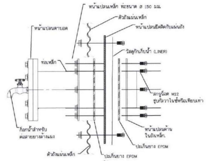
แบบขยาย หน้าแปลนคาบอด
