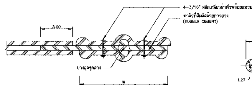
รูปตัด ง-ง
