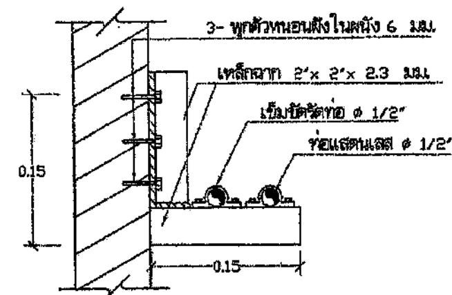
ขยายเหล็กกับท่อสารส้มลงช่องไฮดรอลิค 1:5
