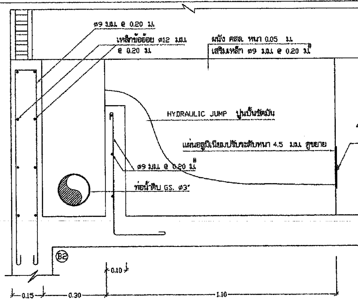
รูปตัด ๑ - ๑ 1 : 10
