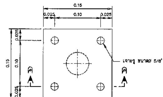
ภาคกลาง 1:5
