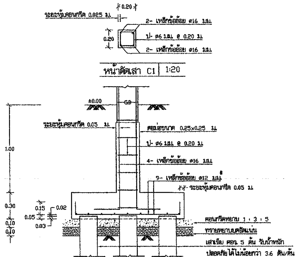
รูปตัด ข - ข 1:20
