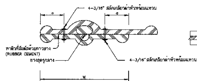
รูปตัด ช-ช
