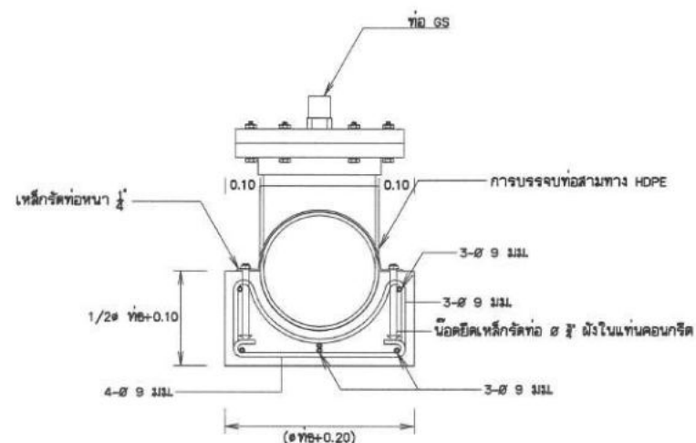
รูปตัดขยาย "1" มาตราส่วน 1:10
