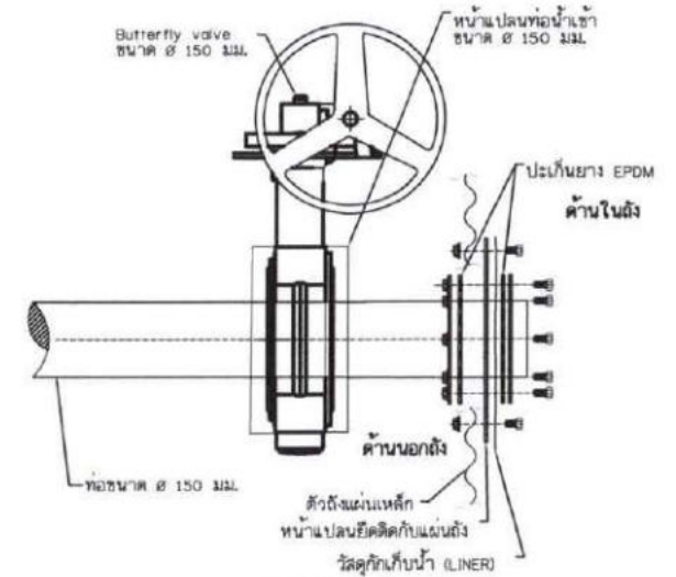
แบบขยาย 4
