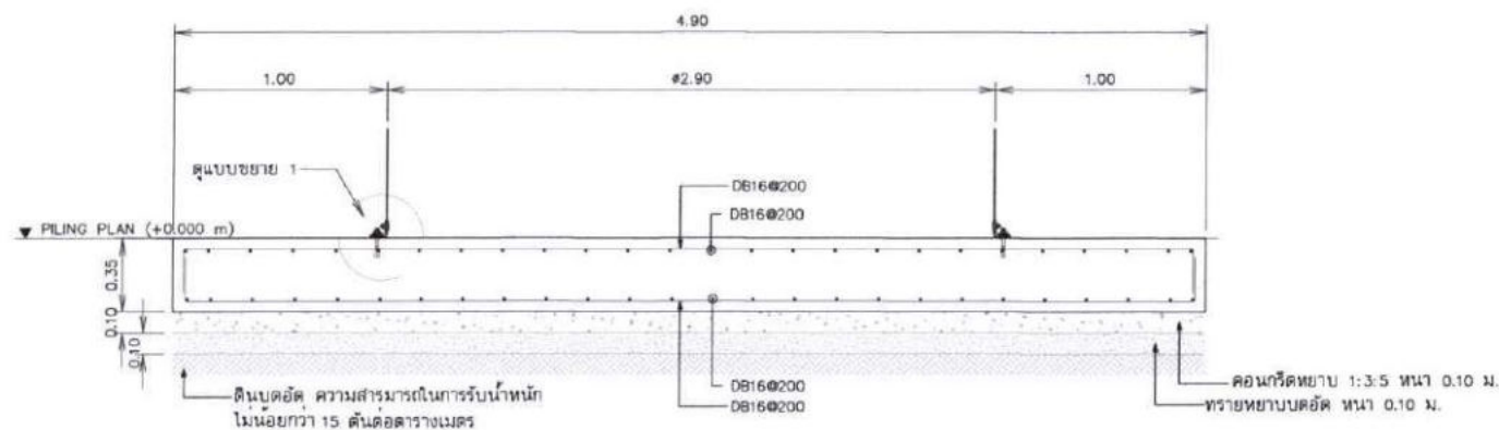
รูปตัด ก - ก
