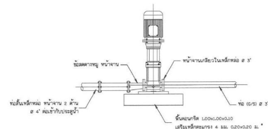
14. การต่อท่อเครื่องสูบน้ำ ไม่แสดงมาตราส่วน
