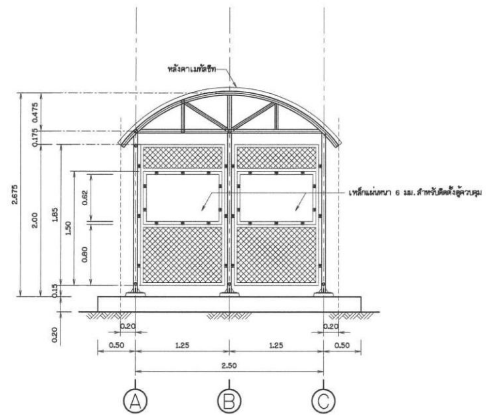
รูปด้าน 2 ไม่แสดงขนาดราดวัน
