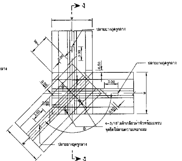
การต่อมุกันทั้ง 3 ชั้น
