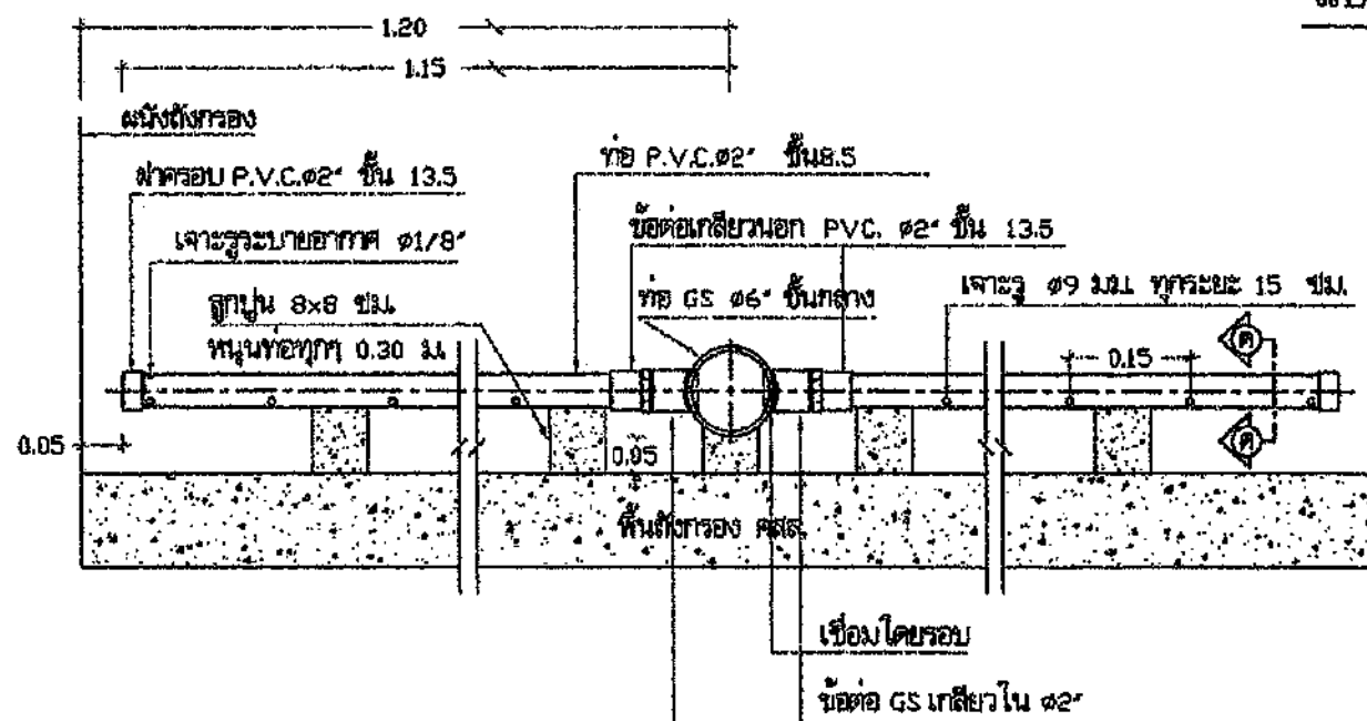
แบบขยายท่อหักงอปลา 1:20
