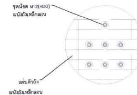
แบบขยาย 10-การประกอบแผ่น ไม่แสดงมาตราส่วน
