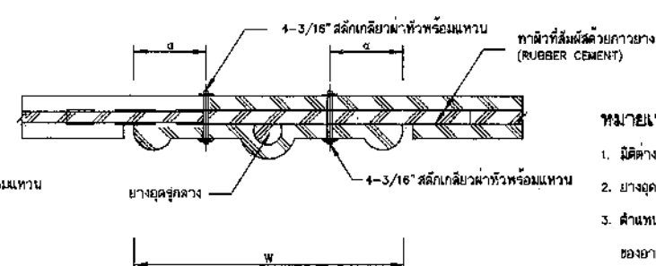
รูปตัด จ-จ
