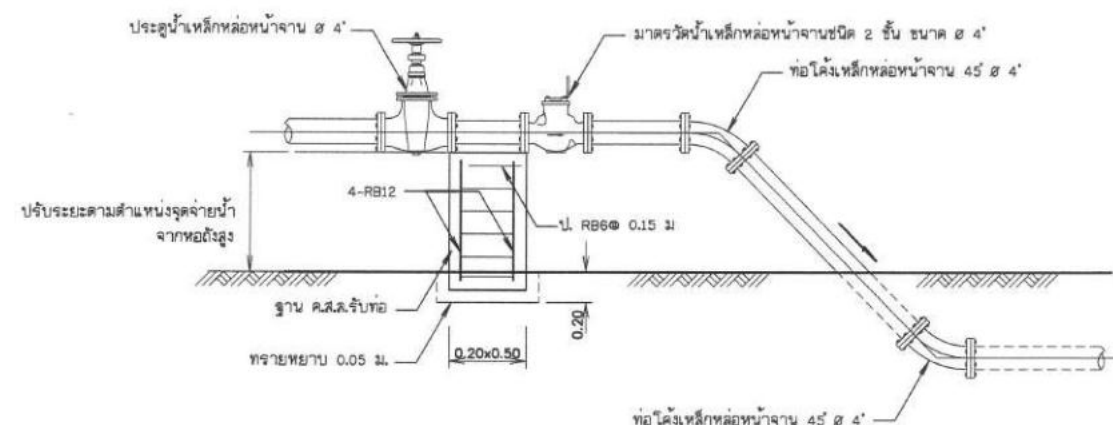
13. การติดตั้งมาตรวัดน้ำบนพื้นดิน Ø 4" ไม่แสดงมาตราส่วน
