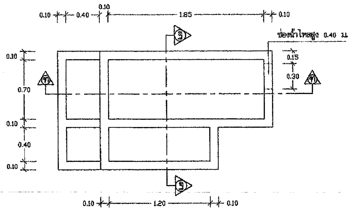
แบบขยายเชิงสารส้มและถังปูนขาว 1:25
