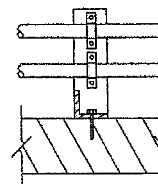
ขยายเหล็กกับท่อสารส้มลงช่องไฮดรอลิค 1:5
