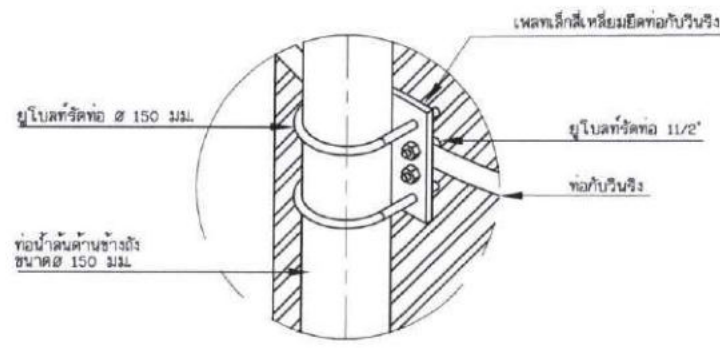
แบบขยาย 2-รูปแบบการประกอบแผ่นฉลึง
