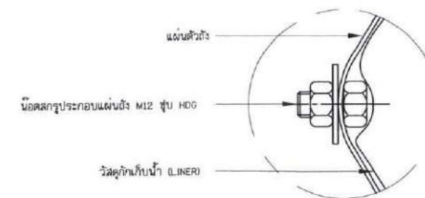
แบบขยาย 9-รูปแบบการประกอบแผ่นถัง ไม่แสดงมาตราส่วน
