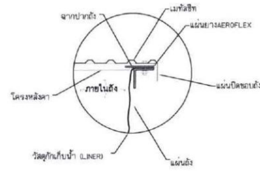
แบบขยาย 3-จุดยึดหลังคากับแผ่นฉลึง
