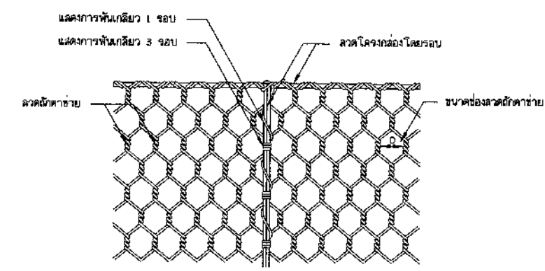
รูปแสดงการผันลวดระหว่างกล่องลวดตาข่ายและฝาปิด
