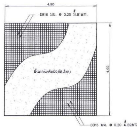
แปลนพื้น
