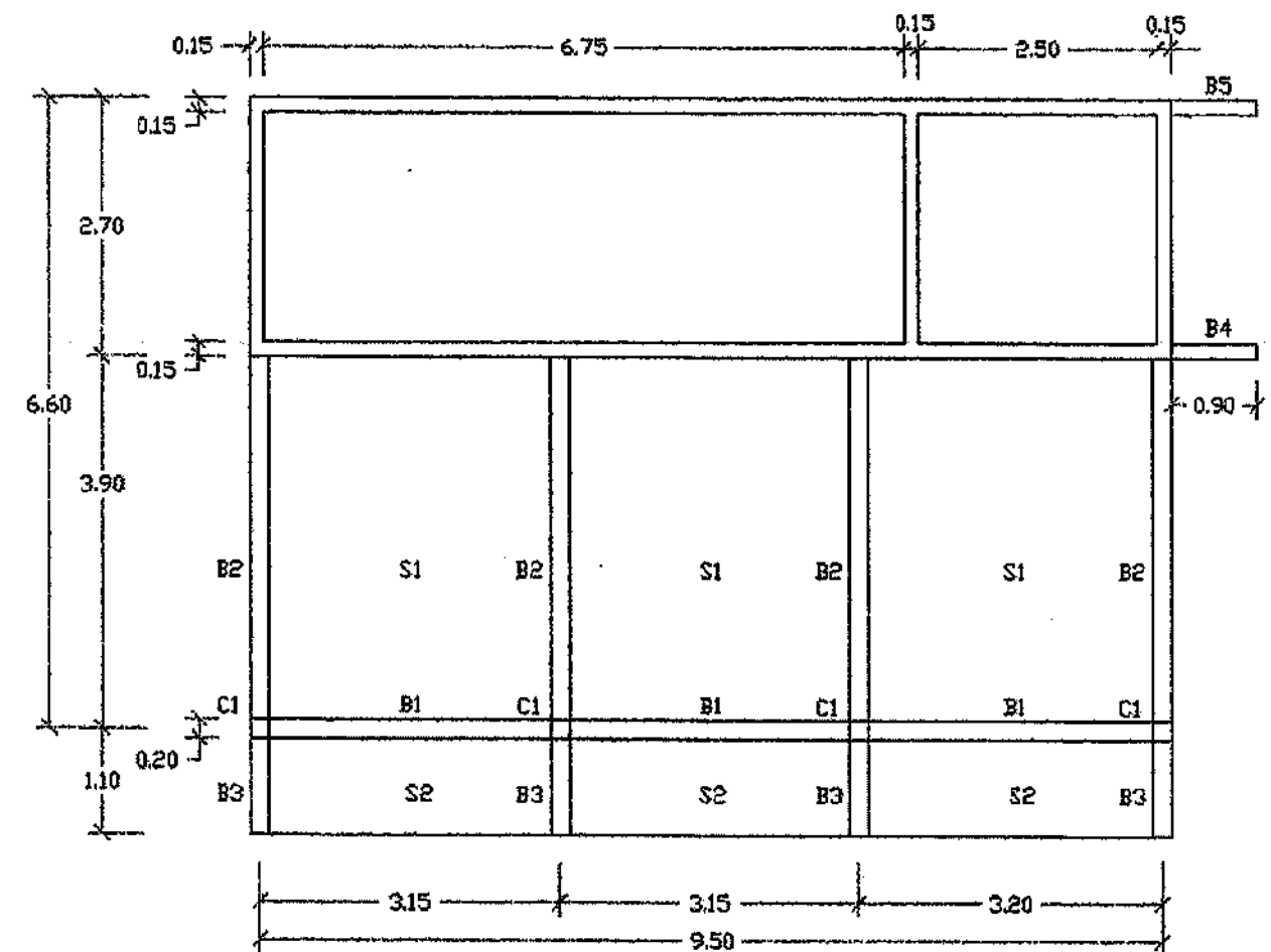
แปลนคานขึ้นบน 1:75
