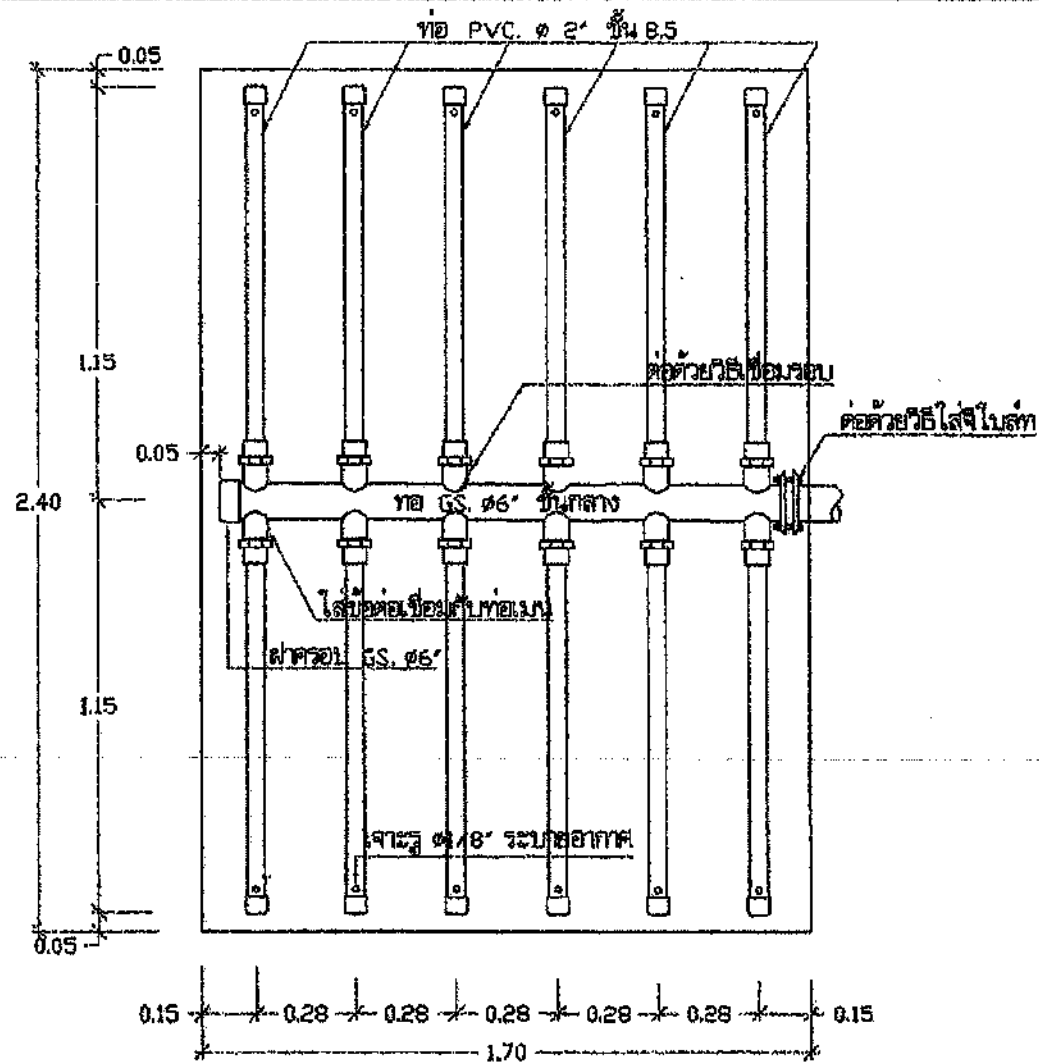
แบบขยายท่อหักงอปลา 1:20
