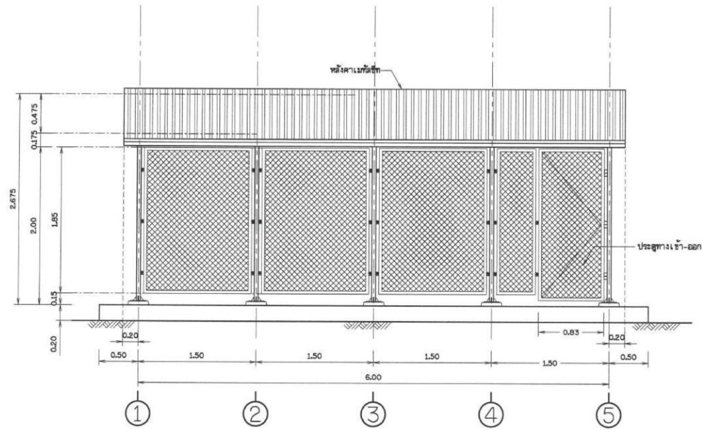
รูปด้าน 1 ไม่แสดงขนาดราดวัน
