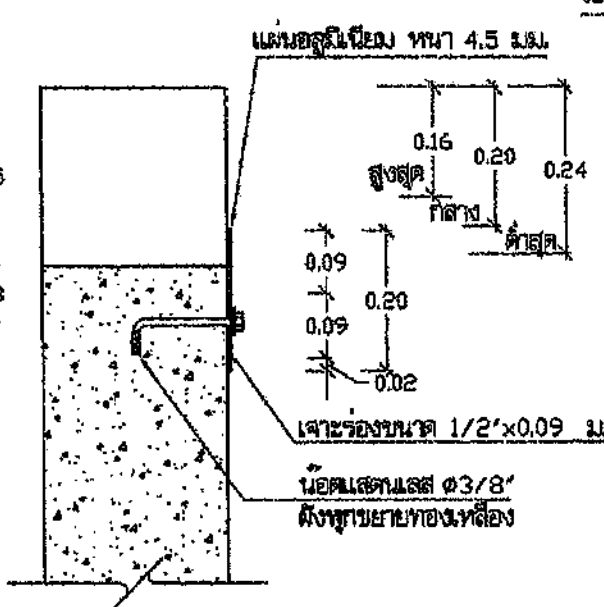
แบบขยายแผ่นปิดกั้นน้ำ 1 : 10
