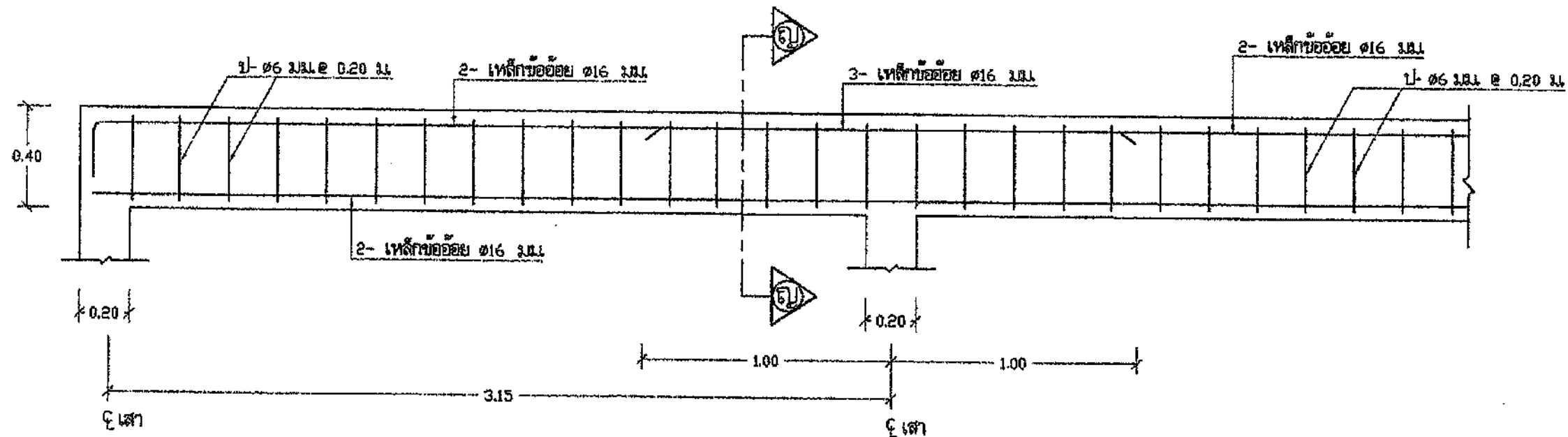
แบบขยายคาน B 1 1:20
