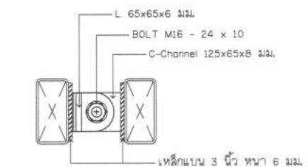
แบบขยายตัวเชื่อม มาตราส่วน 1 : 100
