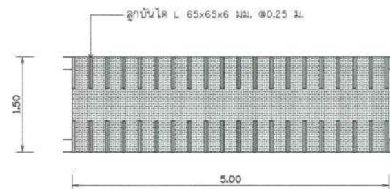
แบบขยายลูกบันไดสะพานช่วงที่ 3 มาตราส่วน 1 : 100
