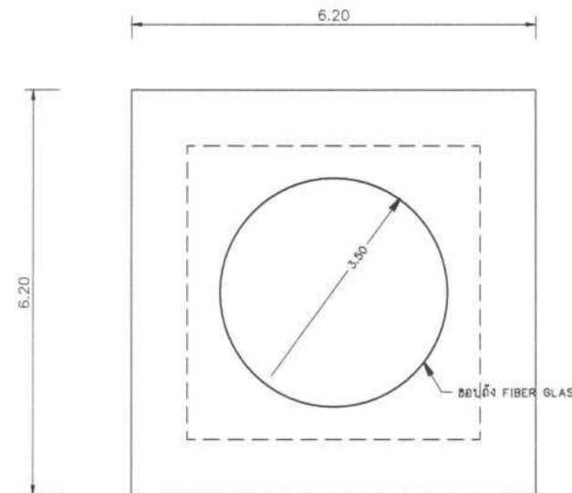
แปลนฐานจากแผ่ มาตราส่วน 1 : 100
