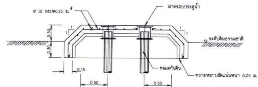
รูปตัดอาคารจุดแยก มาตราส่วน 1:20
