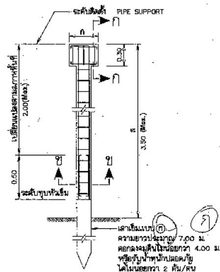
การเสริมเหล็กตอม่อแบบที่ 1 ไม่แสดงขนาดรวม
