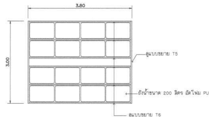
แบบขยายแพลอยสะพานช่วงที่ 2 มาตราส่วน 1 : 100
