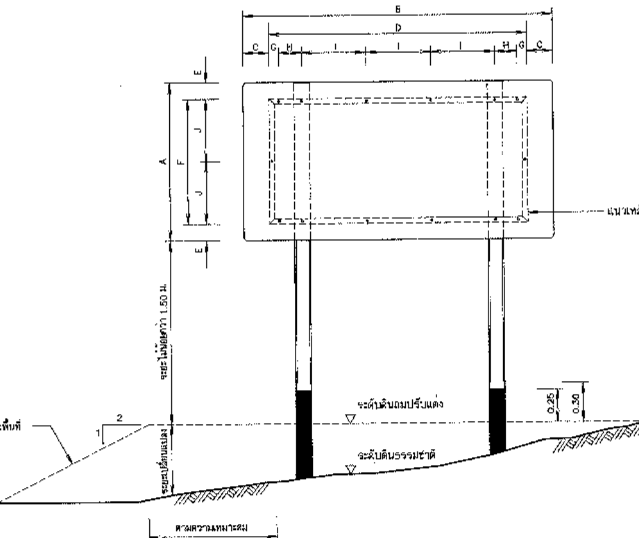
รูปแสดงการประกอบแผ่นป้าย มาตรฐาน 1:20
