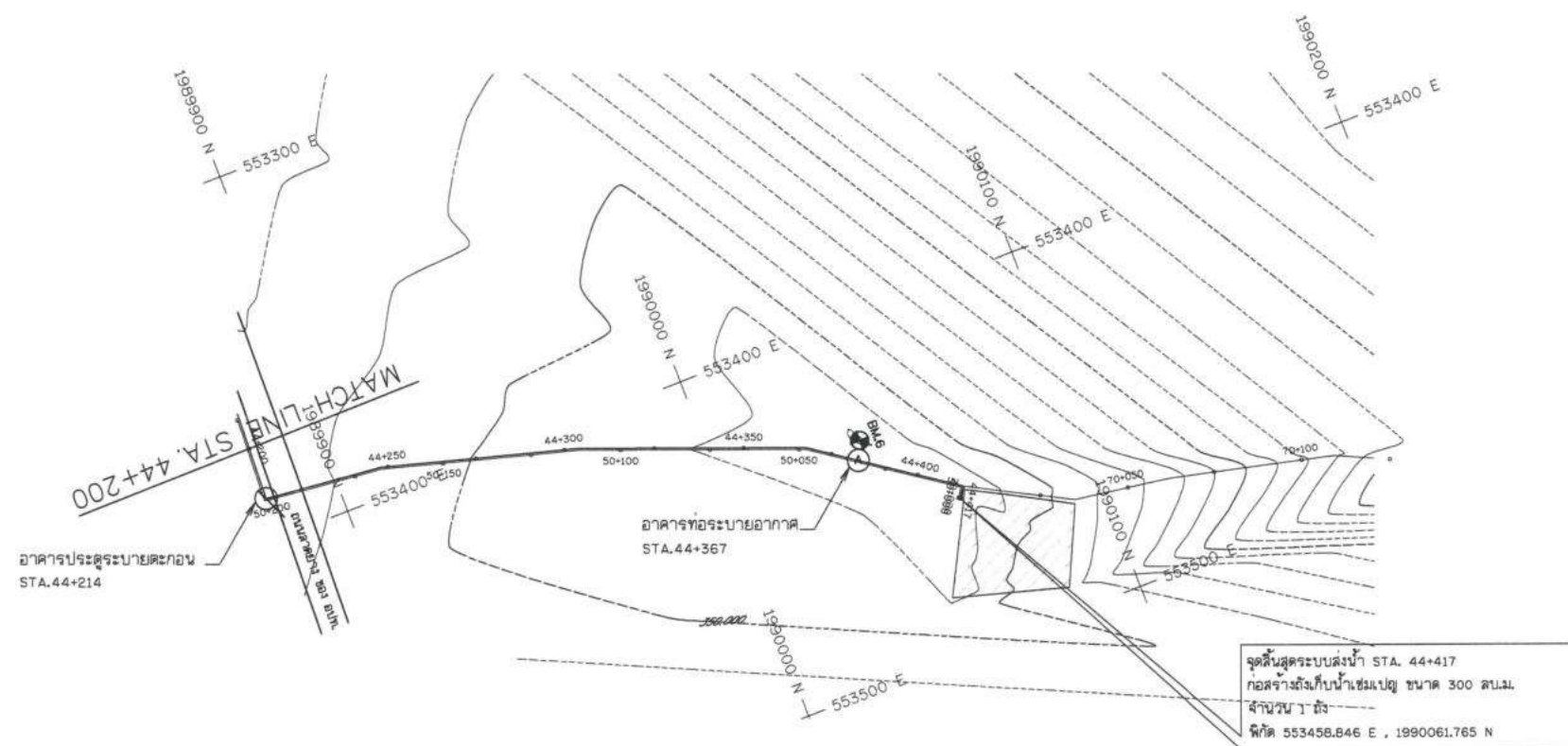
แปลนทั่วไป STA. 44+200 - 44+417
