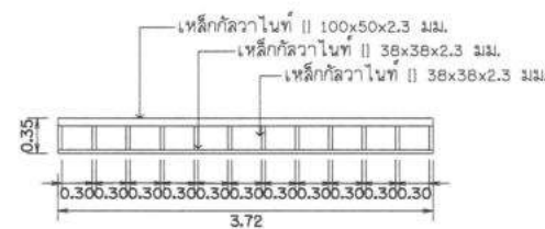
แบบขยาย T6 มาตราส่วน 1 : 100
