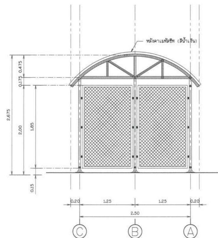
รูปด้าน 2 โมเดลตามตราตัว
