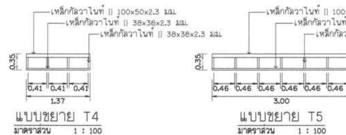
แบบขยายแพลอยสะพานช่วงที่ 2 มาตราส่วน 1 : 100
