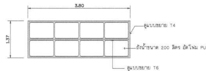
แบบขยายแพลอยสะพานช่วงที่ 1 มาตราส่วน 1 : 100
