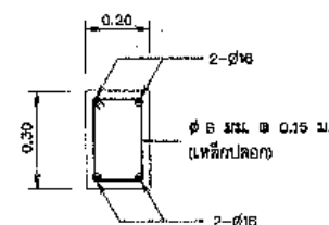
รูปตัด ก-ก ไม่แสดงขนาดรวม
