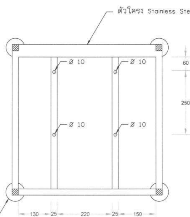
แท่นวางปั้มน้ำ
