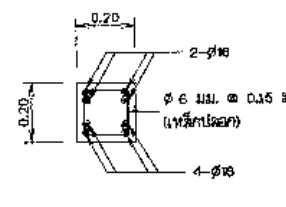
รูปตัด ข-ข ไม่แสดงขนาดรวม
