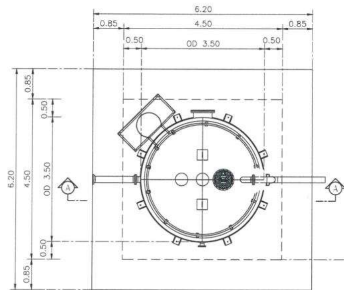
FOOTING PLAN มาตราส่วน 1 : 75
