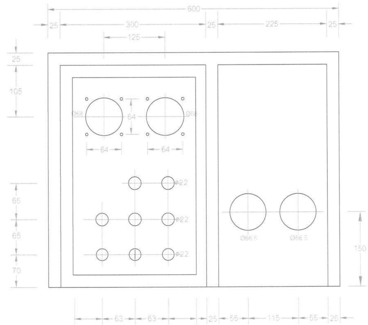
ด้านหน้า แสดงการเจาะรูเพื่อติดตั้งอุปกรณ์
