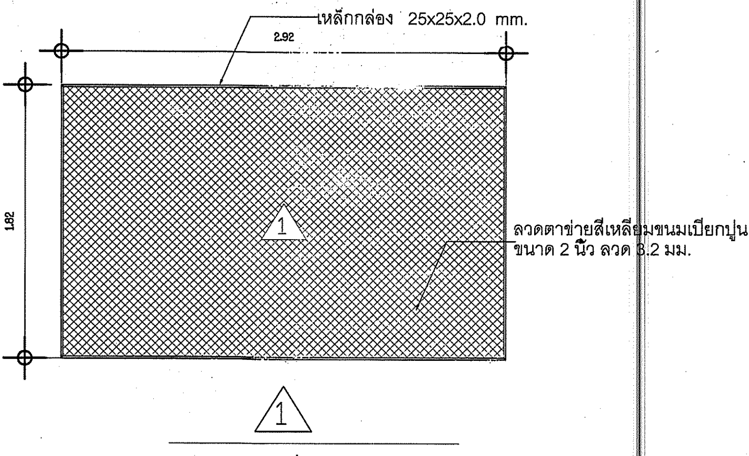
ขยาย Plate ยึดเสา มาตราส่วน 1:25
