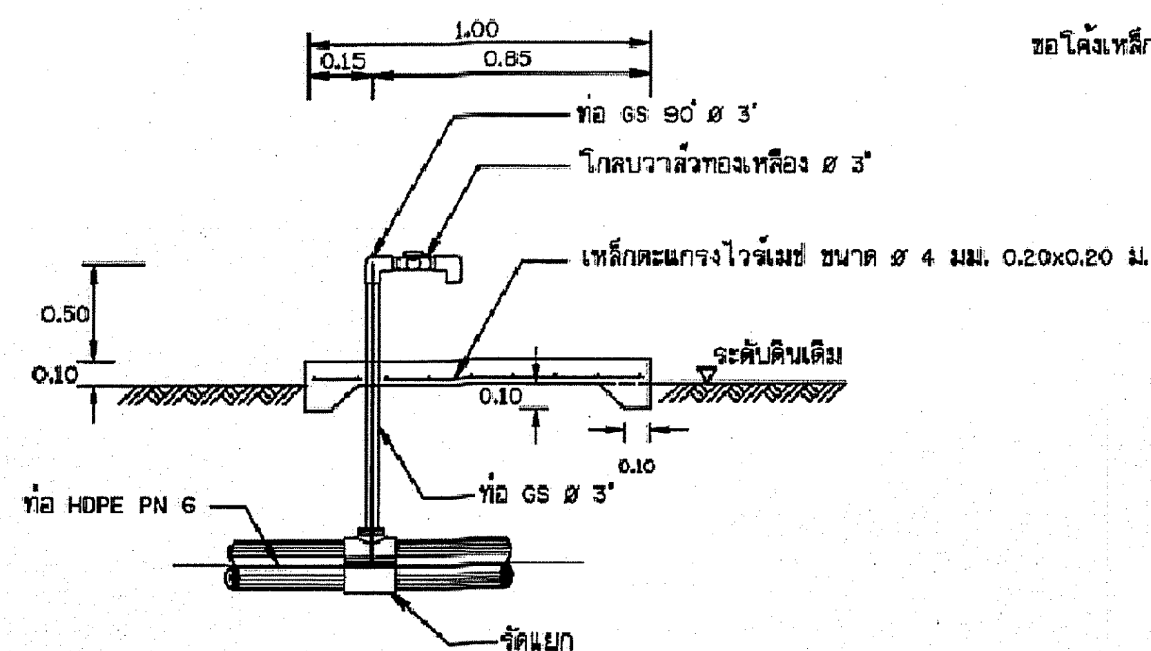
รูปตัด ก - ก มาตราส่วน No. ๕๐๐๐
