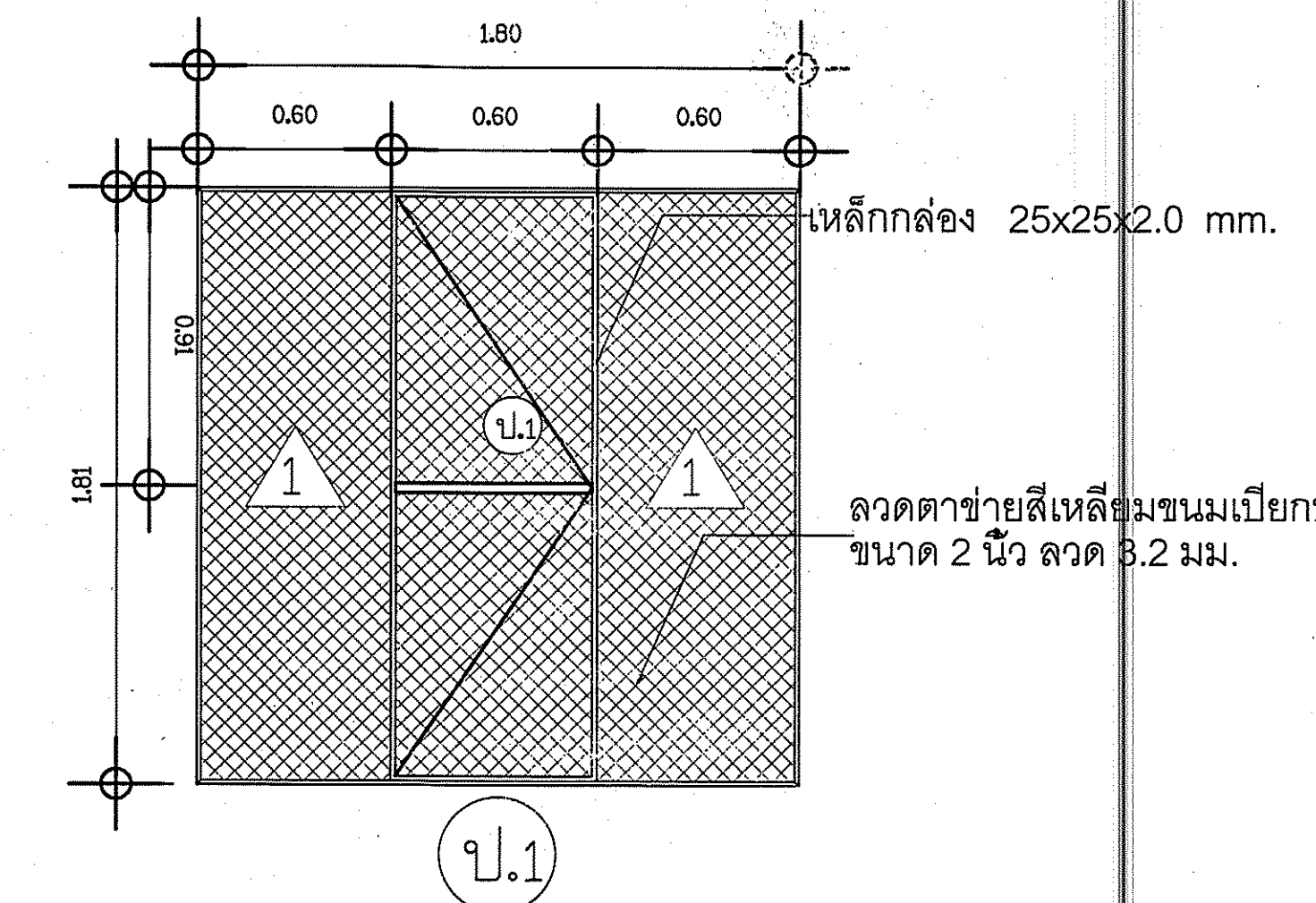
ขยาย Plate ยึดเสา มาตราส่วน 1:20
