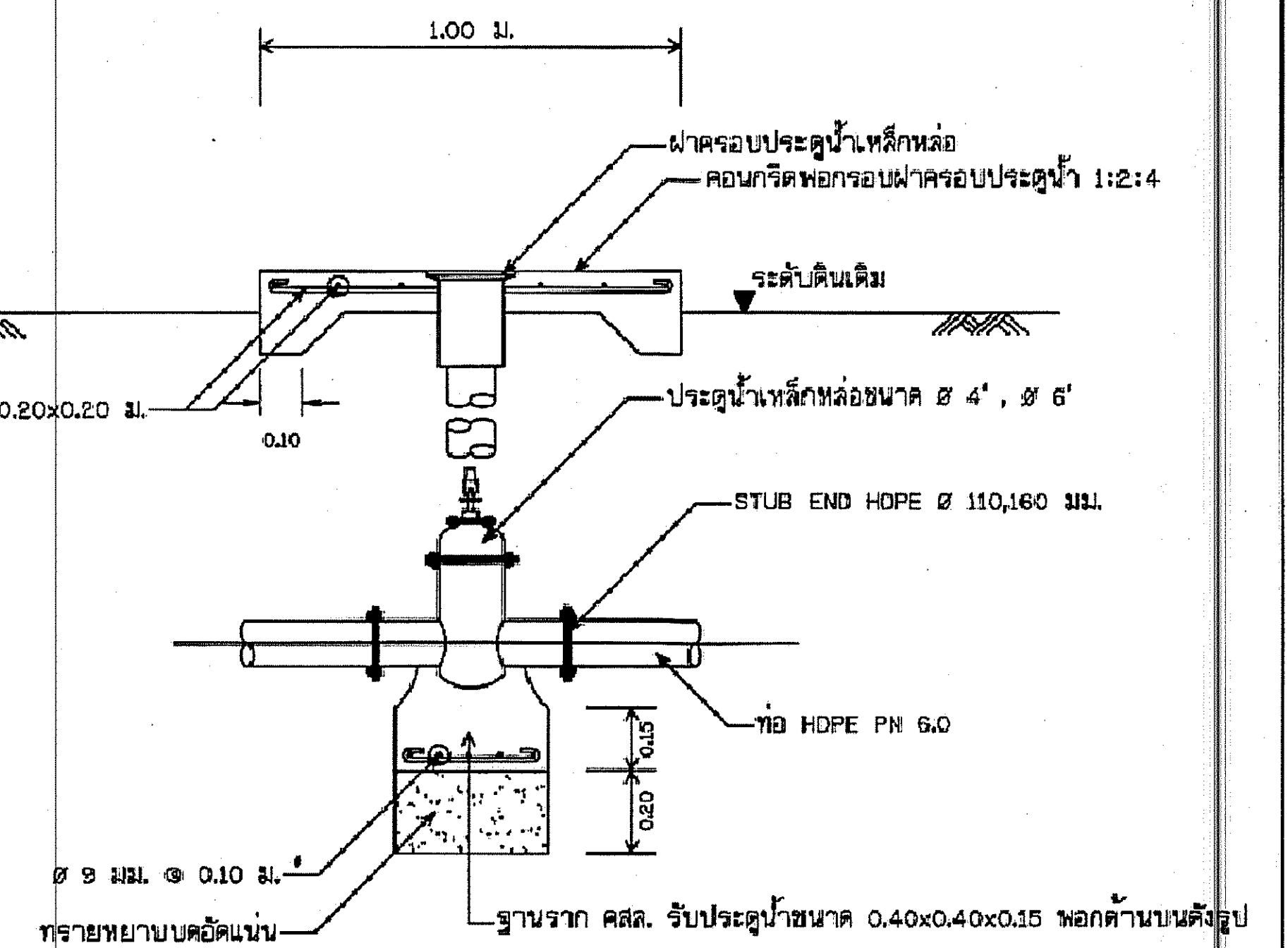
รูปตัด ค - ค แสดงการติดตั้งประตูกำแพงใต้ดิน
