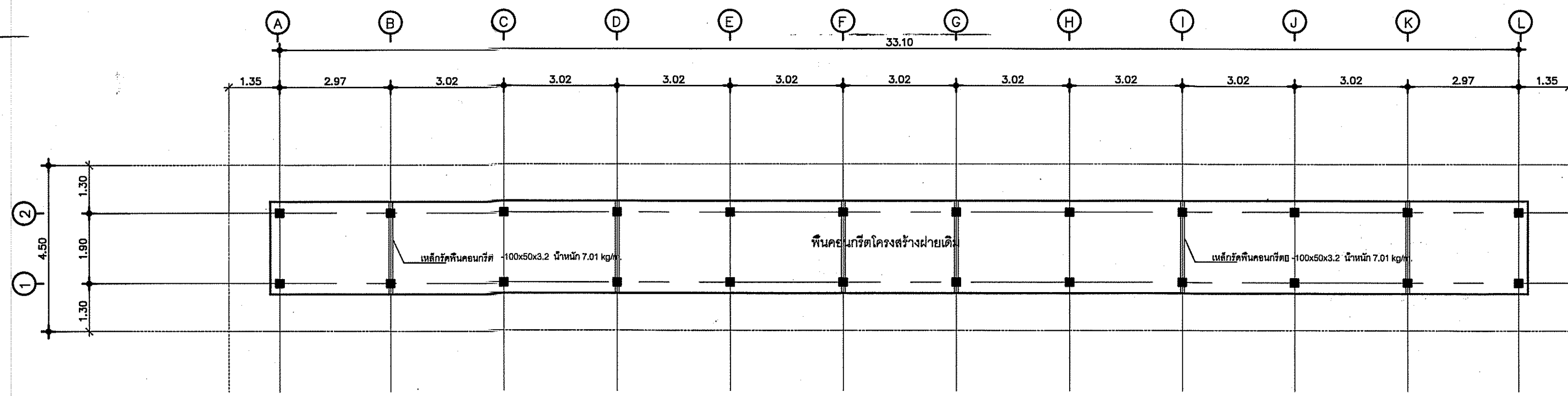
แปลนเสา
