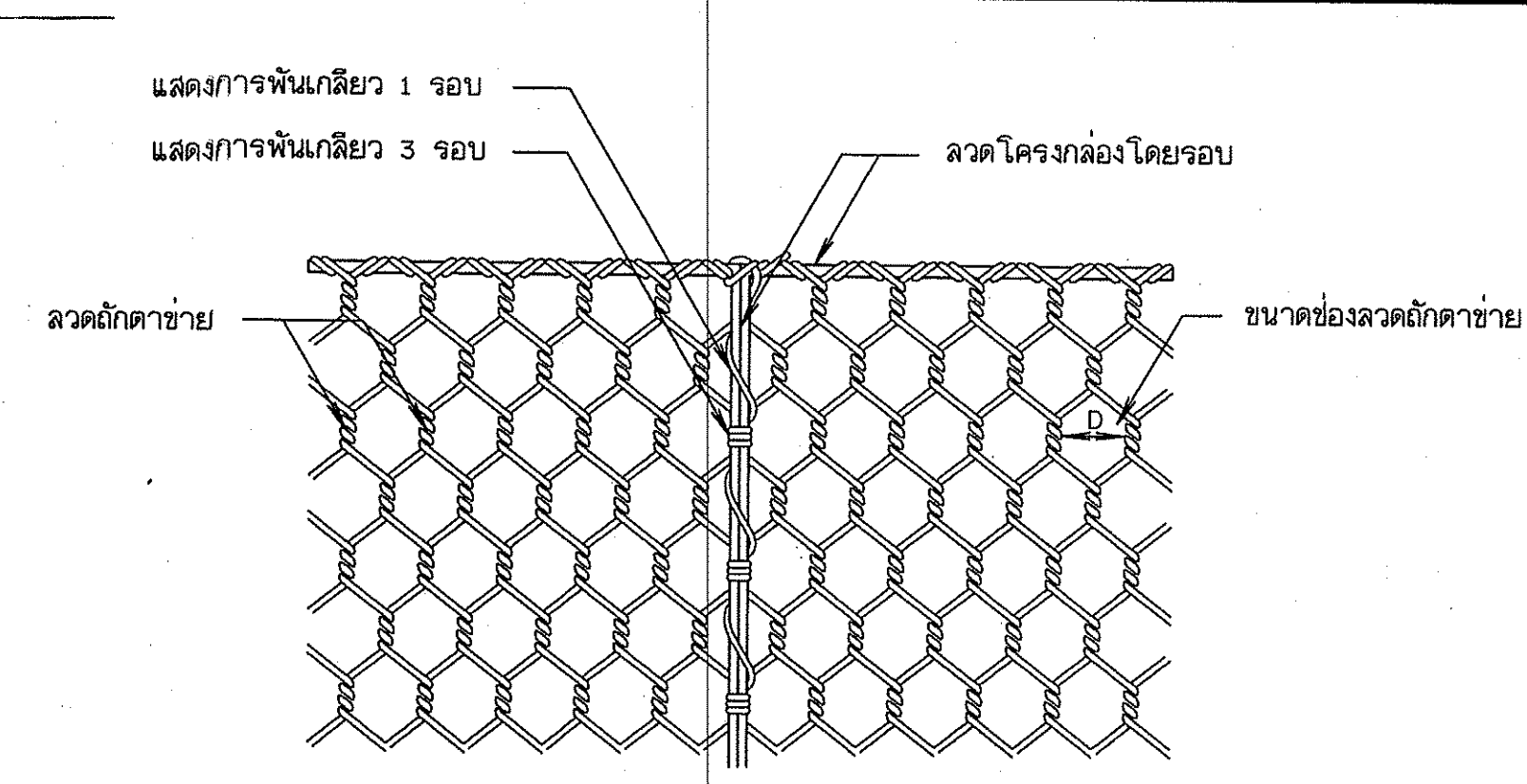
รูปแสดงการพันลวดระหว่างกล่องลวดตาข่ายและฟาบิด
