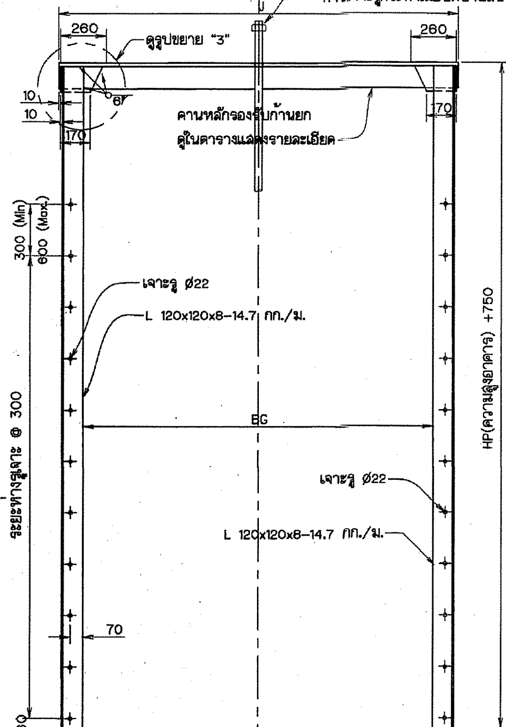
กรอบบาน เหล็กเหนียว ไม่แสดงมาตรฐาน
