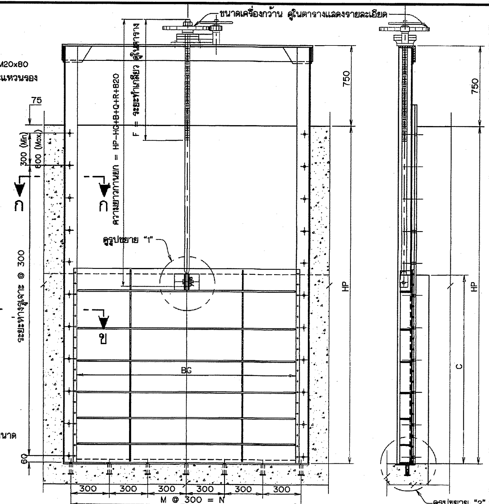
รูปแสดงการติดตั้งเครื่องกว้น และการประกอบบาน
