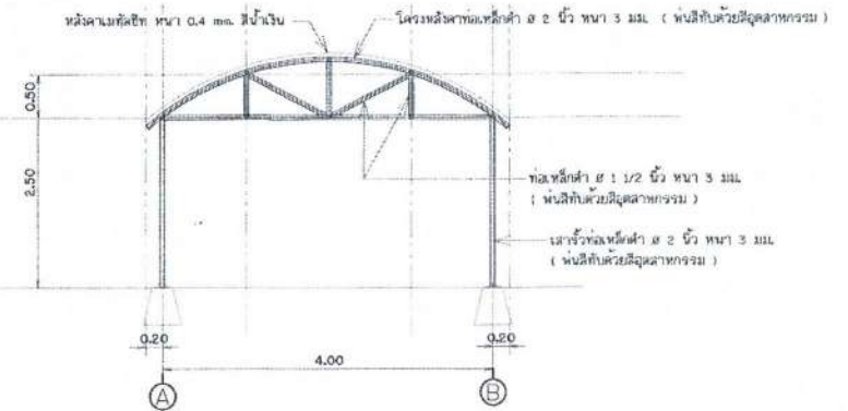
รูปตัด โครงหลังคาคลุม โมเดลขนาดจริง
