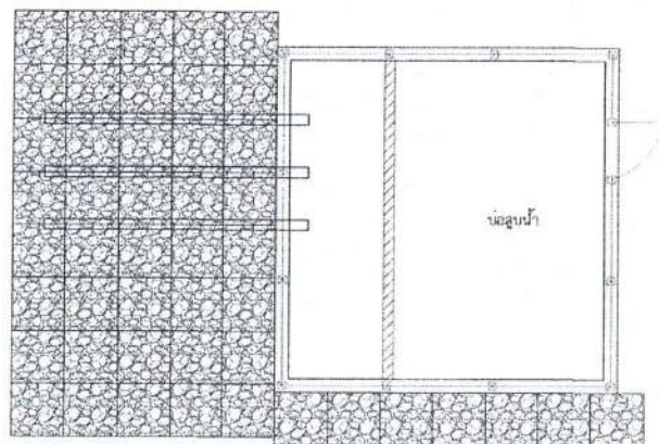
แปลนระบบสูบน้ำ ขนาด 18.5 KW.
