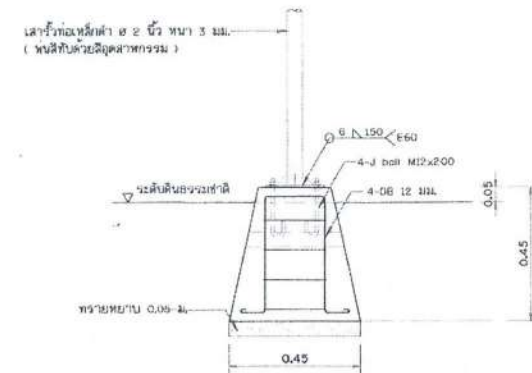
รูปขยายฐานราก โครงหลังคาคลุม (ด้านข้าง) โมเดลขนาดจริง
