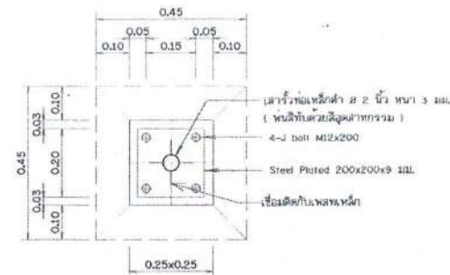
รูปขยายฐานราก โครงหลังคาคลุม โมเดลขนาดจริง
