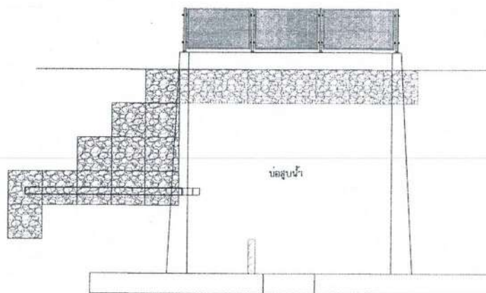
รูปด้านข้างระบบสูบน้ำ ขนาด 18.5 KW.
