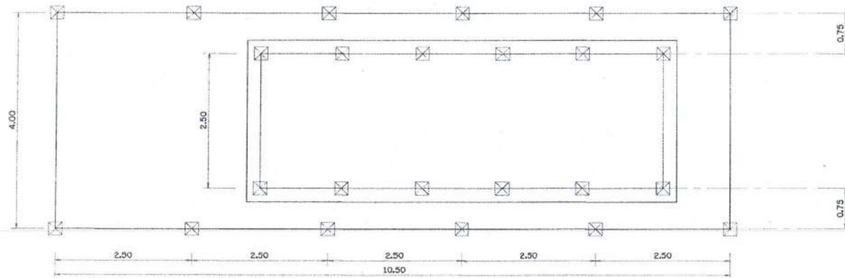
แบบแปลน โครงหลังคาคลุม โมเดลขนาดจริง
