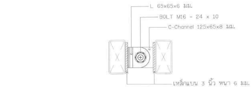
แบบขยายตัวเชื่อม มาตราส่วน 1 : 100
