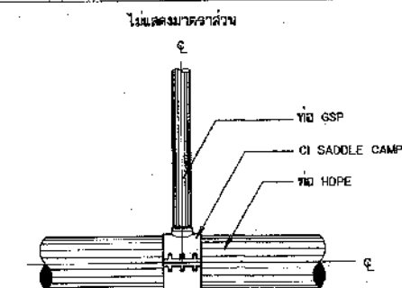
การบรรจุท่อสามทาง HDPE กับท่อ GSP แบบ CI SADDLE CLAMP (สำหรับอาคารจุดปล่อยน้ำ อาคารประจวบประจวบตอน อาคารท่อระบายอากาศ กรณีที่ท่อส่งน้ำขนาดเส้นผ่านศูนย์กลางน้อยกว่าหรือเท่ากับ 315 มม.)
