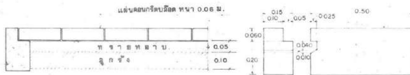
ขยายบันไดคอนกรีต 1810
