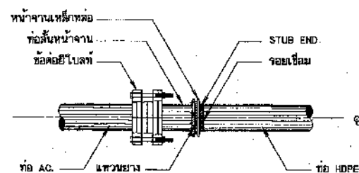
การบรรจุท่อ AC. กับท่อ HDPE ไม่แสดงขนาดราส่วน
