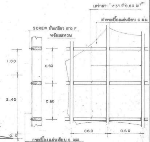
รูปขยายเคร่า, ๗๑ | ๘ 20
