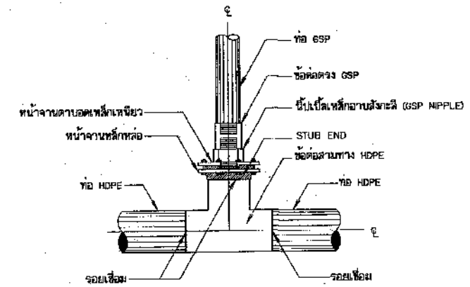
การบรรจุท่อสามทาง HDPE กับท่อ GSP แบบข้อต่อ (สำหรับอาคารจุดปล่อยน้ำ อาคารประจวบประจวบตอน อาคารท่อระบายอากาศ กรณีที่ท่อส่งน้ำขนาดเส้นผ่านศูนย์กลางมากกว่า 315 มม.)
