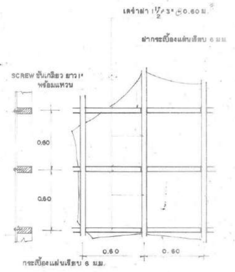
รูปขยายโครงเสา, ฝา 18 20
