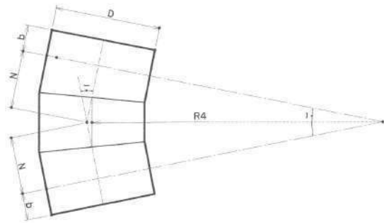
ข้อโค้ง 3 ชั้น (22.5° < 0 < 45°)
