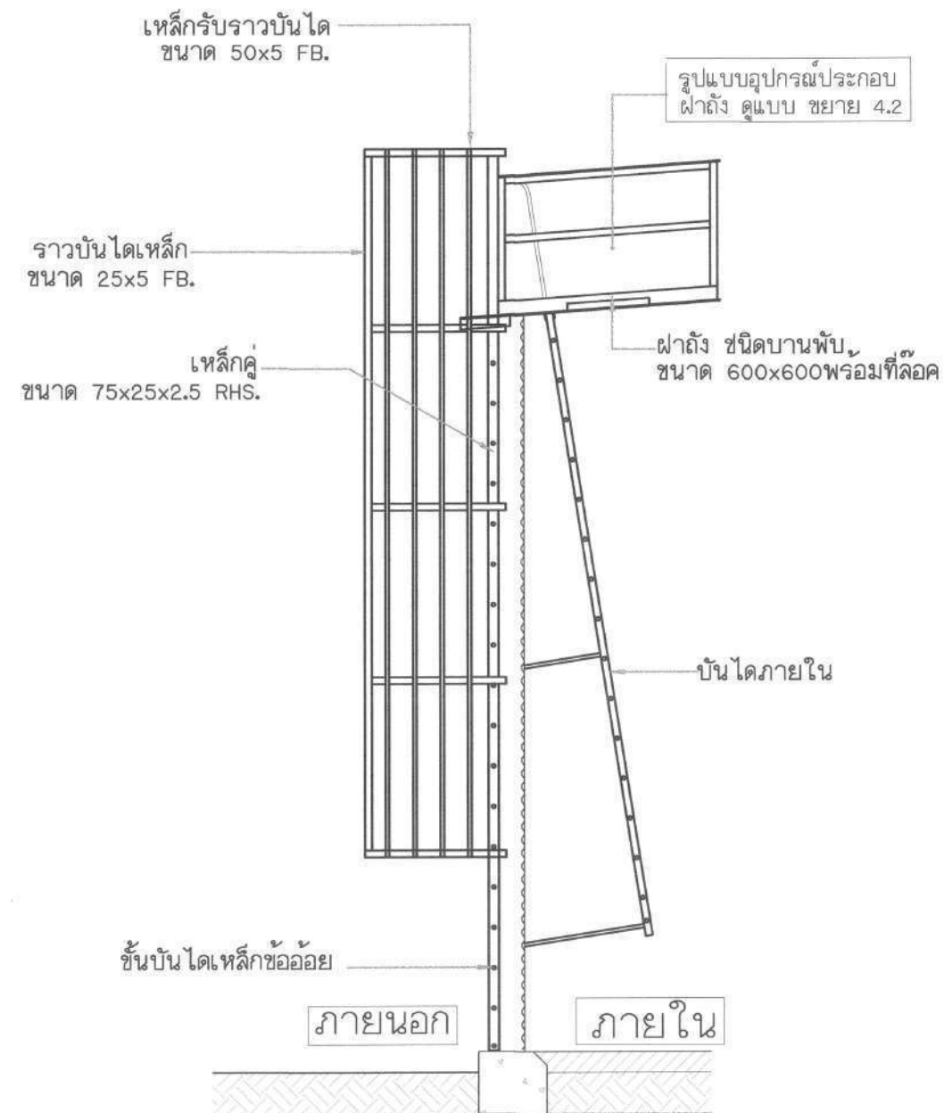
แบบขยาย 4.1 - บันไดทางเข้าถึง 6.4 m. มาตราส่วน 1 : 50
