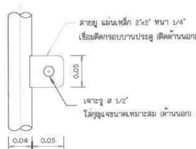
แบบขยายสายโยง ไม่แสดงขนาดราวล้วน
