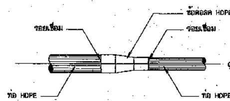
การบรรจุท่อ HDPE กับข้อต่อท่อ HDPE ไม่แสดงมาตรฐาน
