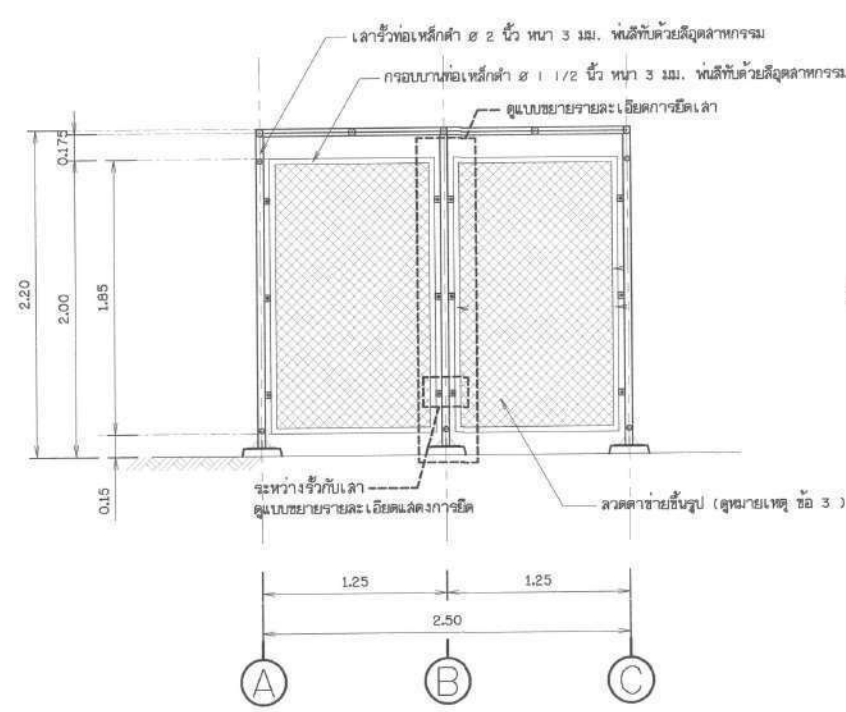
แบบขยายรั้ว 2 ไม่แสดงขนาดราวล้วน
