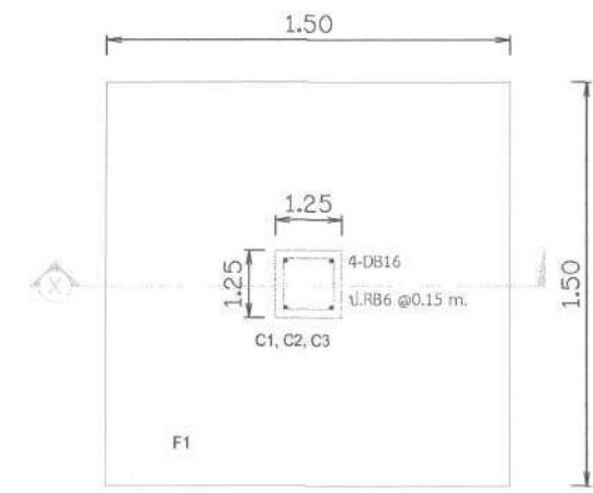
FOOTING F1 SCALE (A3) 1:30
