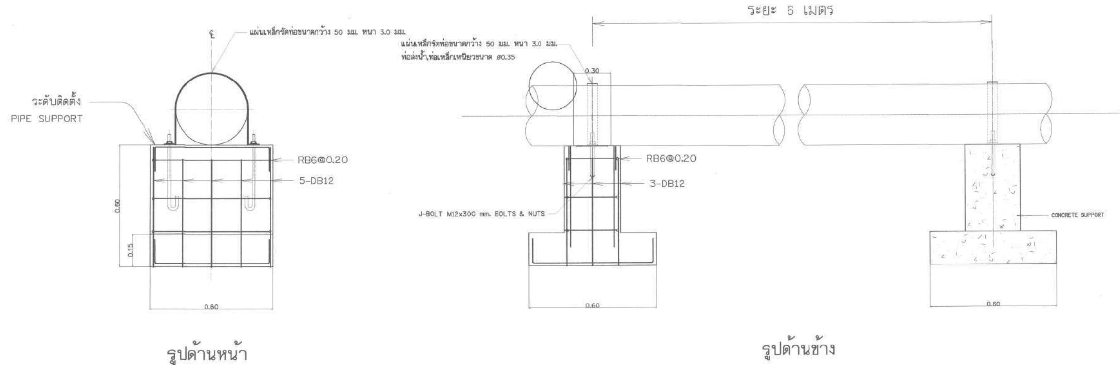
ดอมม่อรับท่อ Ø350 มม. มาตราส่วน
