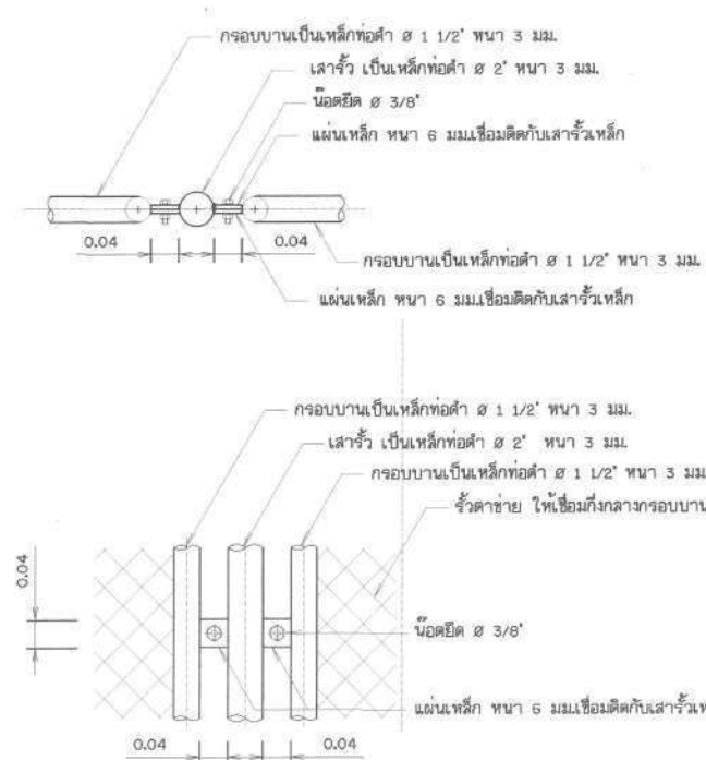
แบบขยายรายละเอียดแสดงการยึดระหว่างรั้วกับเสา ไม่แสดงขนาดราวล้วน
