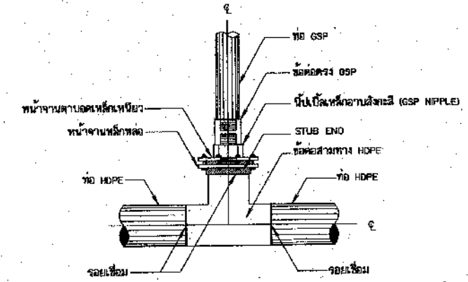
การบรรจุท่อสามทาง HDPE กับท่อ GSP แบบข้อต่อ สำหรับอาคารชลประทาน อาคารประสูตระบายตะกอน อาคารท่อระบายอากาศ กรณีท่อส่งน้ำขนาดเส้นผ่านศูนย์กลางน้อยกว่า 315 มม.
