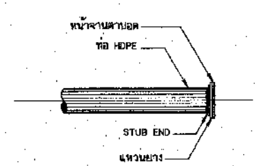
การปิดปลายท่อ ไม่แสดงมาตรฐาน
