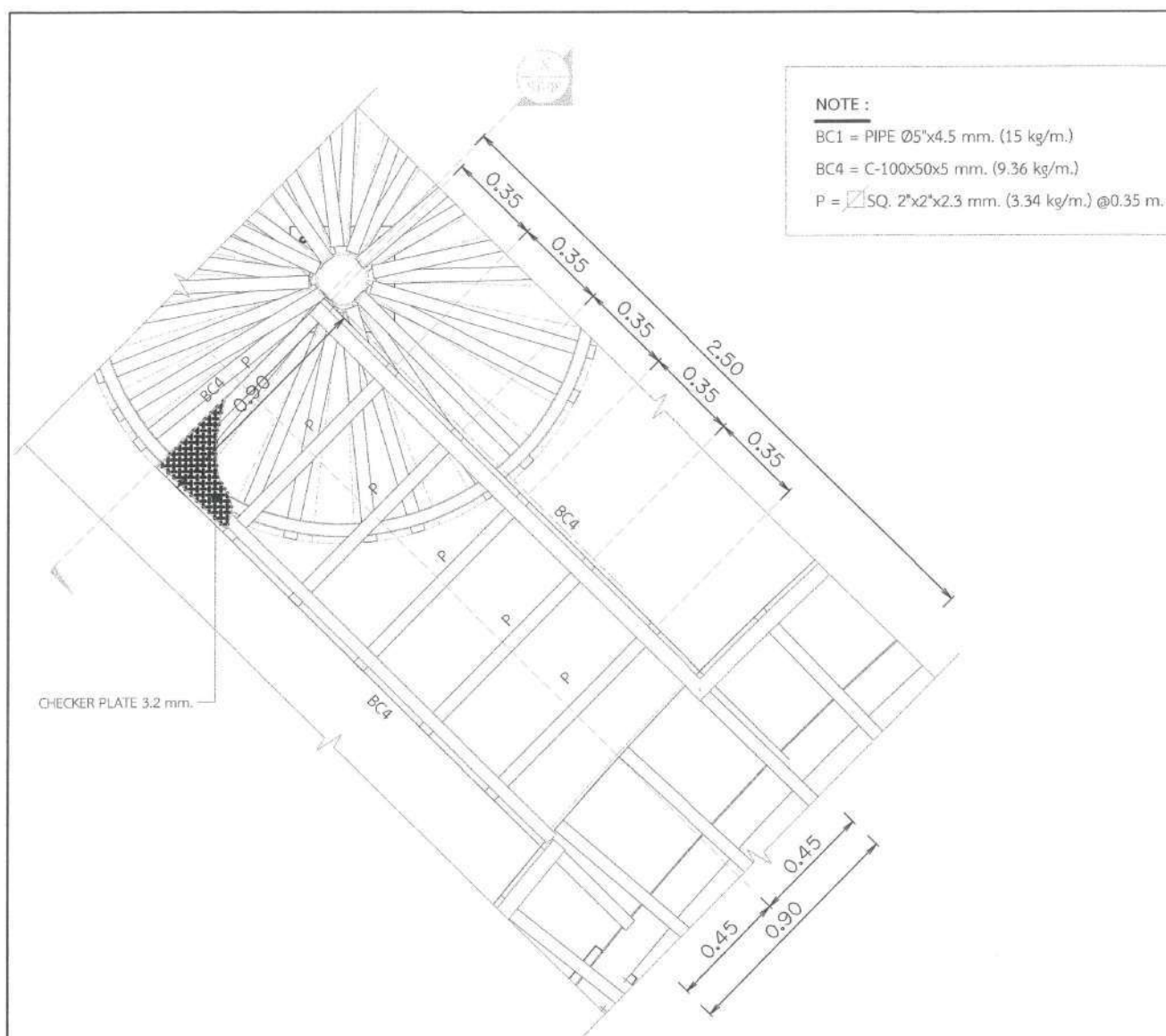
DETAIL : A SCALE (A3) 1 : 25
