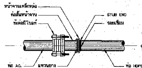
การบรรจุท่อ AC กับท่อ HDPE ไม่แสดงมาตรฐาน
