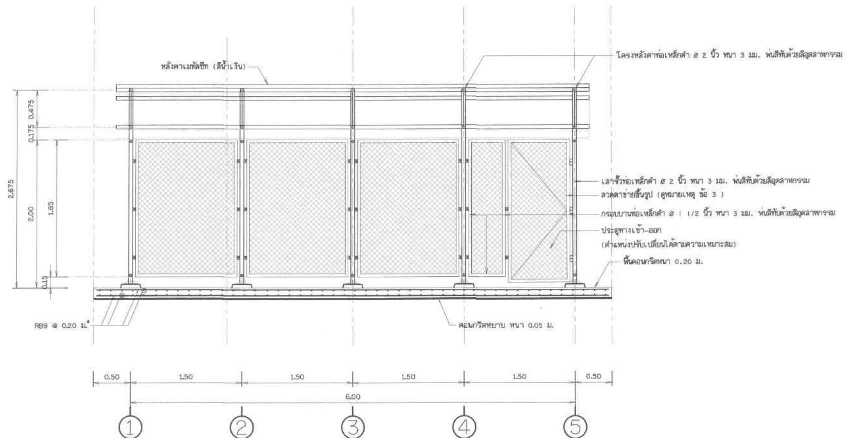
รูปตัด ก - ก
