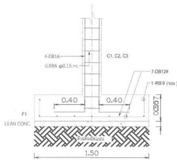
SECTION X-X : F1 SCALE (A3) 1:30
