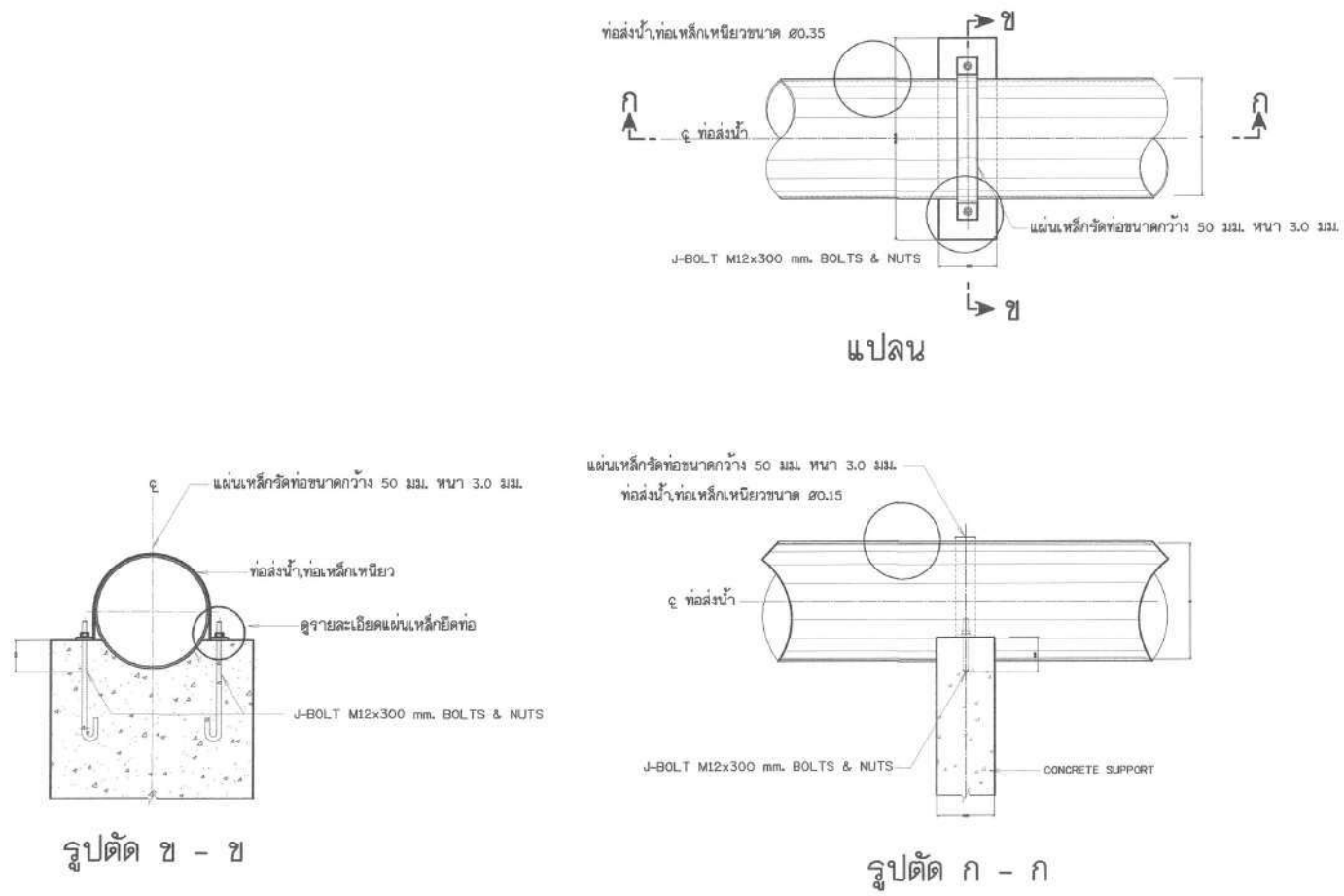
รายละเอียดการยึดท่อ ไม่แสดงมาตราส่วน
