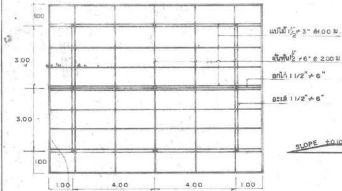
แปลนโครงหลังคา 18100
