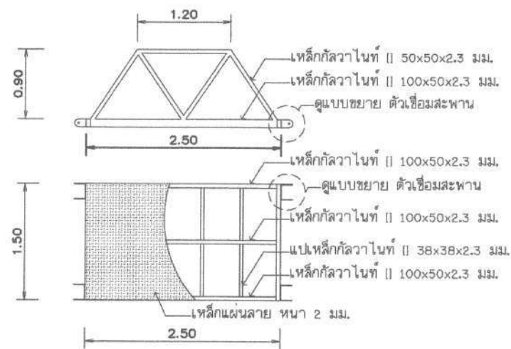
แบบขยายสละพานช่วงที่ 1,3,5
