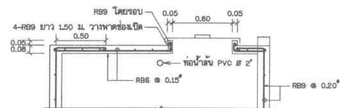
แสดงการเสริมเหล็กฝาลัง มาตราส่วน 1:20
