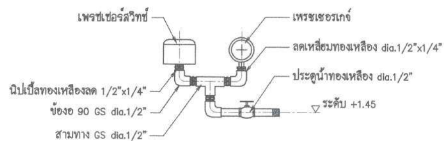
แบบขยายสวิตช์ควบคุมและเกจ์ความดัน ไม่แสดงมาตราส่วน
