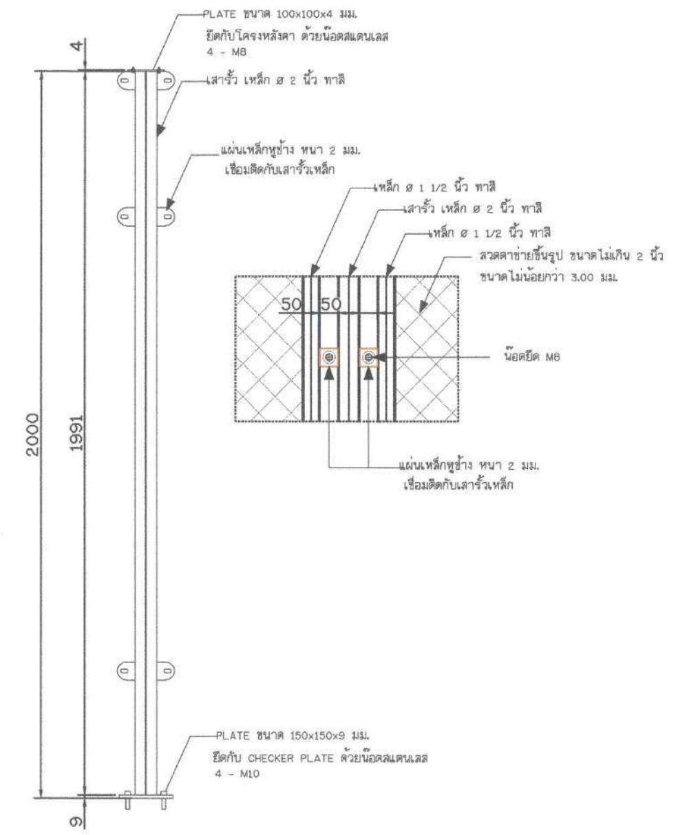
แบบขยายรายละเอียดแสดงการยึดรั้ว
