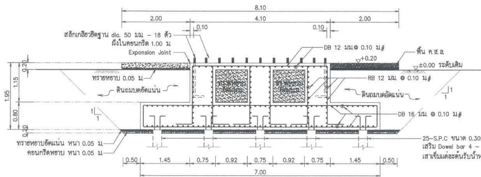
รูปตัด ก-ก
