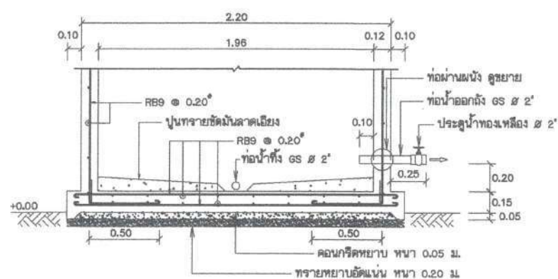
แสดงการเสริมเหล็กพื้นถัง มาตราส่วน 1:20
