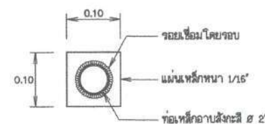
ขยายท่อผ่านผนัง มาตราส่วน 1:5
