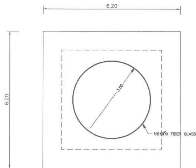
แปลนฐานรากแผ่ มาตราส่วน 1:100
