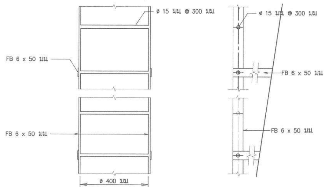
ภาพขยายบันได "1" ภายในห้องถึงเหล็กเก็บน้ำ
