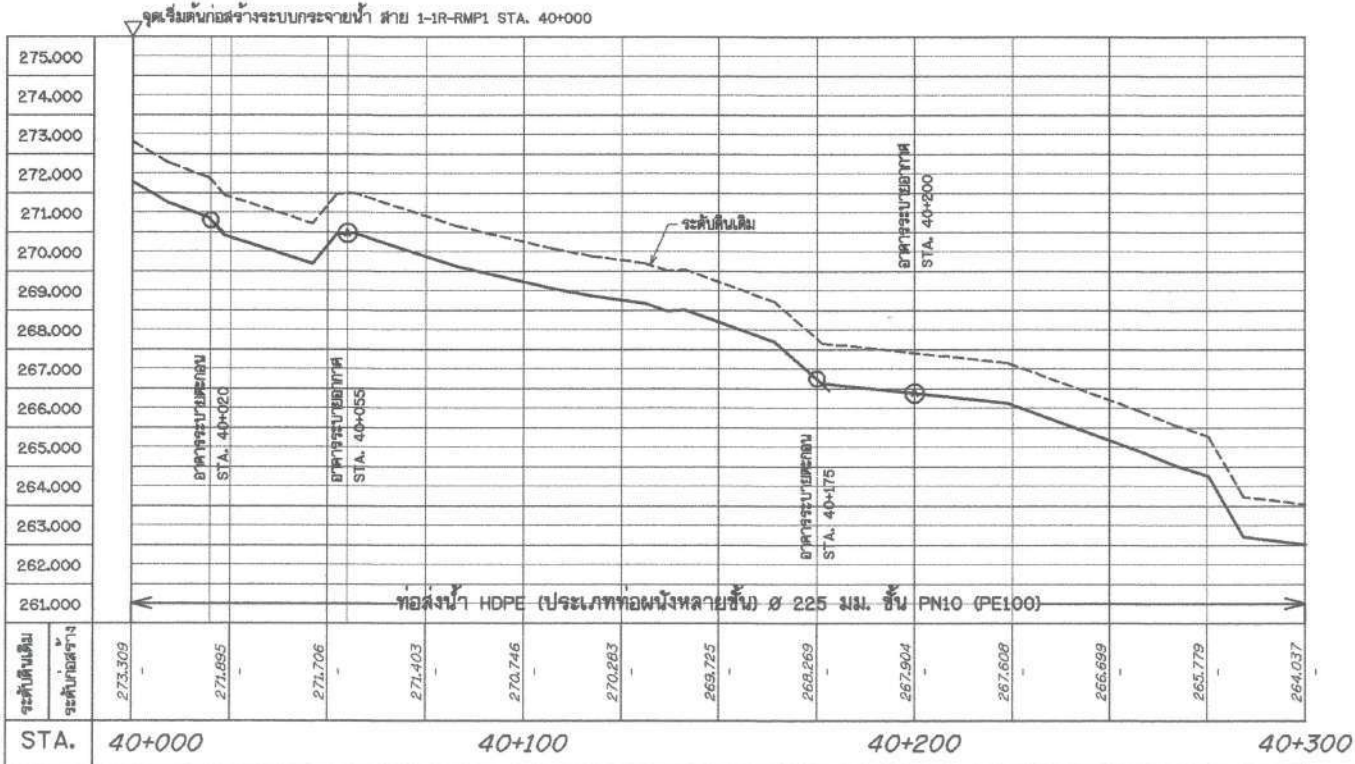
รูปตัดตามแนวยาวระบบกระจายน้ำ สาย 1-1R-RMP1 มาตราส่วน แนวนอน 1:1,000 แนวตั้ง 1:100
