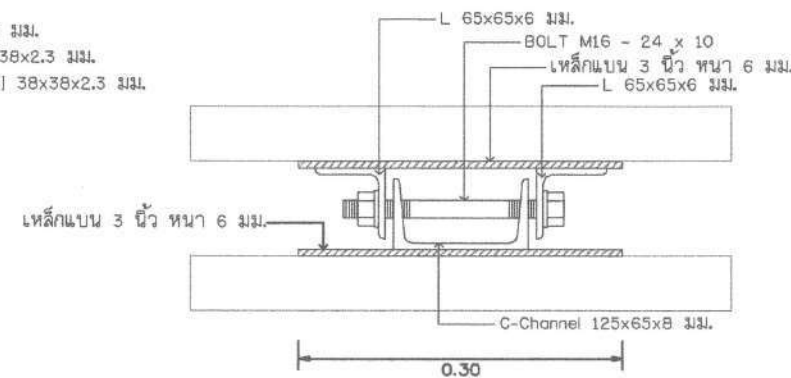
แบบขยายตัวเชื่อม
