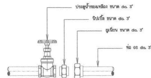
แบบขยายการประสานท่อระหว่างถัง มาตราส่วน 1:20
