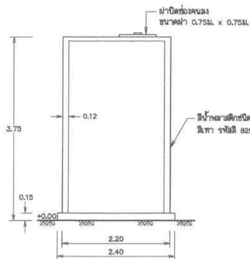
ด้านข้าง มาตราส่วน 1:40
