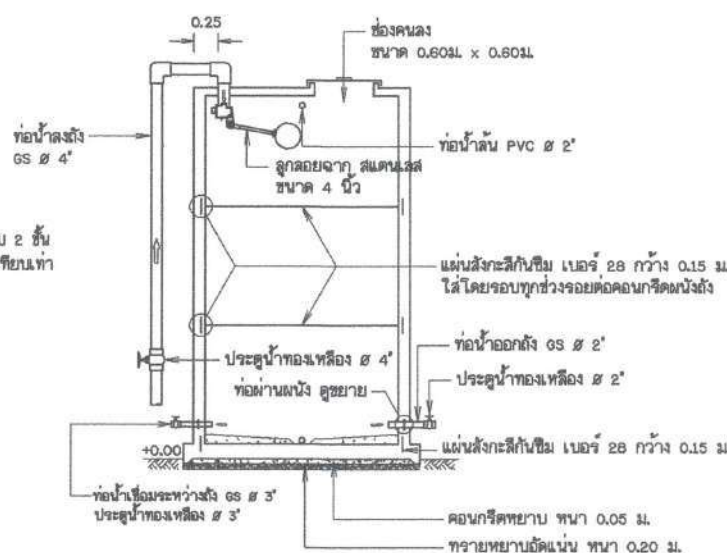
รูปตัด (1) มาตราส่วน 1:40
