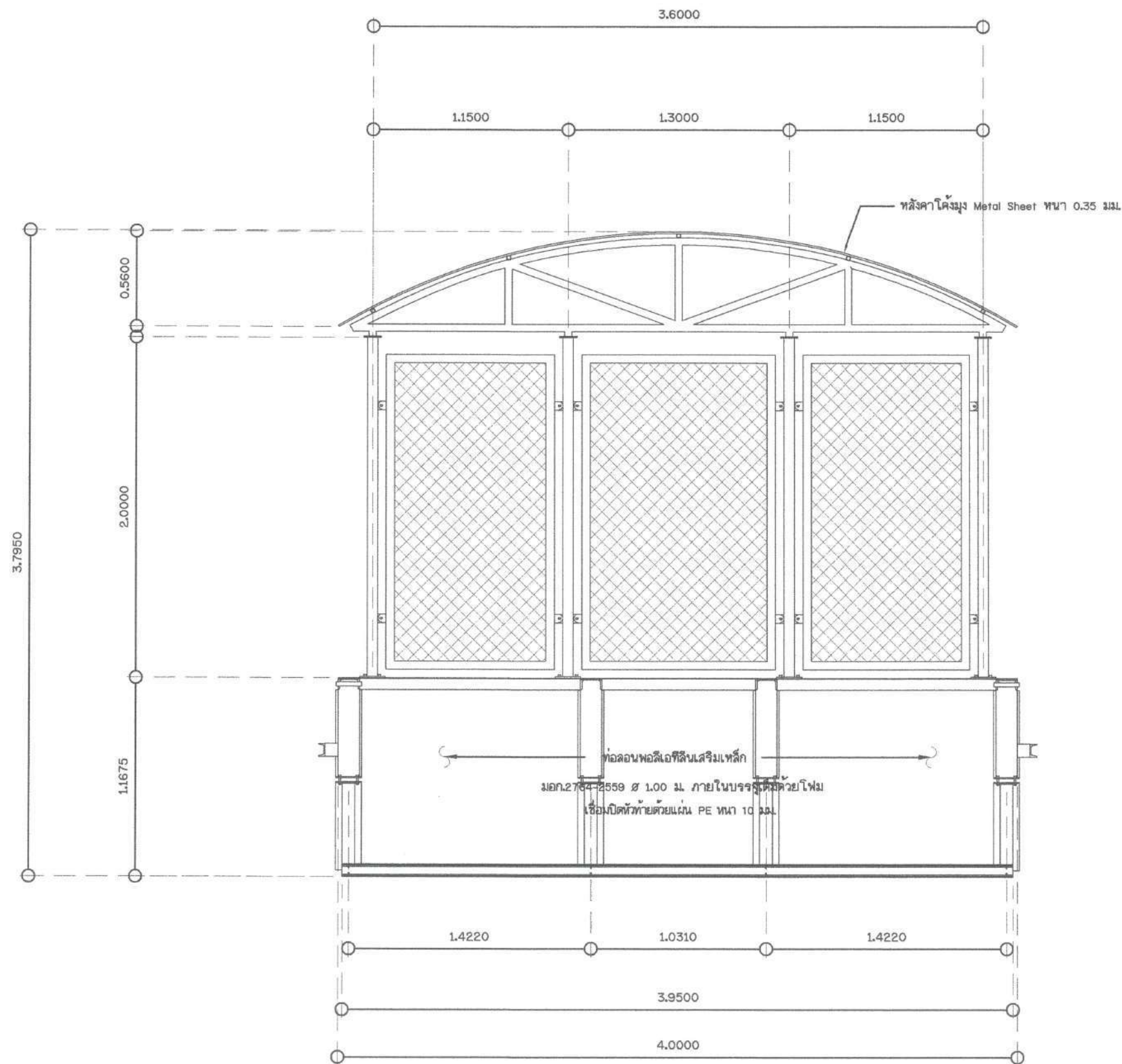
รูปด้าน ② SCALE 1:30
