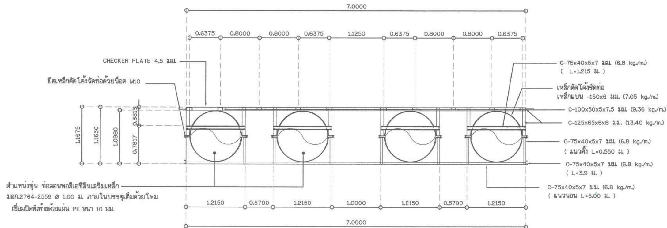
รูปตัด ข - ข SCALE 1:50
