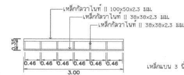
แบบขยาย T4
