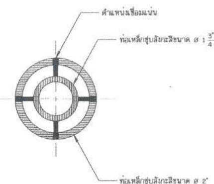
รูปตัด ข-ข
