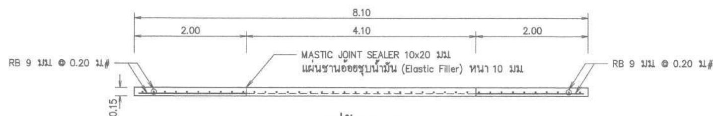
รูปตัด ข-ข
