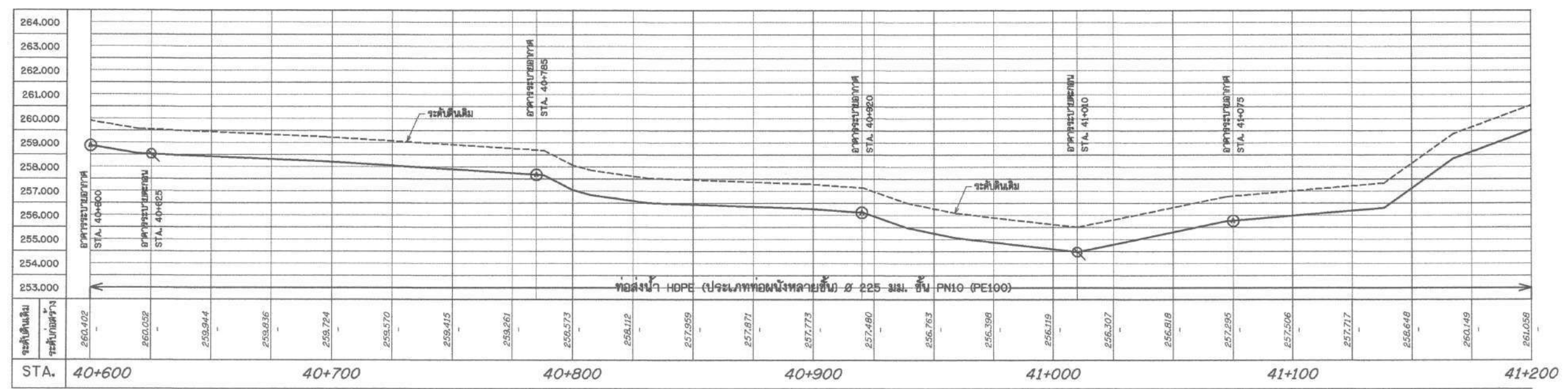
รูปตัดตามแนวยาวระบบกระจายน้ำ สาย 1-1R-RMP1 มาตราส่วน 1:1,000 แนวตั้ง 1:100
