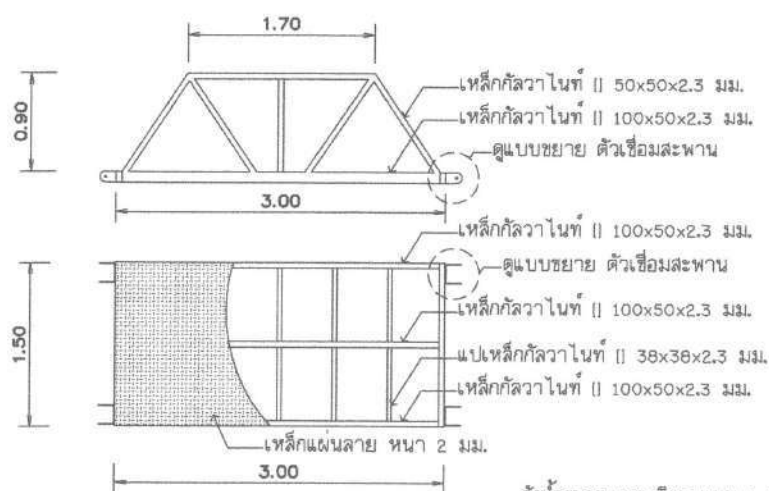
แบบขยายสละพานช่วงที่ 2,4
