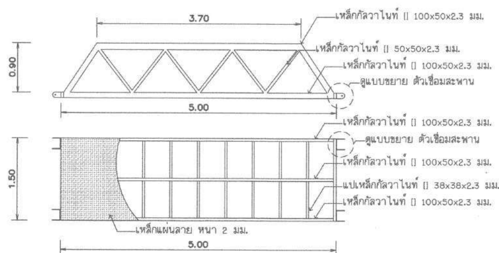
แบบขยายสละพานช่วงที่ 6
