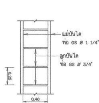
ขยายบันได มาตราส่วน 1:20
