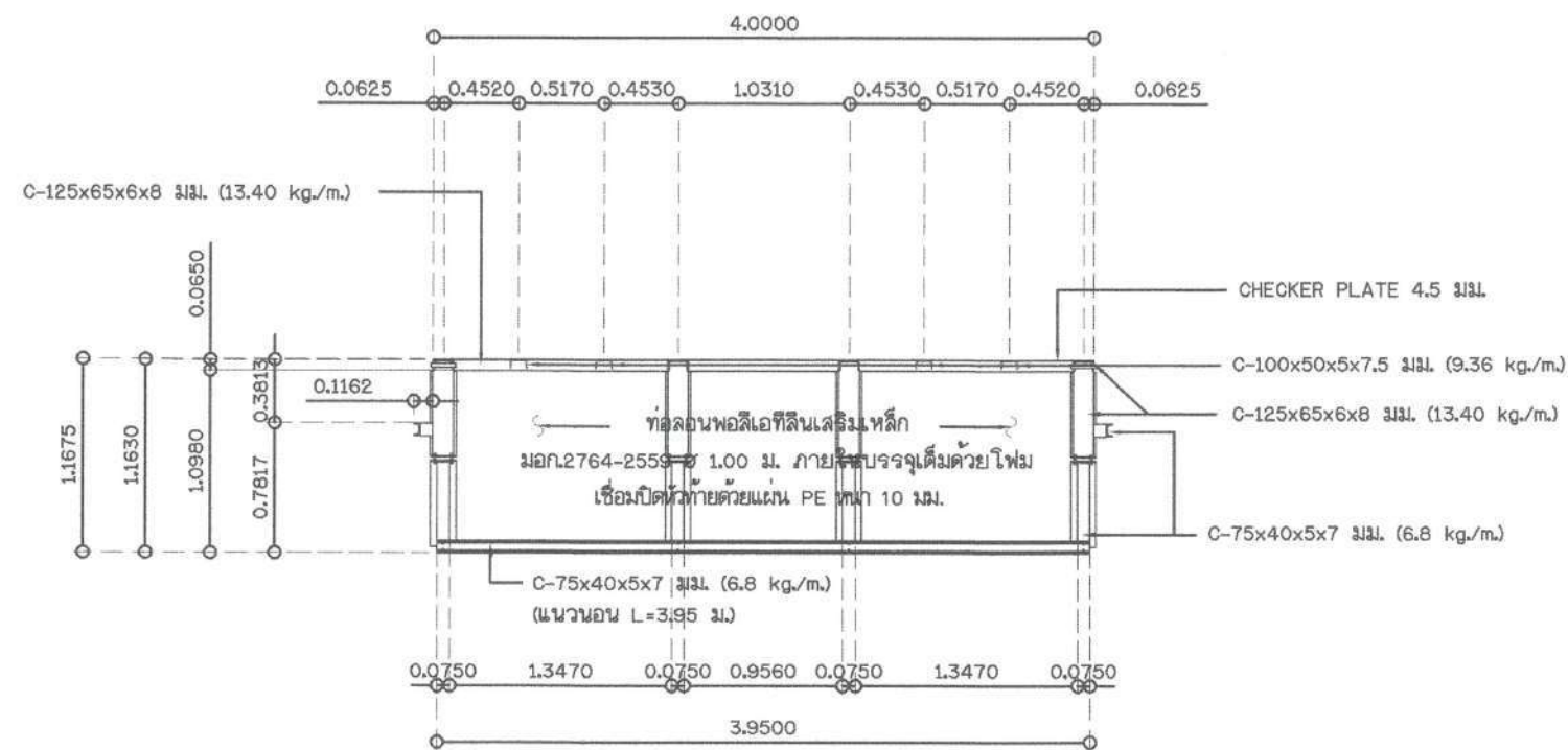
รูปตัด ก - ก SCALE 1:50
