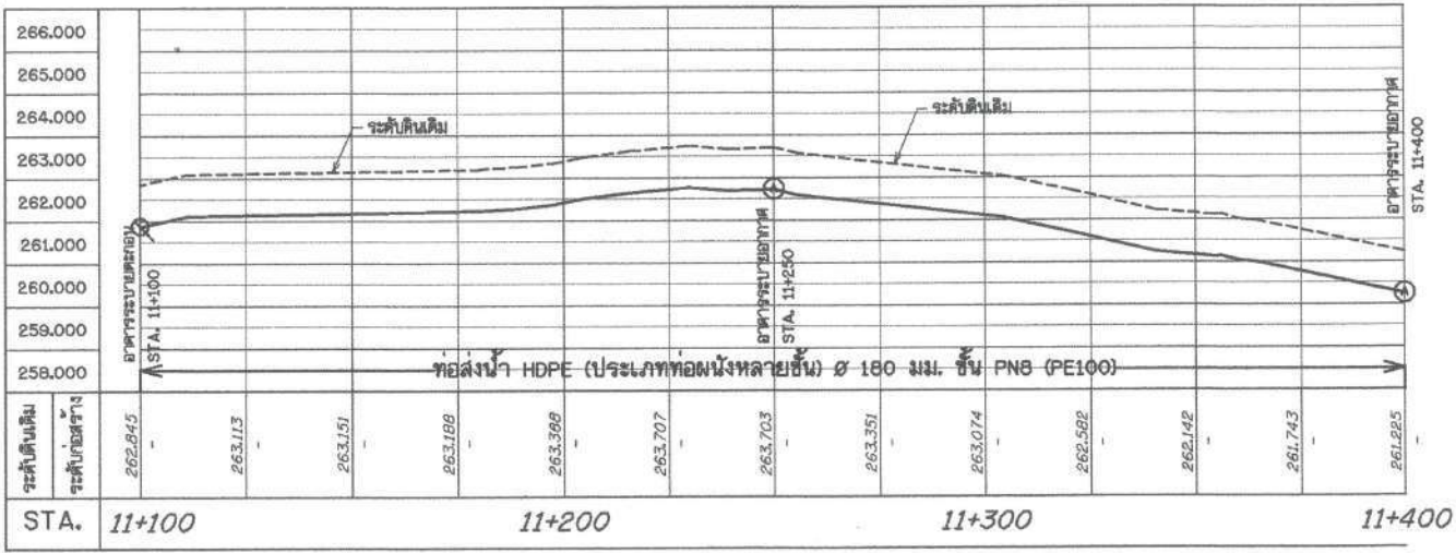
รูปตัดตามแนวยาวระบบกระจายน้ำ สาย RMP1 มาตรฐาน 1:1,000 แนวตั้ง 1:100
