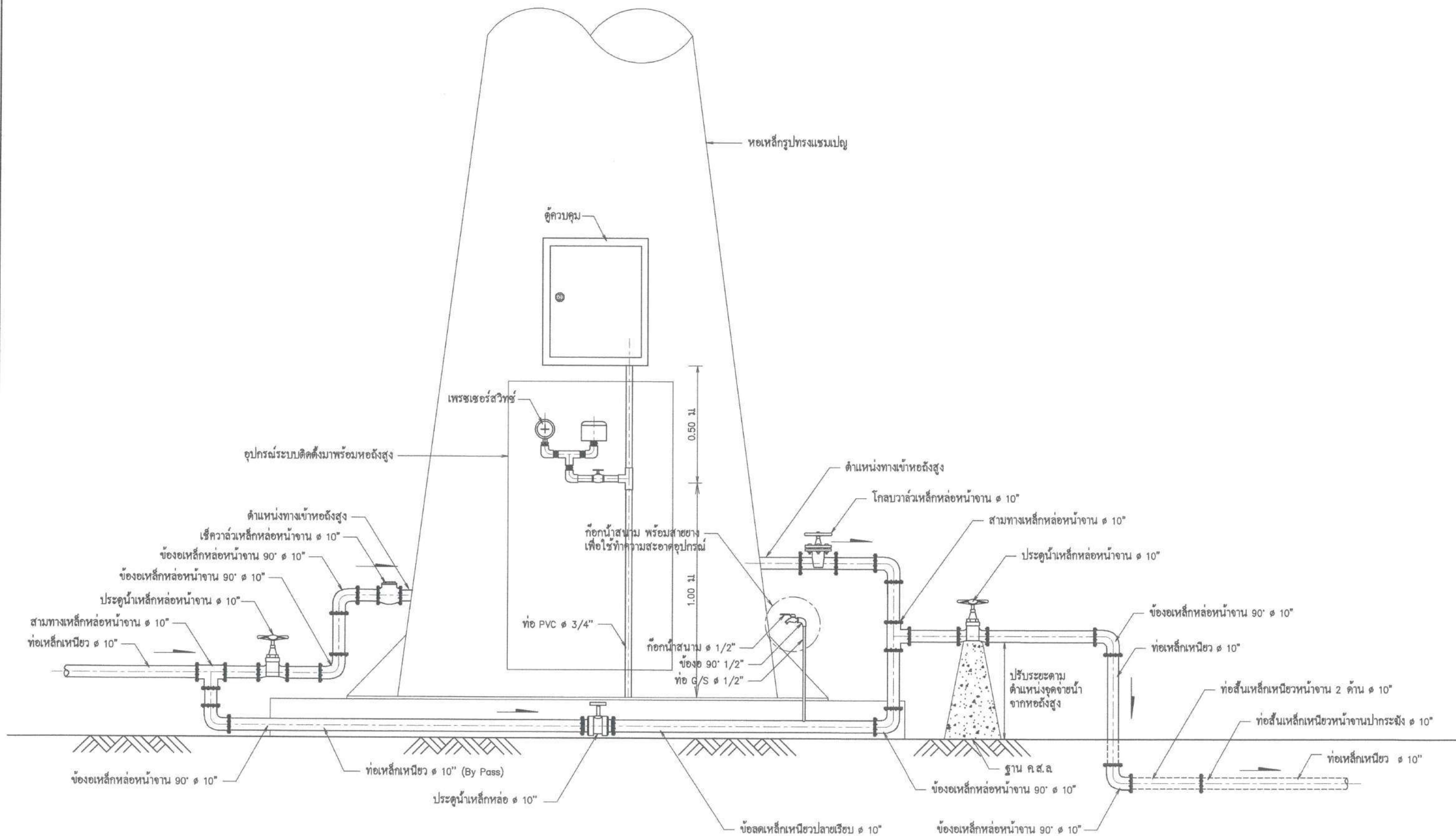
รูปแสดงรายละเอียดการต่อท่อและอุปกรณ์ออกจากถังเหล็กรูปทรงแรมแปญ ไม่แสดงมาตราส่วน
