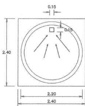
แสดงมิติบ่อรวมตะกอน มาตราส่วน 1:40
