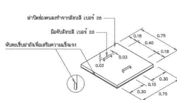
ขยายฝาปิดช่องคนลง มาตราส่วน not to scale
