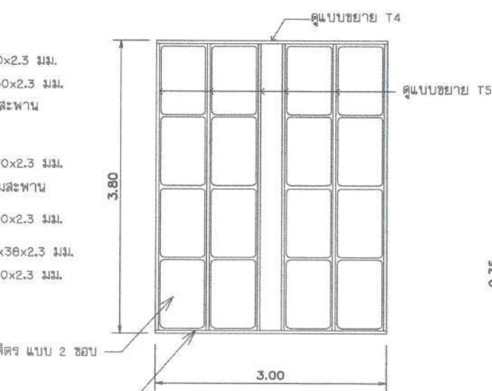
แบบขยายแพลงสละพานช่วงที่ 2,4
