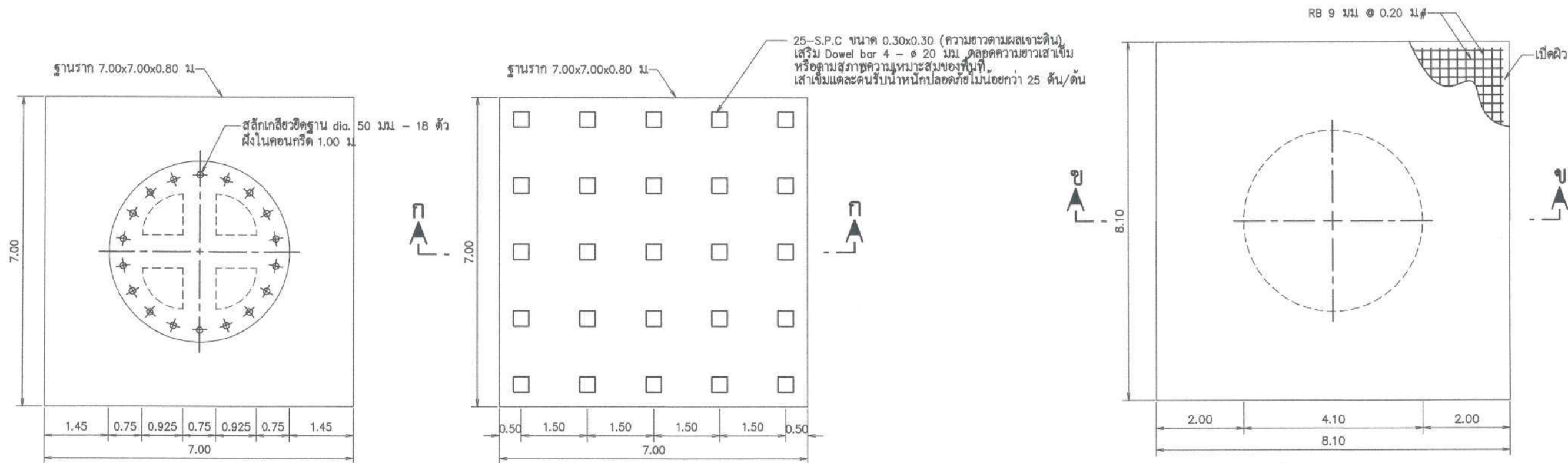
แปลนพื้นคอนกรีตเสริมเหล็ก
