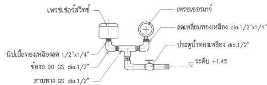
แบบขยายสวิทช์ควบคุมและเกจ์ความดัน ไม่แสดงมาตราส่วน
