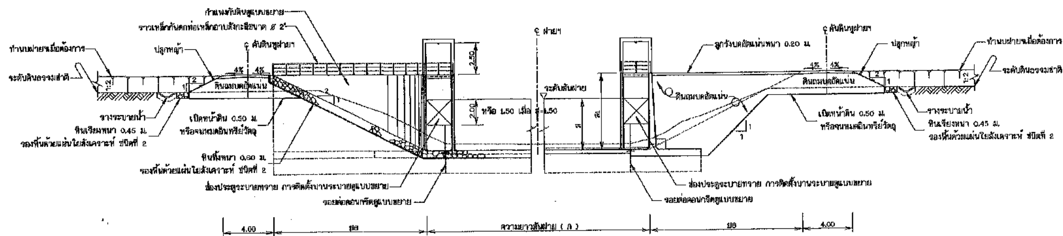
รูปตัด ข - ข
