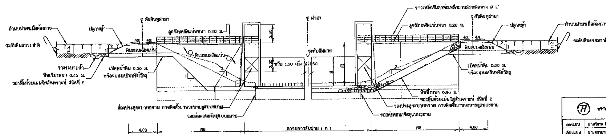
รูปตัด ค - ค
