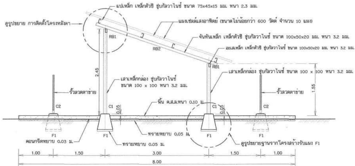
รูปด้านข้าง ไม่แสดงขนาดจริง
