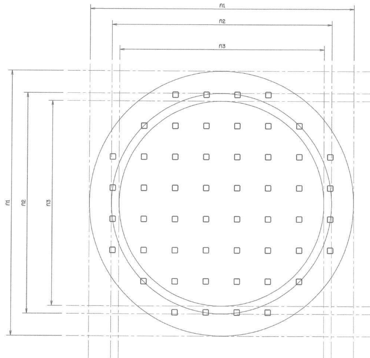
แพลนเสารั้ว ถึงเก็บน้ำ Fusion Bonded Epoxy (FBE) ขนาด 1,100 ลบ.ม. มาตราส่วน 1:100
