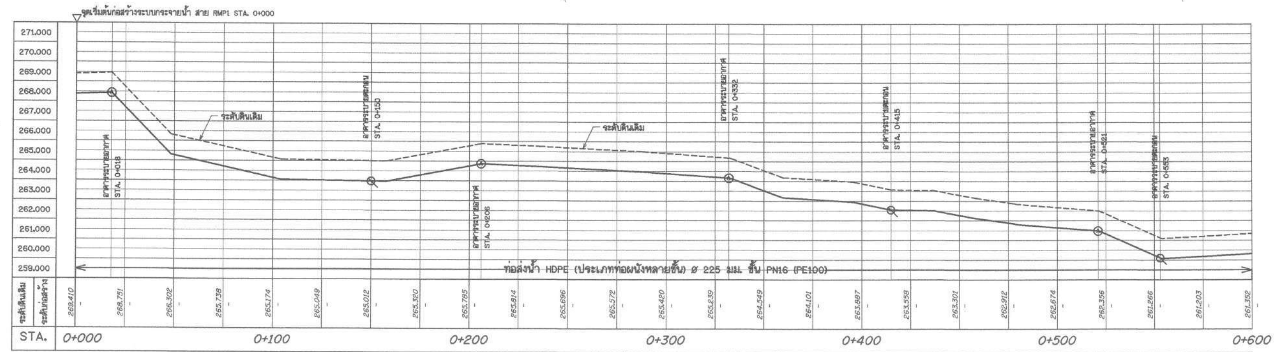
รูปตัดตามแนวยาวระบบกระจายน้ำ สาย RMP1 STA. 0+000 - 0+600 มาตรฐาน 1:1,000 แนวตั้ง 1:100
