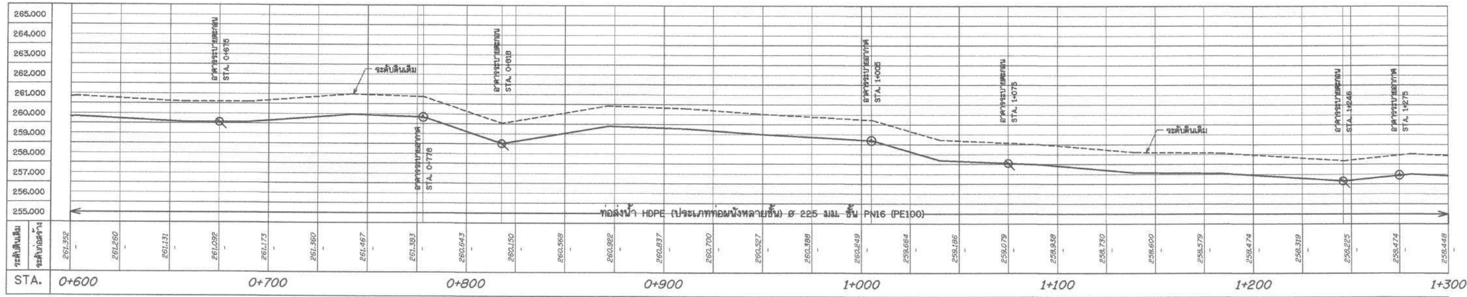
รูปตัดตามแนวยาวระบบกระจายน้ำ สาย RMP1 STA. 0+600 - 1+300 มาตราส่วน 1:1,000 แนวถนน 1:1,000 แนวราง 1:100
