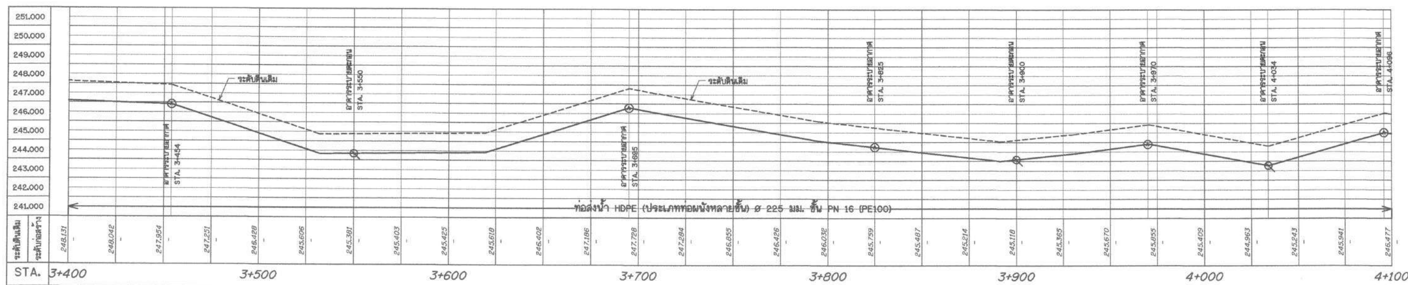
รูปตัดตามแนวยาวระบบกระจายน้ำ สาย RMP1 STA. 3+400 - 4+100 มาตราส่วน 1:1,000 แนวตั้ง 1:100
