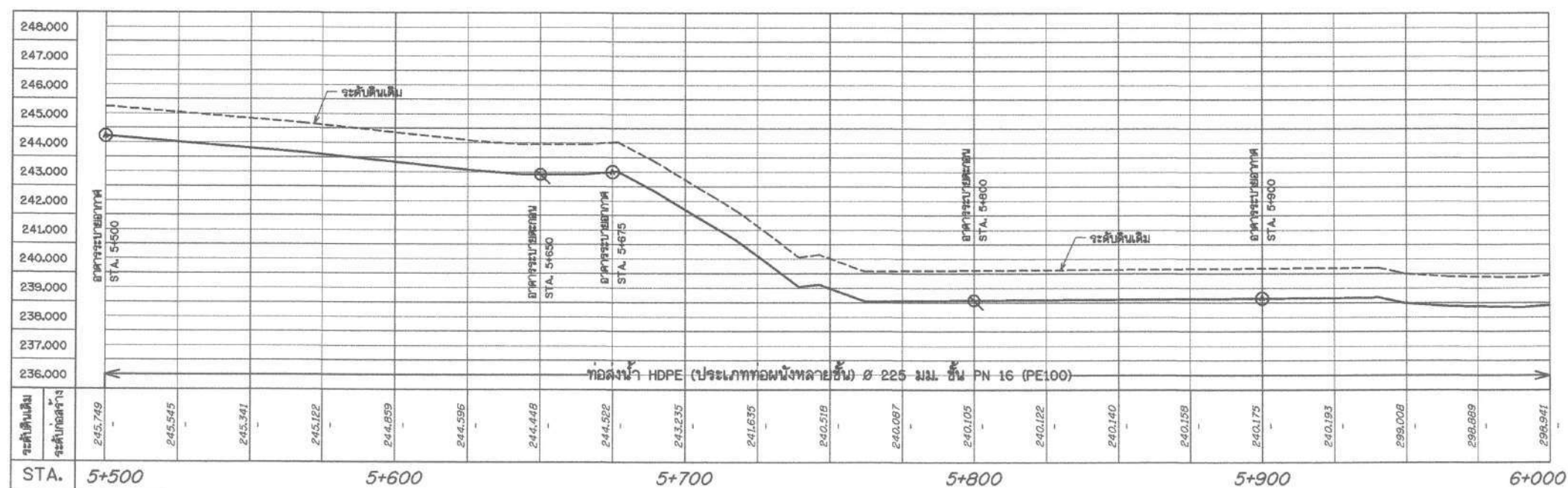
รูปตัดตามแนวสายระบบกระจายน้ำ สาย RMP1 STA. 5+500 - 6+000
