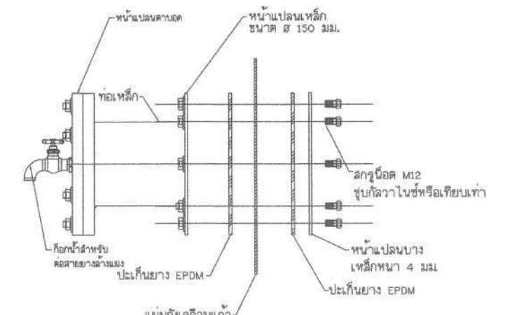
แบบขยายหน้าแปลนดาบอด scale NTC.
