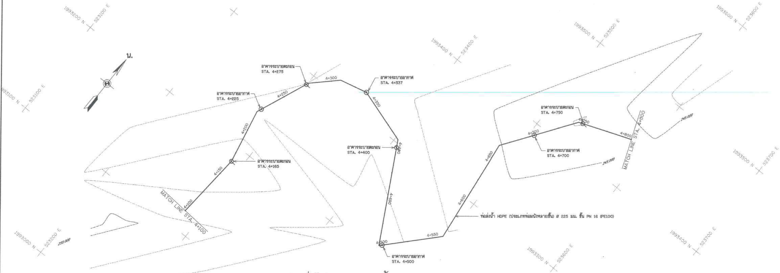
แปลนทั่วไประบบกระจายน้ำ สาย RMP1 STA. 4+100 - 4+800
