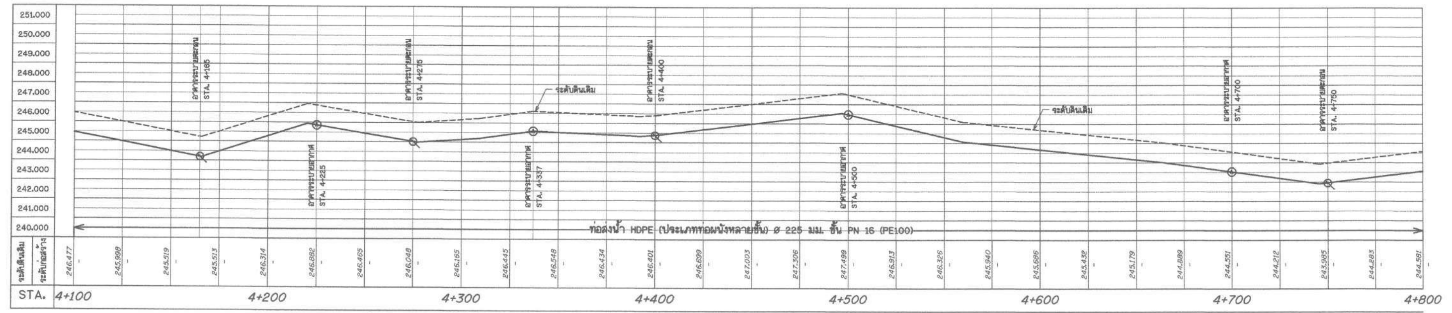
รูปตัดตามแนวยาวระบบกระจายน้ำ สาย RMP1 STA. 4+100 - 4+800
