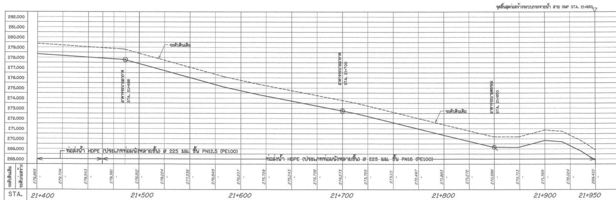
แปลนทั่วไประบบกระจายน้ำ สาย RMP STA. 21+400 - 21+950 มาตราส่วน 1:1,000
