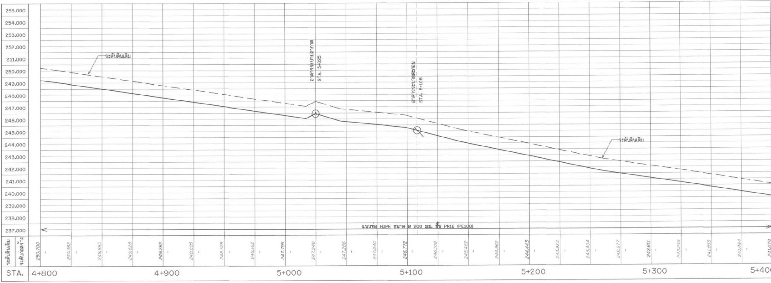
รูปตัดตามแนวยาว กม. 0+000 STA. 4+800 - 5+400 มาตรฐาน 1:1,000 แนวตั้ง 1:100
