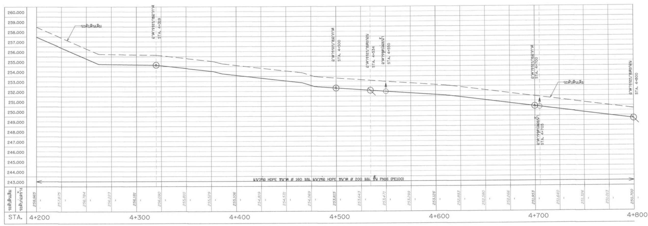
รูปตัดตามแนวยาว กม. 0+000 STA. 4+200 - 4+800 มาตรฐาน 1:1,000 แนวตั้ง 1:100
