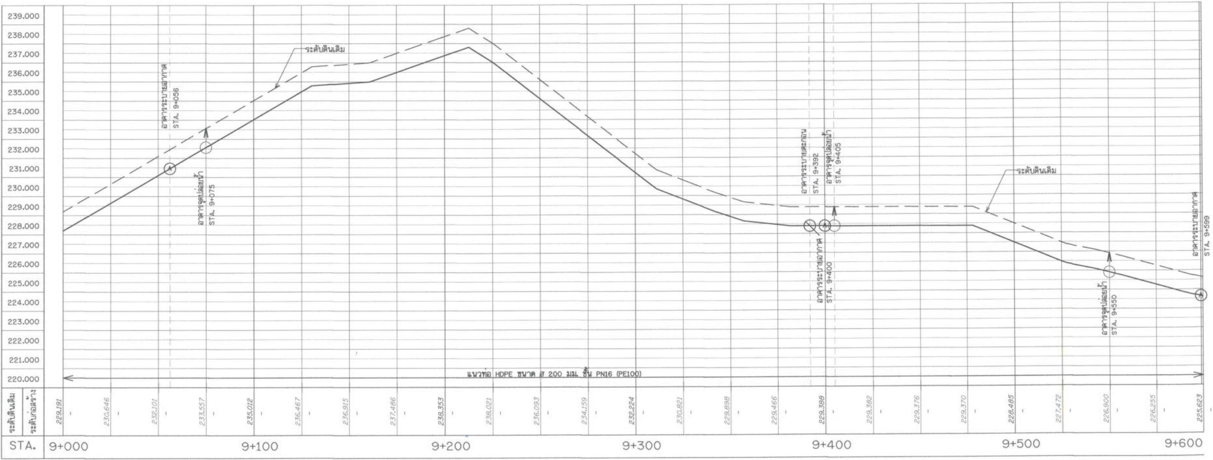
รูปตัดตามแนวยาว กม. 0+000 STA. 9+000 - 9+600 มาตรฐาน 1:1,000 แนวตั้ง 1:100
