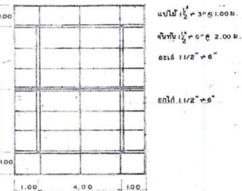
แปลนโครงหลังคา 18100
