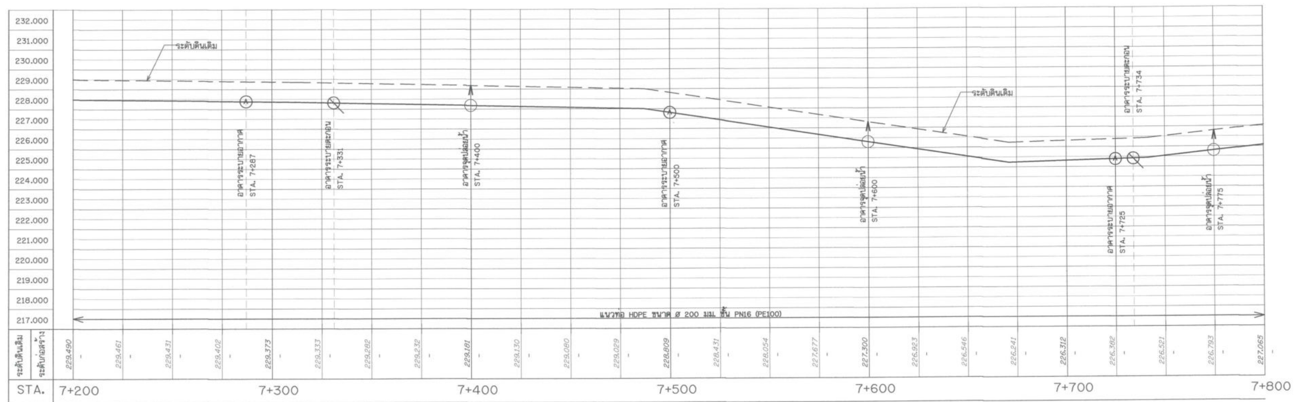
รูปตัดตามแนวยาว กม. 0+000 STA. 7+200 - 7+800 มาตราส่วน 1:1,000 แนวตั้ง 1:100
