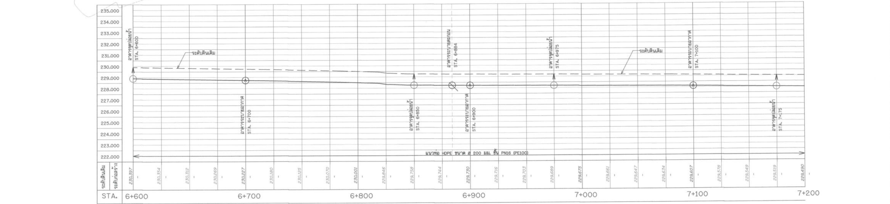
รูปตัดตามแนวยาว กม. 0+000 STA. 6+600 - 7+200 มาตรฐาน 1:1,000
