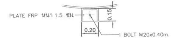
แบบขยาย ขายึดถัง SCALE 1 : 25
