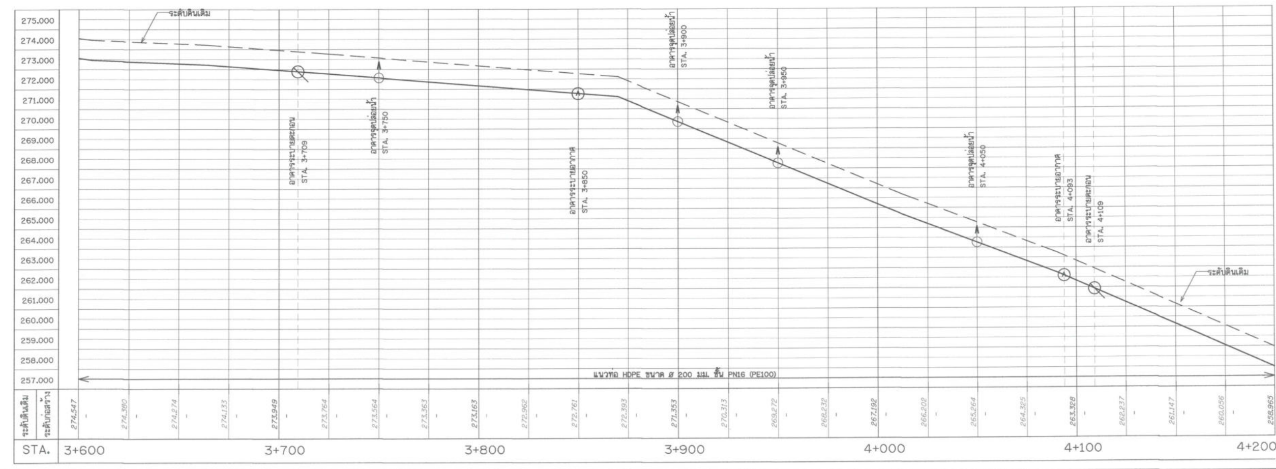
รูปตัดตามแนวยาว กม. 0+000 STA. 3+600 - 4+200 , กม. 20+000 STA. 20+000 - 20+148 มาตราส่วน 1:1,000 แนวตั้ง 1:100
