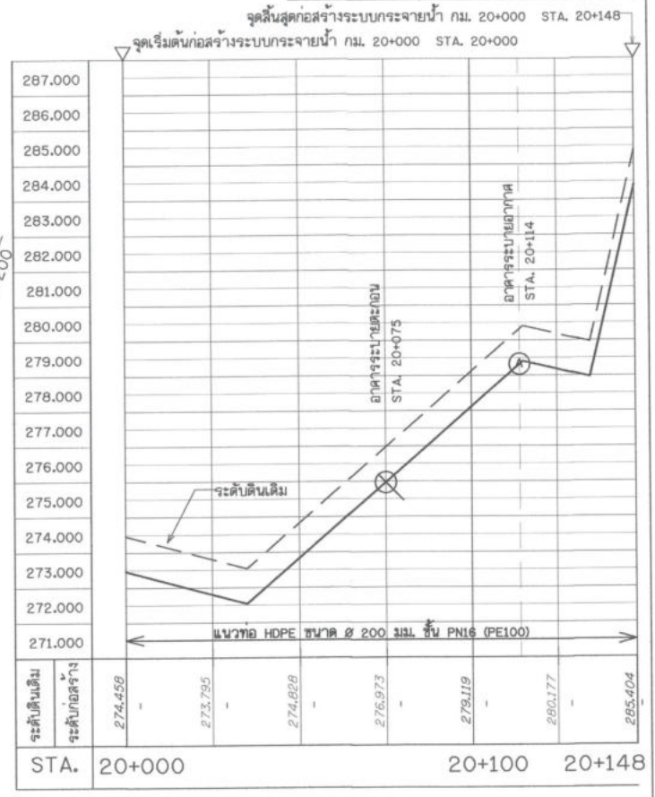
รูปตัดตามแนวยาว กม. 0+000 STA. 3+600 - 4+200 , กม. 20+000 STA. 20+000 - 20+148 มาตราส่วน 1:1,000 แนวตั้ง 1:100
