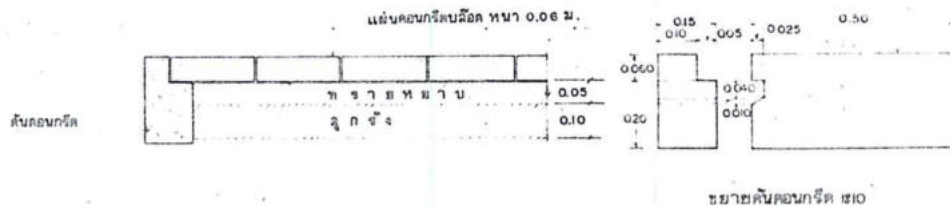
รูปขยายการเรียง I-SECTION 1:10
