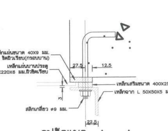
รูปตัดแนว A - A มาตราส่วน 1:2
