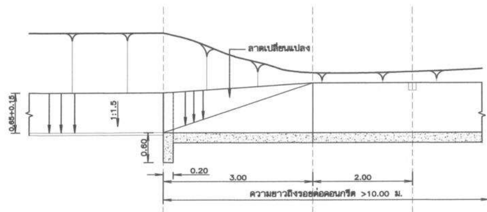
รูปตัดแนว ก - ก
