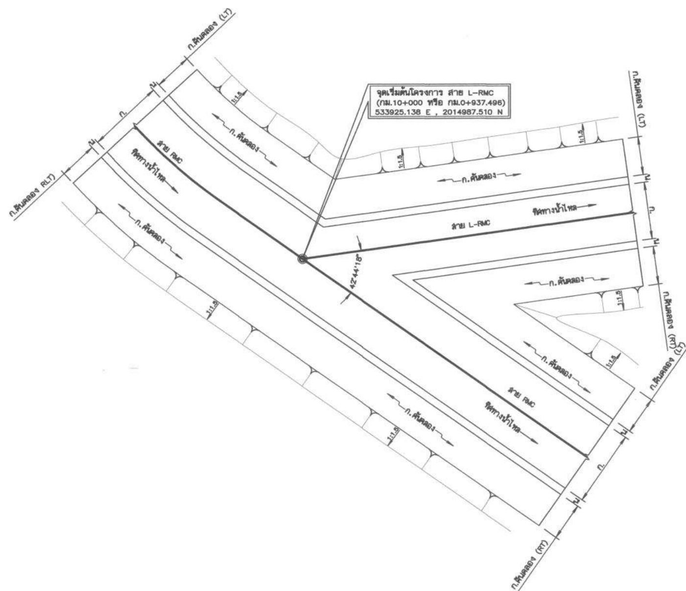
แปลนแสดงจุดแยกคลองส่งน้ำ สาย R-RMC
