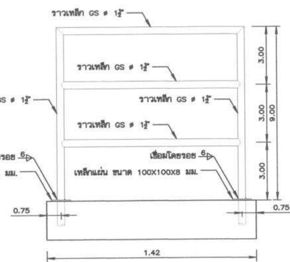
ขยายราวกันตก มาตราส่วน 1:10
