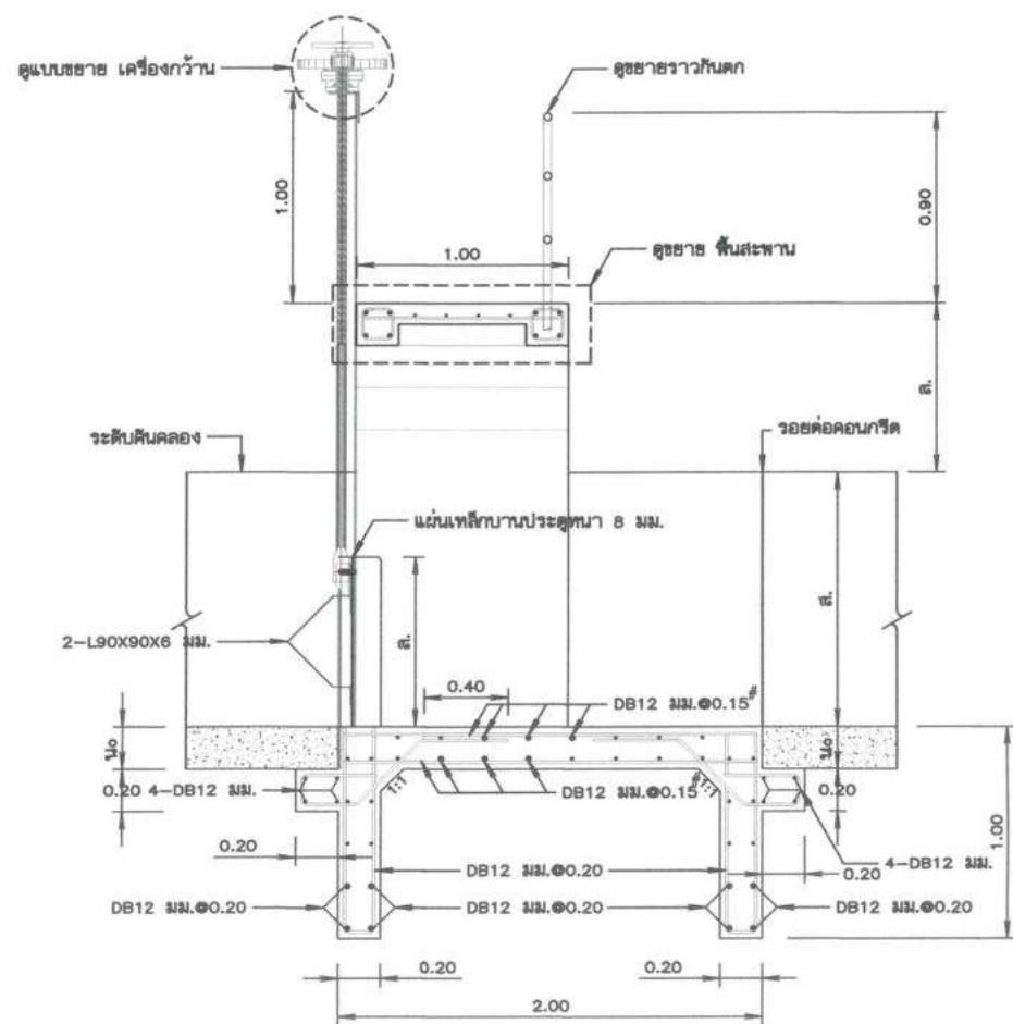
รูปตัดแนว ก - ก มาตราส่วน 1:20
