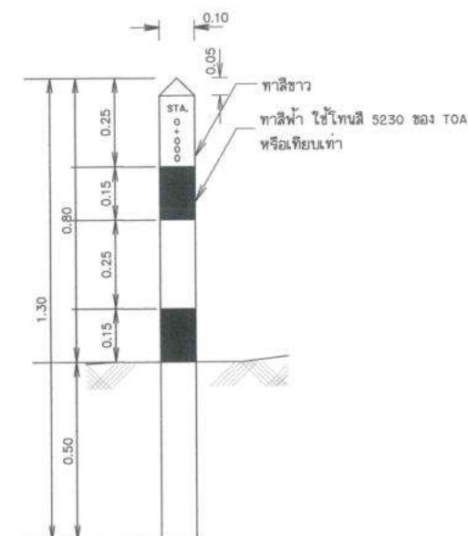
แสดงสัดส่วนหลักบอกแนวท่อ
