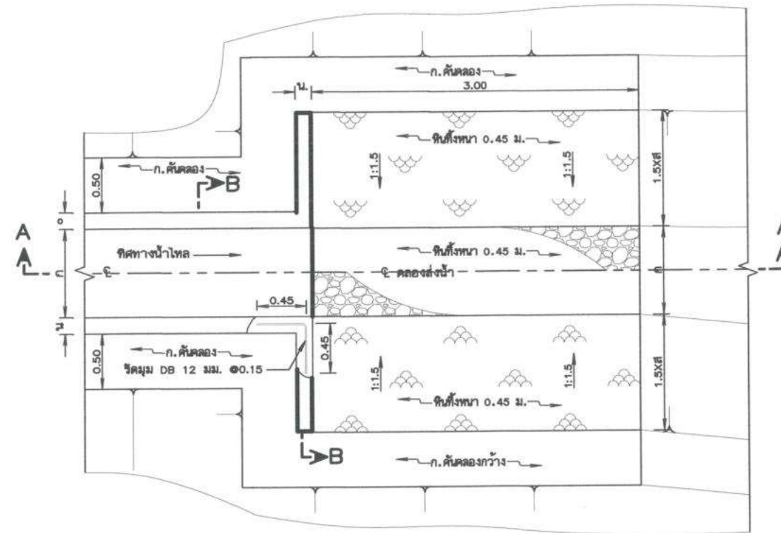
แปลนจุดสิ้นสุดคลองส่งน้ำ
