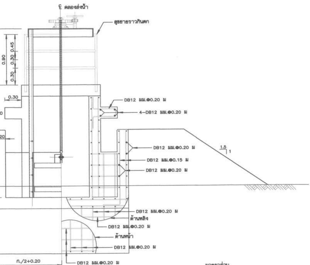
รูปตัดแนว ข - ข มาตราส่วน 1:20
