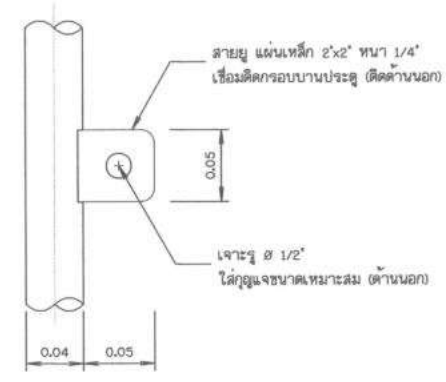
แบบขยายสายยู
