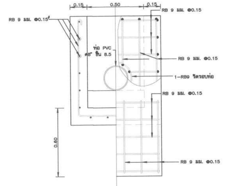
รูปตัดแนว ข - ข มาตราส่วน 1:10
