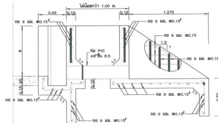
รูปตัดแสดงเสริมเหล็ก INLET-OUTLET TRANSITION มาตราส่วน 1:15
