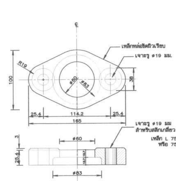
แบบขยายแผ่นปิด มาตราส่วน 1:2
