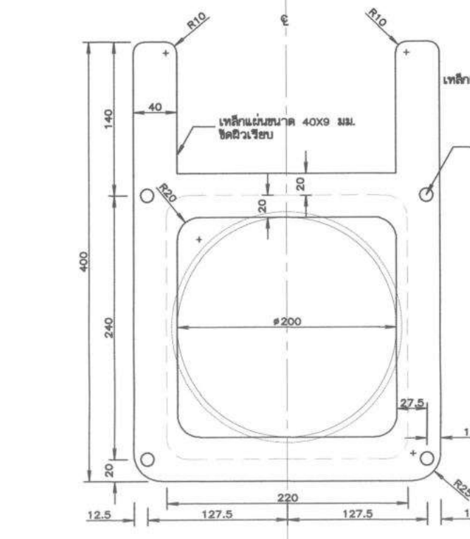
ขยายกรอบบาน มาตราส่วน 1:2.5
