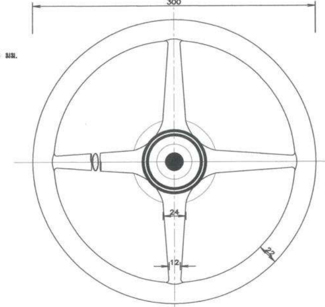
แบบล้อมือหมุน มาตราส่วน 1:2
