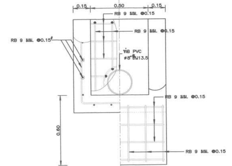
รูปตัดแนว ง - ง มาตราส่วน 1:10
