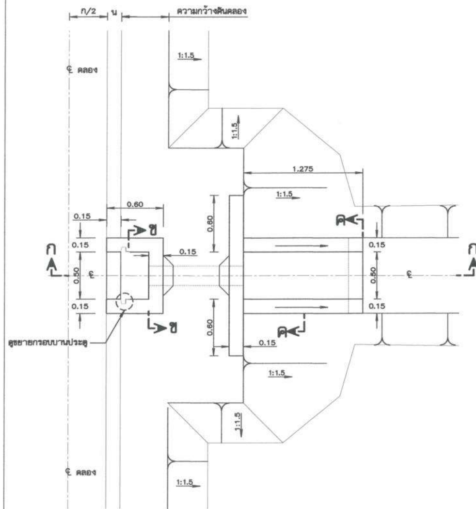
แผนอาคารท่อส่งน้ำเข้านา มาตราส่วน 1:20
