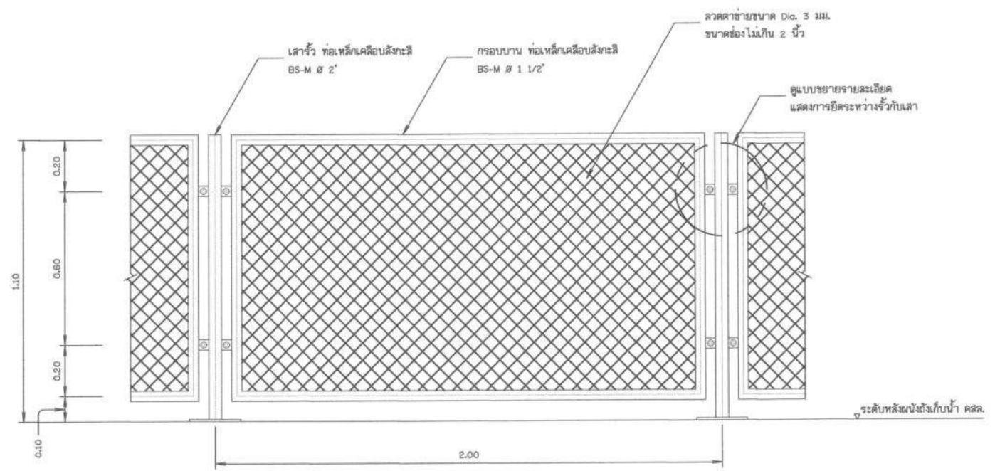
แบบขยายราวกันตก
