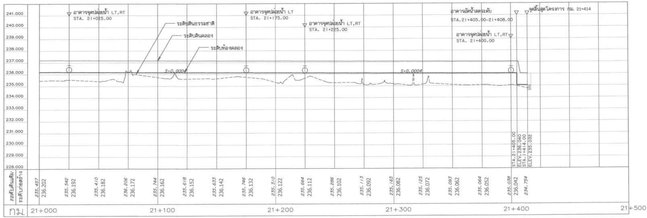
รูปตัดตามแนวยาว สาย R-RMC มาตราส่วน 1:1,000 แนวยาว 1:100
