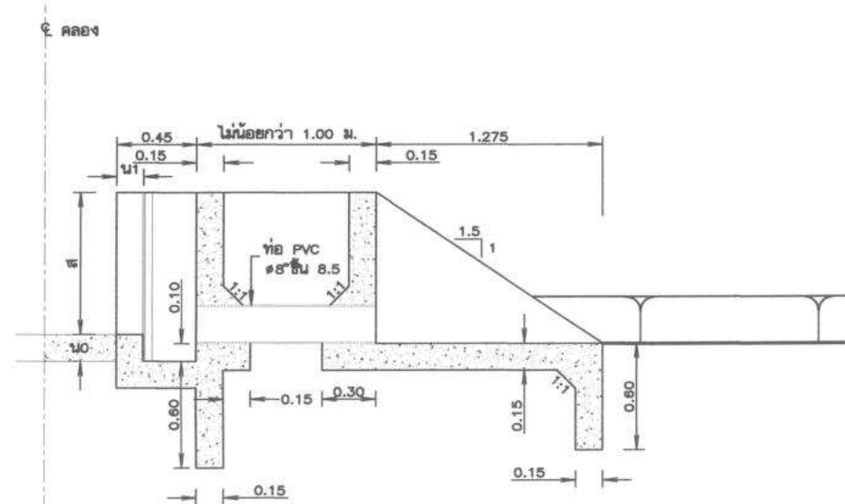
รูปตัดแนว ก - ก มาตราส่วน 1:20
