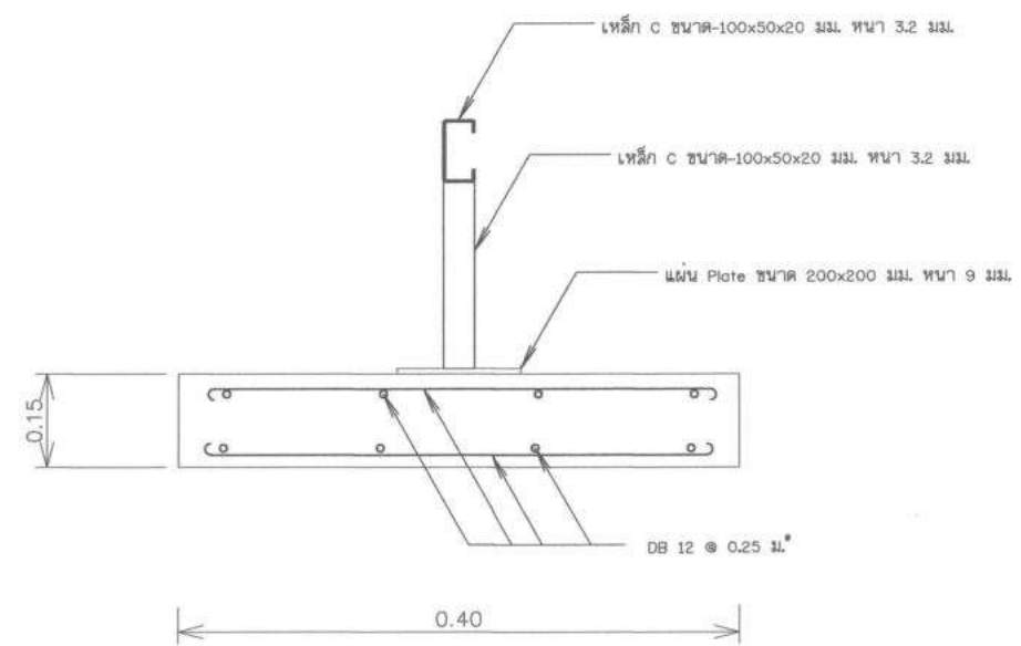
รูปตัดโครงสร้างรับท่อ ไม่แสดงมาตราส่วน
