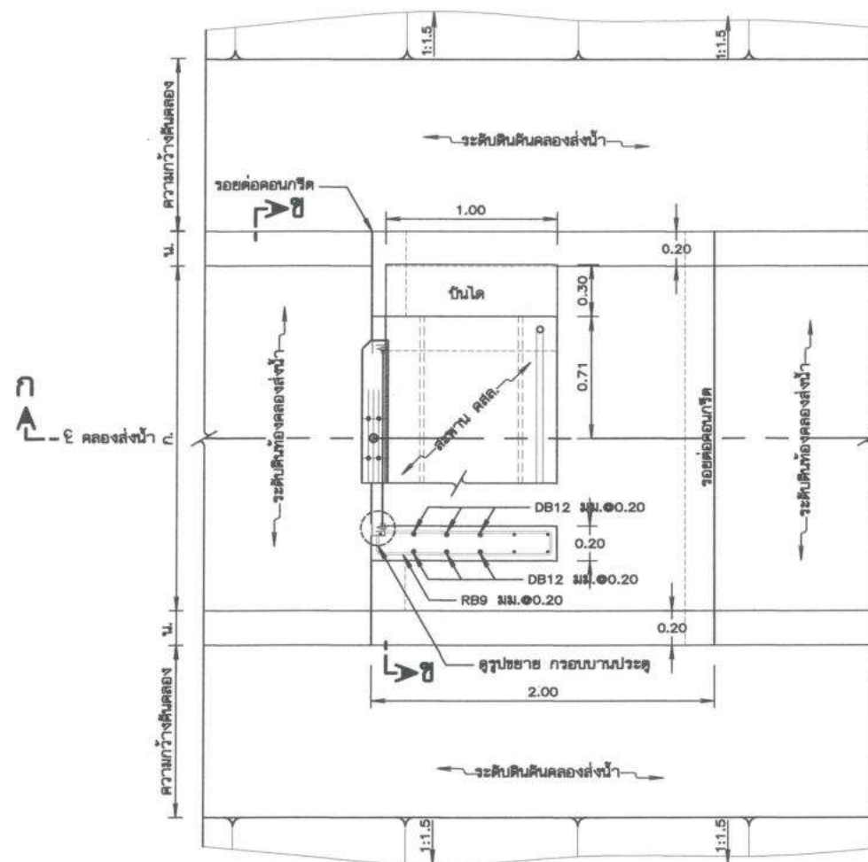
แปลนอาคารยึดน้ำ มาตราส่วน 1:20
