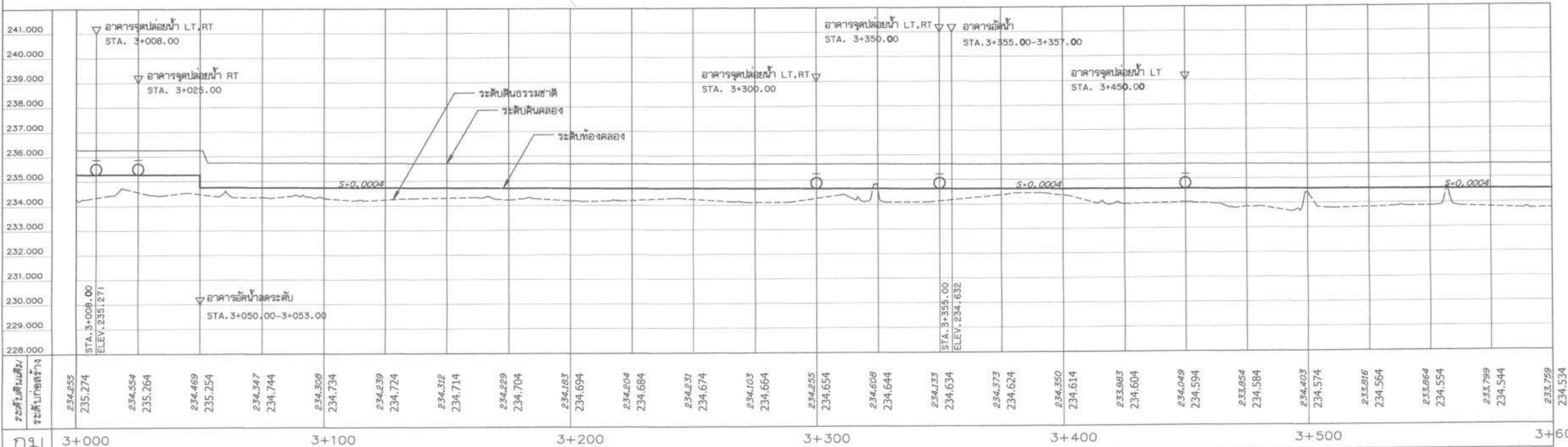
รูปตัดตามแนวยาว สาย RMC มาตราส่วน 1:1,000 แนวตั้ง 1:100
