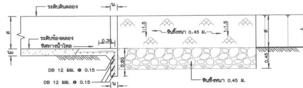
รูปตัดแนว A - A
