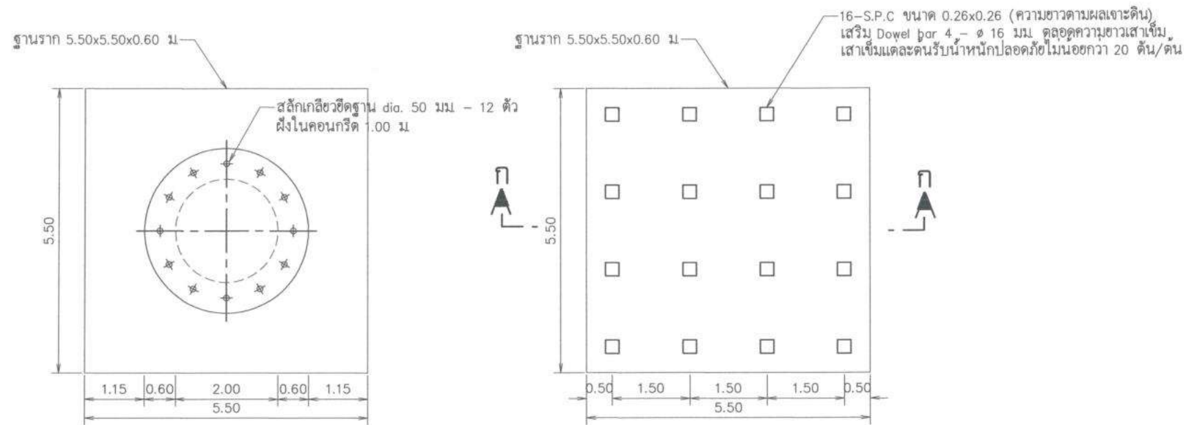
แปลนฐานรากหอดังสูง (แบบเสาเข็ม)
