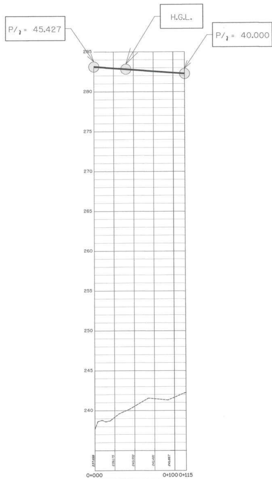
รูปตัดตามแนวยาวแสดง H.G.L. สาย RMP STA. 0+000 - 0+115 ไม้เล็งวัดขนาดจริง
