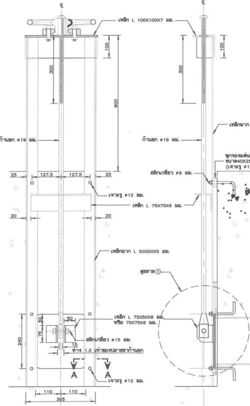
บาน ก้านยกและโครงยก มาตราส่วน 1:5 แสดงการติดตั้ง มาตราส่วน 1:5
