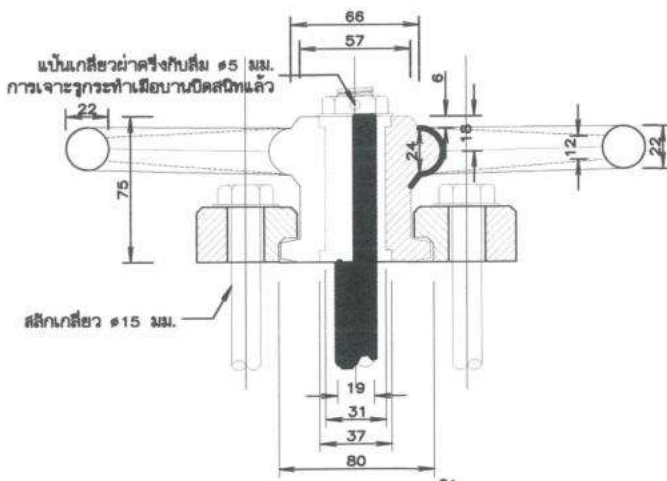
แสดงการติดตั้ง มาตราส่วน 1:2
