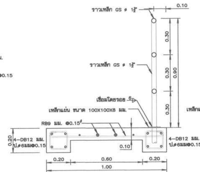
รูปตัดแนว A - A มาตราส่วน 1:10
