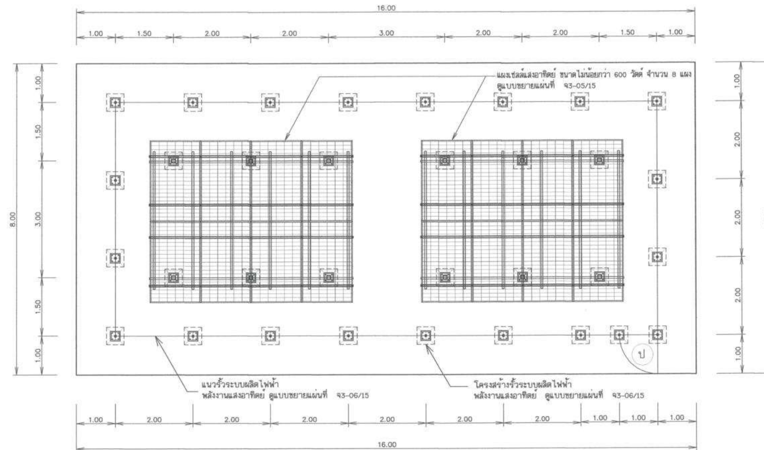
แปลนการติดตั้งแผงเซลล์แสงอาทิตย์ พร้อมรั้ว
