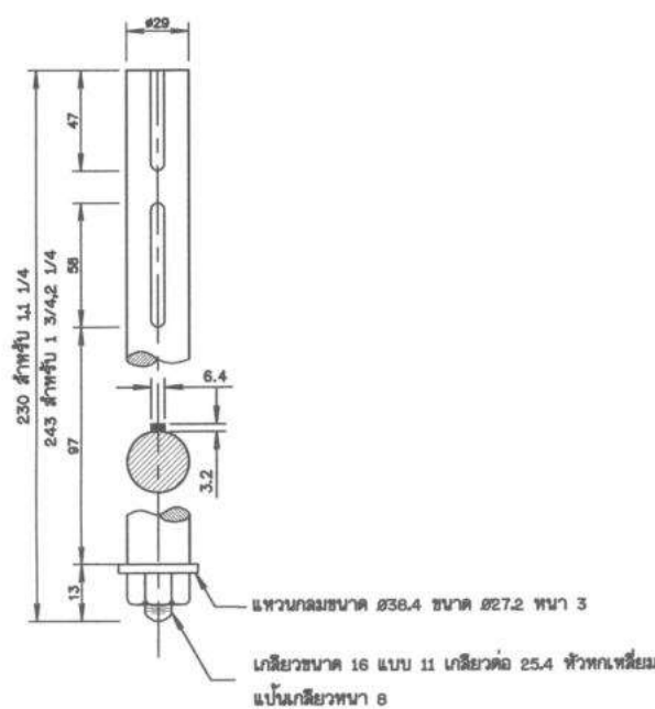
เพลาลูกเบี้ยว มาตราส่วน 1:2
