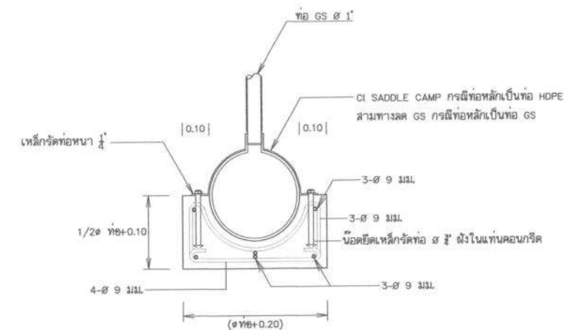
รูปตัดขยาย '1'
