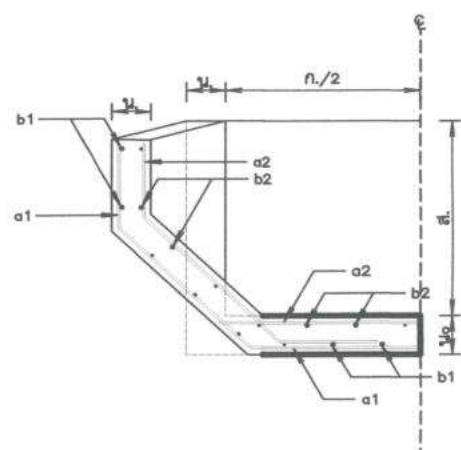
รูปตัดแนว y - y
