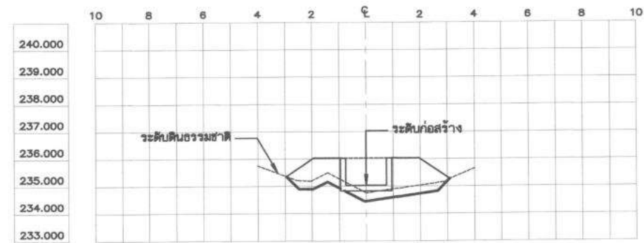
กม. 21+414 จุดสิ้นสุดโครงการ สาย R-RMC
