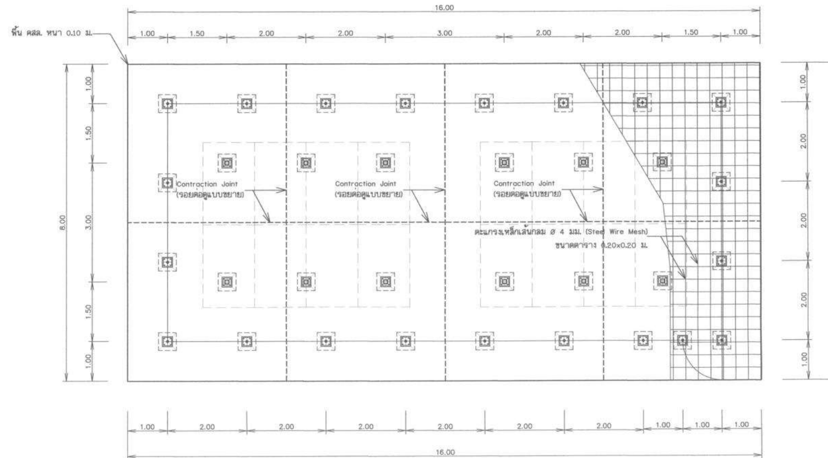
แปลนขยายรอยต่อพื้นคอนกรีต
