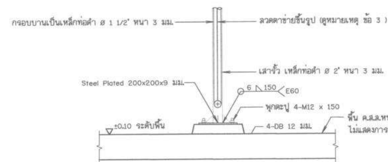
แบบขยายรายละเอียดแสดงการยึด ไม่แสดงมาตราส่วน
