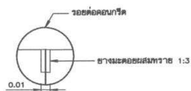
แปลนขยาย พื้นสะพาน มาตราส่วน 1:20
