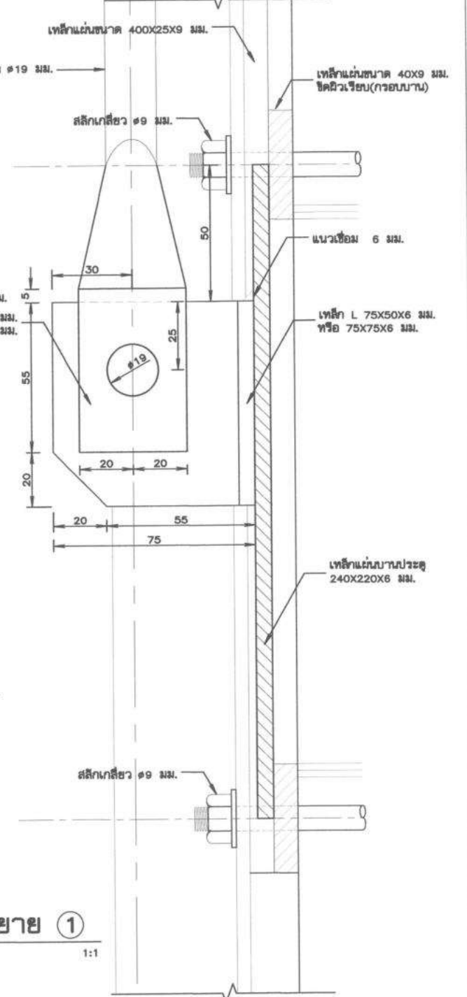
แบบขยาย 1 มาตราส่วน 1:1 มาตราส่วน 1:1 0 20.00 40.00 60.00 80.00 100.00 มม. มาตราส่วน 1:2 0 50.00 100.00 150.00 200.00 มม. มาตราส่วน 1:2.5 0 50.00 100.00 150.00 200.00 250.00 มม. มาตราส่วน 1:5 0 100.00 200.00 300.00 400.00 500.00 มม.
