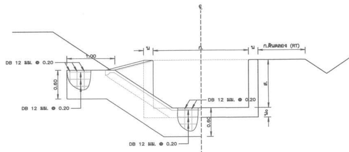
รูปตัดแนว x - x
