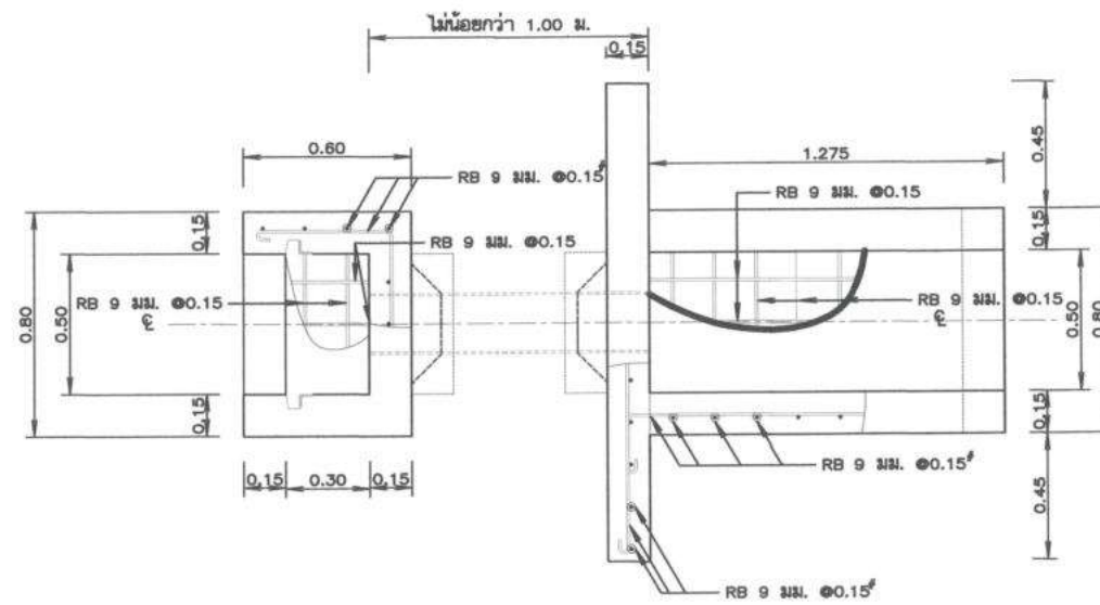
แปลนแสดงสัดส่วน INLET-OUTLET TRANSITION มาตราส่วน 1:15
