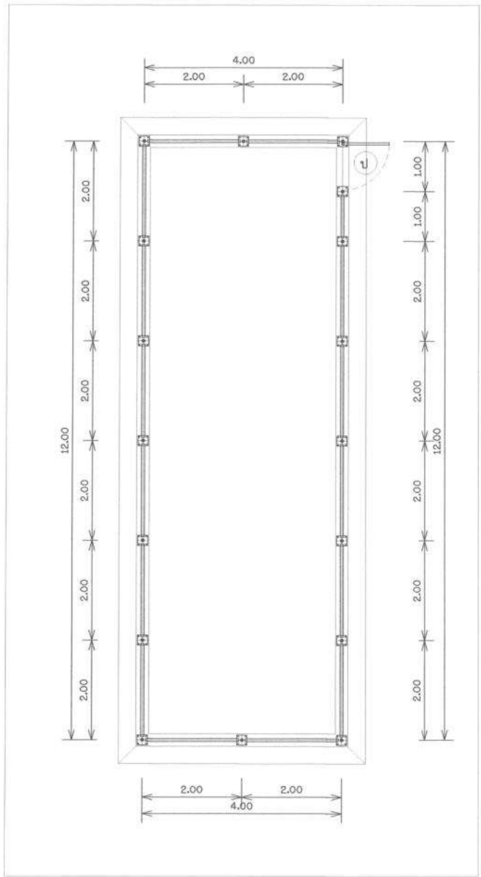
แบบแปลนรื้อลวดตาข่าย (ถังเก็บน้ำ)
