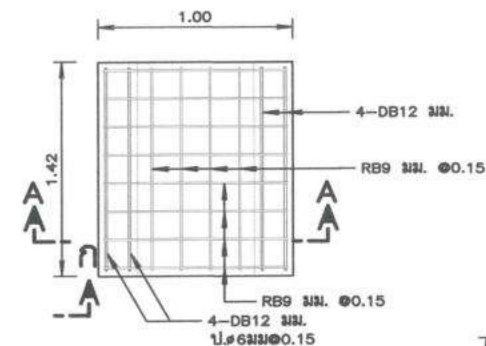
แปลนขยาย พื้นสะพาน มาตราส่วน 1:20
