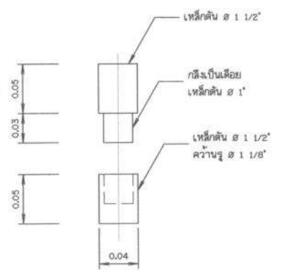
แบบขยายบานพับบูทเหล็ก
