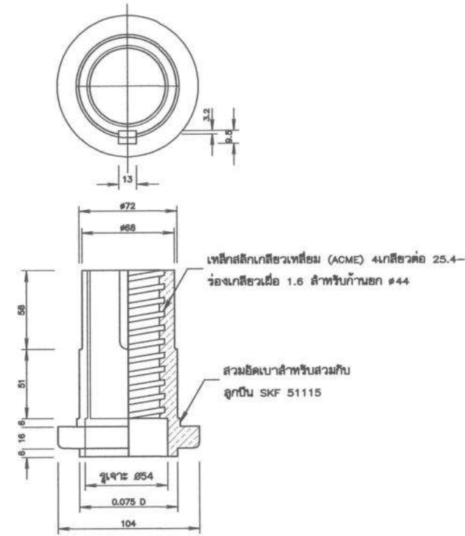
ปั๊มเกลียวยก บรอนซ์ 6
