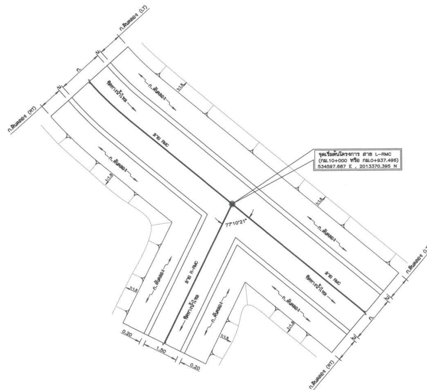
แปลนแสดงจุดแยกคลองส่งน้ำ สาย L-RMC
