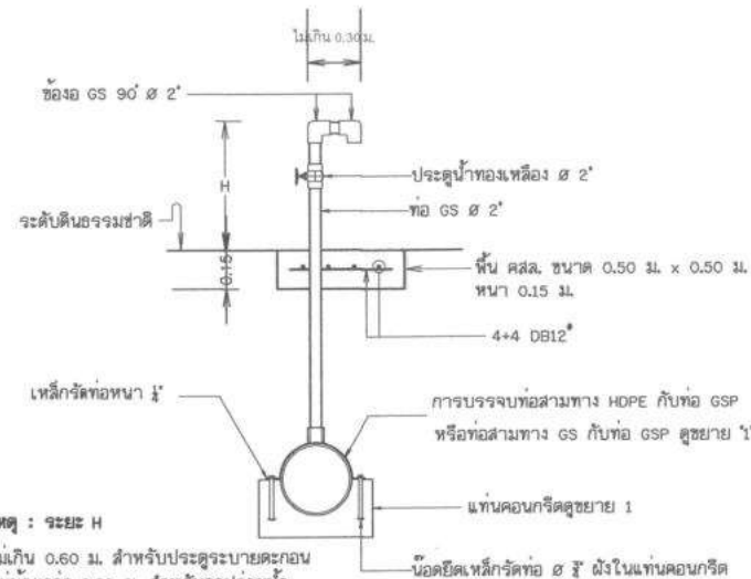
รูปตัดอาคารประตูระบายตะกอน
